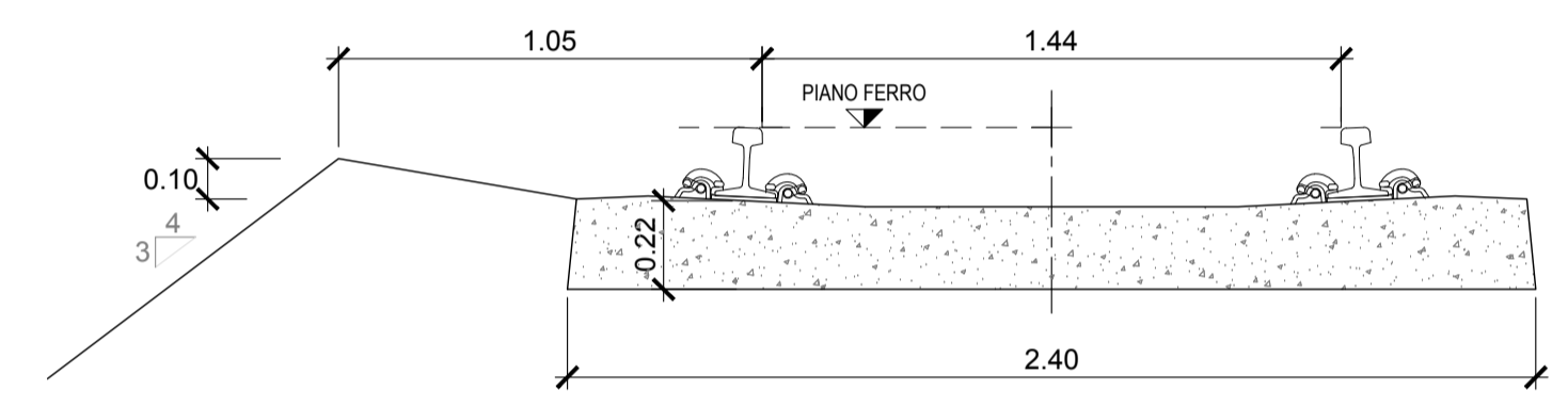
DETTAGLIO 1 - scala 1:20
