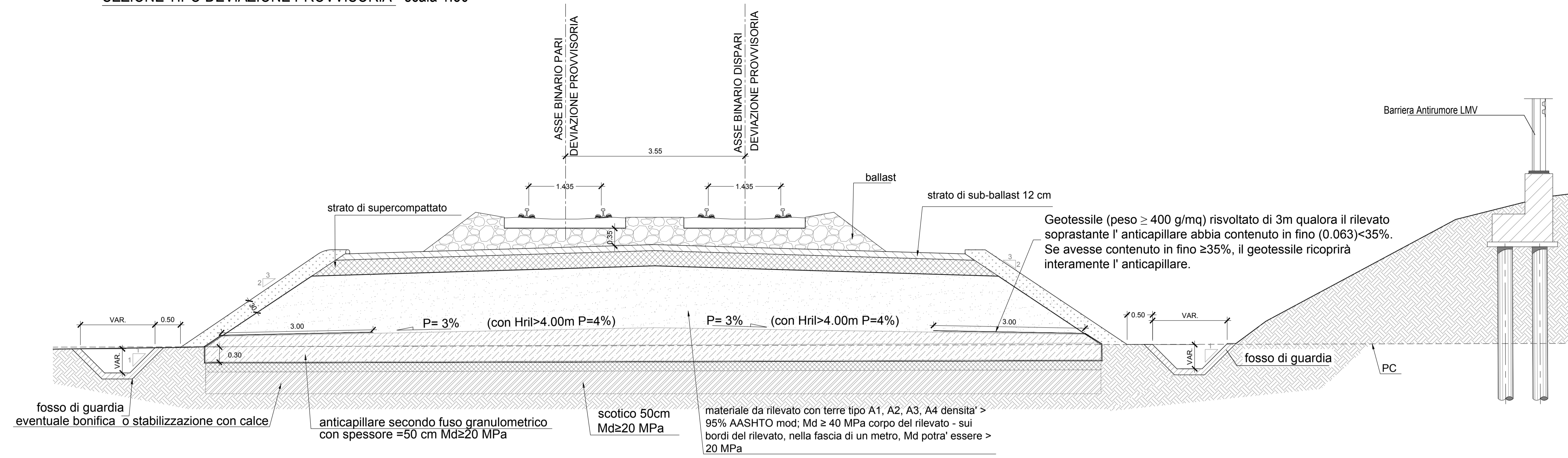
SEZIONE TIPO DEVIAZIONE PROVVISORIA (da pk 0+000 a pk 0+300) - scala 1:50
