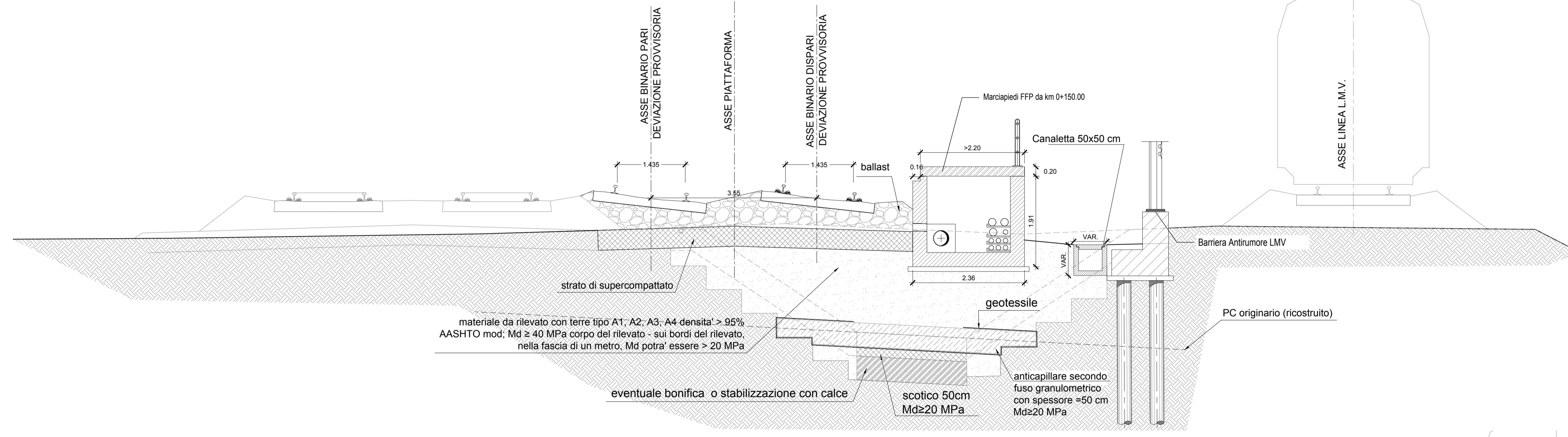
SEZIONE TIPO DEVIAZIONE PROVVISORIA (da pk 0+300 a pk 0+450) - scala 1:50
