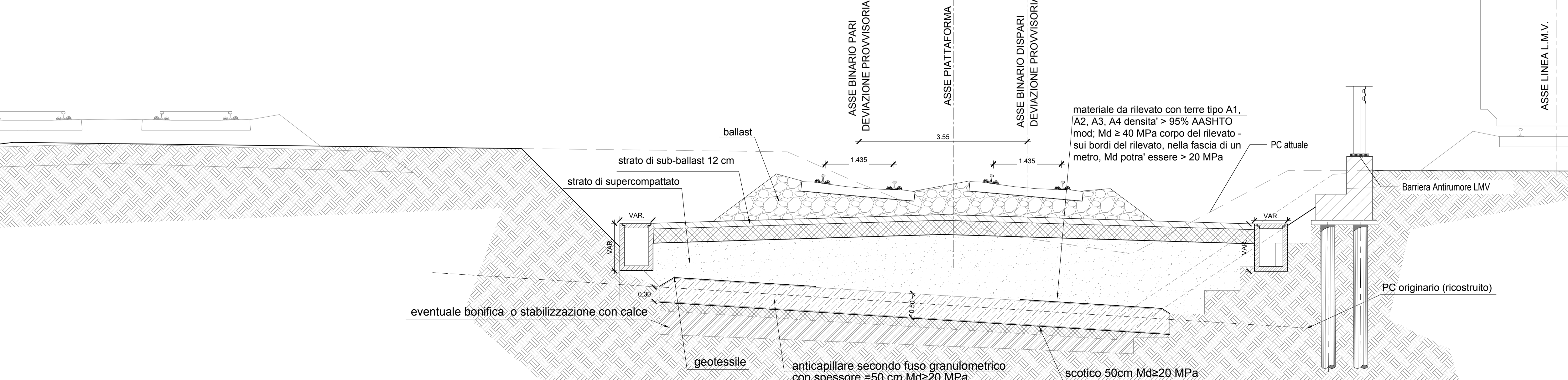
SEZIONE TIPO DEVIAZIONE PROVVISORIA (da pk 0+300 a pk 0+450) - scala 1:50
