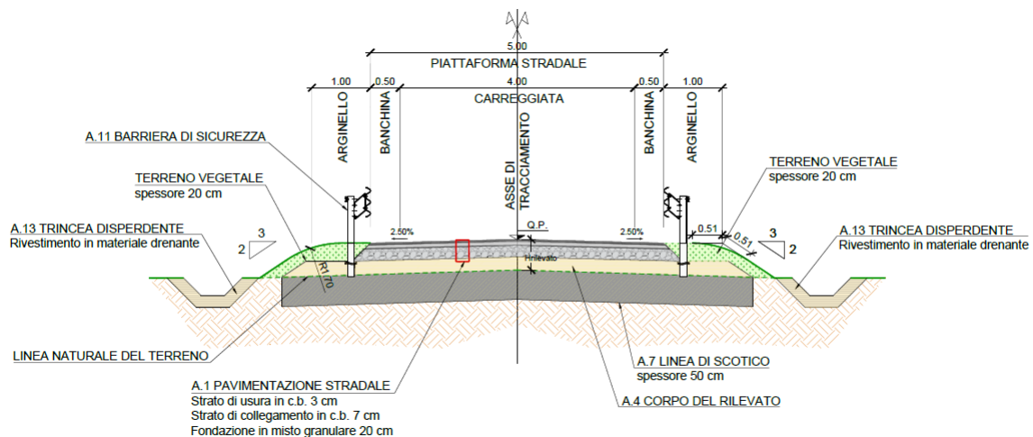
Figura 1: Sezione tipologica
