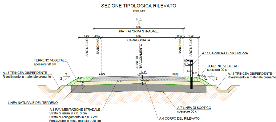
Figura 1: Sezione tipologica
