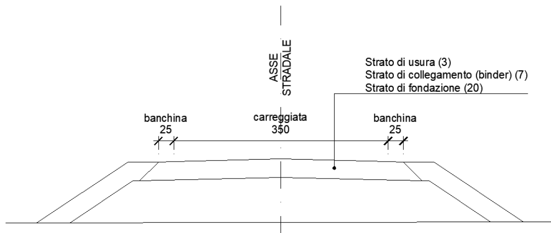
Figura 1: Sezione tipologica
