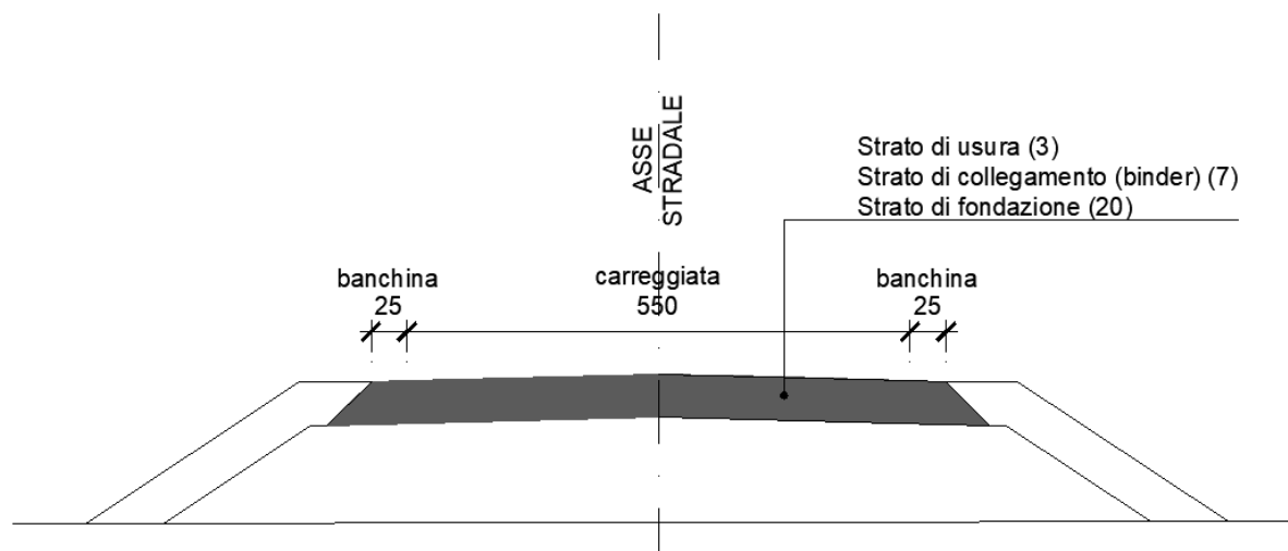
Figura 1: Sezione tipologica
