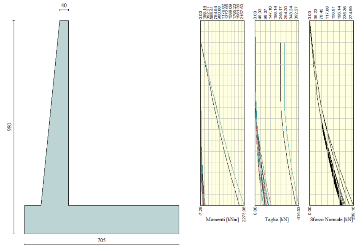
Figura 11: Sollecitazioni agenti sul paramento murario (involuppo SLU)
