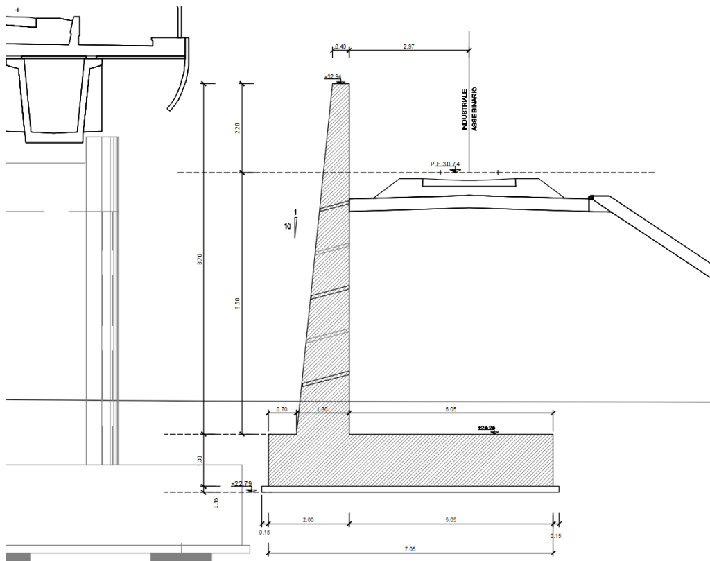
Figura 1: Sezione tipologica TIPO F*
