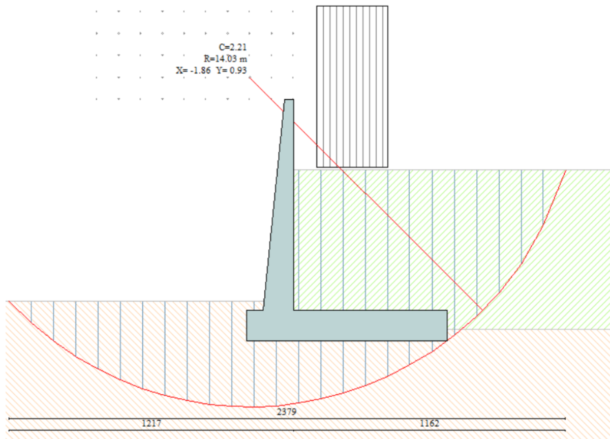
Figura 16: Stabilità globale del sistema terra-muro
