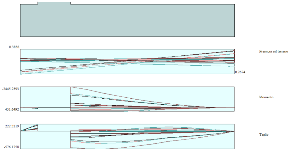
Figura 18: Sollecitazioni agenti in fondazione (involuppo SLU)
