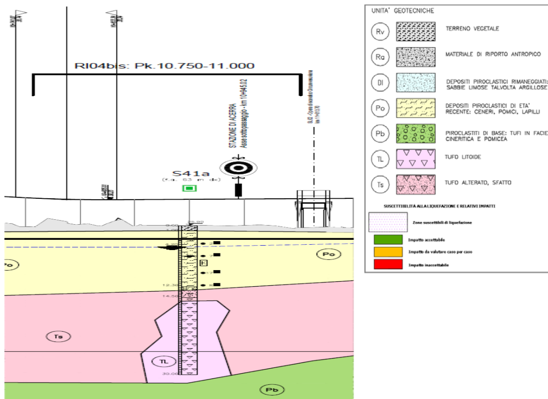
Figura 6 – Stralcio profilo geotecnico
