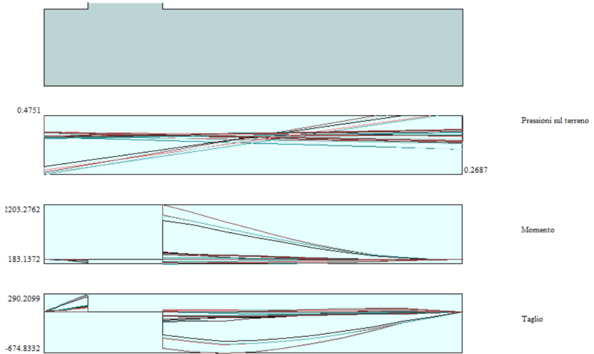
Figura 12: Sollecitazioni agenti in fondazione (inviluppo SLU)
