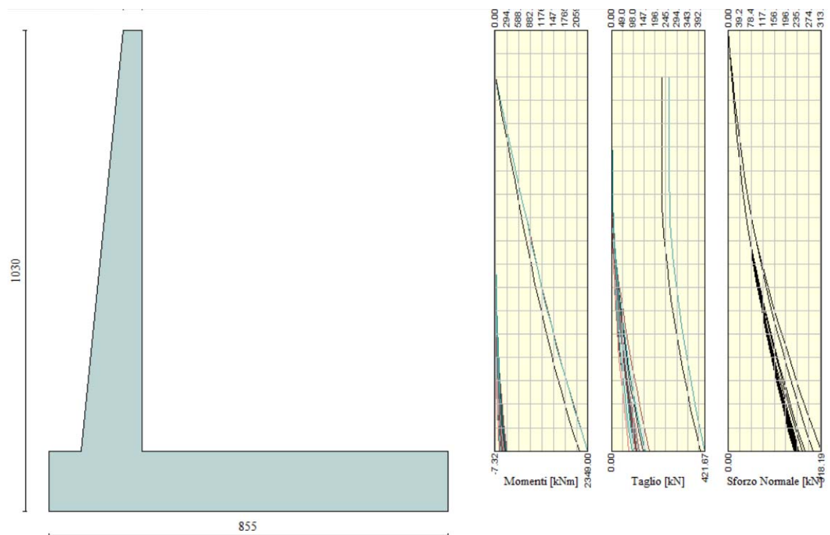
Figura 17: Sollecitazioni agenti sul paramento murario (involuppo SLU)
