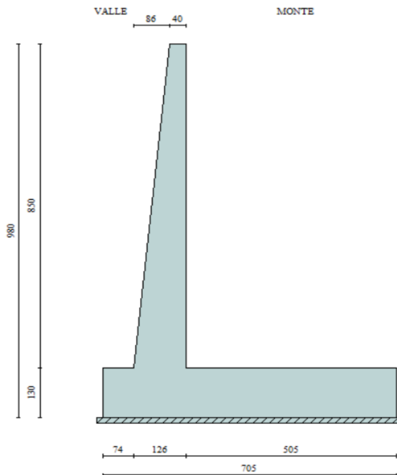
Figura 7: Geometria e dimensioni
