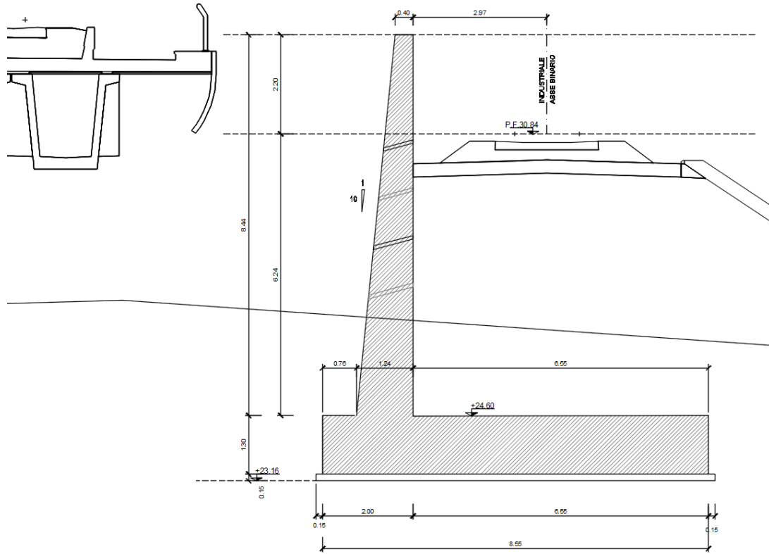
Figura 2: Sezione tipologica TIPO G*
