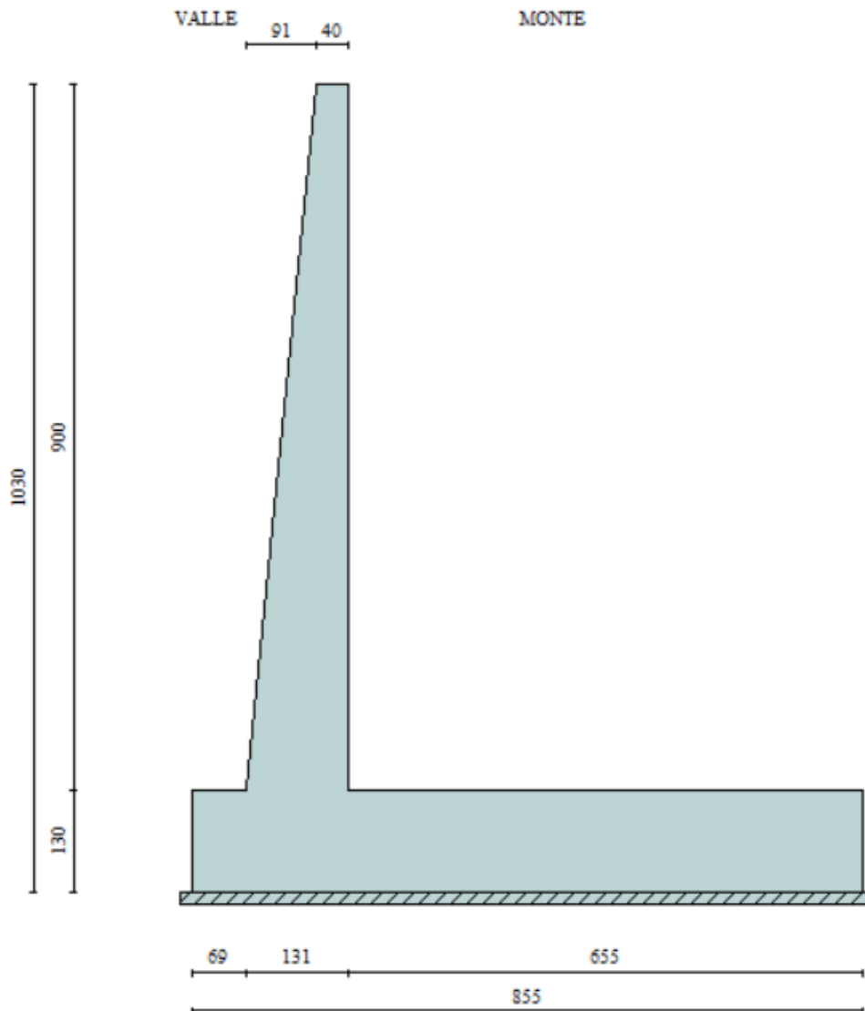
Figura 13: Geometria e dimensioni
