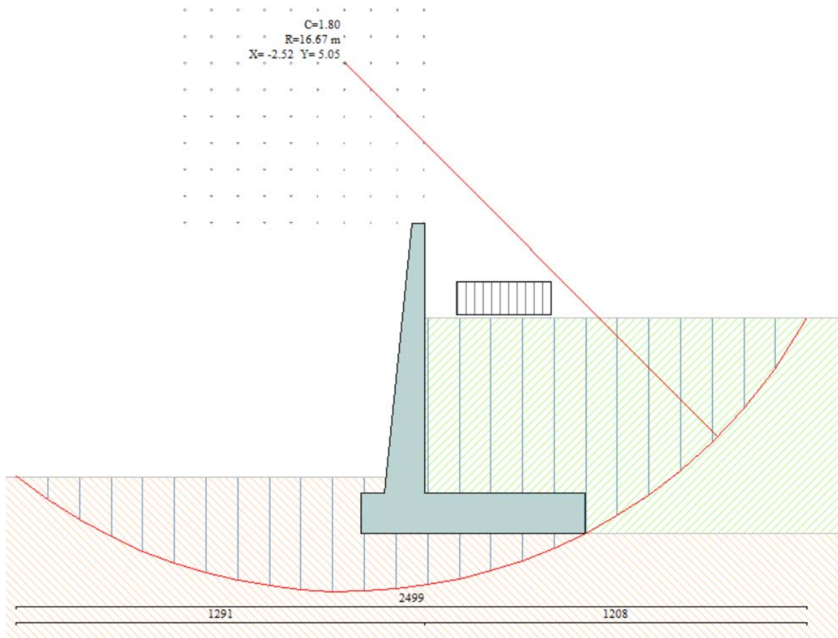
Figura 10: Stabilità globale del sistema terra-muro
