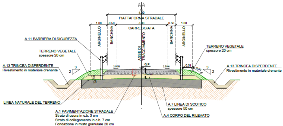
Figura 1: Sezione tipologica
