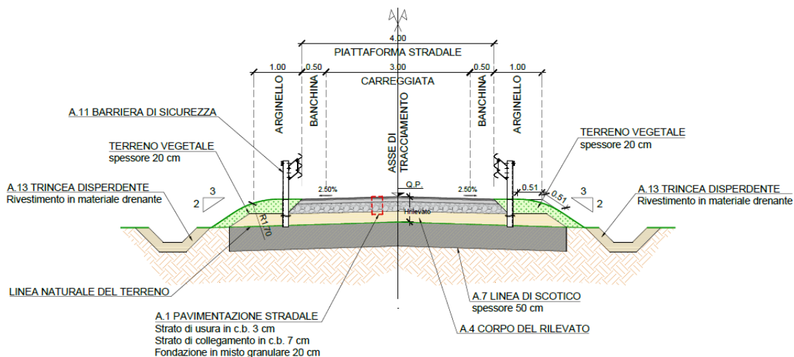
Figura 1: Sezione tipologica
