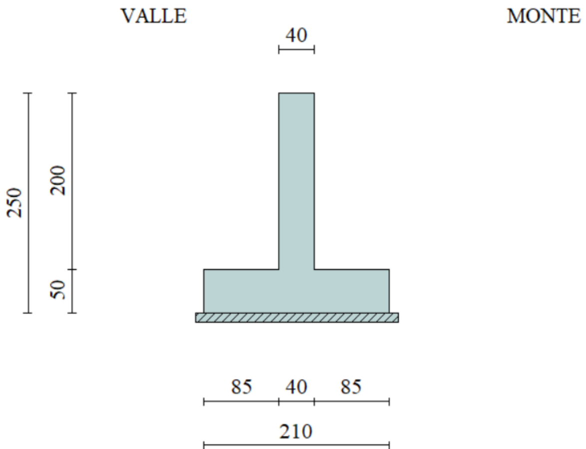
Figura 5: Geometria e dimensioni
