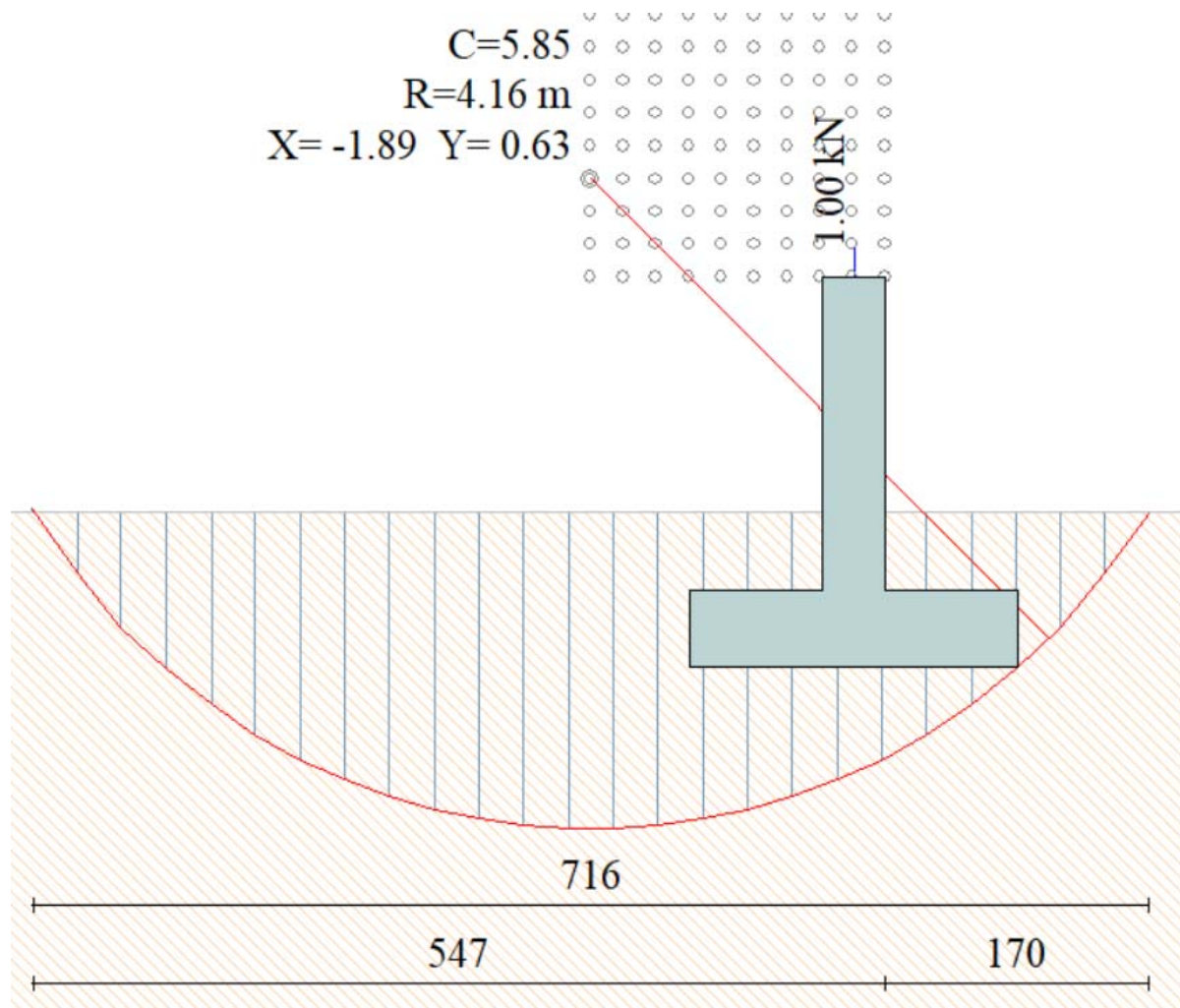
Figura 8: Stabilità globale del sistema terra-muro
