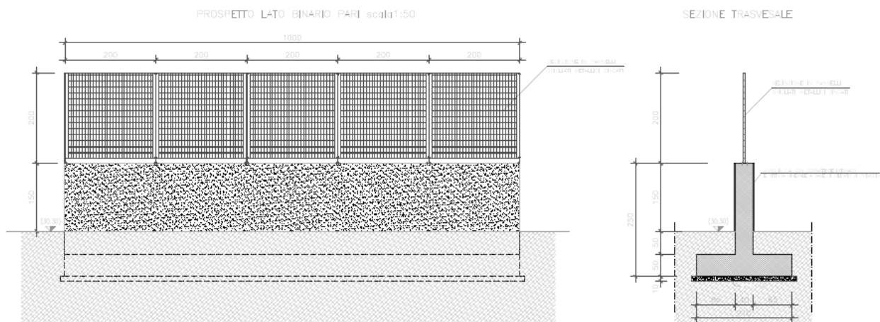
Figura 1: Sezione tipologica
