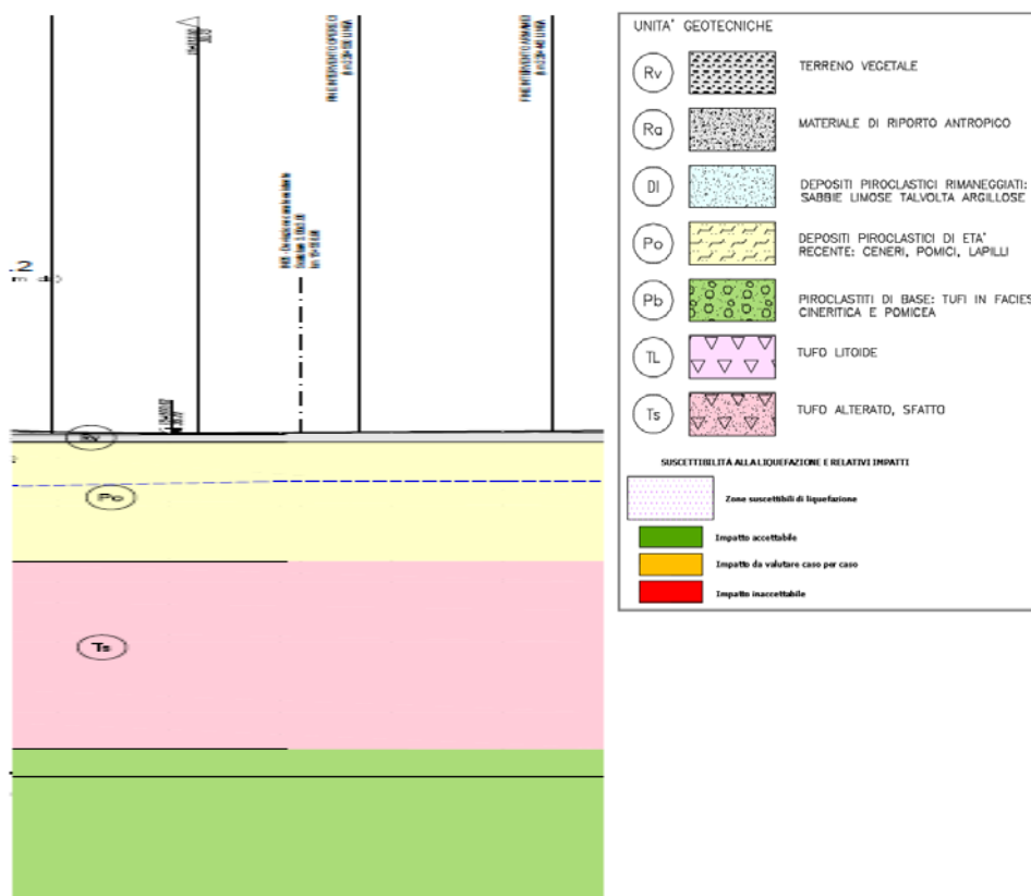
Figura 3 - Stralcio profilo geotecnico
