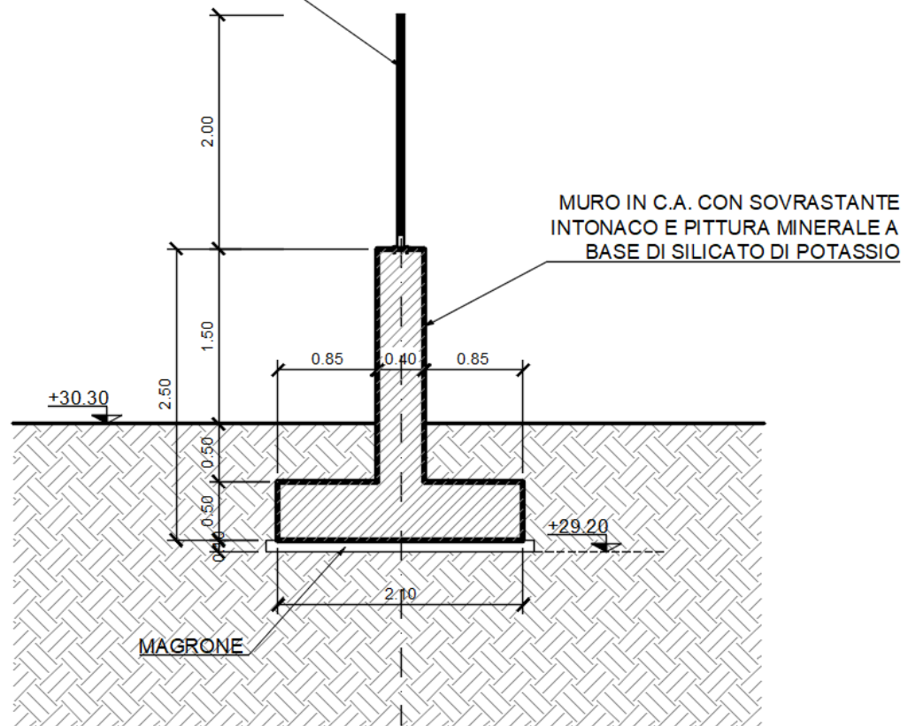
Figura 4: Sezione trasversale tipo
