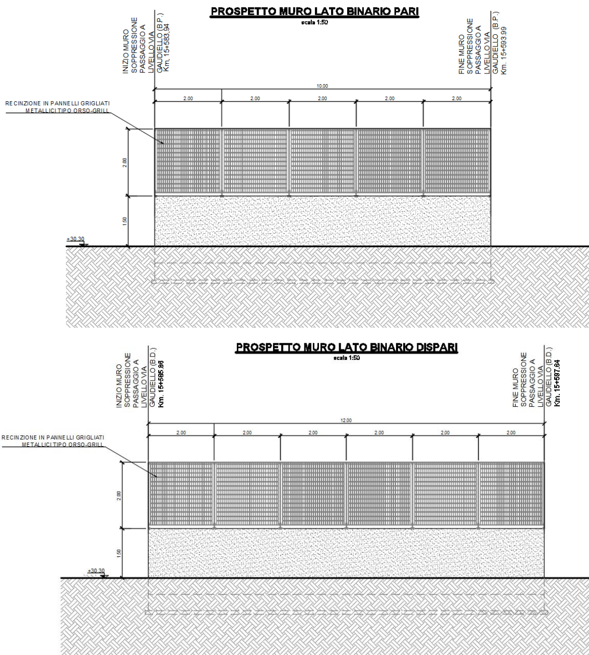
Figura 3 – Profilo longitudinale
