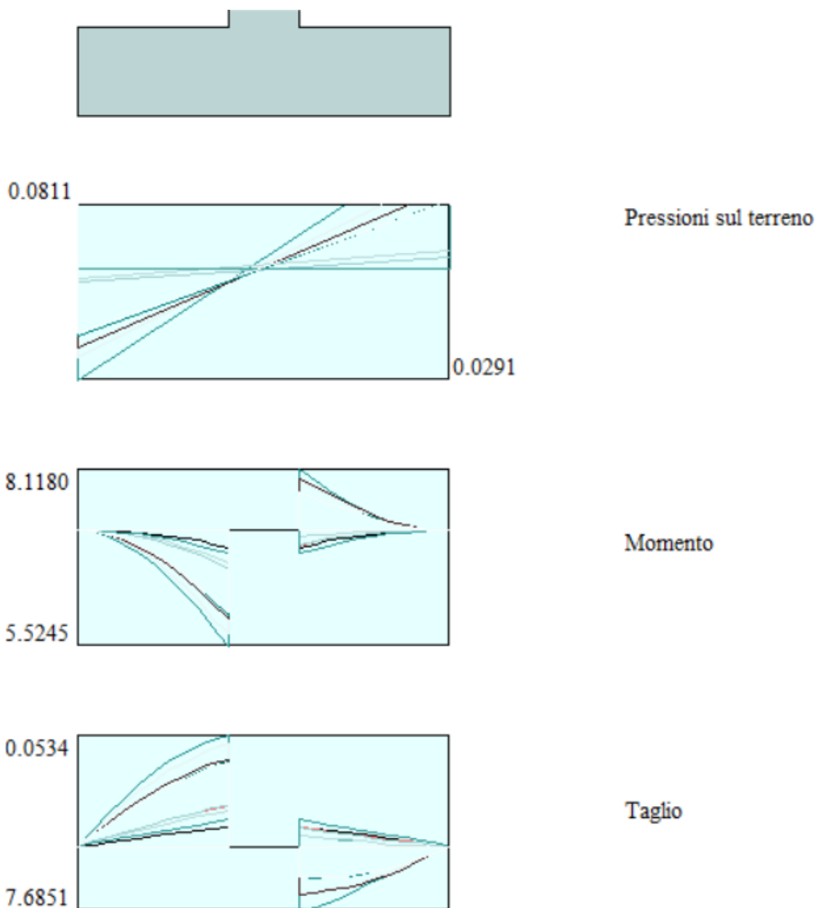
Figura 10: Sollecitazioni agenti in fondazione (inviluppo SLU)
