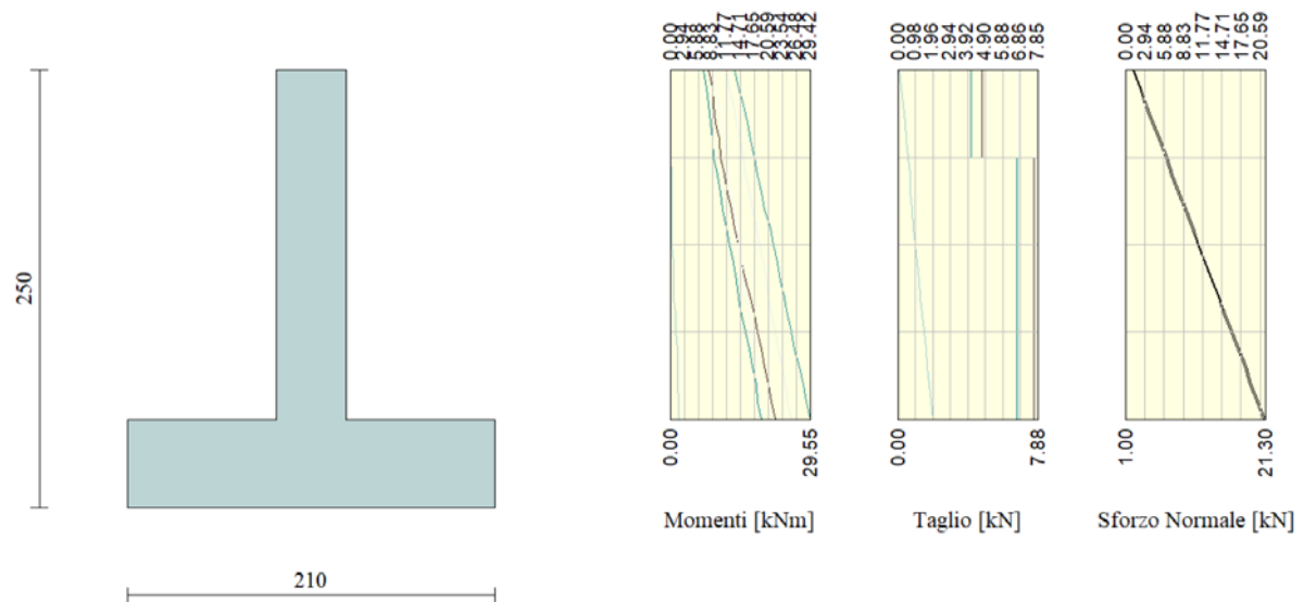
Figura 9: Sollecitazioni agenti sul paramento murario (involuppo SLU)
