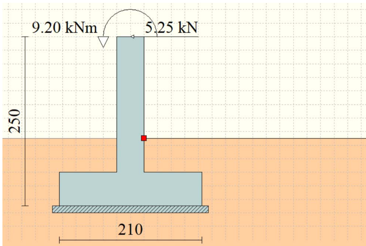
Figura 6: Profilo del terreno
