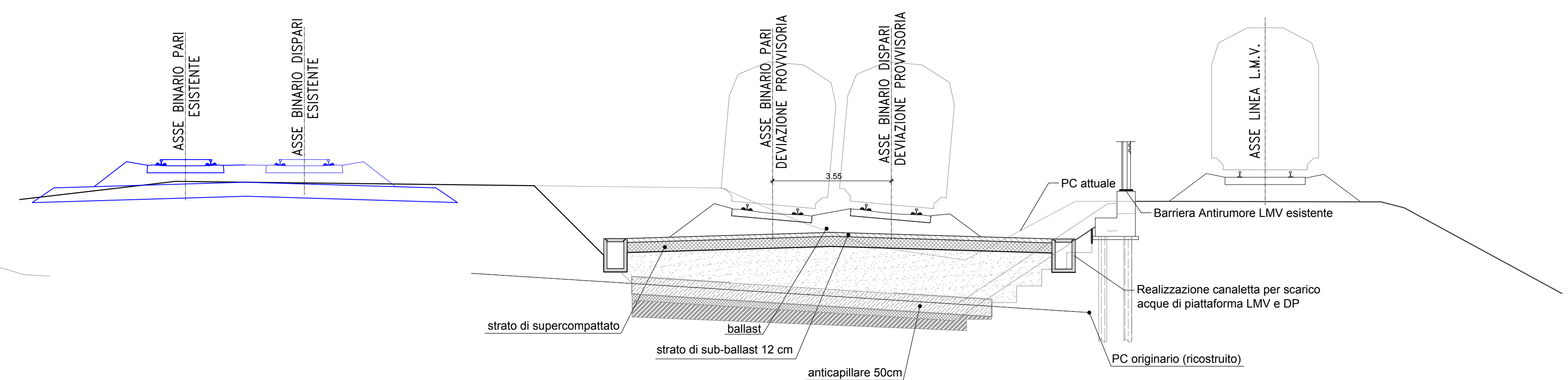
SEZIONE 2 (da pk 0+300 a pk 0+450) Scala 1:100
