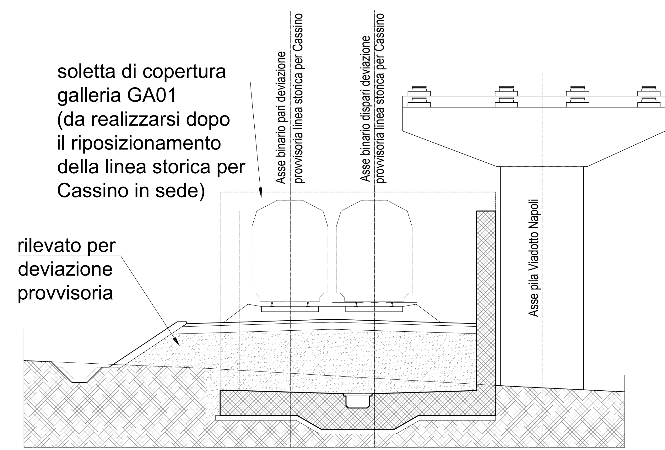
SEZIONE A-A Scala 1:200
