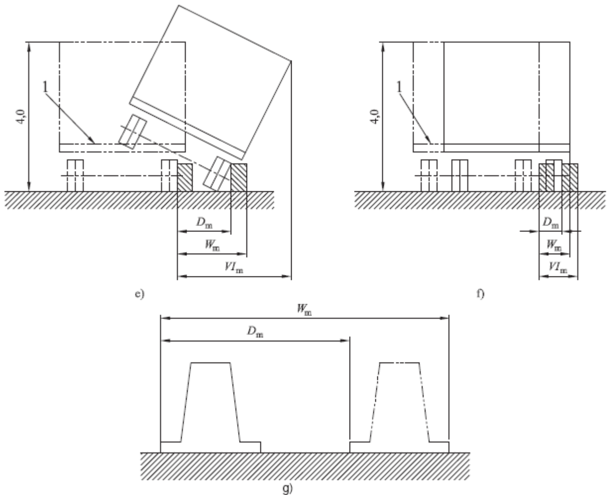
Figura 3: Prospetto 4 Valori misurati di deflessione dinamica ( D_m ), larg. operativa ( W_m )
