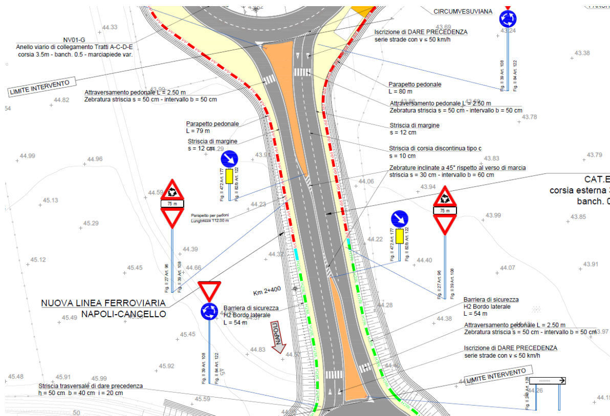
Figura 4: Barriere di sicurezza
