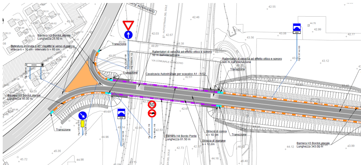
Figura 7: Planimetria Barriere di sicurezza Tratto C2
