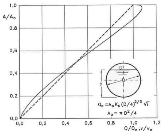
Figura 7 : Andamento della portata in funzione della sezione liquida della condotta.
