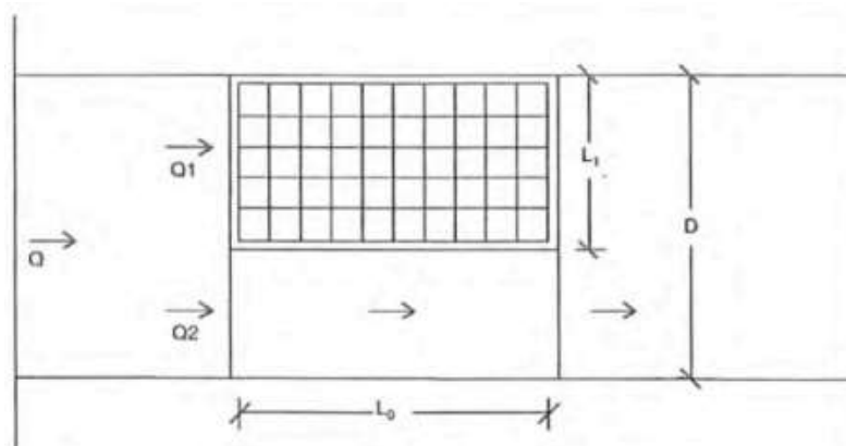
Figura 15 : schema di deflusso in prossimità di una coditoia
