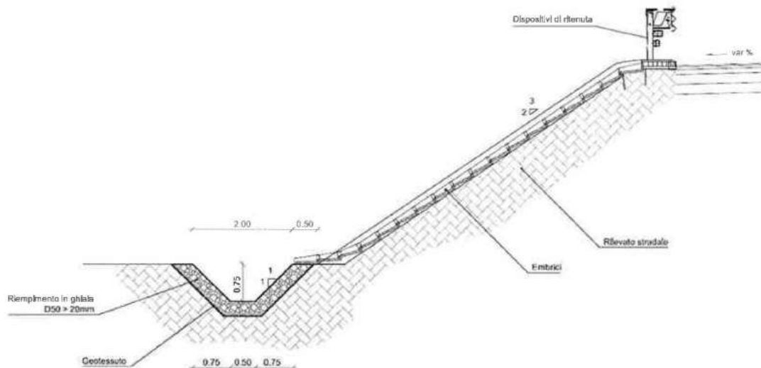
Figura 10 : Sistema di drenaggio stradale, embrice e fosso di guardia.
