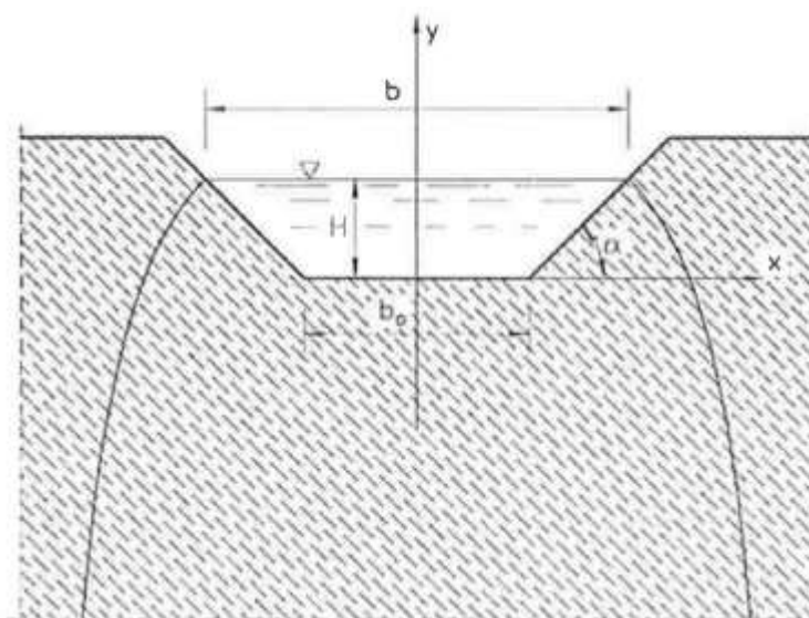
Figura 11 : Schema del funzionamento dispersivo del fossato dispersivo.
