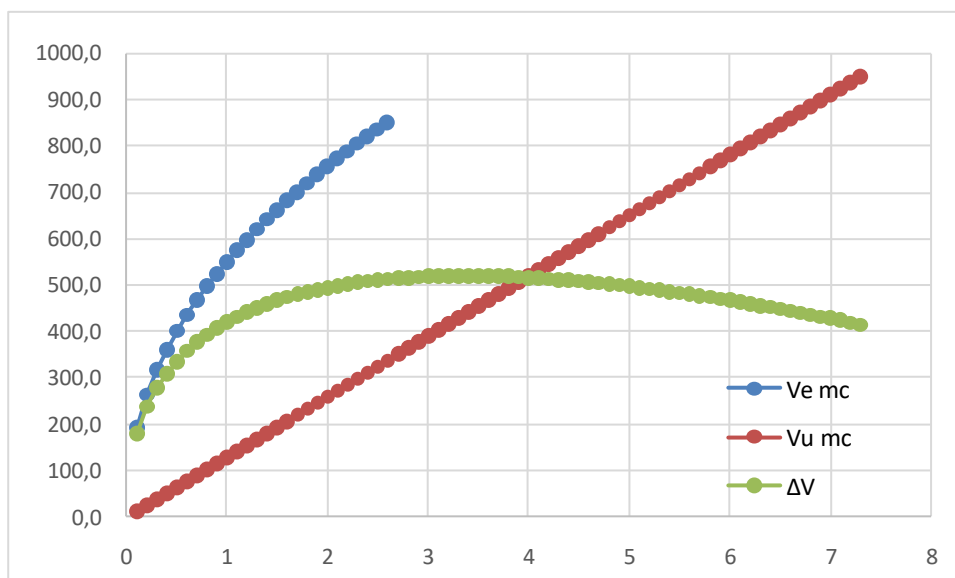
Figura 16 - Volume laminato dalla trincea disperdente TD01D (ramo C)
