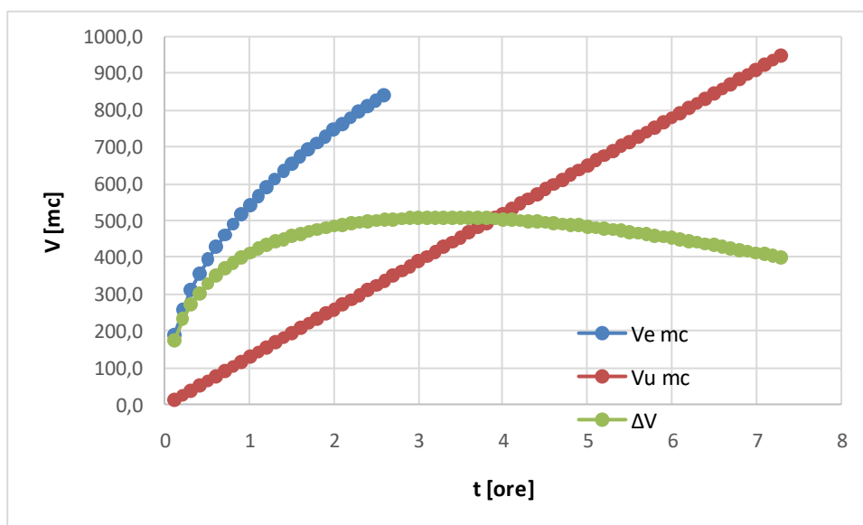
Figura 19 - Volume laminato trincea disperdente TD01C (parcheggio FS)
