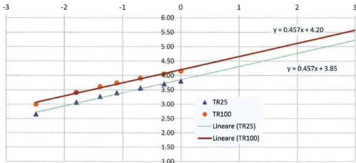
Figura 4 : Curva biparametrica sul piano bilogarithmico per l'area omogenea C2
