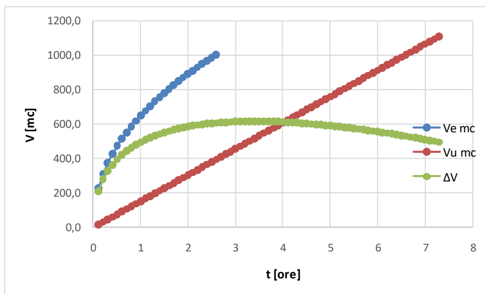
Figura 17- Volume laminato trincea disperdente TD01A (parcheggio Circumvesuviana)
