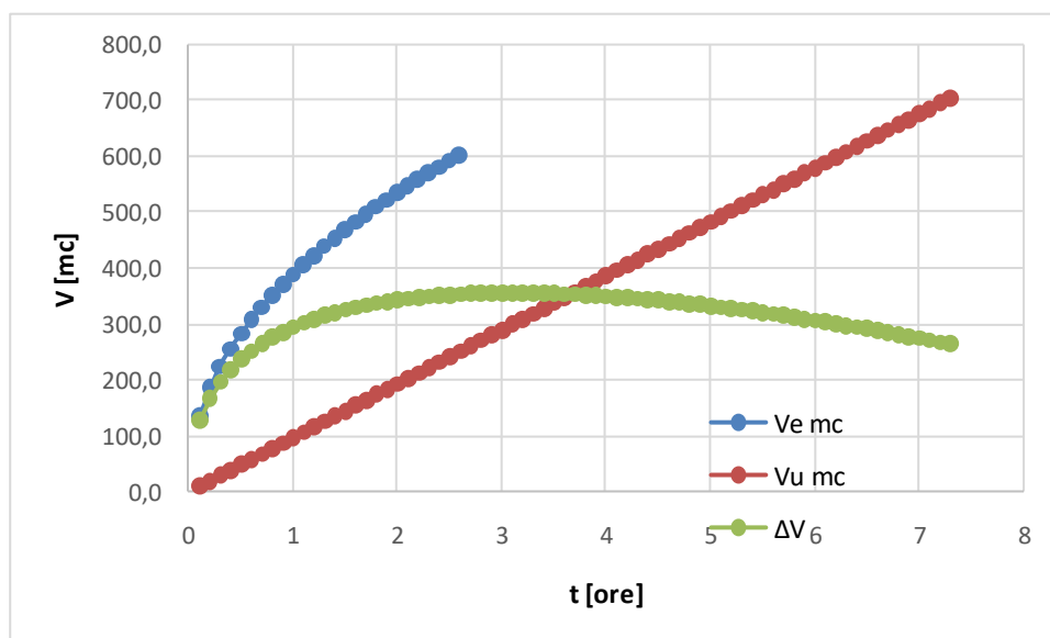
Figura 18 - Volume laminato trincea disperdente TD01B
