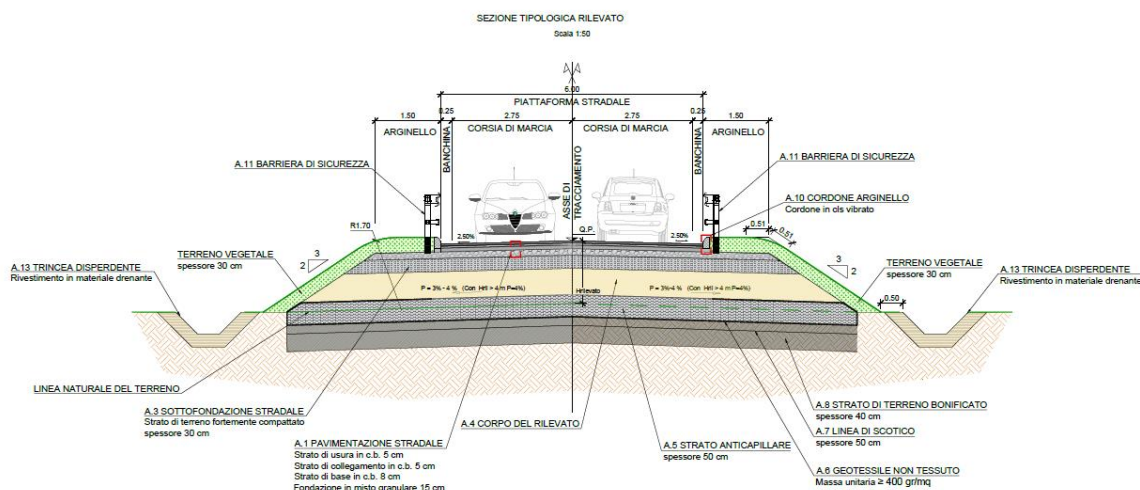
Figura 2: Sezione tipologica
