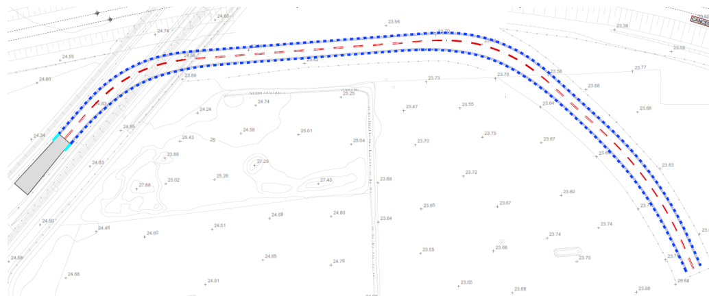
Figura 5: Identificazione della Barriera classe H1 Bordo laterale in blu
