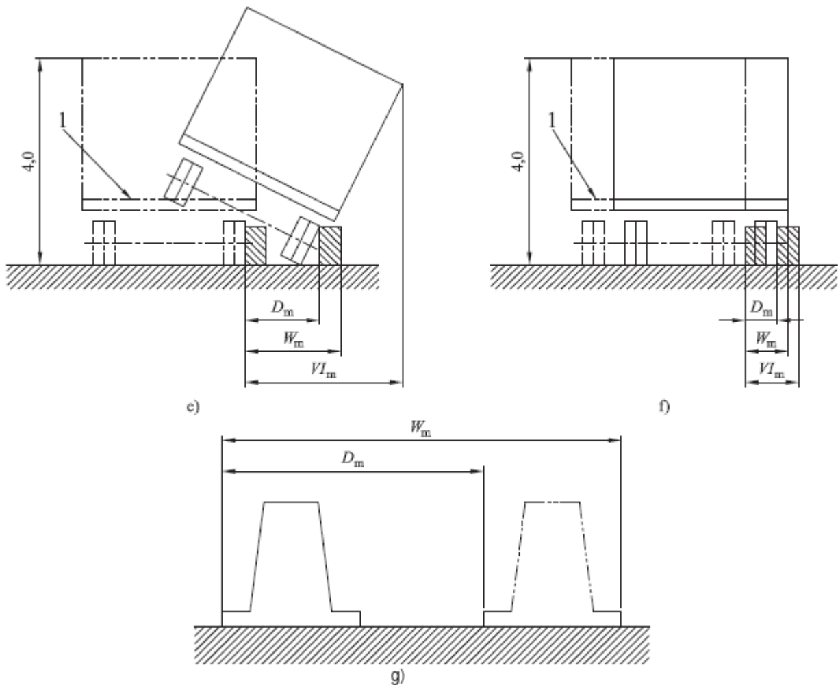
Figura 5: Prospetto 4 Valori misurati di deflessione dinamica ( D_m ), larg. operativa ( W_m ) intrusione del veicolo ( Vl_m )
