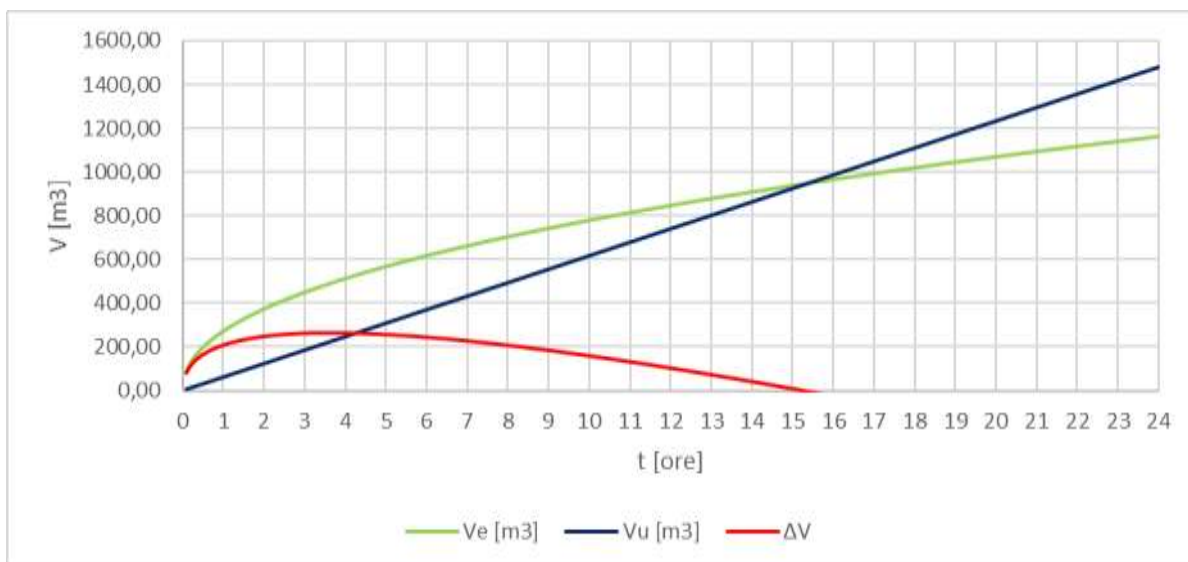
Figura 15: volume laminato dalla trincea disperdente
