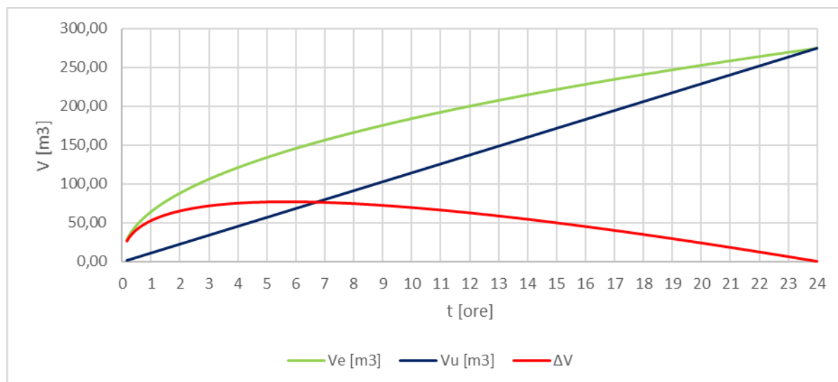
Figura 16: volume laminato dalla trincea disperdente
