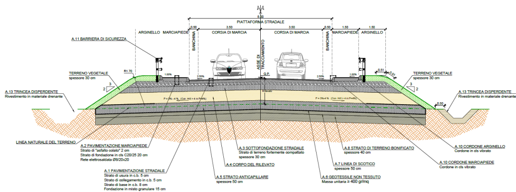
Figura 2: Sezione tipologica in rilevato
