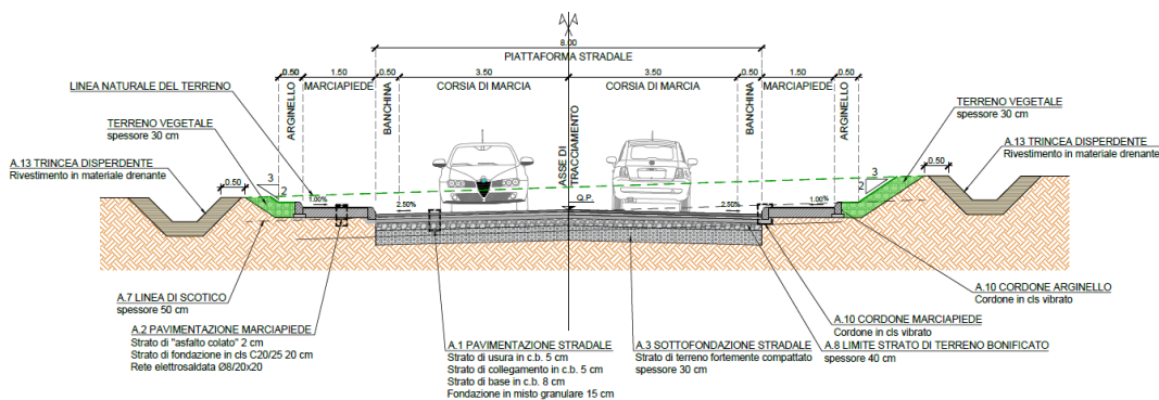
Figura 3: Sezione tipologica in trincea
