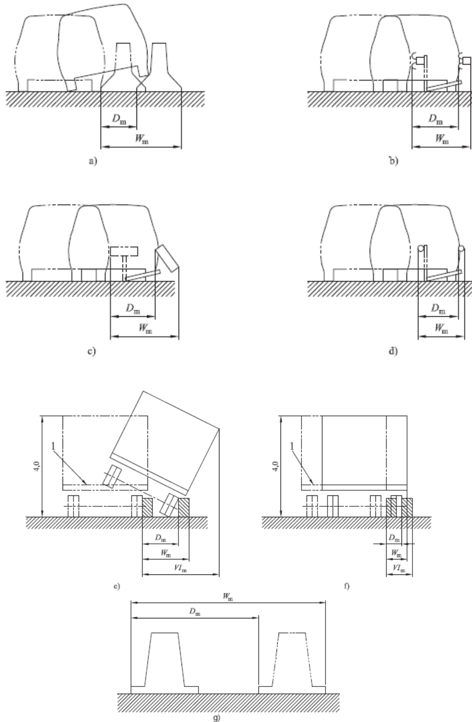
Figura 5: Prospetto 4 Valori di deflessione dinamica ( D_m ), larg. operativa ( W_m ), intrusione del veicolo ( V_{Im} )
