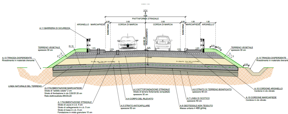
Figura 2: Sezione tipologica in rilevato
