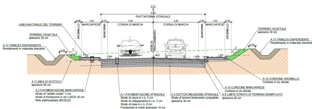
Figura 3: Sezione tipologica in trincea
