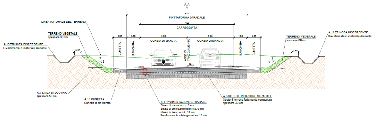
Figura 4: Sezione tipologica in trincea
