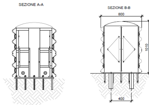
Figura 10: Sezioni trasversali attenuatore d'urto
