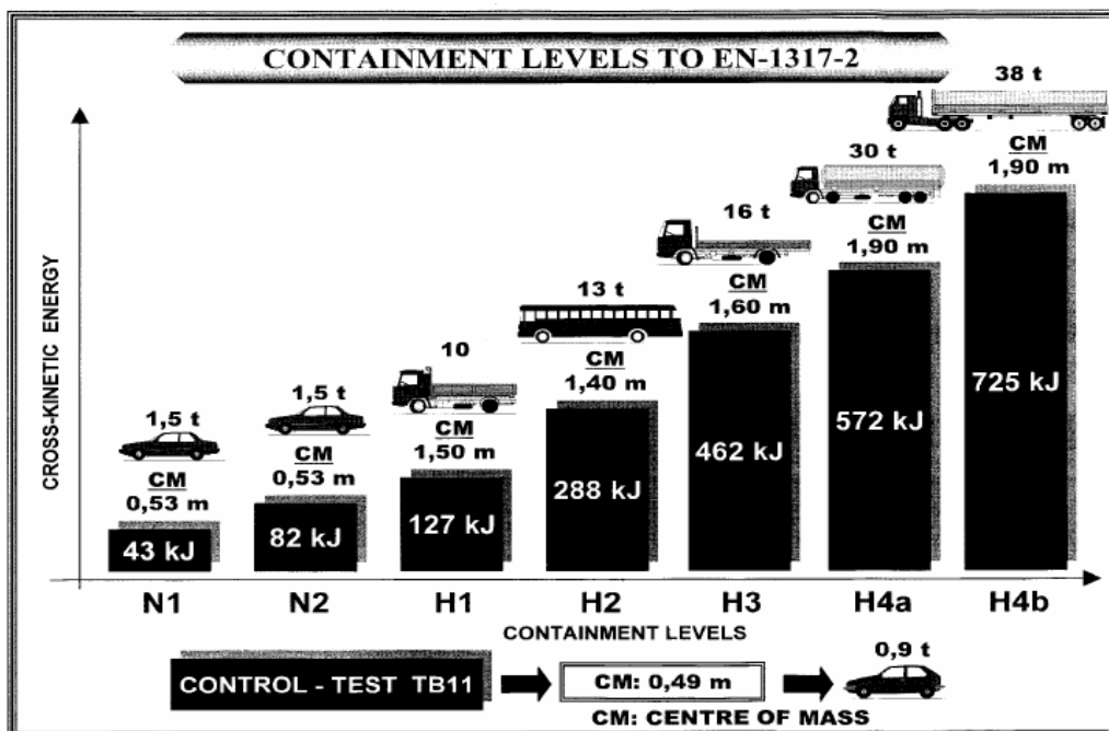
Figura 5: Classi di contenimento
