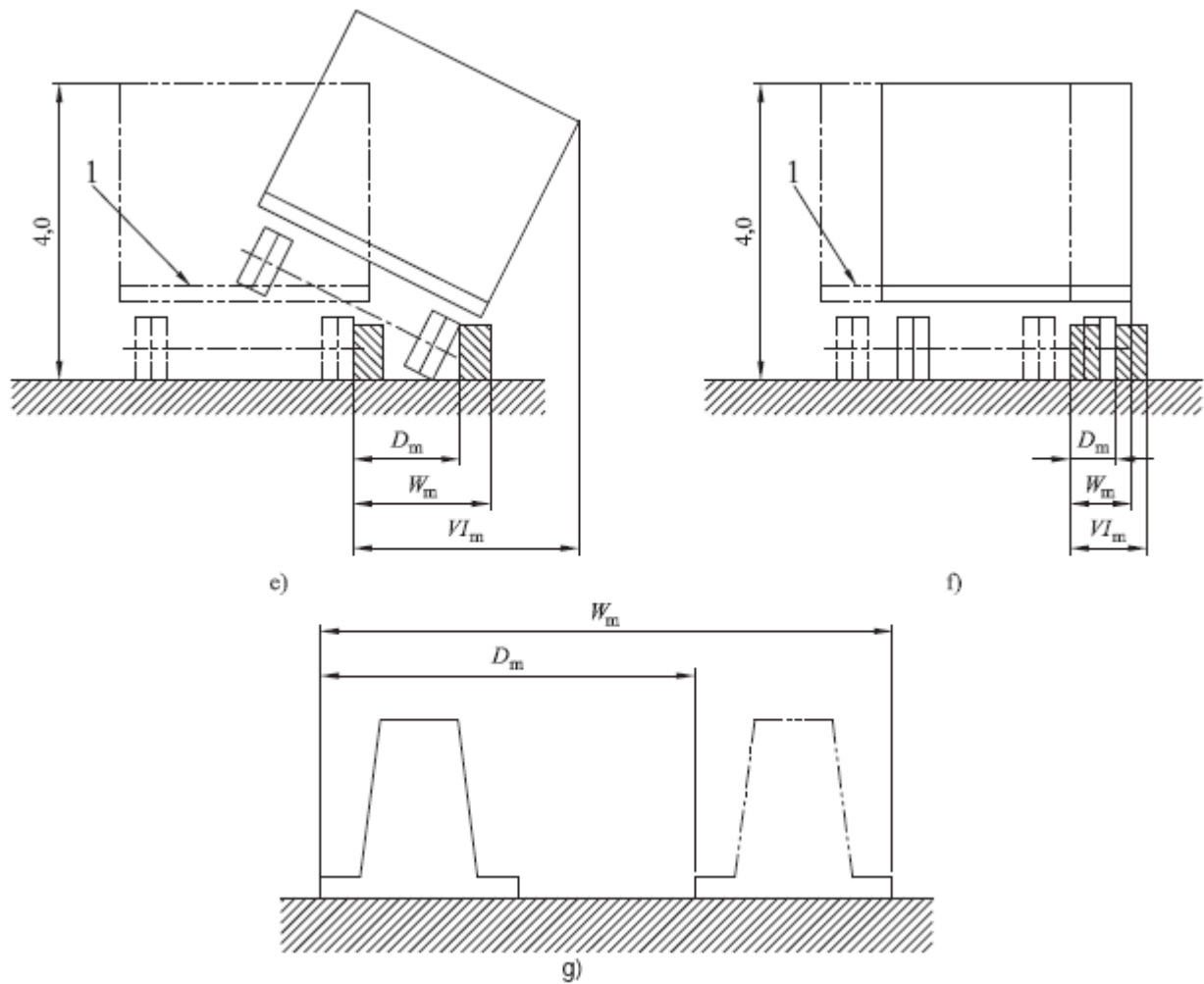
Figura 6: Prospetto 4 Valori misurati di deflessione dinamica ( D_m ), larg. operativa ( W_m ) intrusione del veicolo ( V_{I_m} )
