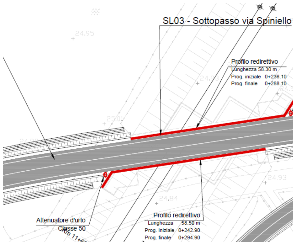
Figura 7: Identificazione dei profili ridirettivi
