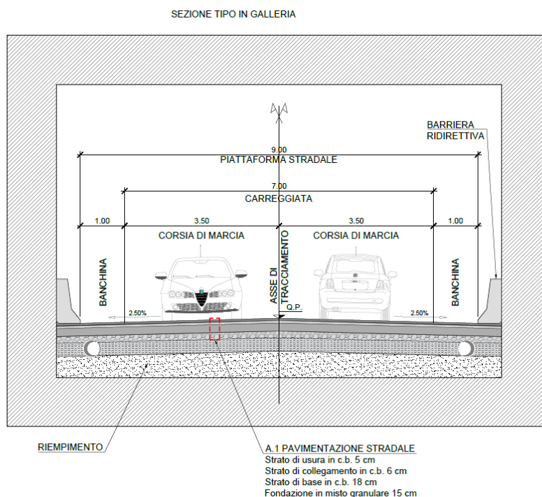
Figura 3: Sezione tipologica in galleria
