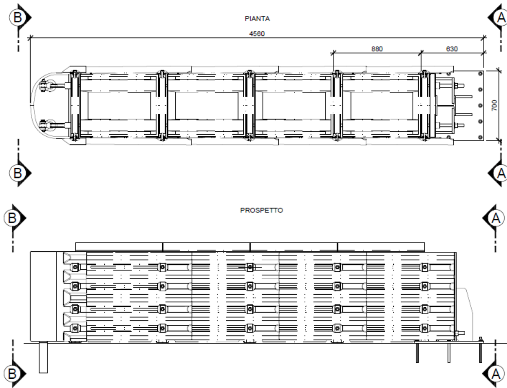
Figura 9: Pianta e prospetto attenuatore d'urto
