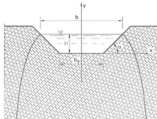
Figura 13 : Schema del funzionamento del fosso disperdente.
