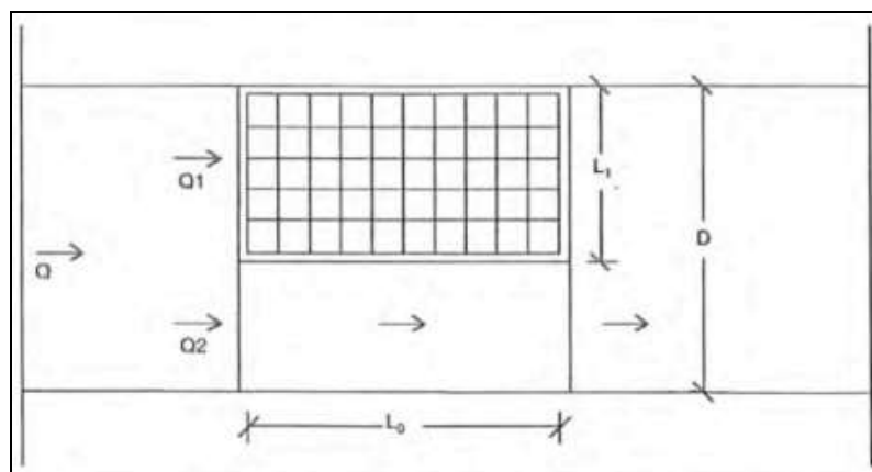
Figura 10 : schema di deflusso in prossimità di una caditoia
