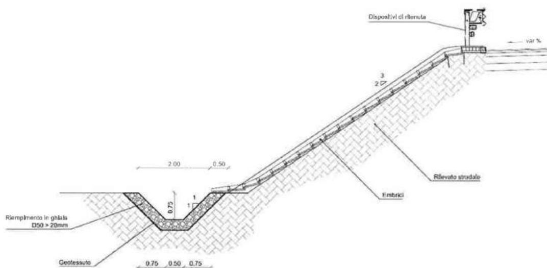
Figura 12 : Sistema di drenaggio stradale, embrice e fosso di guardia.
