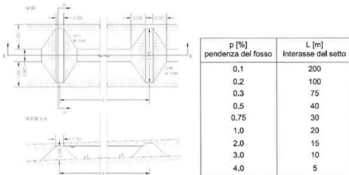
Figura 14 : Setti lungo i fossi disperdenti.
