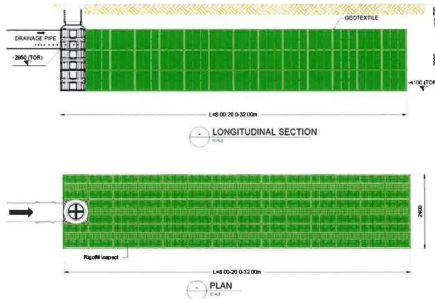
Figura 15 : Tipologico di trincea drenante con moduli in materiale plastico
