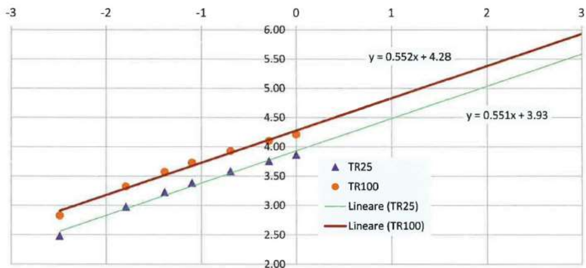
Figura 5 : Curva biparametrica sul piano bilogaritmico per l'area omogenea C3
