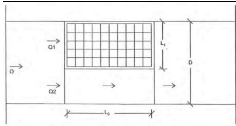
Figura 14 : schema di deflusso in prossimità di una coditoia
