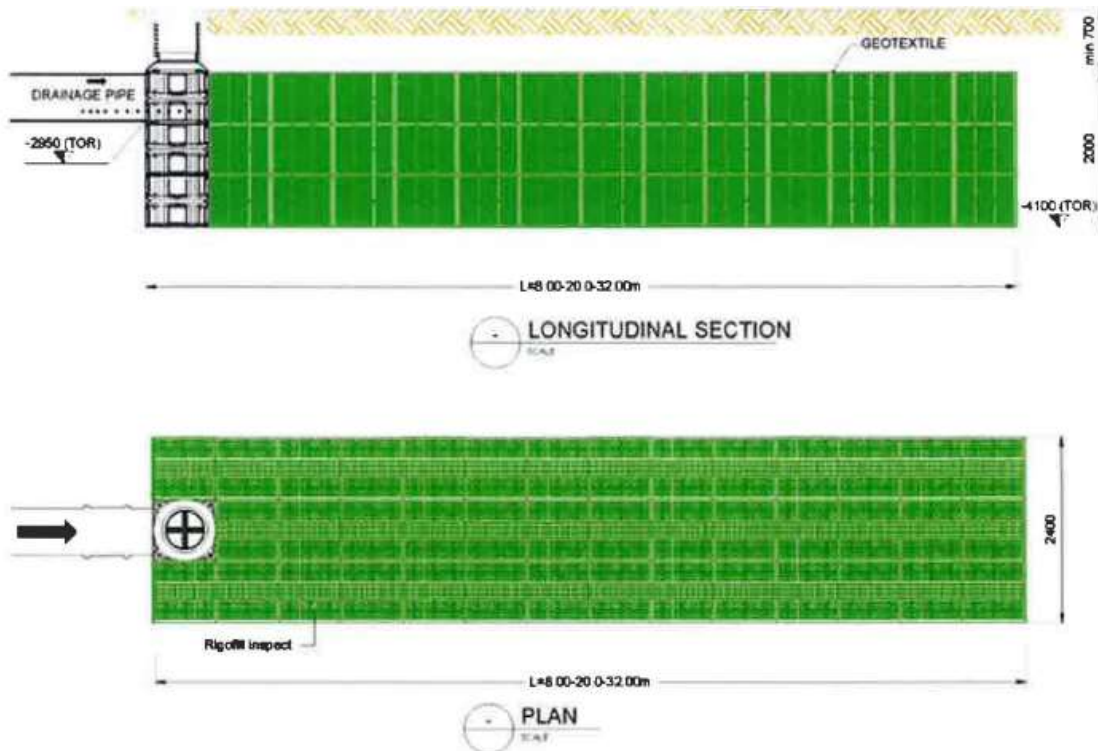
Figura 12 : Tipologico di trincea drenante con moduli in materiale plastico
