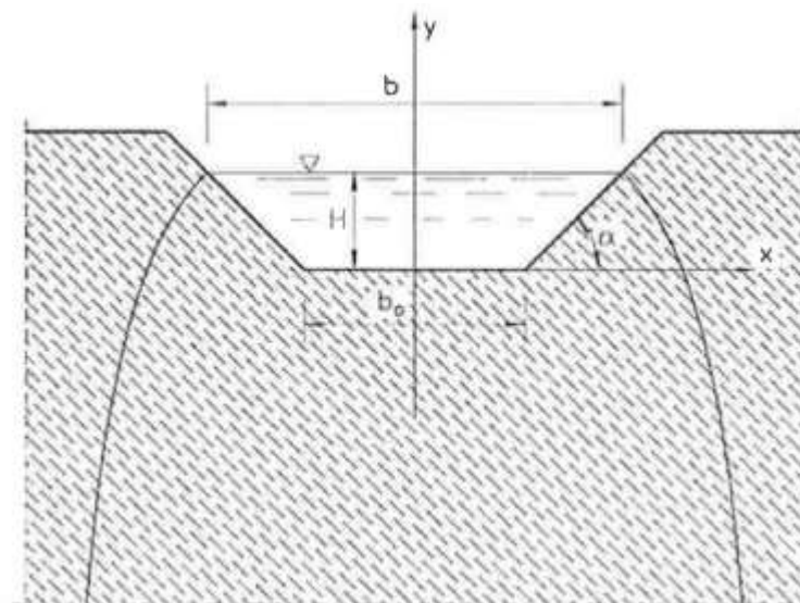
Figura 10 : Schema del funzionamento del fosso disperdente.
