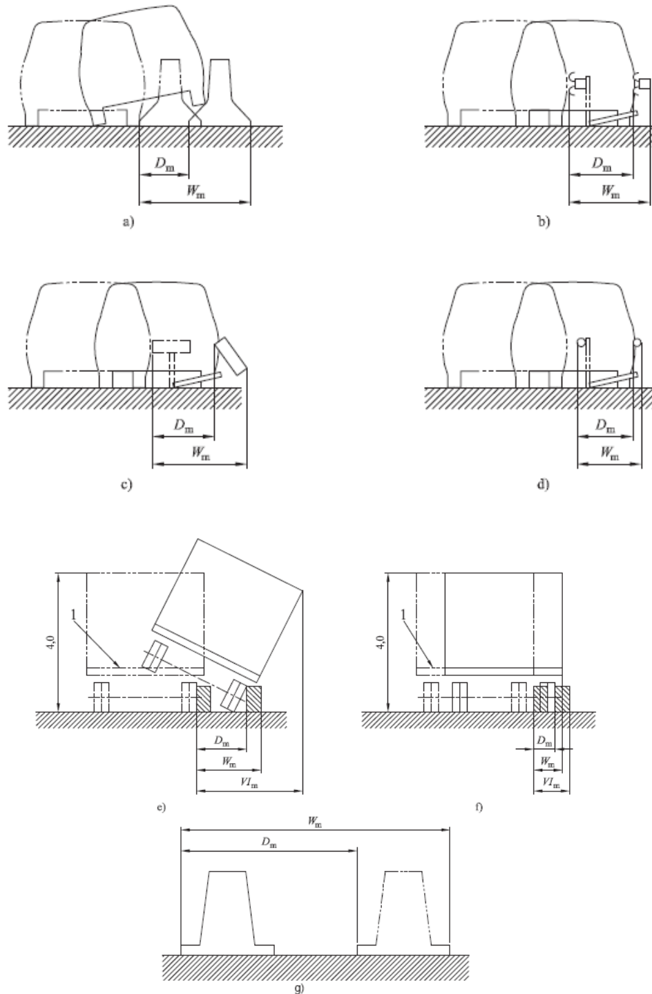
Figura 5: Prospetto 4 Valori misurati di deflessione dinamica ( D_m ), larg. operativa ( W_m ) intrusione del veicolo ( V_{Im} )
