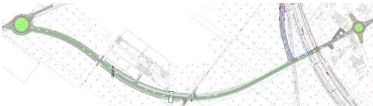
Figura 8: Identificazione delle Barriera classe H2 bordo laterale in verde
