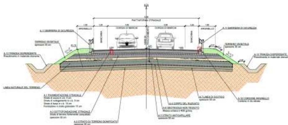
Figura 2: Sezione tipologica in rilevato
