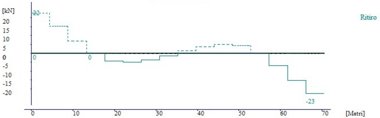
Elementi 201-222
