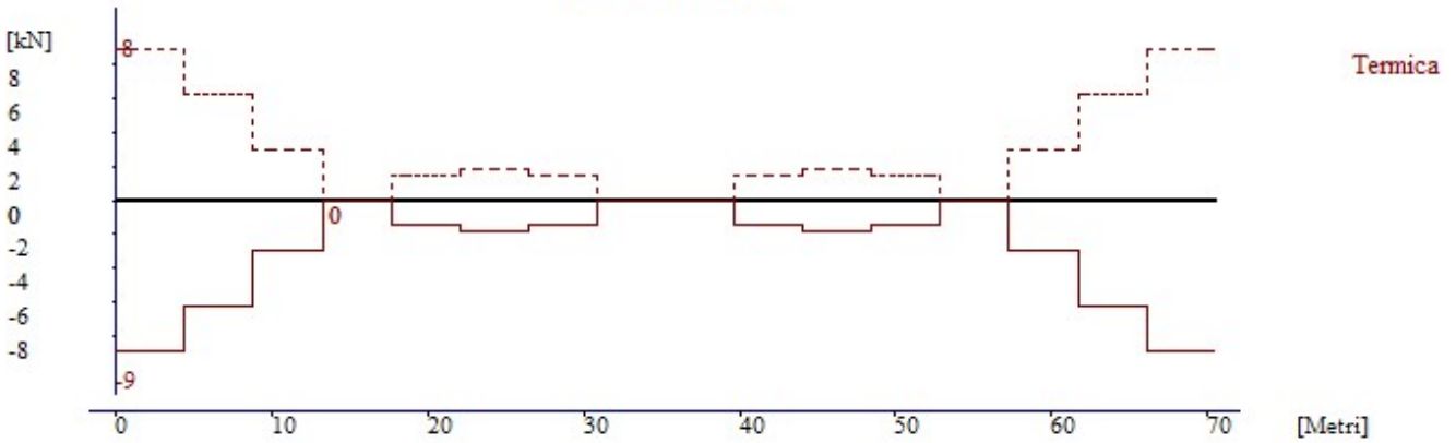
Elementi 201-222
