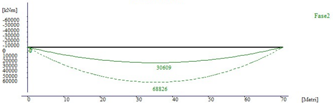
Elementi 101-122
