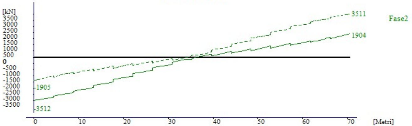
Elementi 201-222
