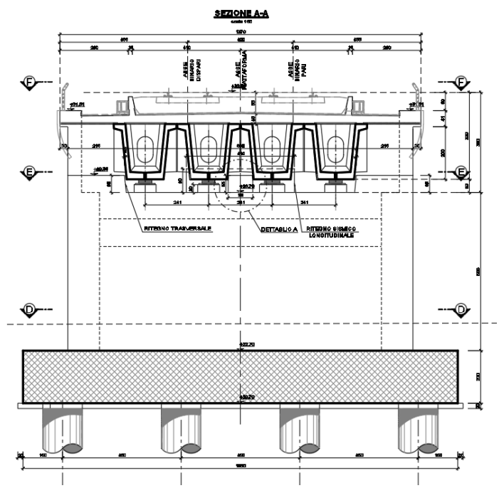
Figura 4: Sezione Trasversale
