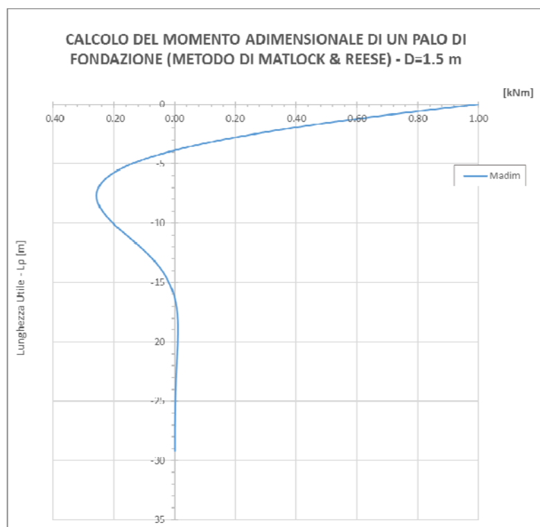
Figura 20: Diagramma del Momento adimensionale lungo il palo
