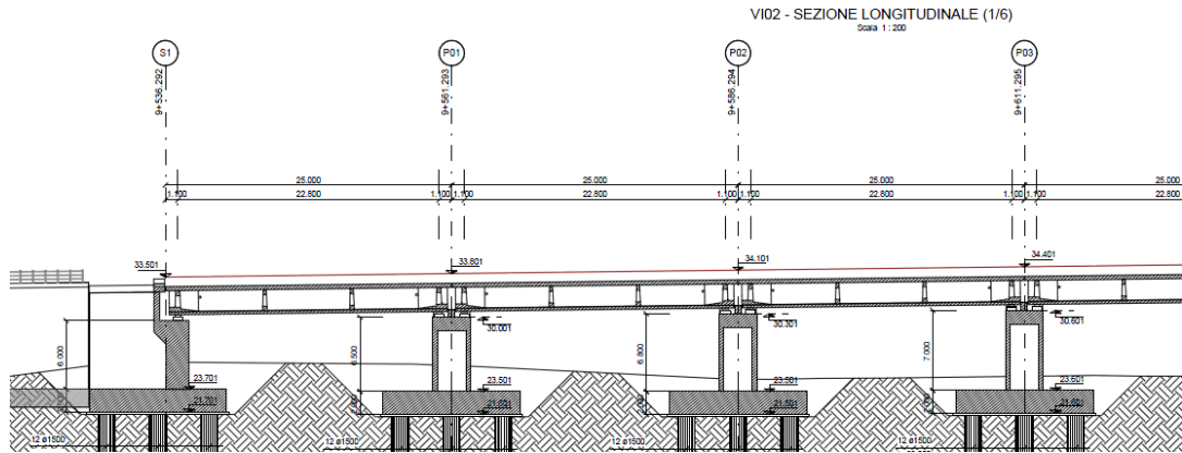
Figura 2: Profilo longitudinale
