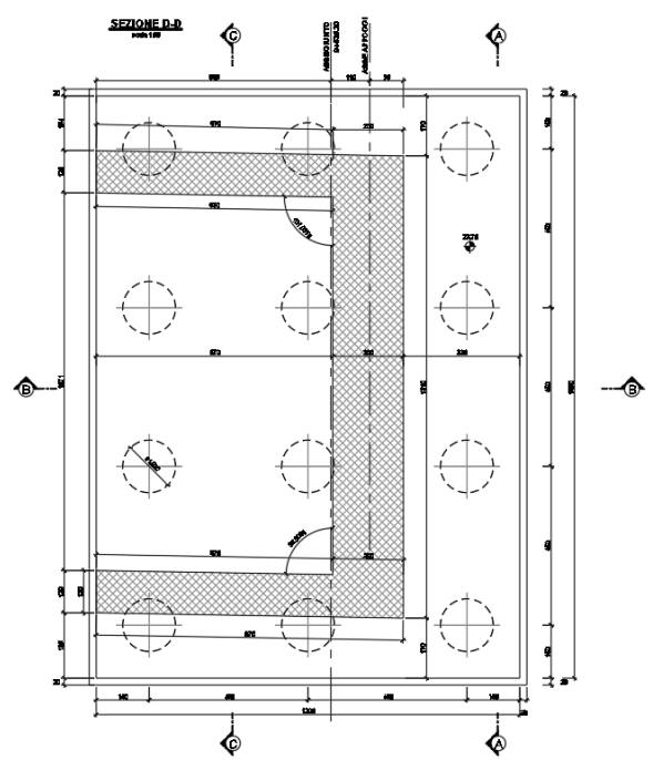
Figura 5: Pianta
