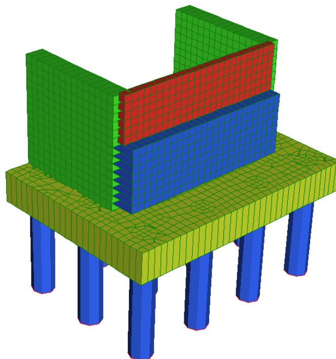
Figura 19: Modellazione tridimensionale agli Elementi Finiti
