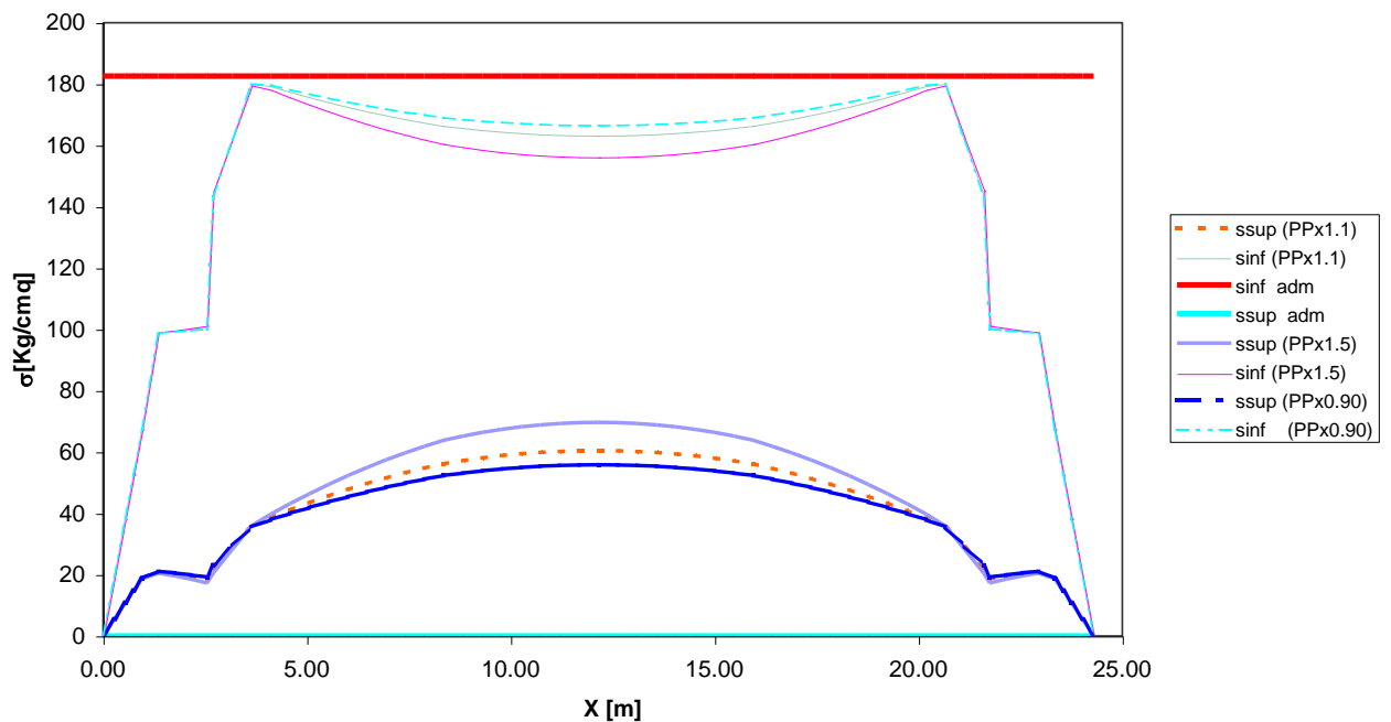
Tensioni ai lembi della trave in fase di sollevamento Rckj=400 daN/cm 2
