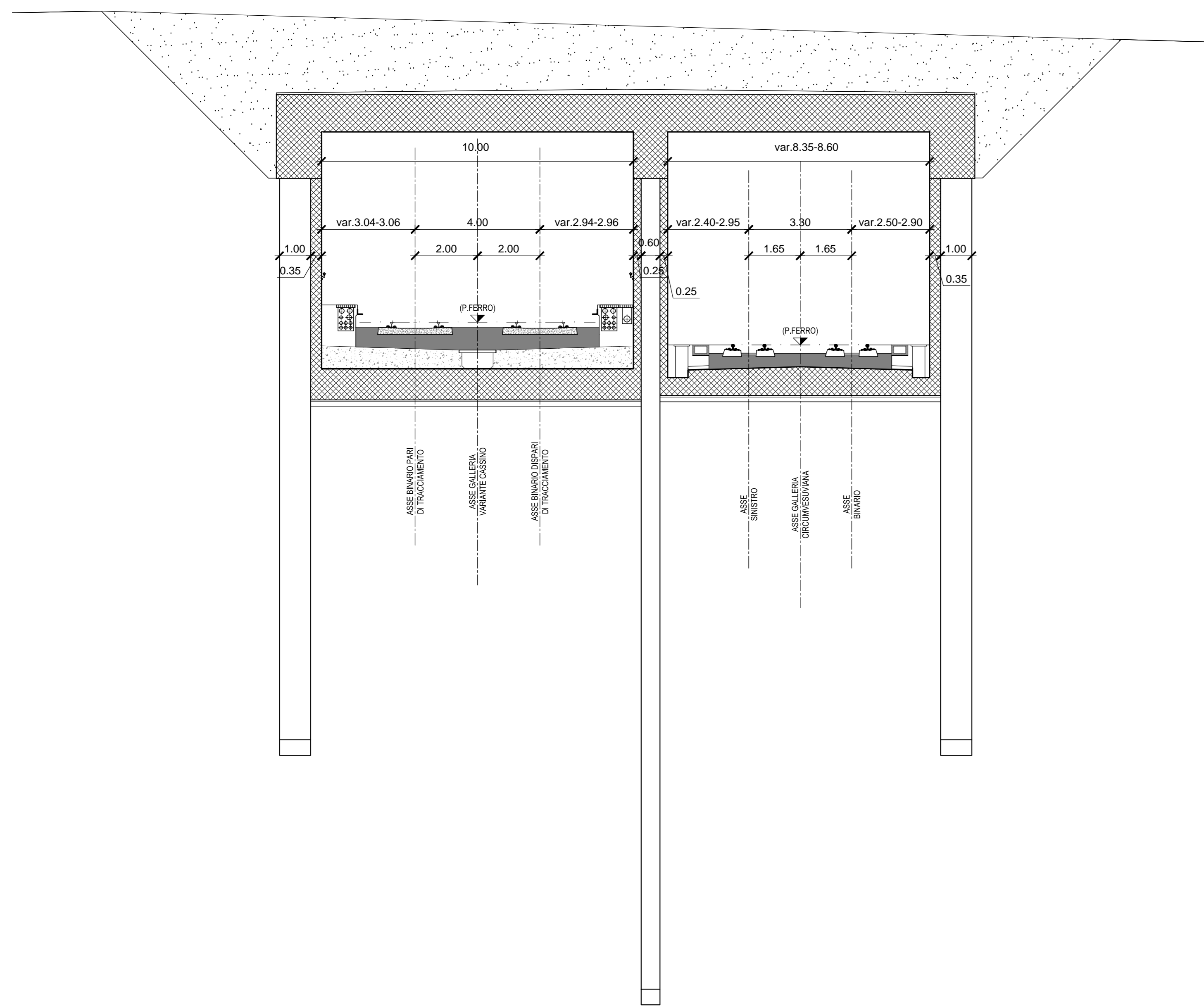
SEZIONE TRASVERSALE IN GALLERIA TIPO "C2"
