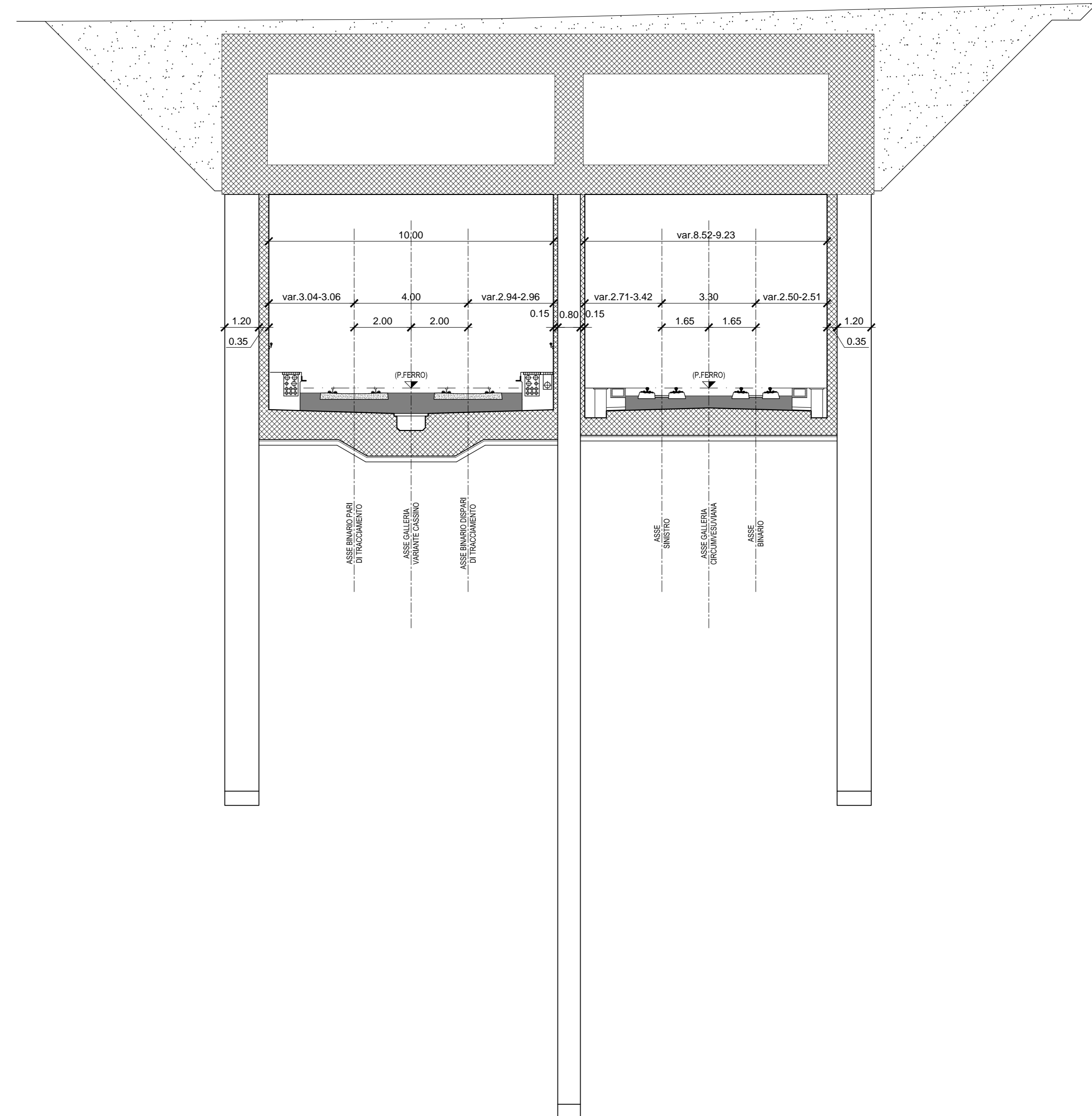
SEZIONE TRASVERSALE IN GALLERIA TIPO "H"
