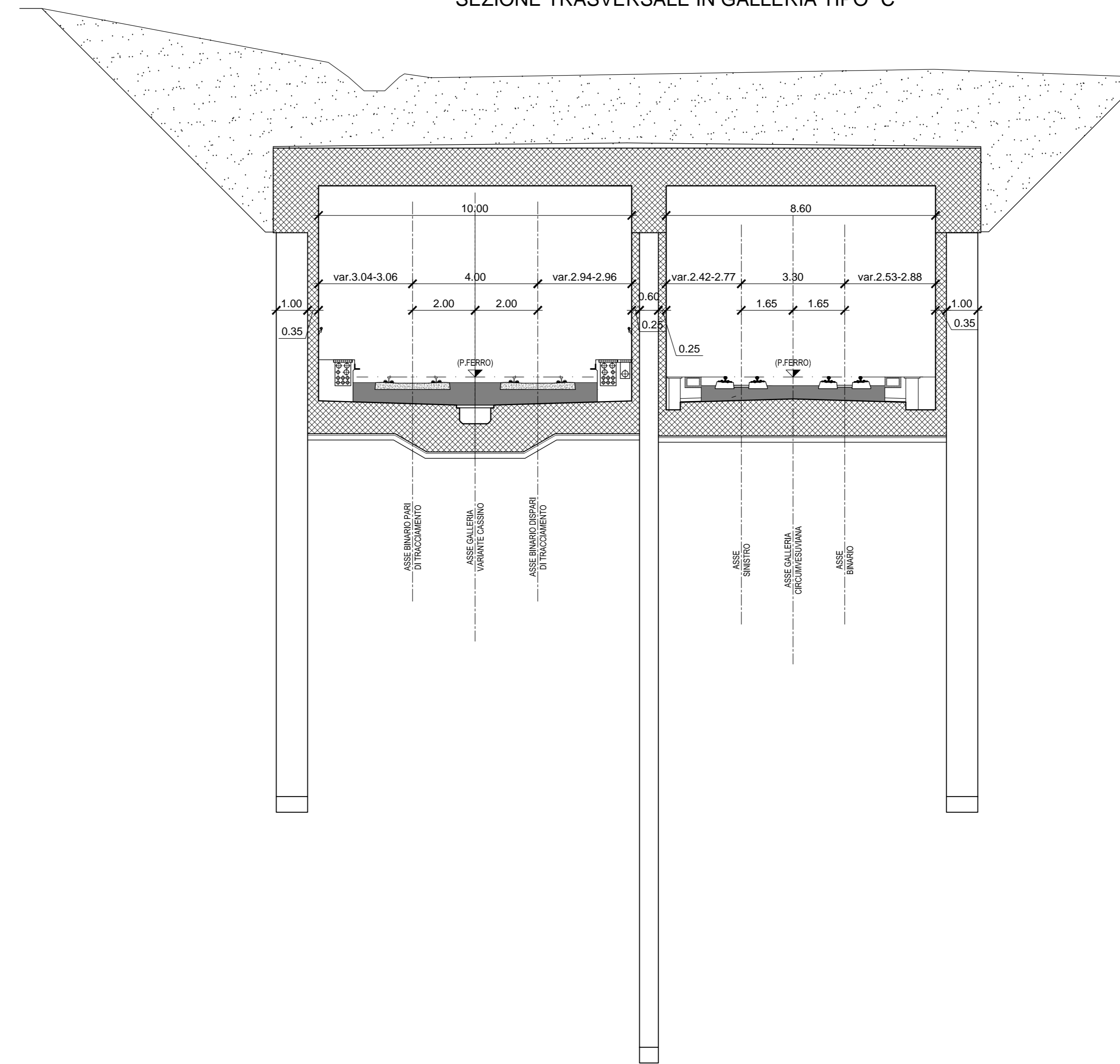
SEZIONE TRASVERSALE IN GALLERIA TIPO "C"
