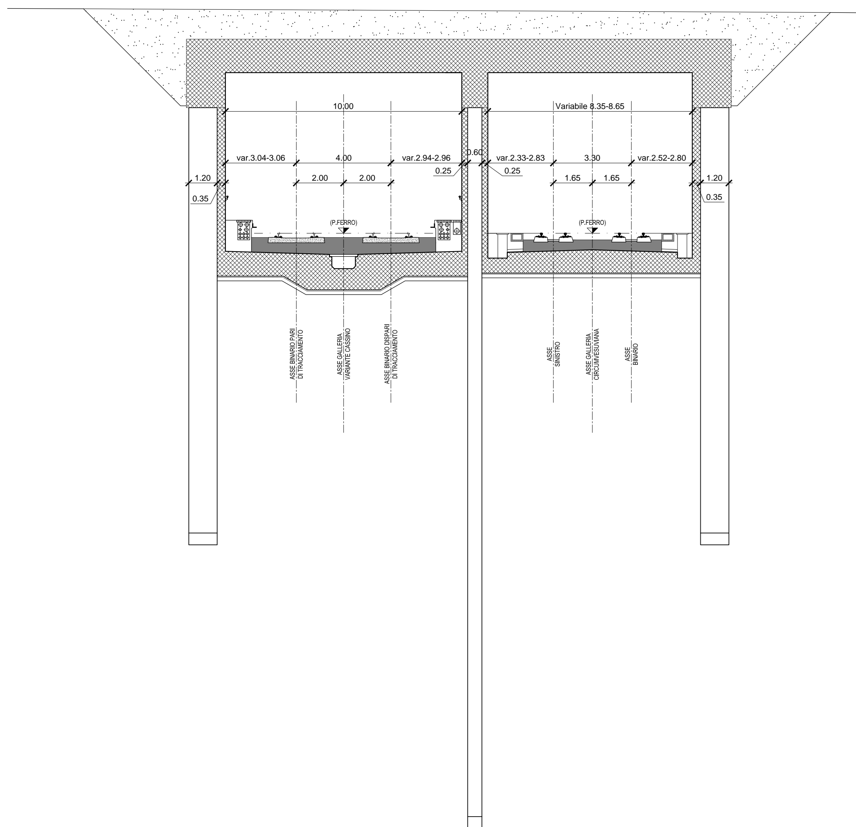
SEZIONE TRASVERSALE IN GALLERIA TIPO "D"
