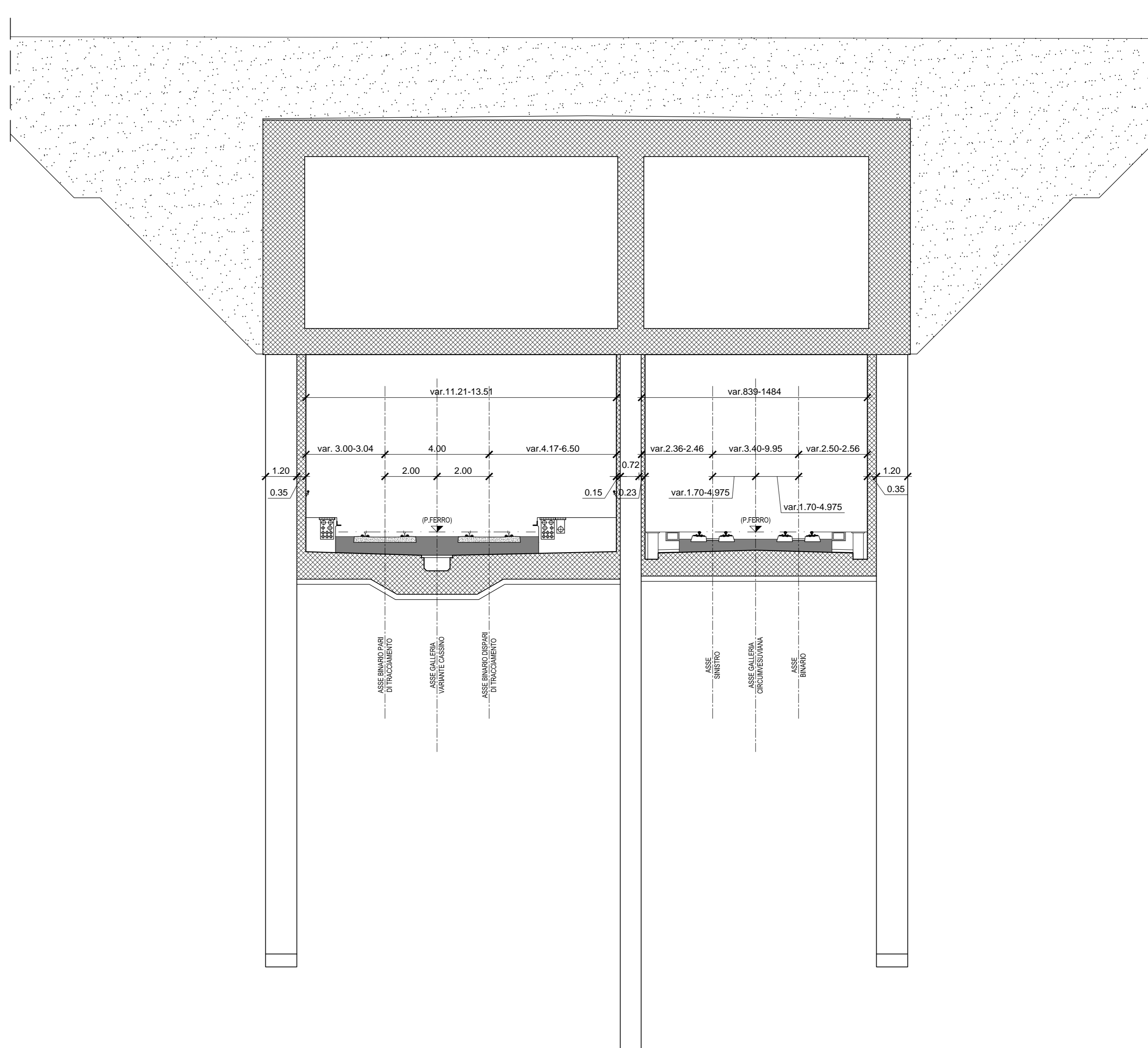
SEZIONE TRASVERSALE IN GALLERIA TIPO "N"
