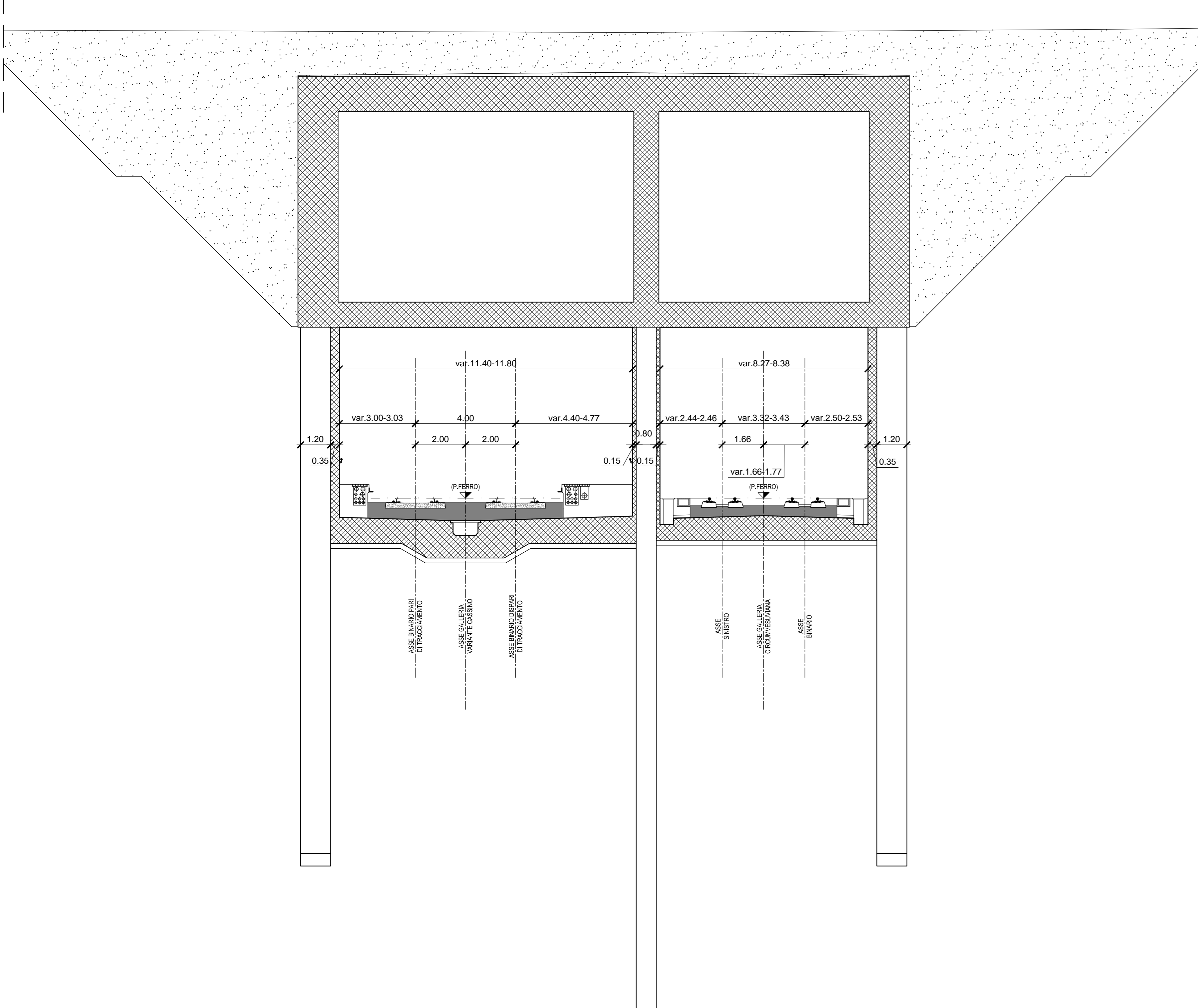
SEZIONE TRASVERSALE IN GALLERIA TIPO "M"
