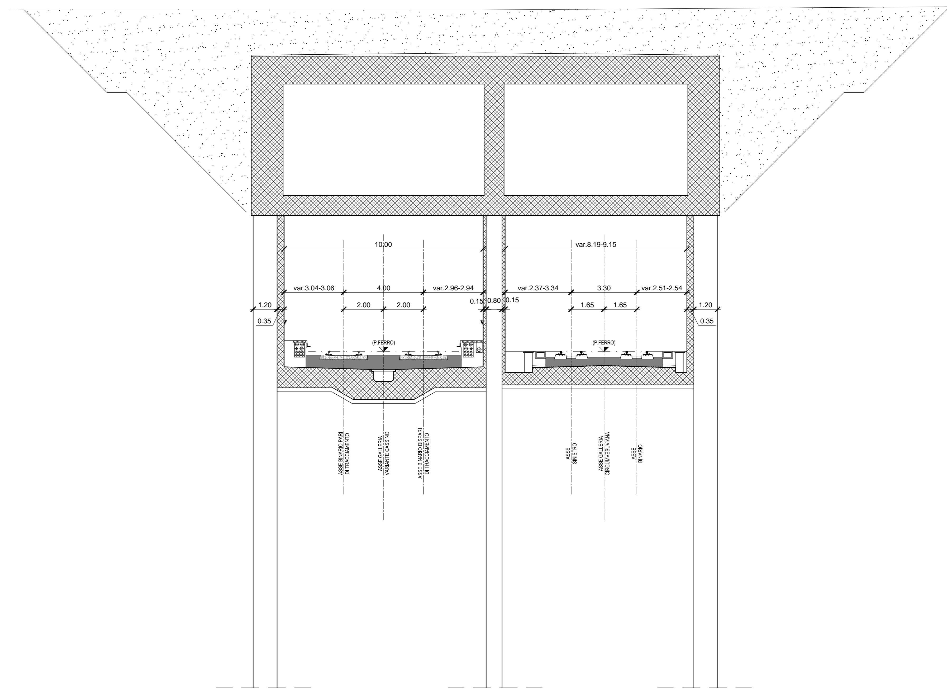
SEZIONE TRASVERSALE IN GALLERIA TIPO "L"
