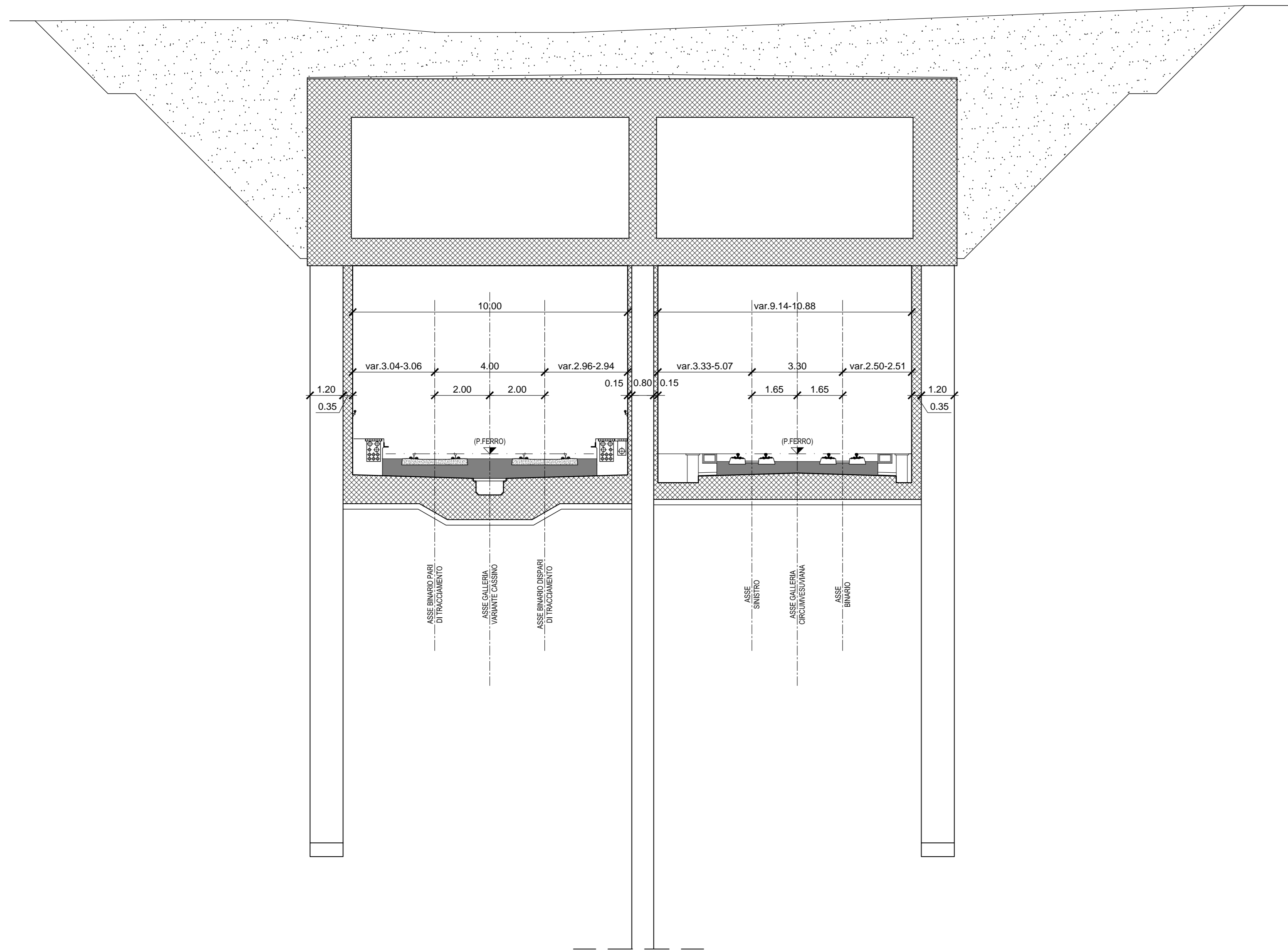
SEZIONE TRASVERSALE IN GALLERIA TIPO "I"
