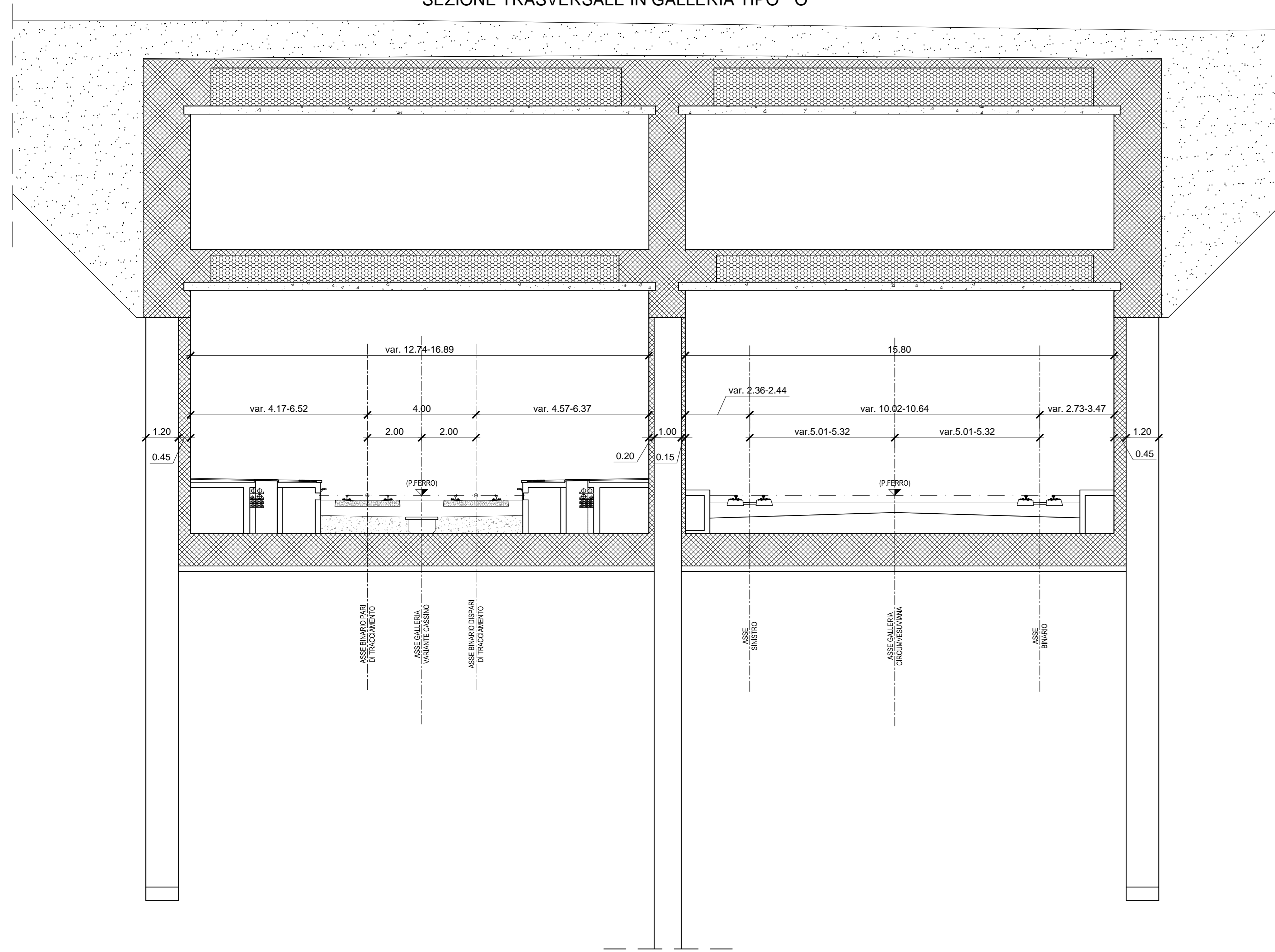
SEZIONE TRASVERSALE IN GALLERIA TIPO " O " "
