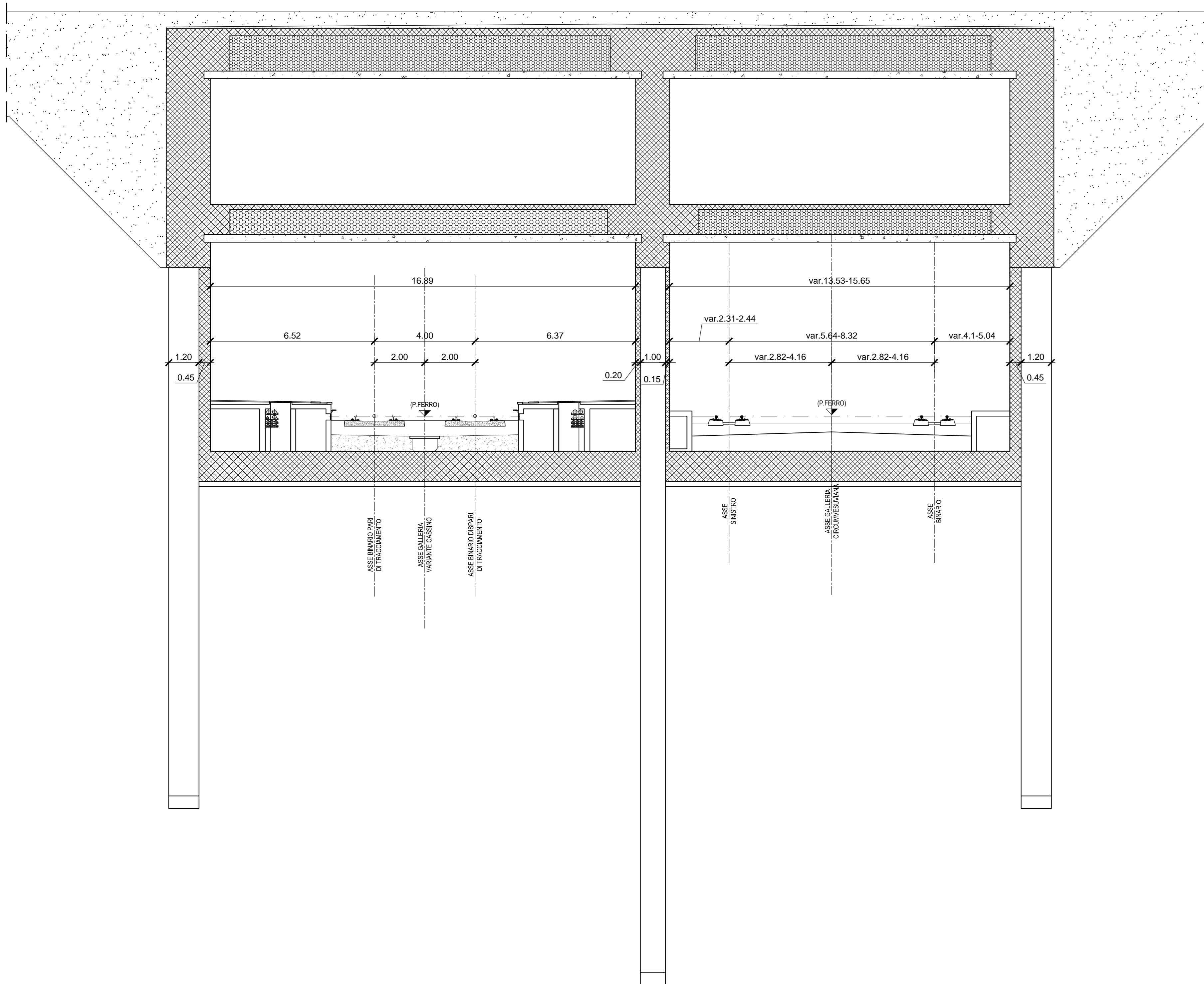
SEZIONE TRASVERSALE IN GALLERIA TIPO " O " "
