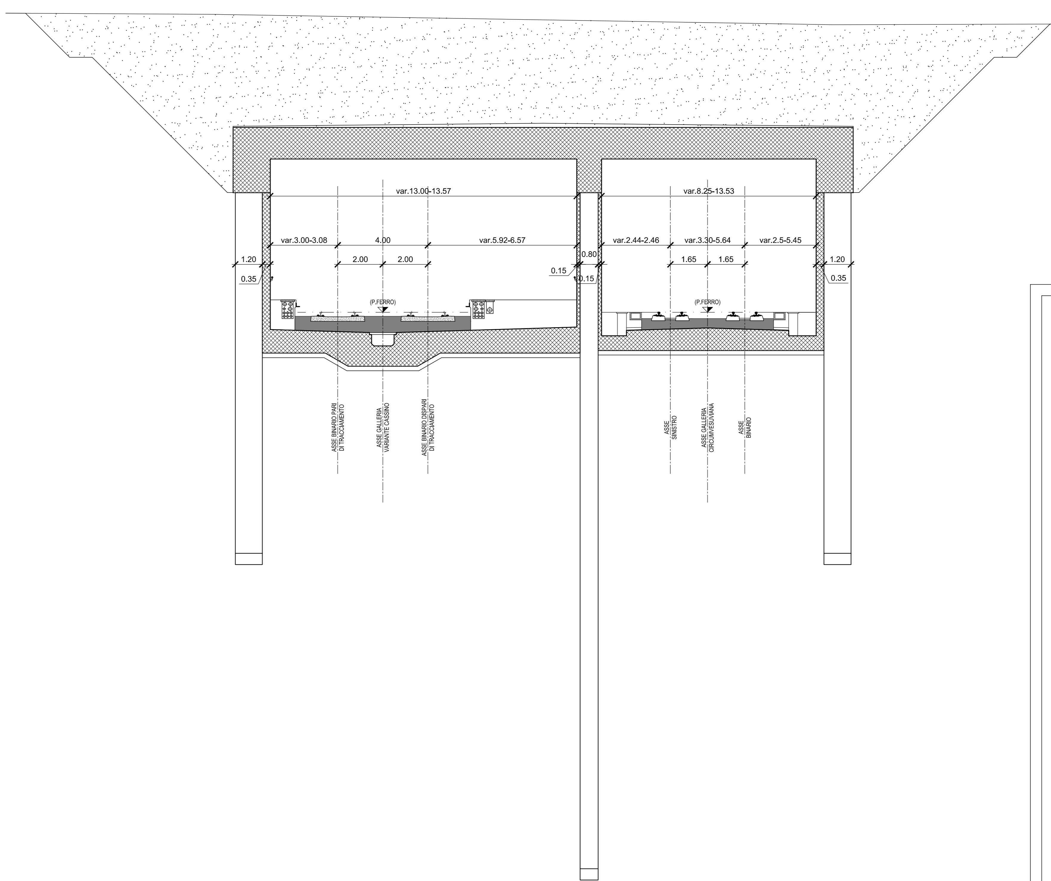
SEZIONE TRASVERSALE IN GALLERIA TIPO " P " "
