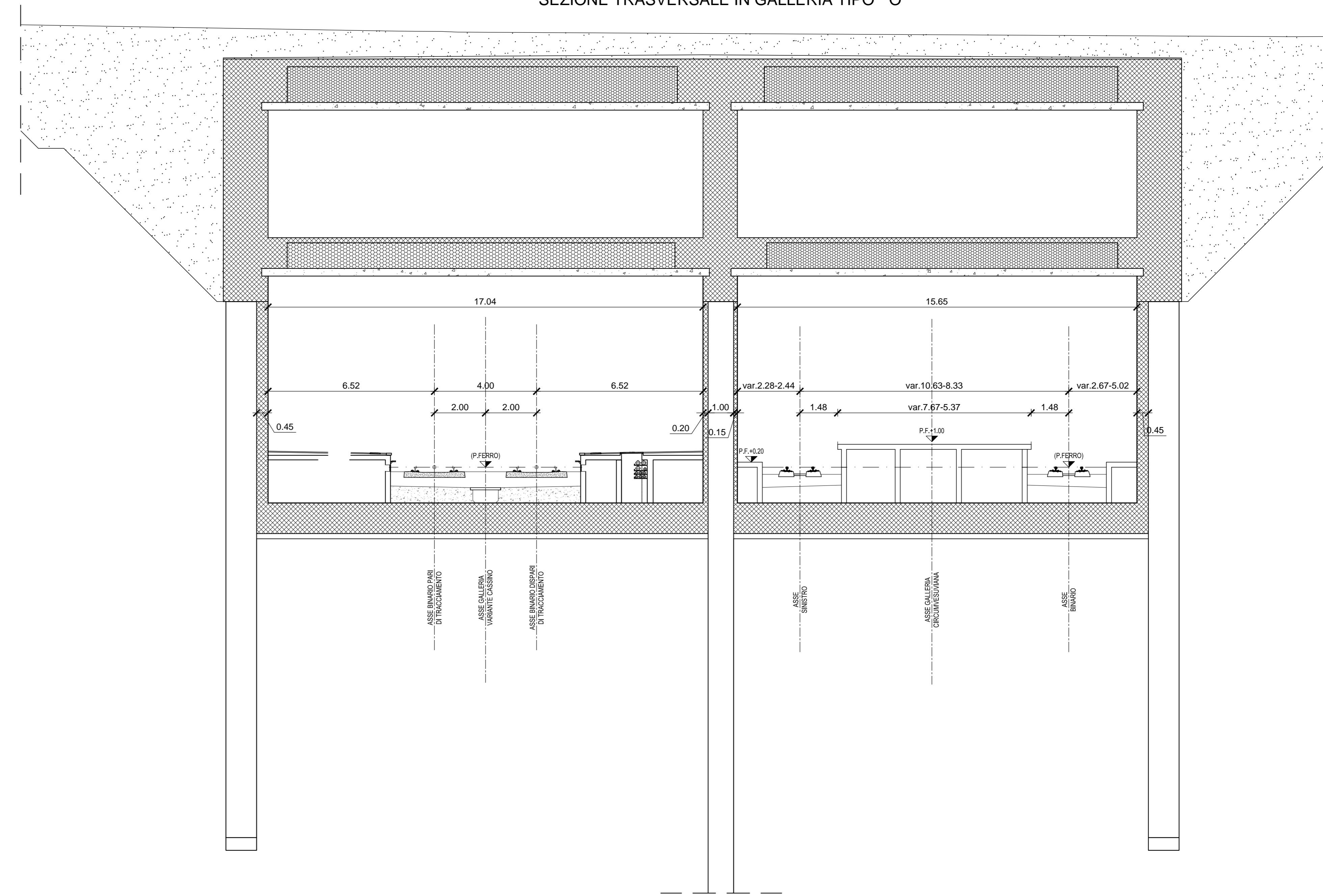
SEZIONE TRASVERSALE IN GALLERIA TIPO " O " "
