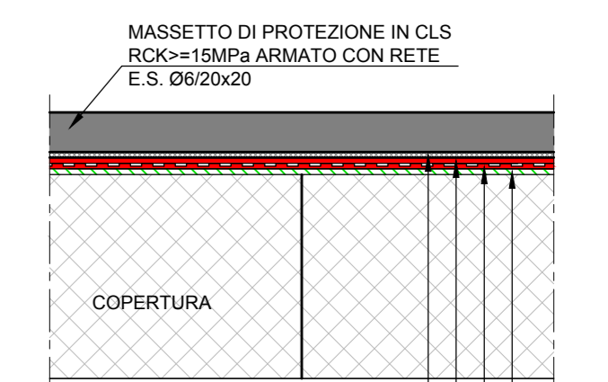
STRATO DI COMPENSAZIONE TNT IN PP 800 g/m² GUAINA IN PVC LISCIO sp = 2 mm GUAINA IN PVC STRUTTURATO sp = 2 mm STRATO DI PROTEZIONE TNT IN PP + ACCAPE 800 g/m² min.
