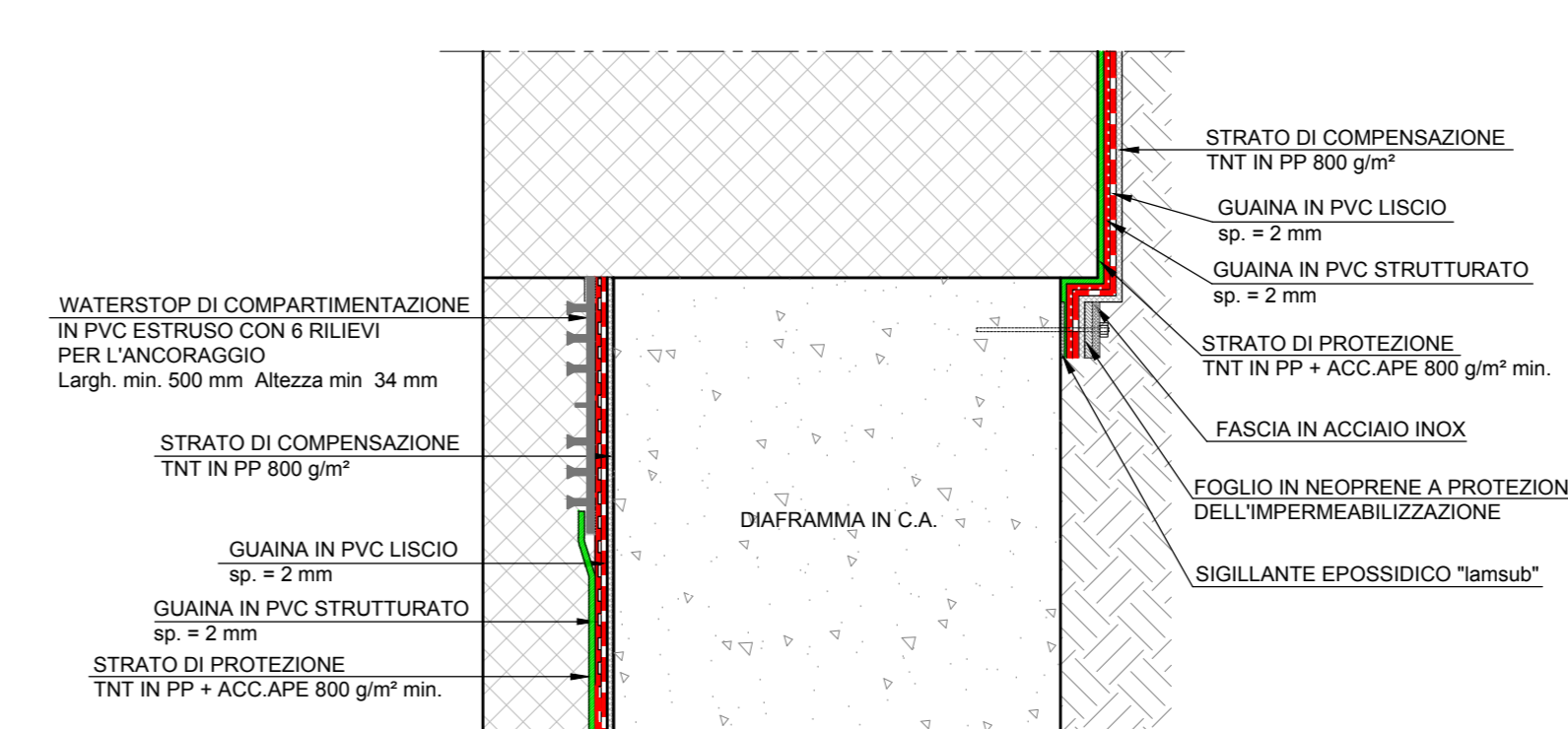
PARTICOLARE 2
