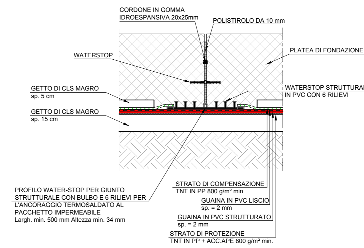
PARTICOLARE 5
