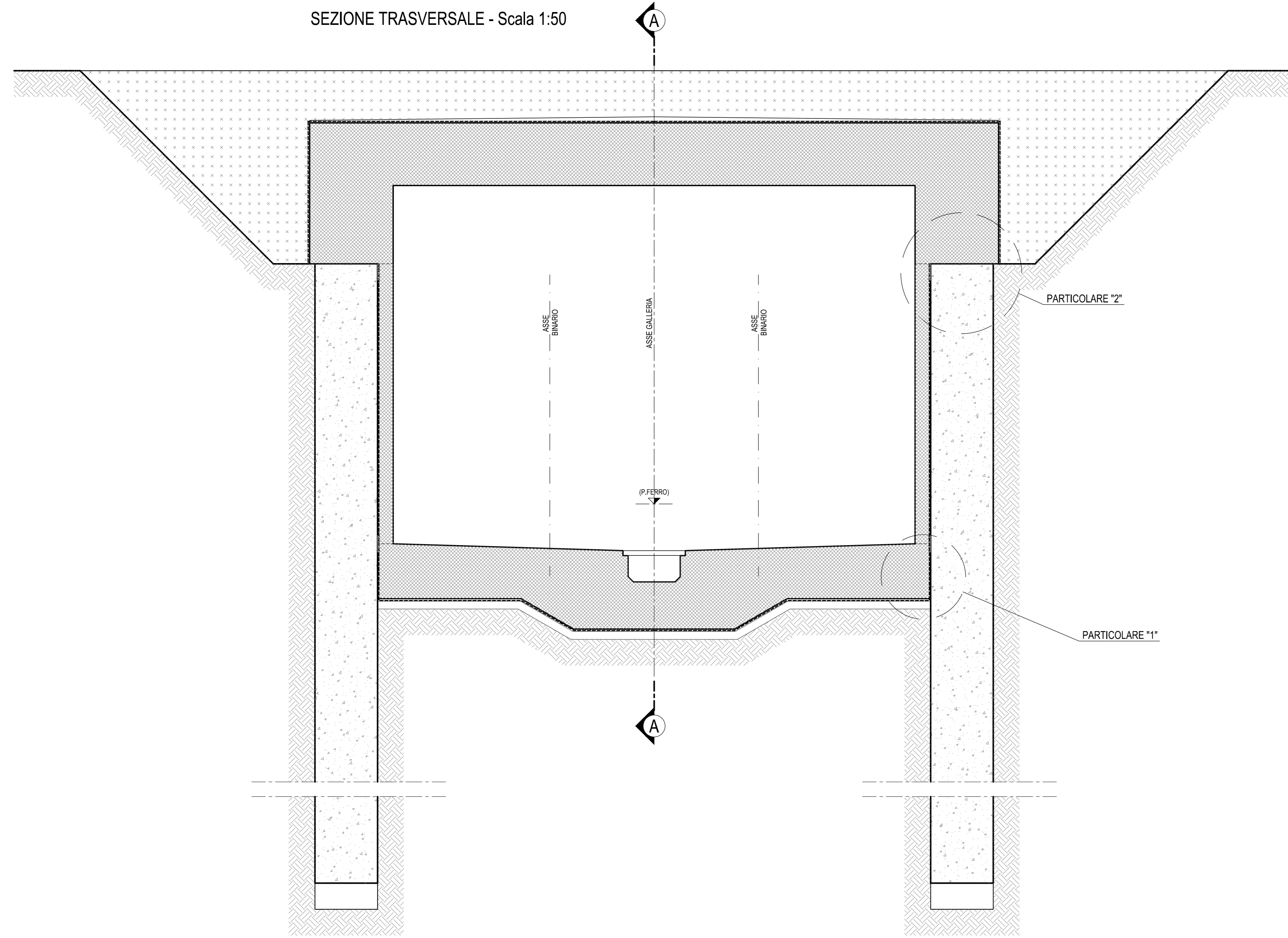
SEZIONE TRASVERSALE - Scala 1:50
