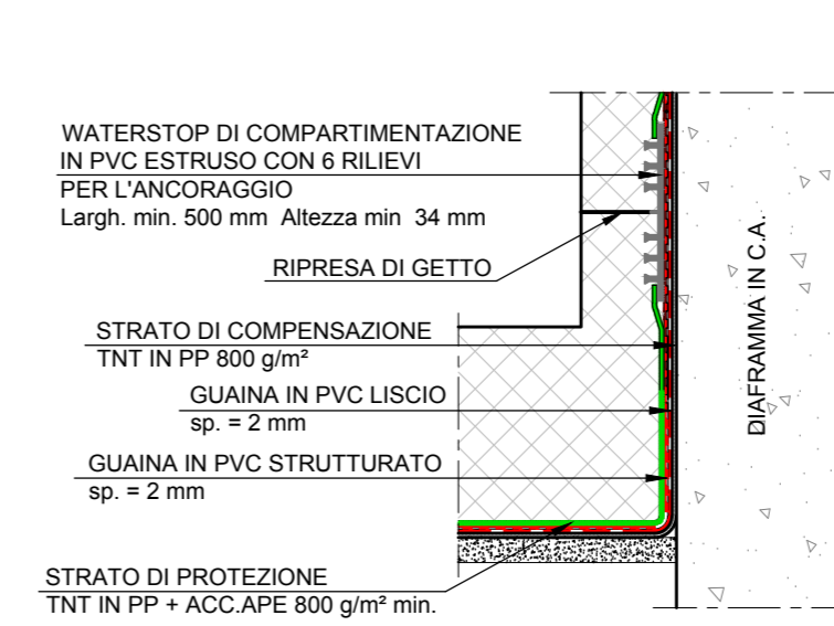
PARTICOLARE 1
