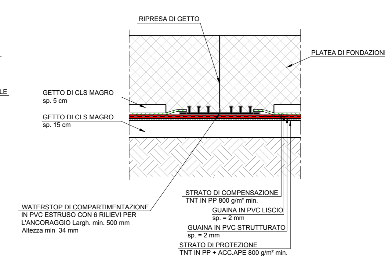
PARTICOLARE 6
