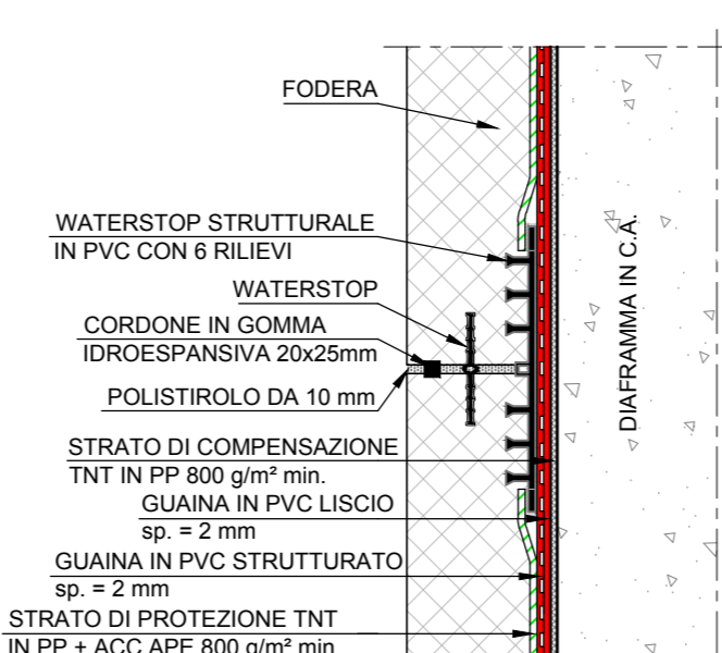
PARTICOLARE 7
