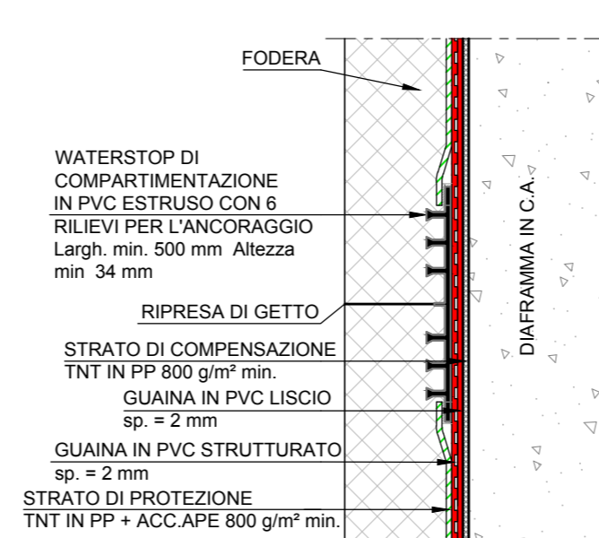
PARTICOLARE 8
