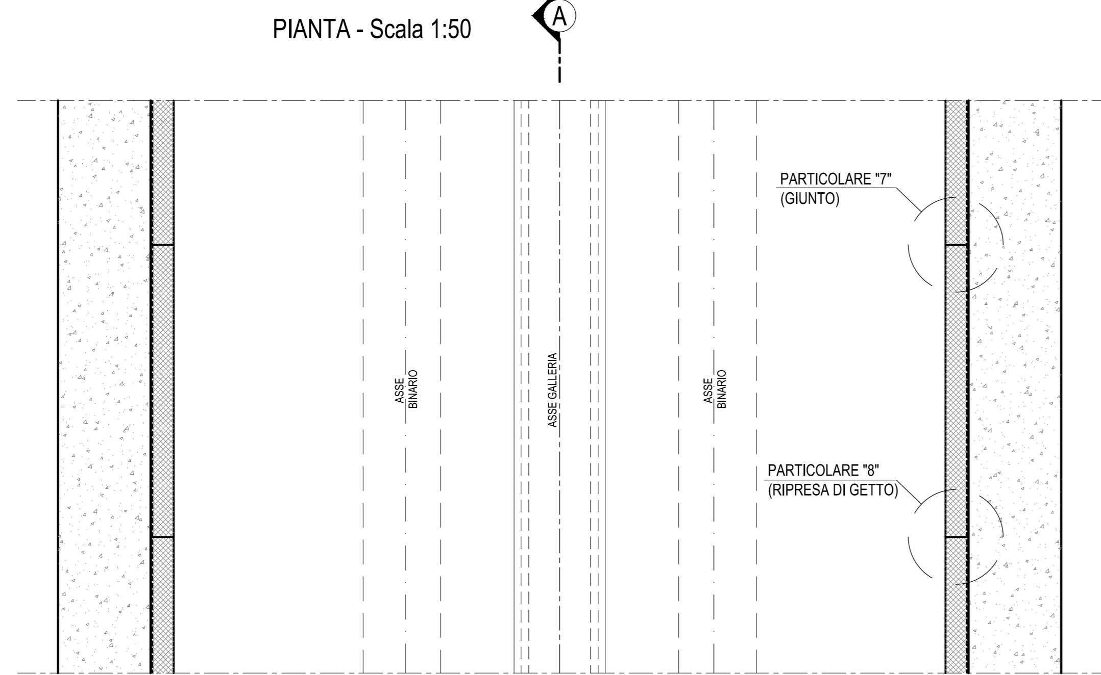
PIANTA - Scala 1:50
