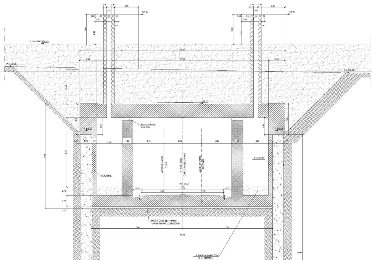
Figura 4. Sezione trasversale
