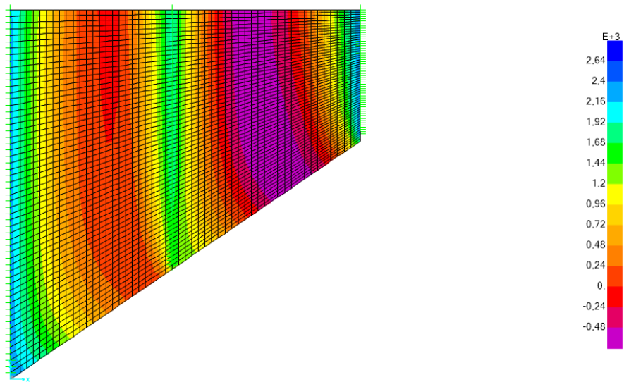
Inviluppo SLE RAR – M_{yy} Max
