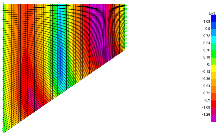
Inviluppo SLE RAR – M_{yy} Min
