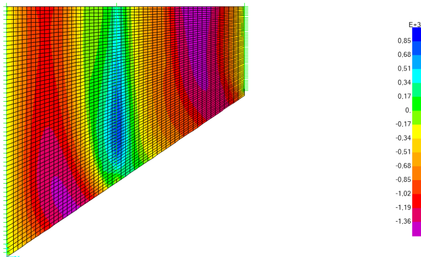
Inviluppo SLU sismiche – M_{yy} Min
