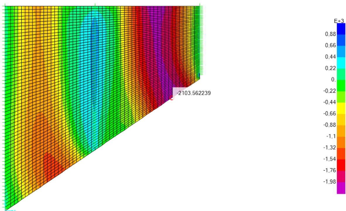
COMB5 – Massimo momento flettente riferito alle direzioni principali di sforzo (cioè somma vettoriale di tutte le componenti flessionali M_{xx} , M_{yy} , M_{xy} )
