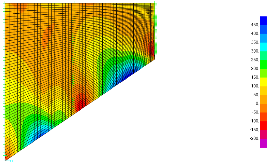
Inviluppo SLE RAR – M_{xy} Max
