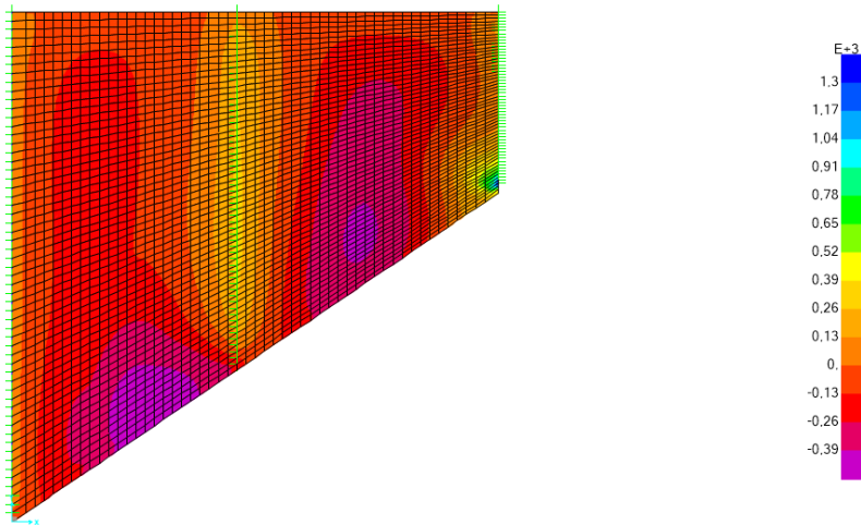
Inviluppo SLU non sismiche – M_{xx} Min
