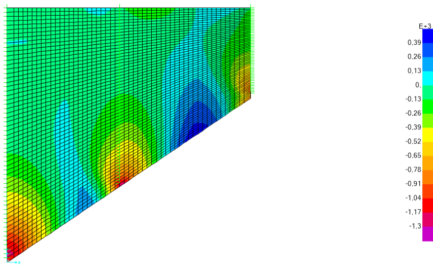
Inviluppo SLU non sismiche – M_{xy} Min
