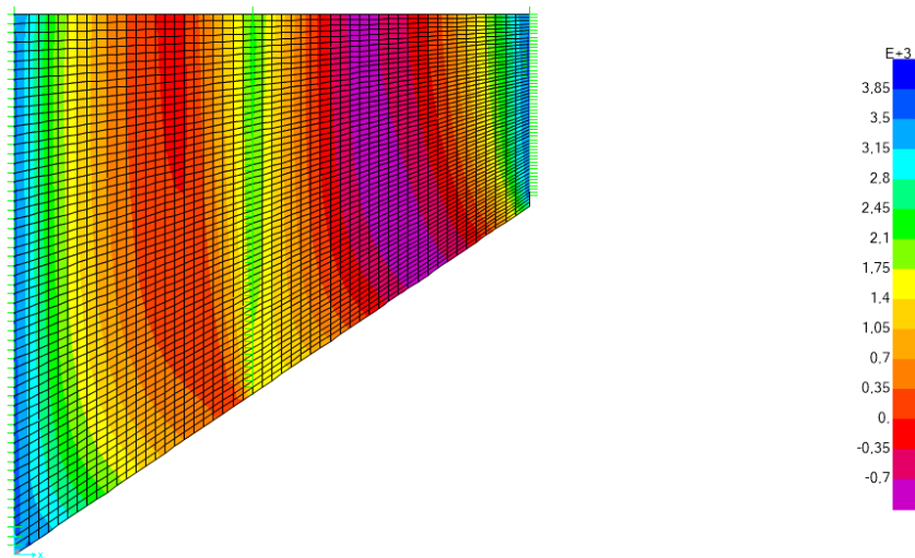
Inviluppo SLU sismiche – M_{yy} Max
