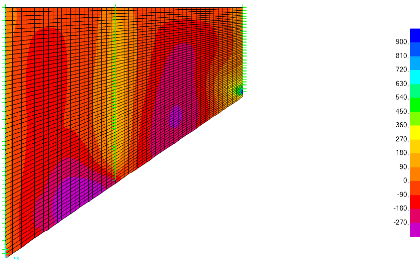
Inviluppo SLE RAR – M_{xx} Min
