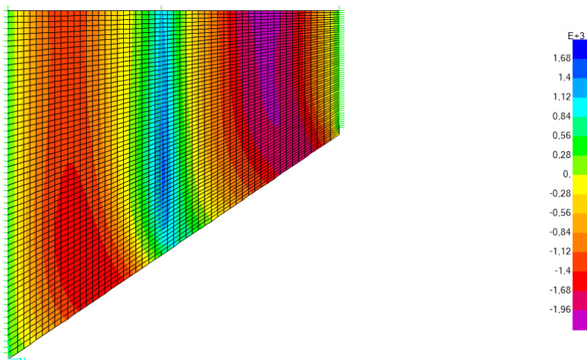
Inviluppo SLU non sismiche – M_{yy} Min
