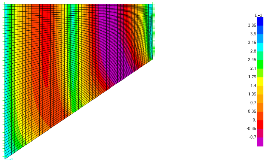
Inviluppo SLU non sismiche – M_{yy} Max
