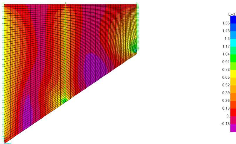
Inviluppo SLU sismiche – M_{xx} Max
