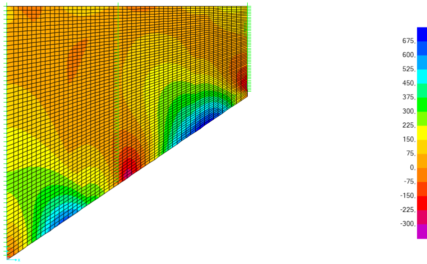
Inviluppo SLU non sismiche – M_{xy} Max
