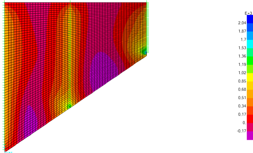
Inviluppo SLU non sismiche – M_{xx} Max
