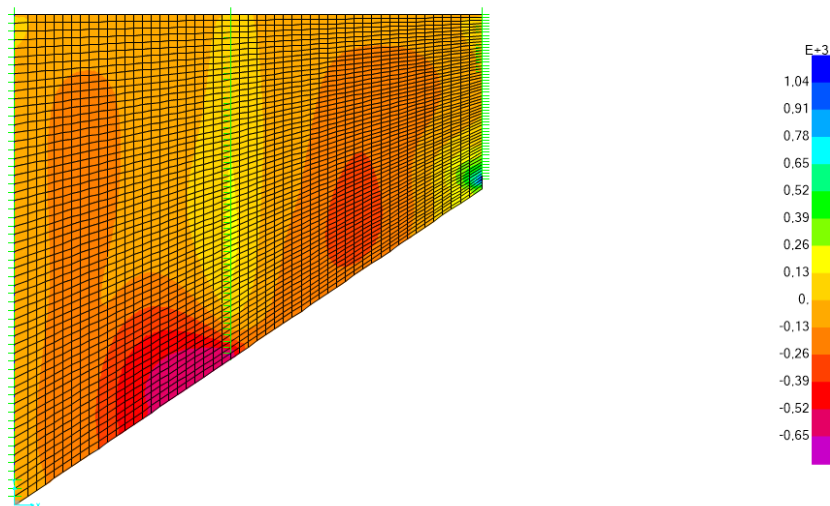
Inviluppo SLU sismiche – M_{xx} Min
