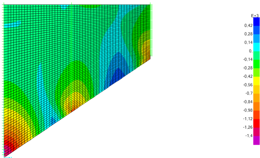
Inviluppo SLU sismiche – M_{xy} Min
