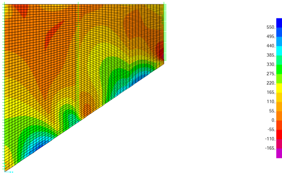
Inviluppo SLU sismiche – M_{xy} Max
