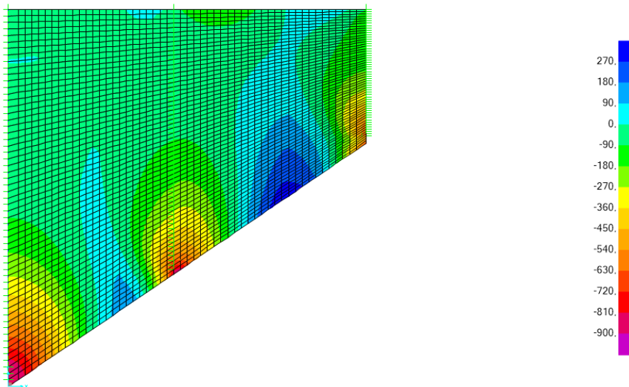
Inviluppo SLE RAR – M_{xy} Min
