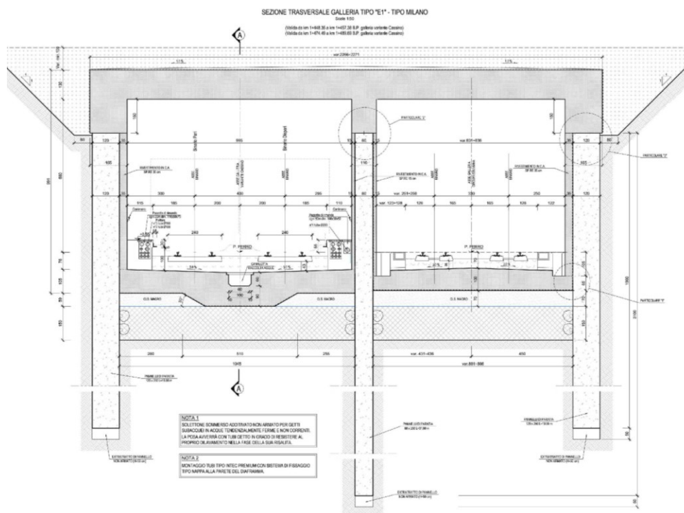
Figura 1 – Sezione trasversale
