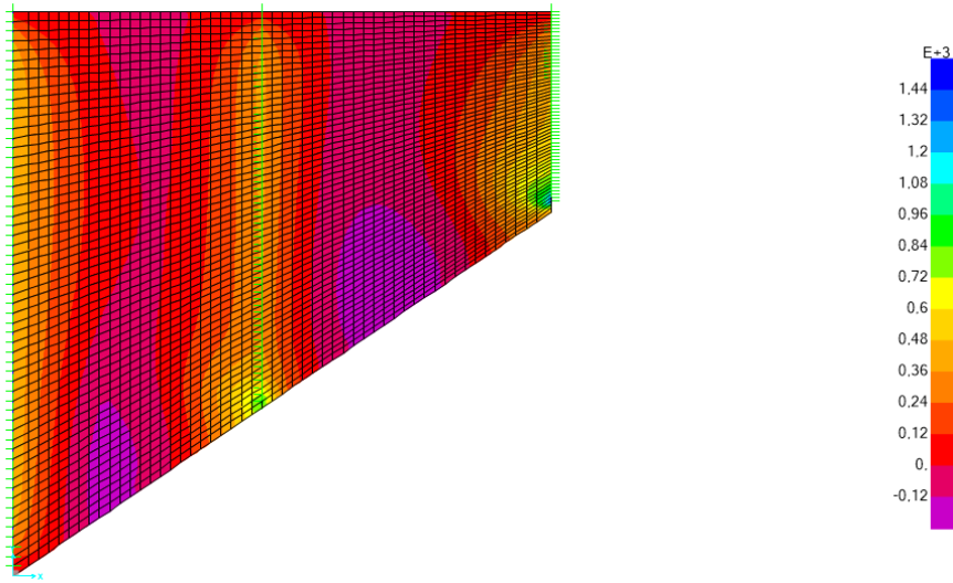
Inviluppo SLE RAR – M_{xx} Max
