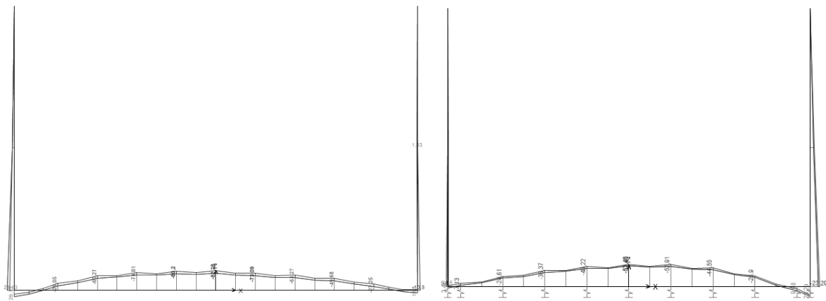
Combinazioni SLE QP - Involuppo – Momento flettente - lato SX e lato DX
