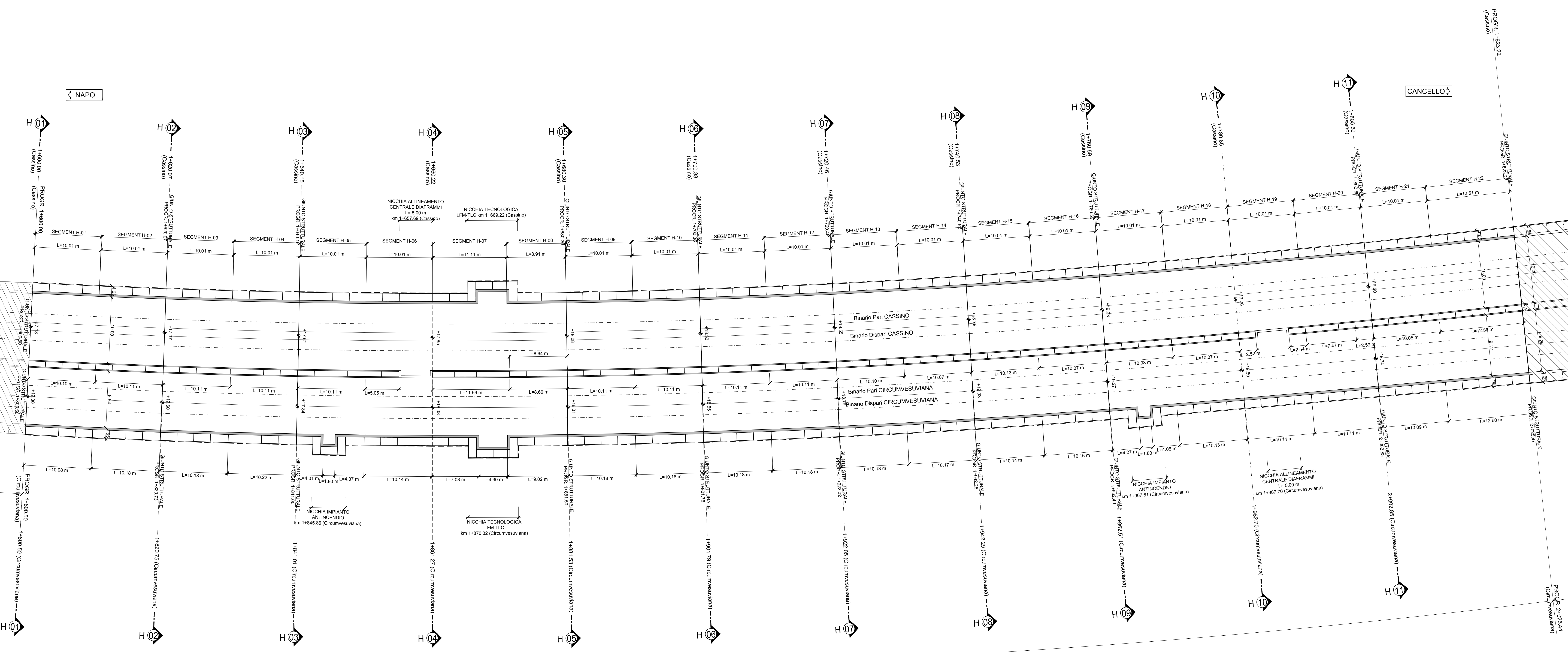
GALLERIA DOPPIA CANNA E DOPPIA ALTEZZA TIPO MILANO L = 223.22 m (SEZIONE TIPO "H")
