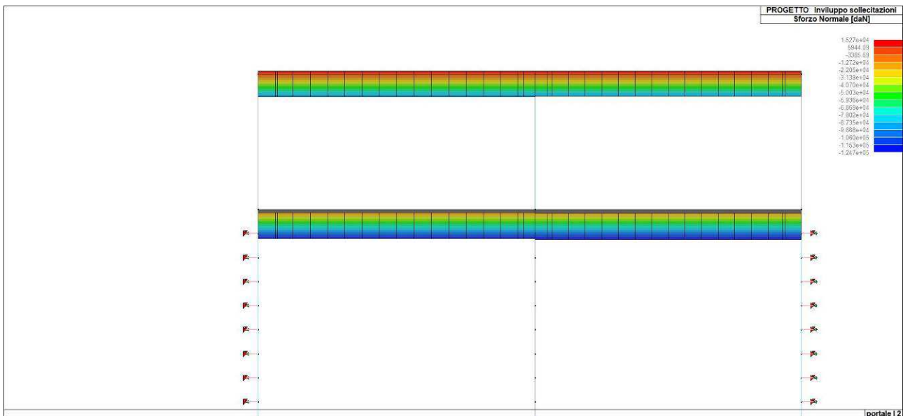
Figura 50. Involuppo dello sforzo normale del solettone di copertura
