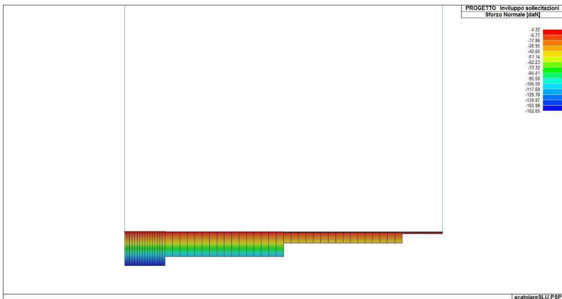
Figura 77. Involuppo dello sforzo normale del solettone di fondazione
