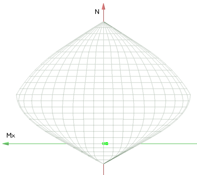
Figura 97. Dominio M-N
