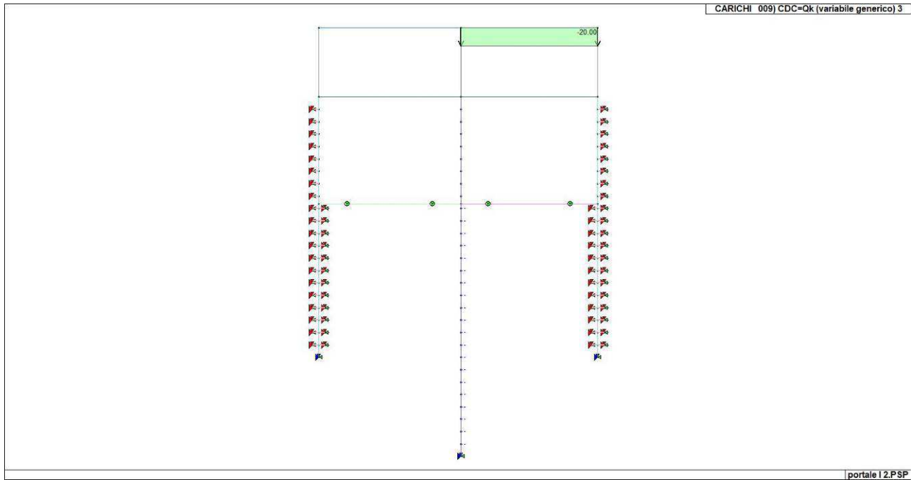
Figura 26. Caso di carico CDC 9 (Accidentale 3)
