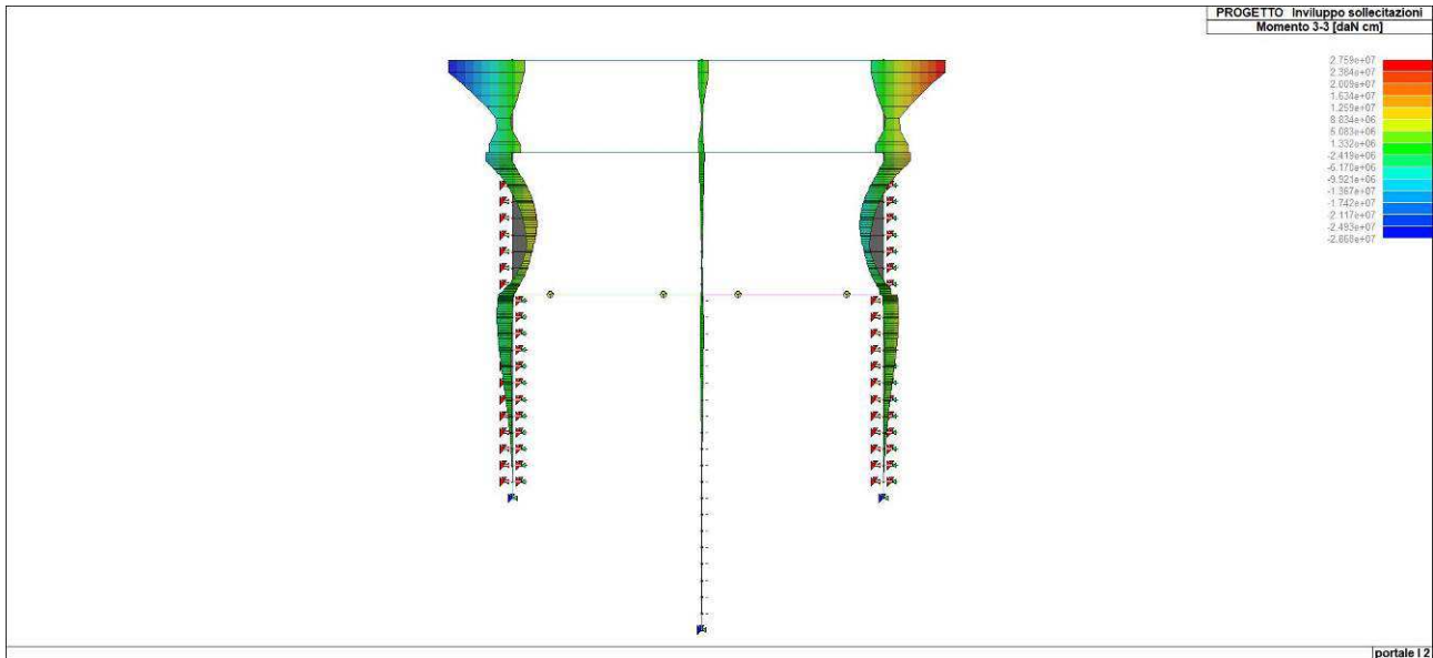
Figura 49. Involuppo del momento flettente di diaframmi e piedritti
