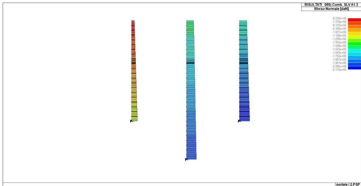
Figura 39. Sforzo normale diaframmi (combinazione 59)
