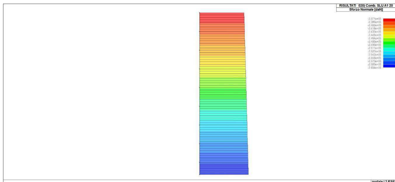
Figura 112. Sforzo normale massimo sul diaframma centrale
