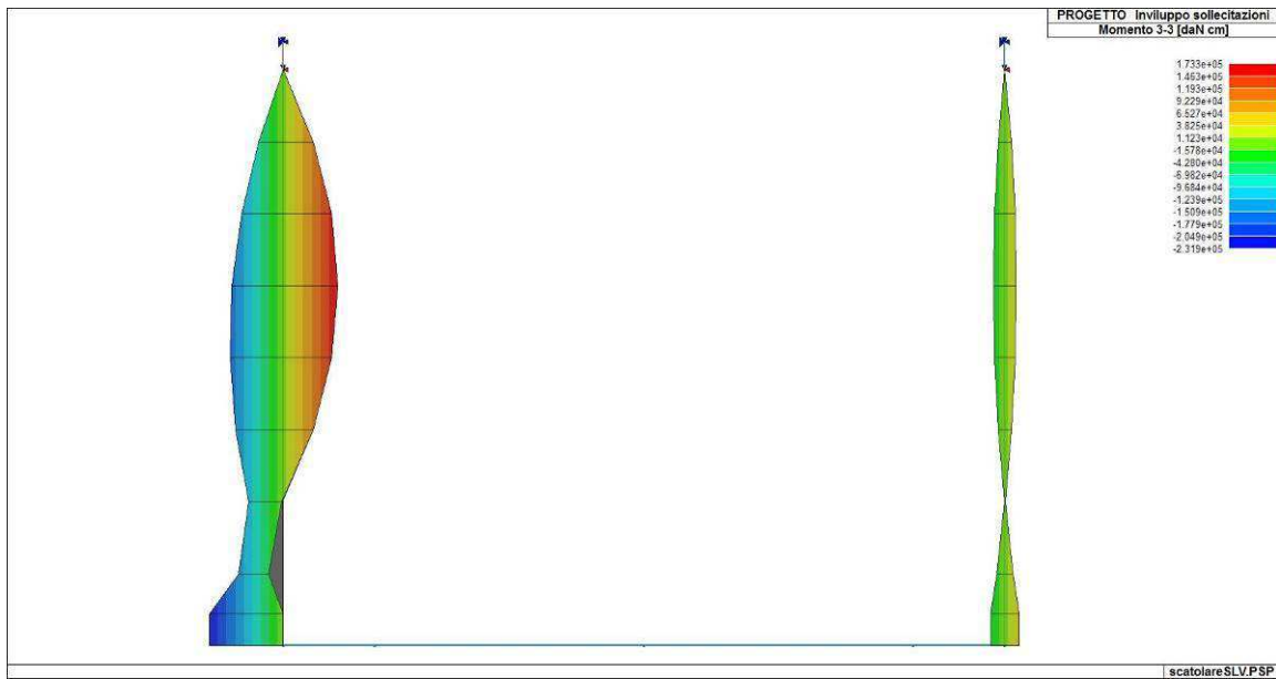
Figura 82. Involuppo del momento flettente delle fodere
