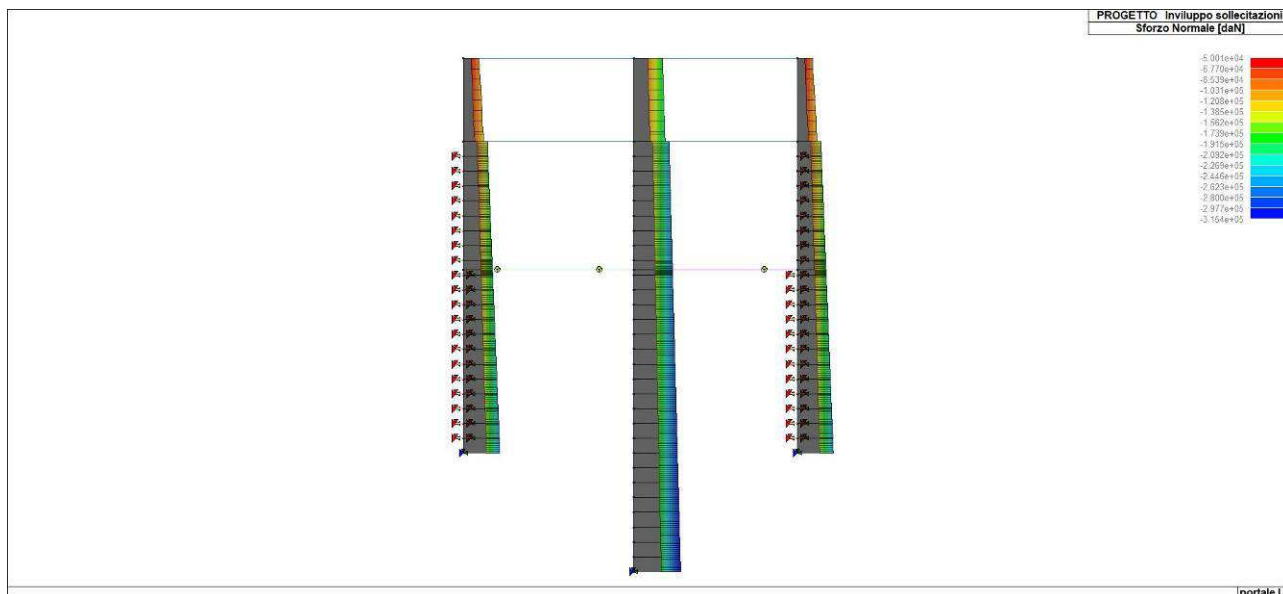
Figura 47. Involuppo dello sforzo normale di diaframmi e piedritti
