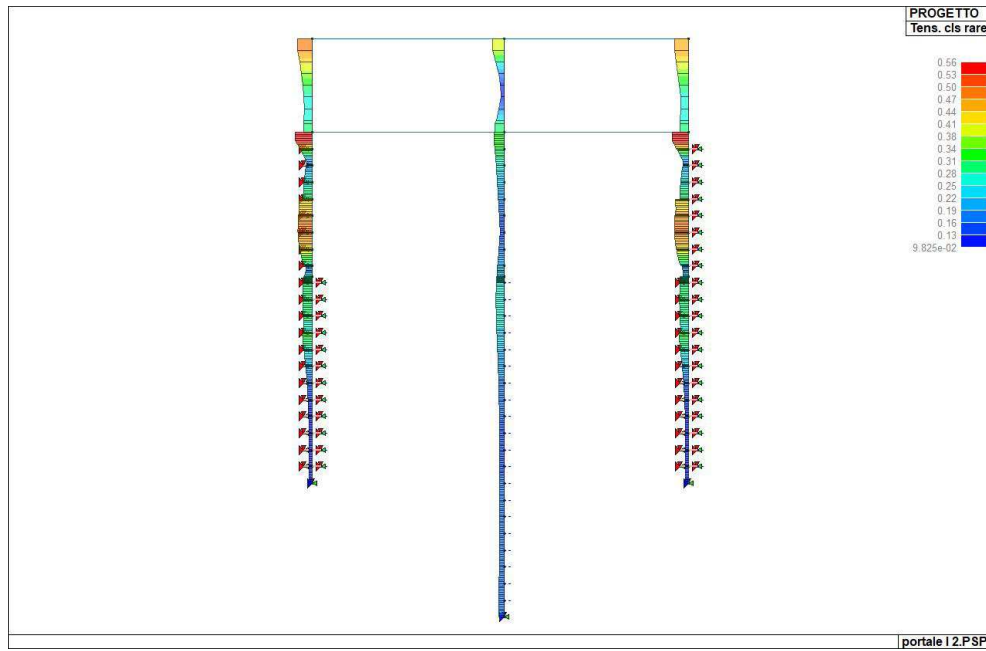
Figura 102. Indice di verifica della tensione del calcestruzzo per combinazioni rare
