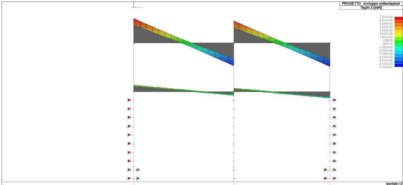
Figura 63. Inviluppo del taglio del solettone di copertura
