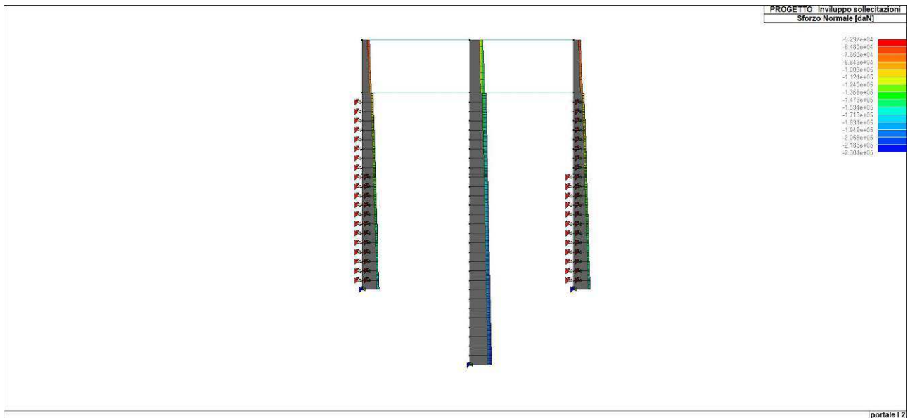
Figura 59. Involuppo dello sforzo normale di diaframmi e piedritti
