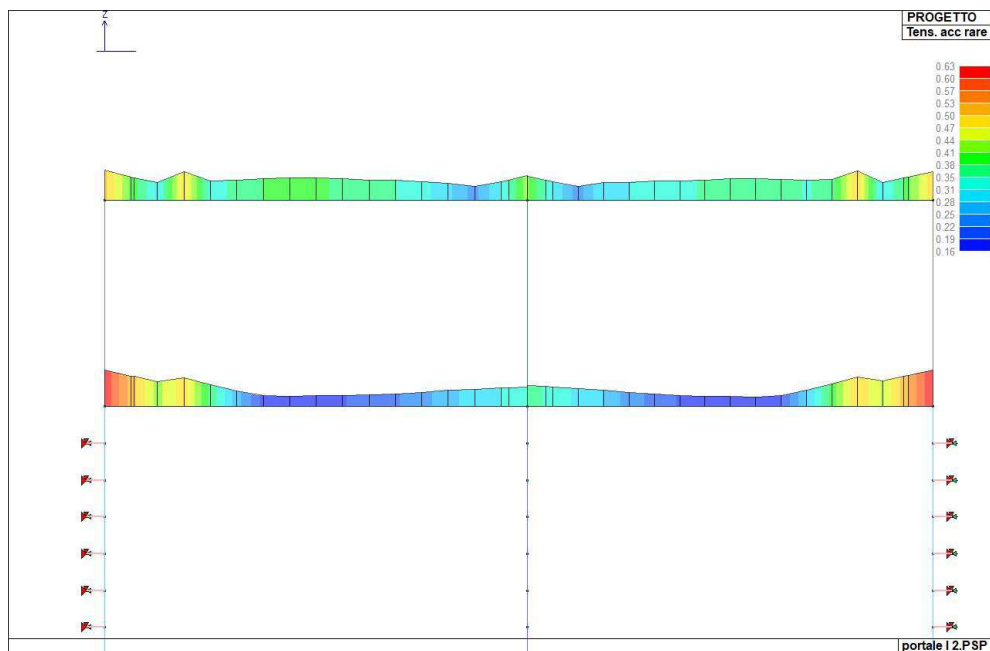
Figura 105. Indice di verifica della tensione dell'acciaio per combinazioni rare
