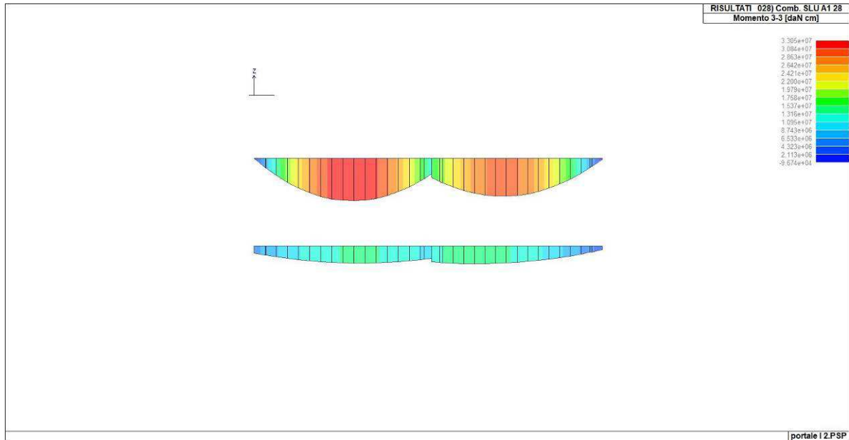
Figura 45. Momento flettente massimo solettone di copertura (combinazione 28)
