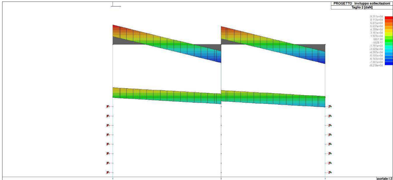
Figura 57. Involuppo del taglio del solettone di copertura
