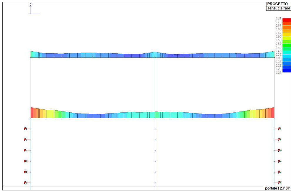
Figura 104. Indice di verifica della tensione del calcestruzzo per combinazioni rare
