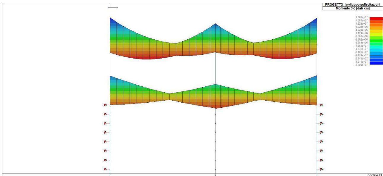
Figura 58. Involuppo del momento flettente del solettone di copertura
