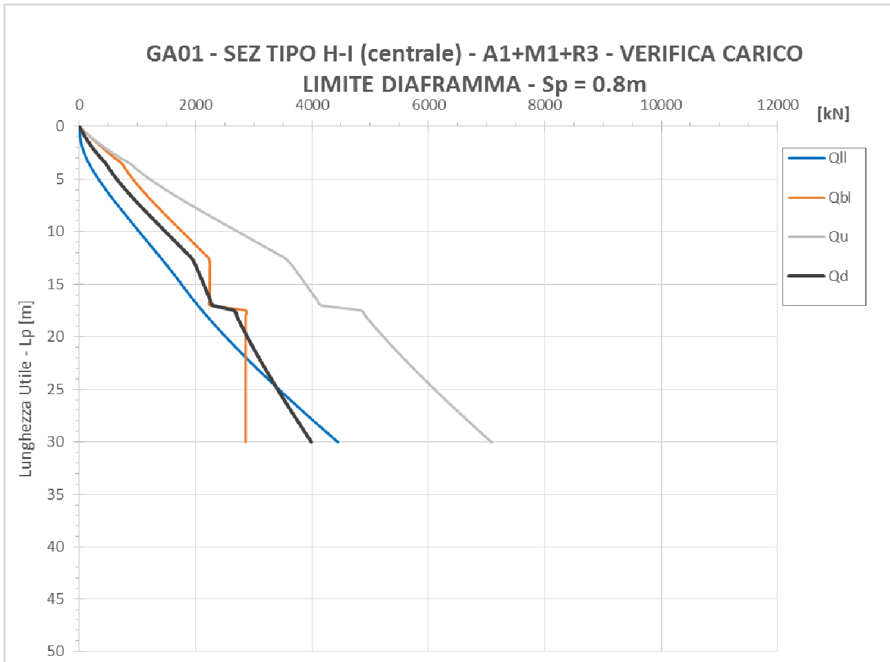
Figura 113. Curva di capacità portante diaframma centrale sezione I
