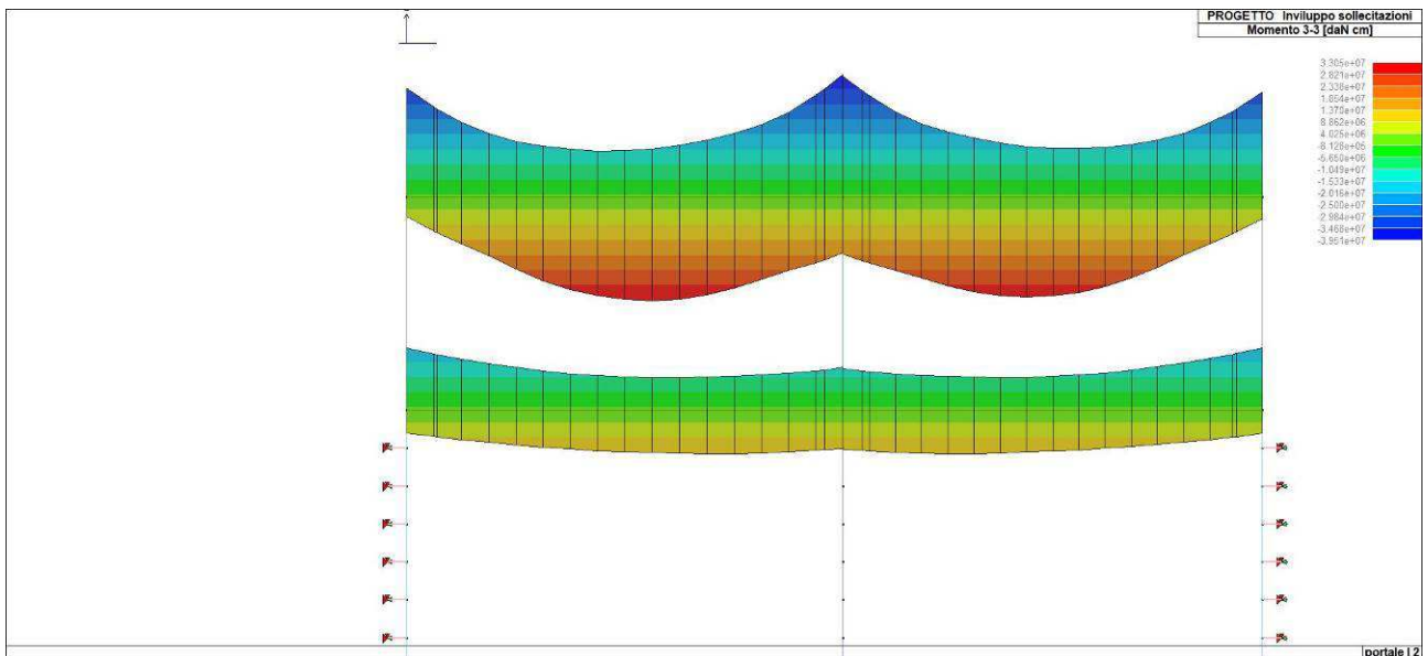
Figura 52. Inviluppo del momento flettente del solettone di copertura
