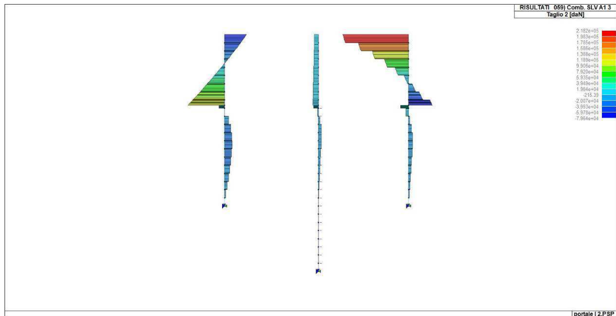
Figura 40. Taglio diaframmi (combinazione 59)
