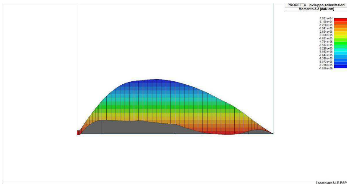
Figura 91. Involuppo del momento flettente del solettone di fondazione
