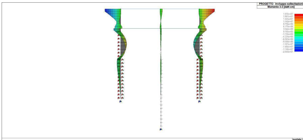
Figura 61. Involuppo del momento flettente di diaframmi e piedritti
