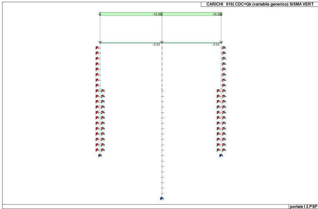
Figura 32. Caso di carico CDC 15 (Sisma verticale)
