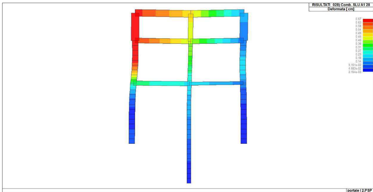
Figura 46. Deformata (combinazione 28)
