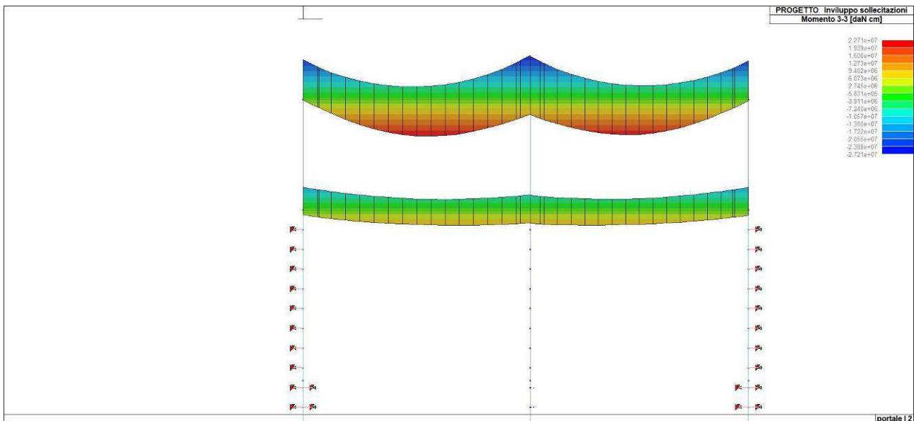
Figura 64. Inviluppo del momento flettente del solettone di copertura
