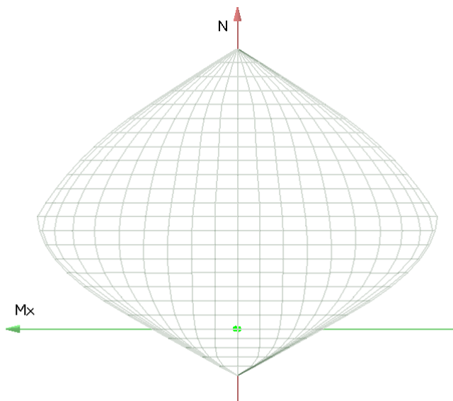
Figura 98. Dominio M-N
