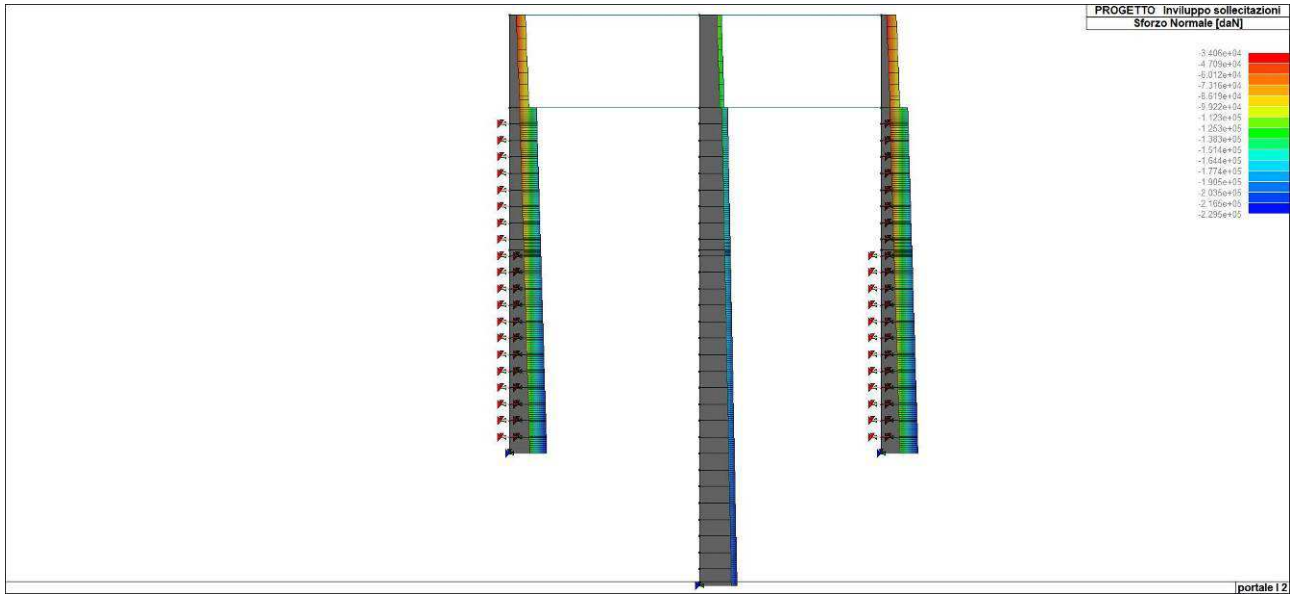
Figura 53. Involuppo dello sforzo normale di diaframmi e piedritti
