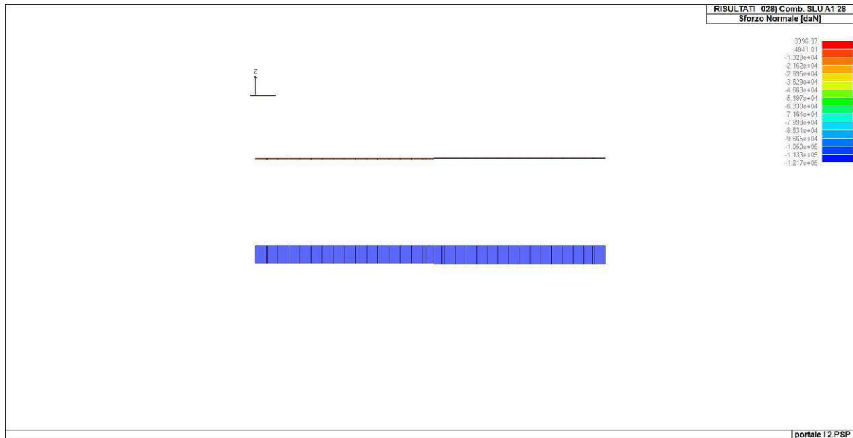
Figura 43. Sforzo normale solettone di copertura (combinazione 28)
