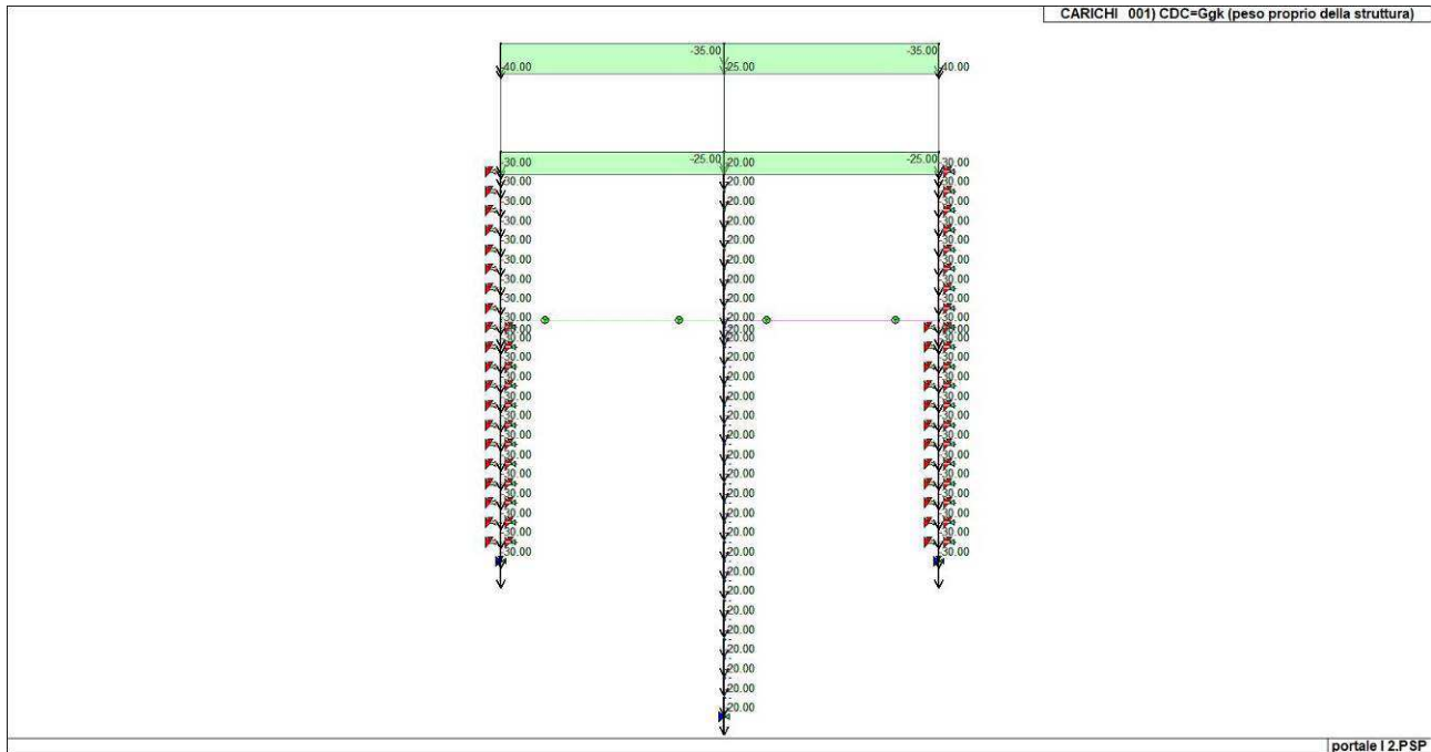
Figura 18. Caso di carico CDC 1 (peso proprio della struttura)
