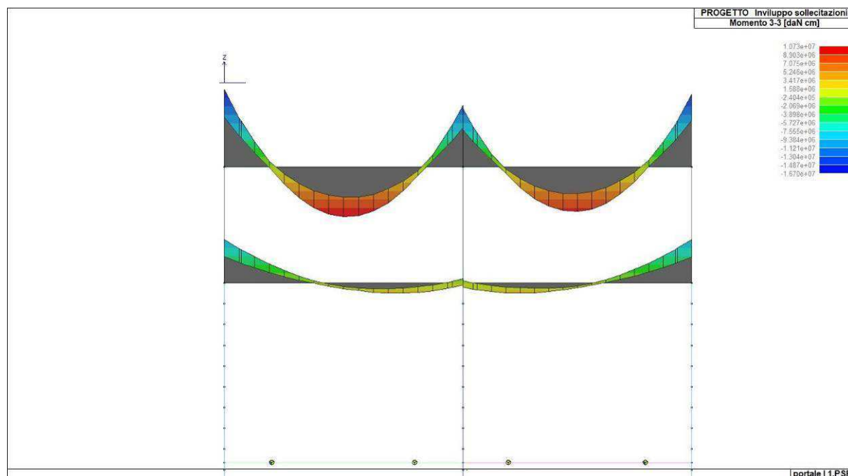
Figura 38. Involuppo del momento flettente del solettone di copertura
