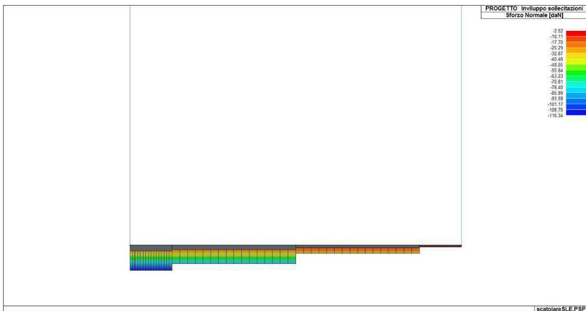
Figura 89. Involuppo dello sforzo normale del solettone di fondazione
