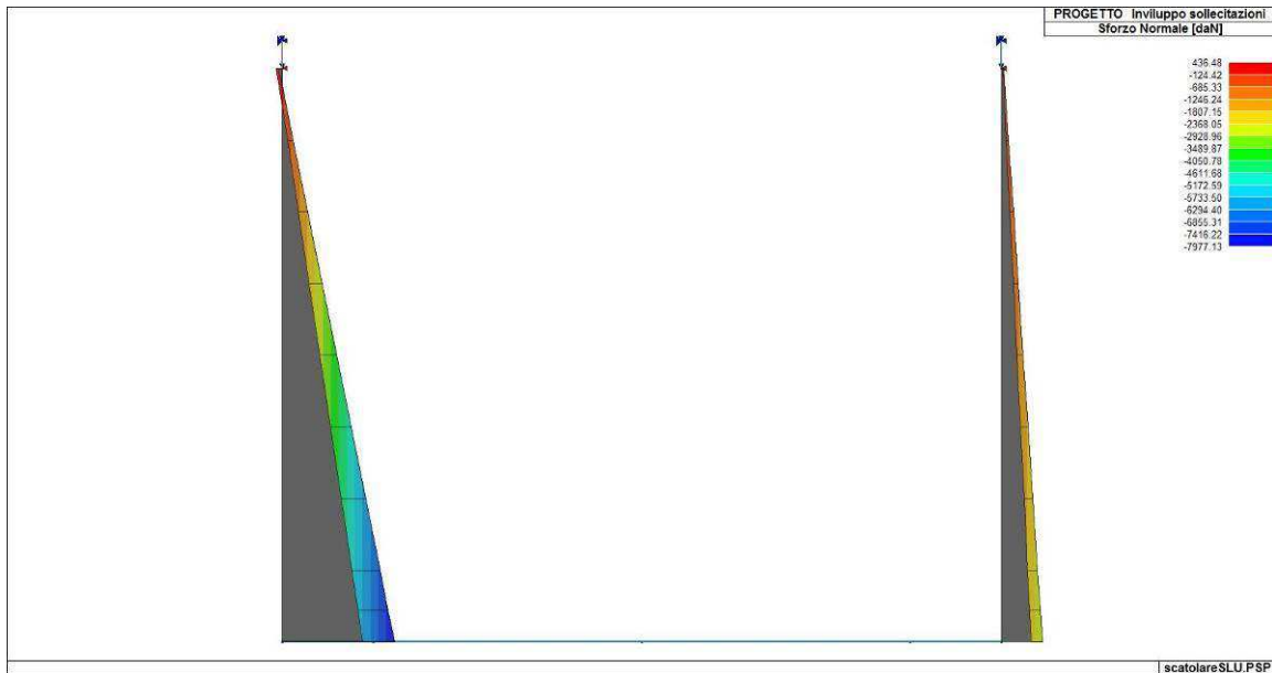
Figura 74. Involuppo dello sforzo normale delle fodere
