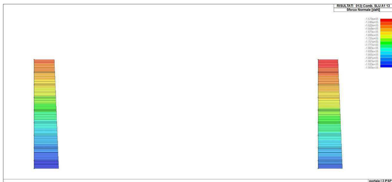
Figura 110. Sforzo normale massimo sui diaframmi laterali
