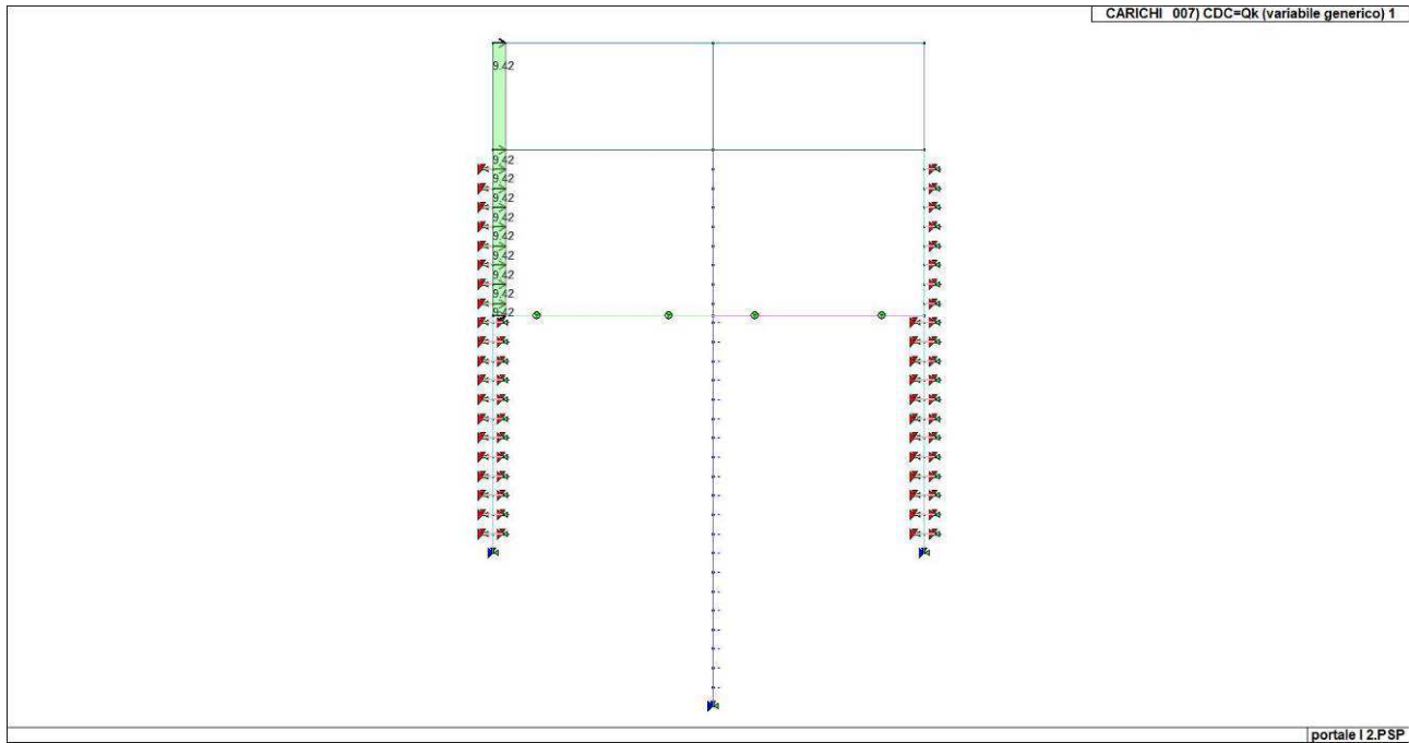
Figura 24. Caso di carico CDC 7 (Accidentale 1)
