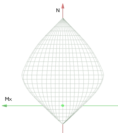
Figura 99. Dominio M-N
