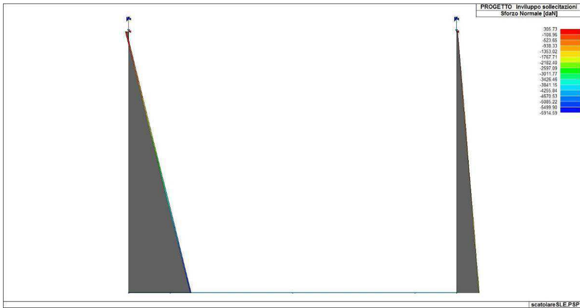
Figura 86. Inviluppo dello sforzo normale delle fodere
