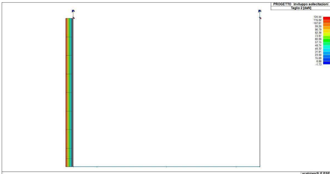
Figura 87. Inviluppo del taglio delle fodere
