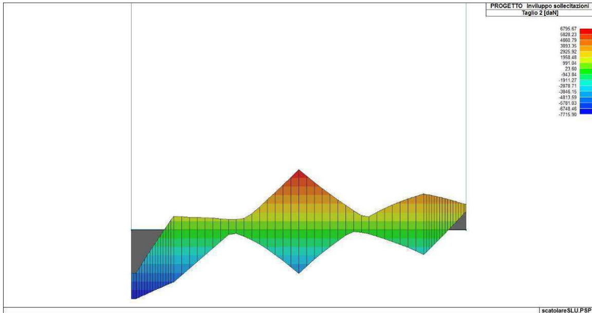
Figura 78. Involuppo del taglio del solettone di fondazione
