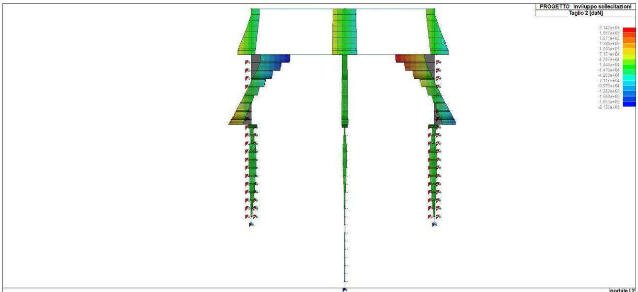
Figura 54. Involuppo del taglio di diaframmi e piedritti
