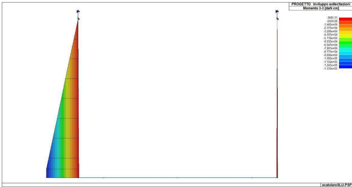
Figura 76. Involuppo del momento flettente delle fodere
