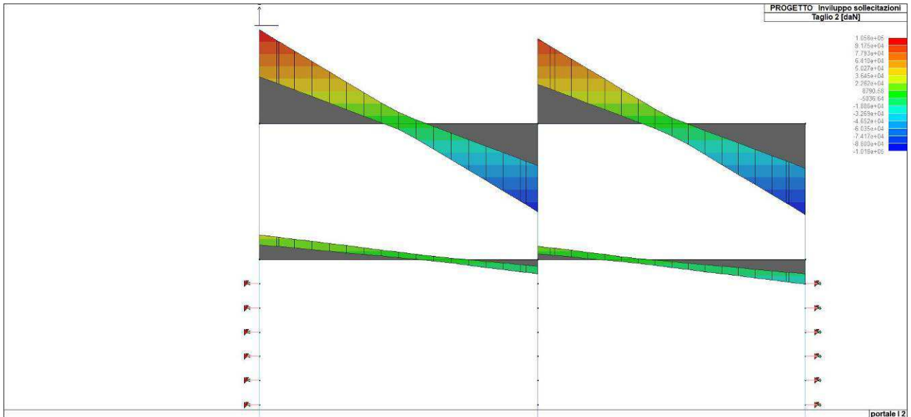
Figura 51. Inviluppo del taglio del solettone di copertura
