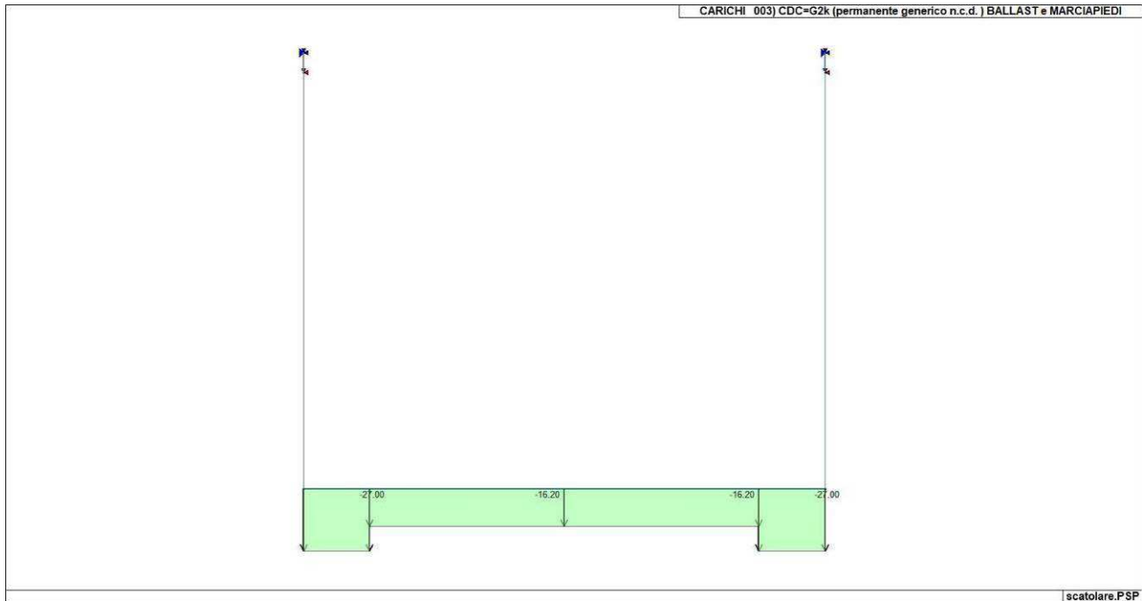
Figura 69. Caso di carico CDC 3 (Permanente ballast e marciapiedi)
