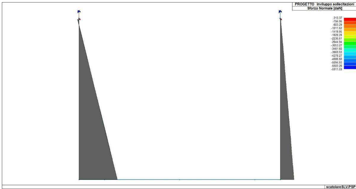
Figura 80. Involuppo dello sforzo normale delle fodere
