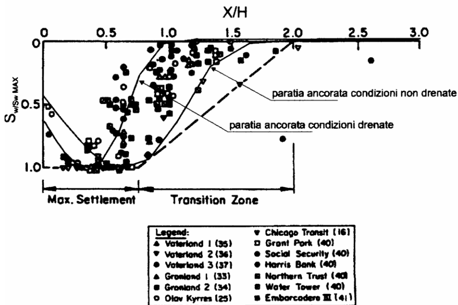
Figura 117. Profili di subsidenza normalizzati (Pane & Tamagnini, 1997 Mana & Clough, 1981)
