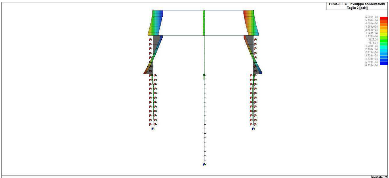
Figura 60. Involuppo del taglio di diaframmi e piedritti
