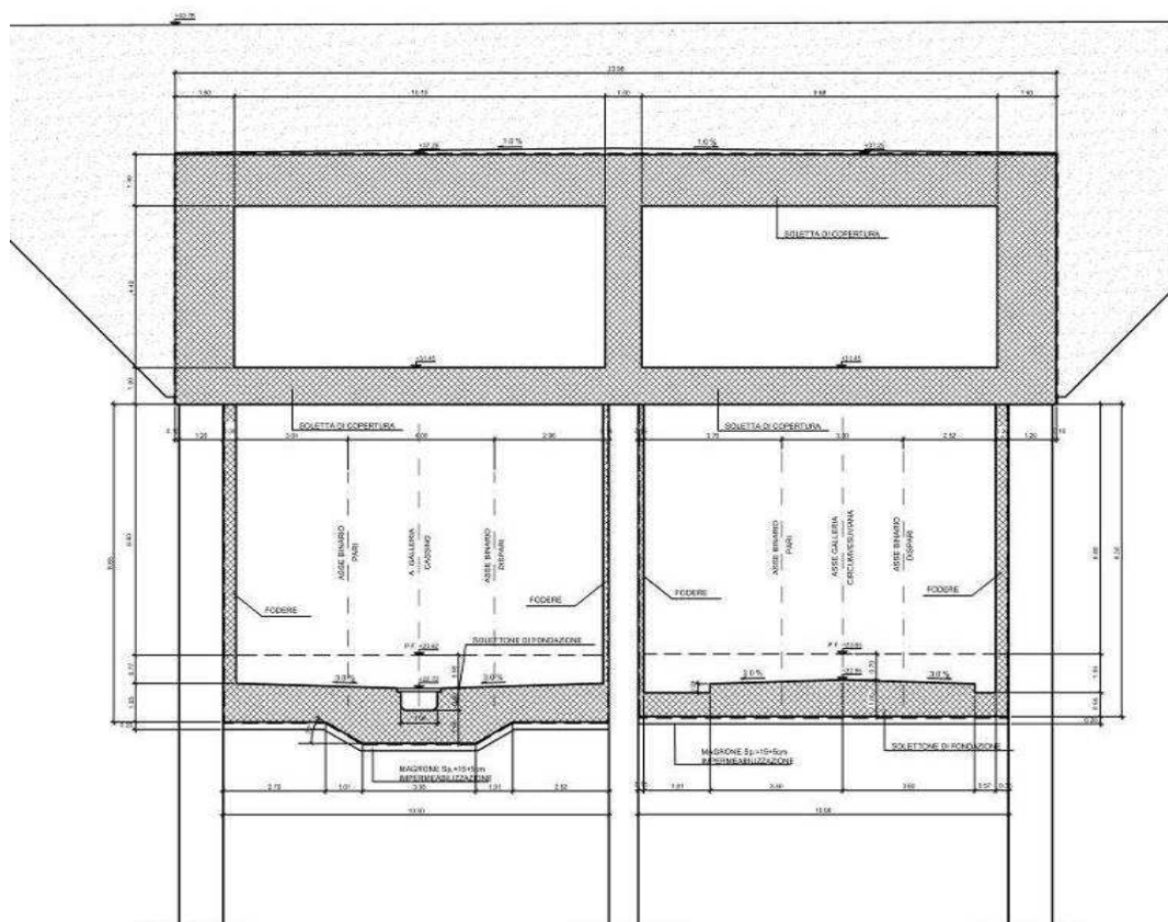
Figura 6. Sezione trasversale
