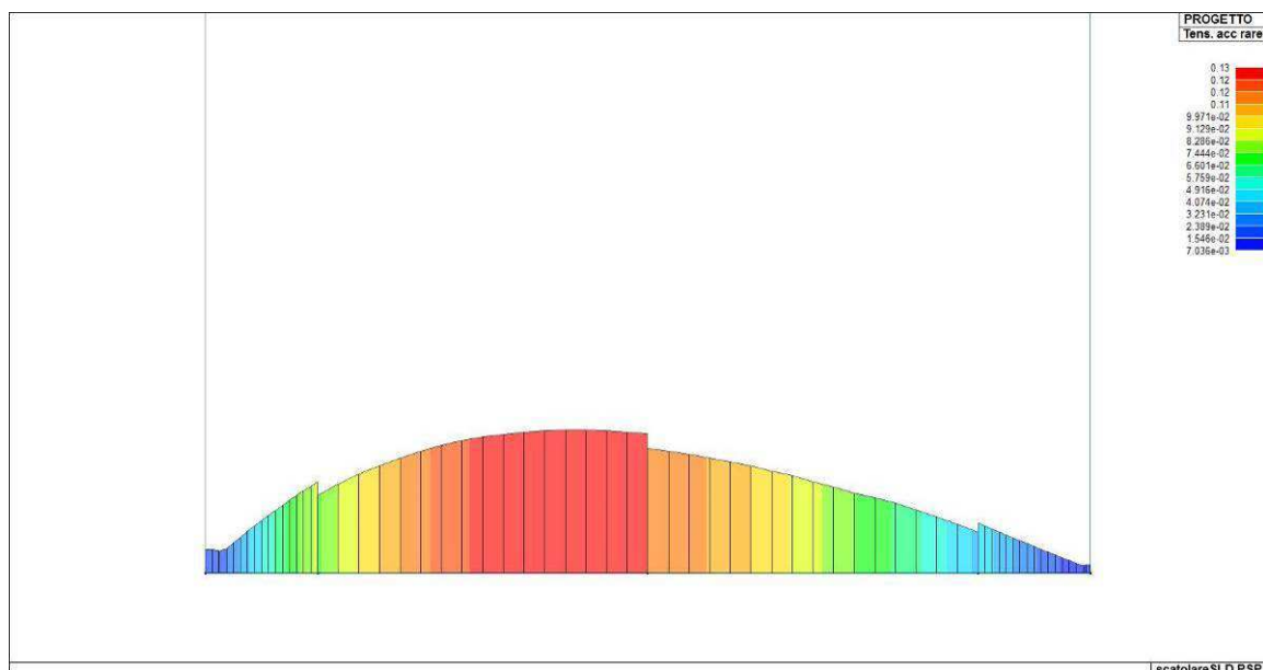
Figura 109. Indice di verifica della tensione dell'acciaio per combinazioni rare
