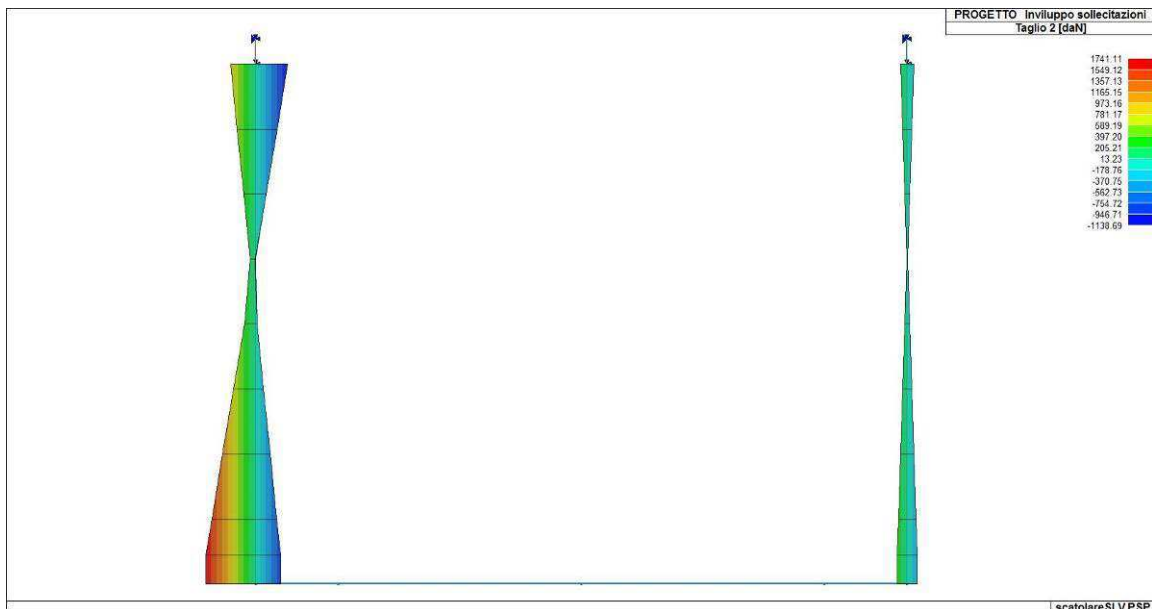
Figura 81. Involuppo del taglio delle fodere
