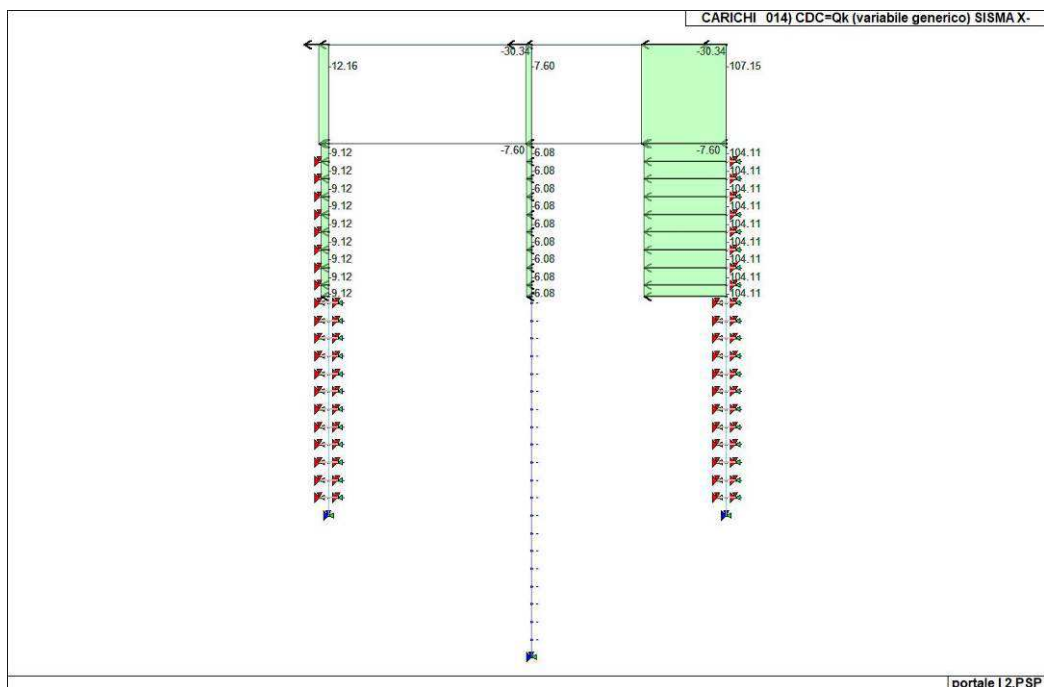
Figura 31. Caso di carico CDC 14 (Sisma X-)
