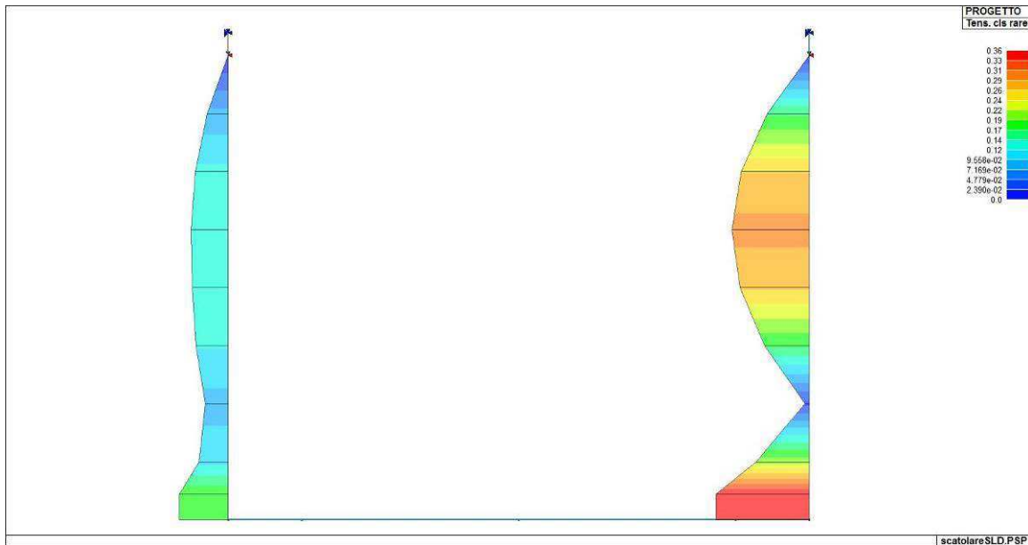
Figura 106. Indice di verifica della tensione del calcestruzzo per combinazioni rare
