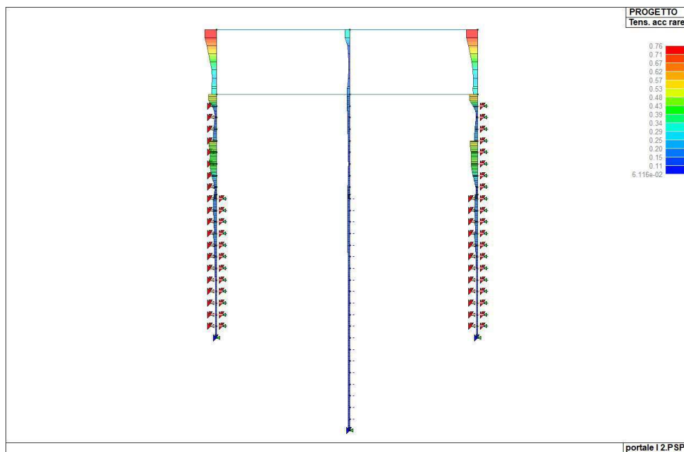
Figura 103. Indice di verifica della tensione dell'acciaio per combinazioni rare
