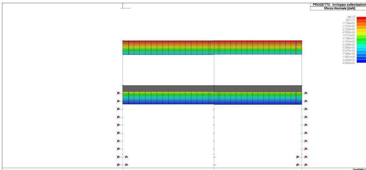
Figura 62. Involuppo dello sforzo normale del solettone di copertura
