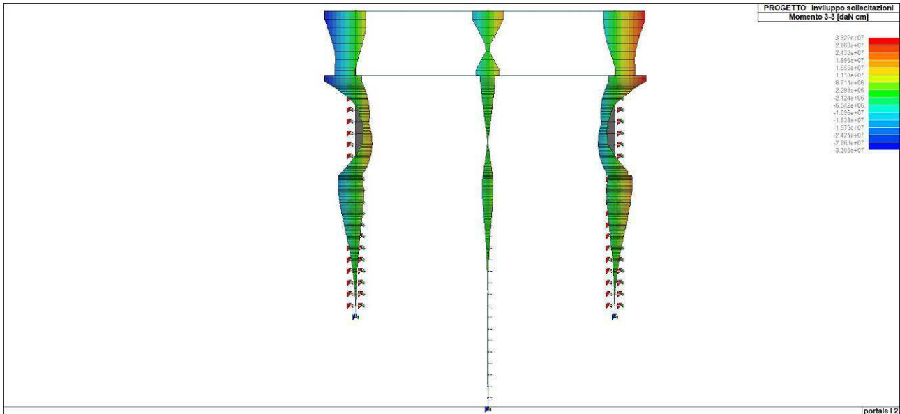
Figura 55. Involuppo del momento flettente di diaframmi e piedritti
