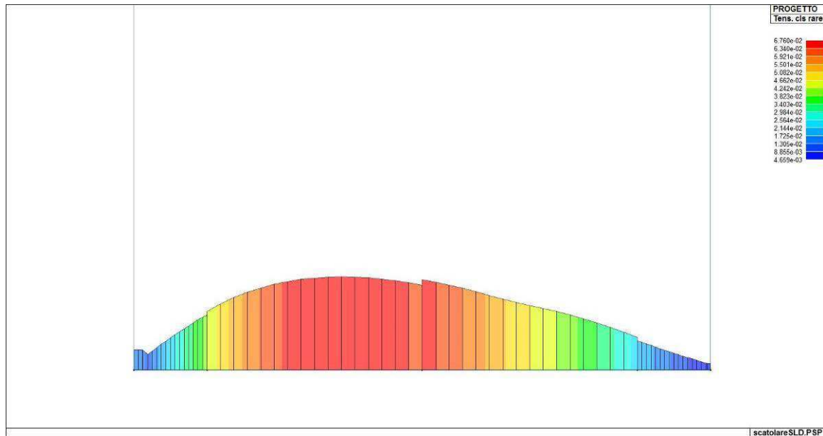
Figura 108. Indice di verifica della tensione del calcestruzzo per combinazioni rare
