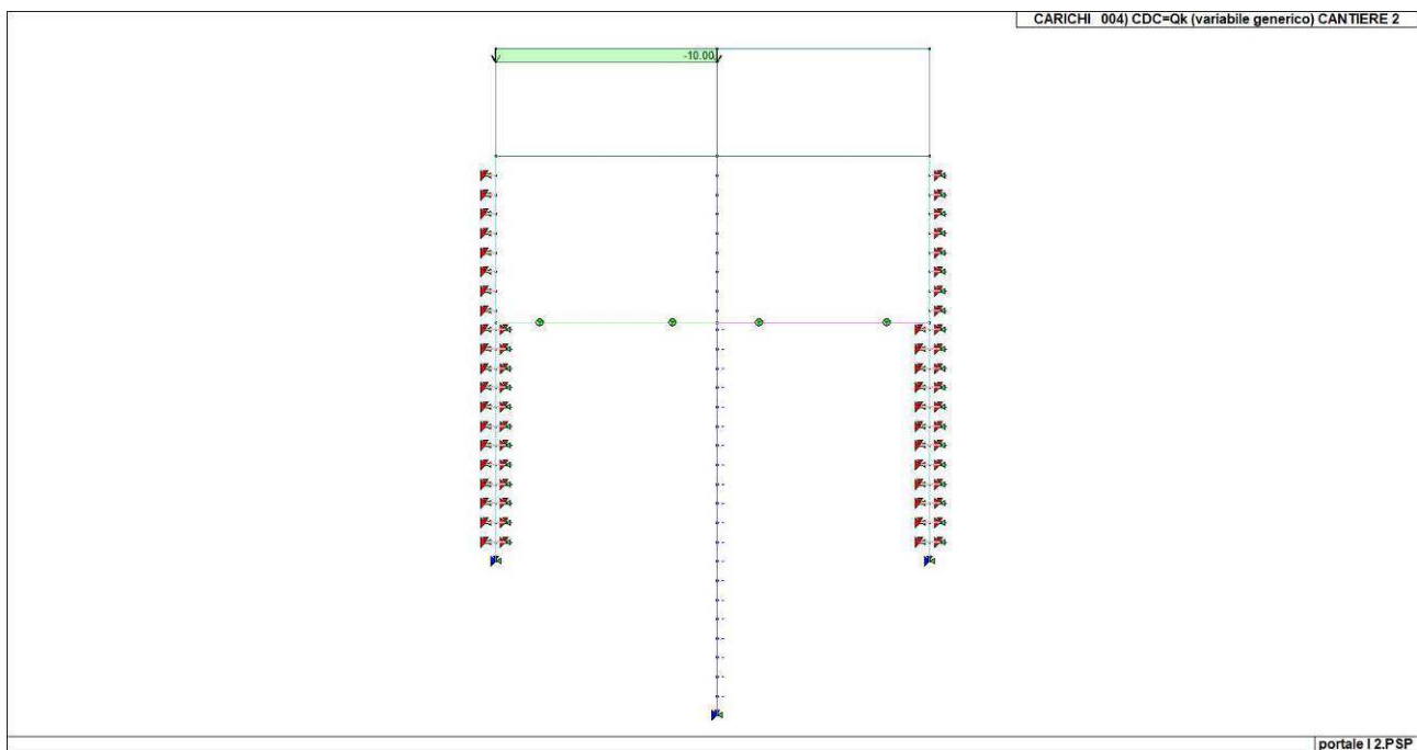
Figura 21. Caso di carico CDC 4 (Cantiere 2)
