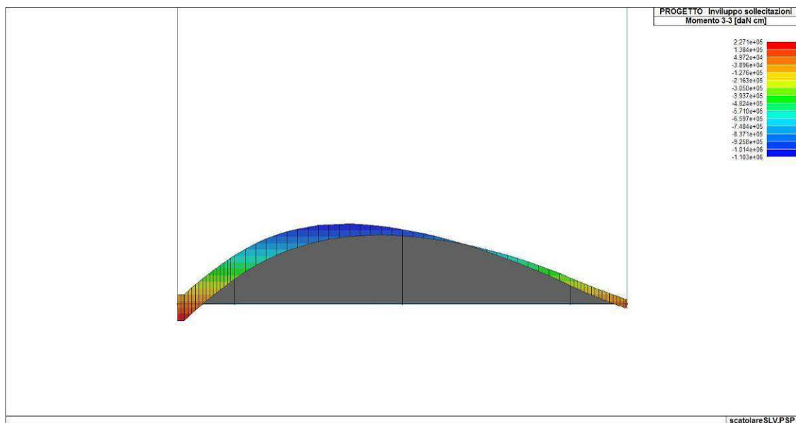
Figura 85. Involuppo del momento flettente del solettone di fondazione
