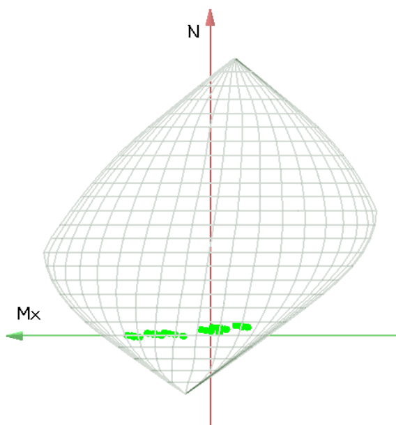
Figura 93. Dominio M-N
