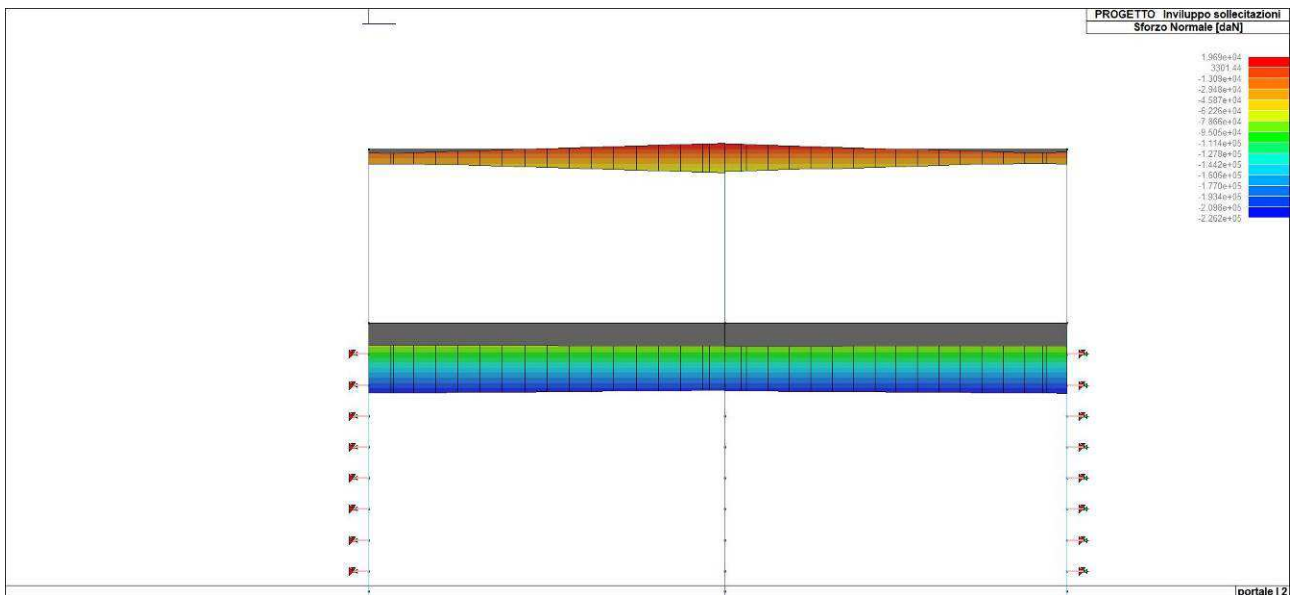
Figura 56. Involuppo dello sforzo normale del solettone di copertura
