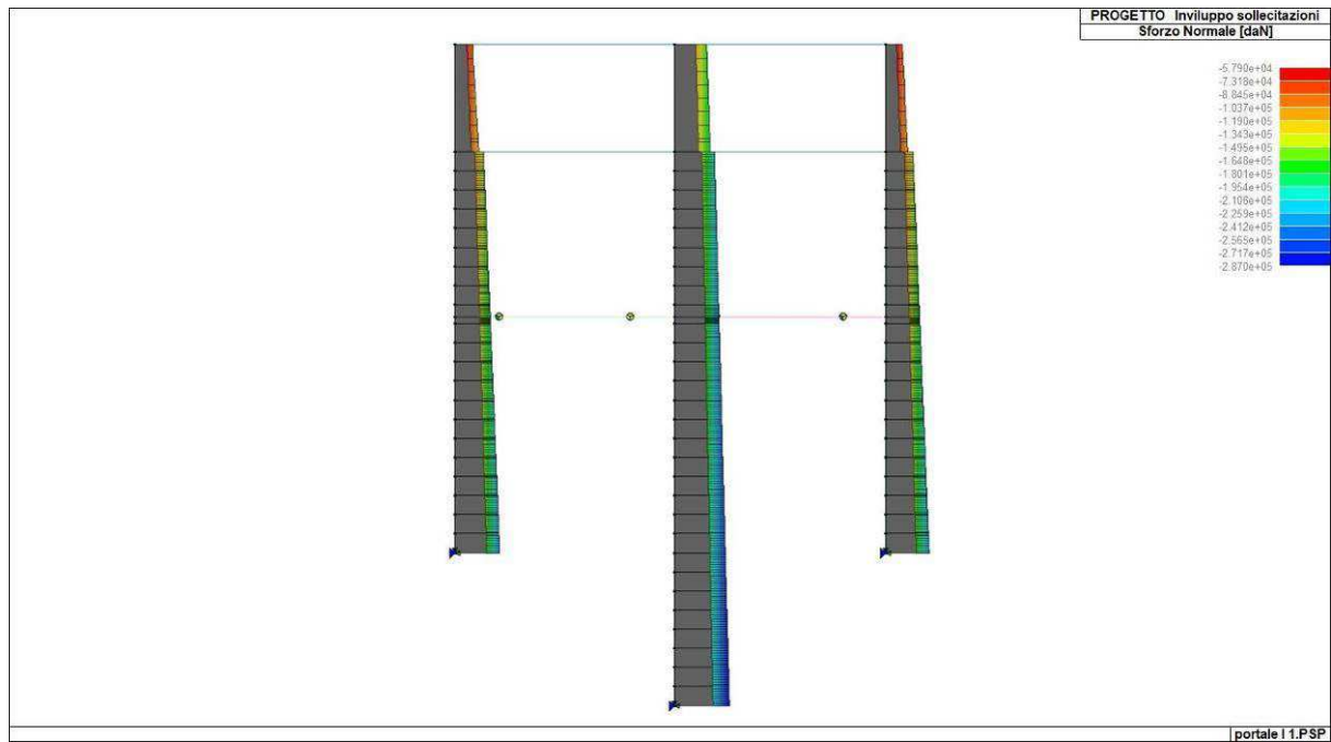
Figura 33. Inviluppo dello sforzo normale di diaframmi e piedritti
