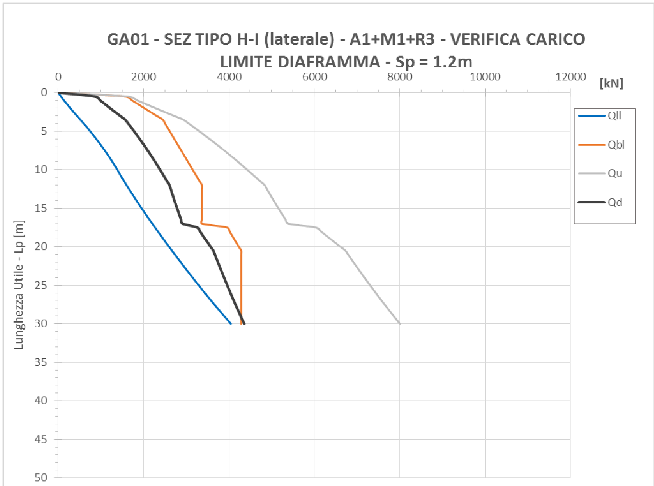
Figura 111. Curva di capacità portante diaframma laterale sezione I
