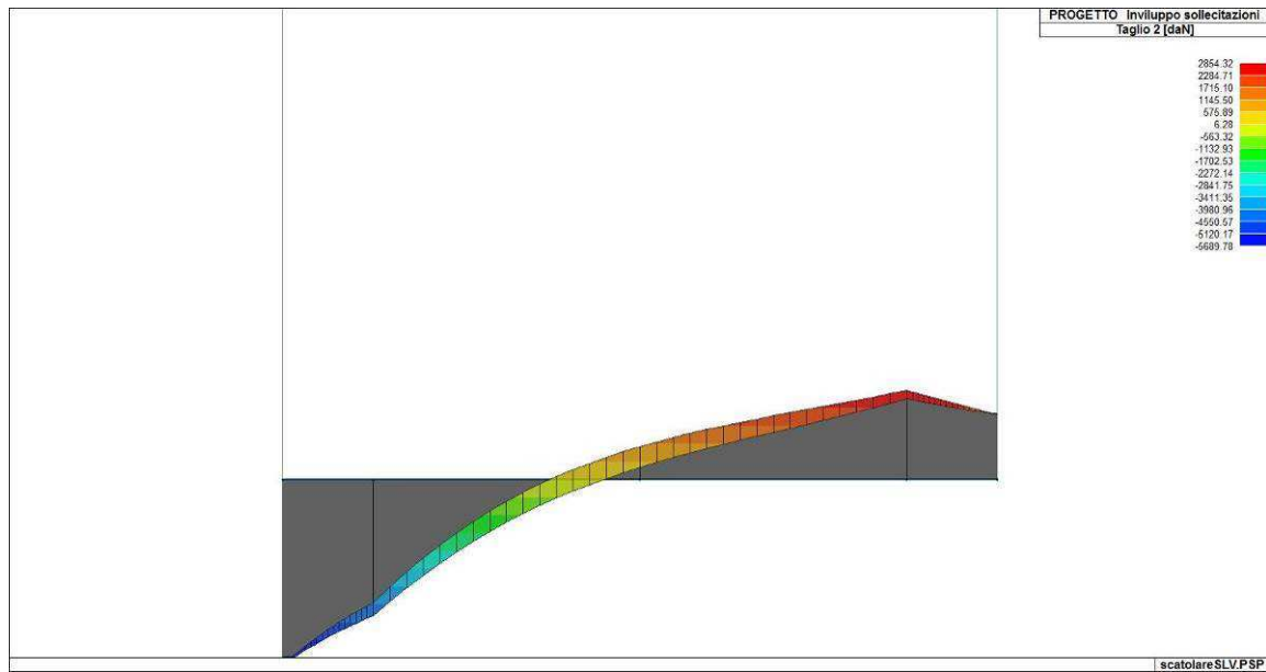
Figura 84. Involuppo del taglio del solettone di fondazione
