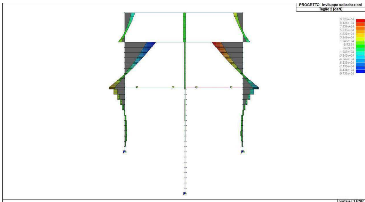
Figura 34. Inviluppo del taglio di diaframmi e piedritti
