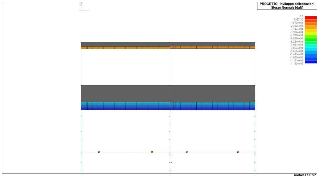
Figura 36. Involuppo dello sforzo normale del solettone di copertura
