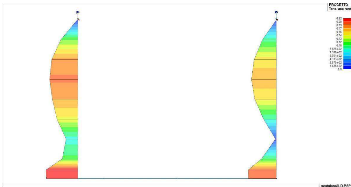
Figura 107. Indice di verifica della tensione dell'acciaio per combinazioni rare
