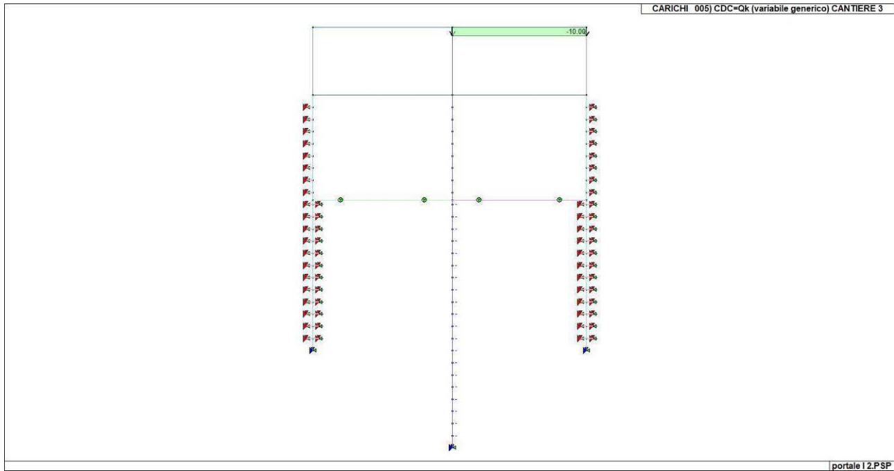
Figura 22. Caso di carico CDC 5 (Cantiere 3)
