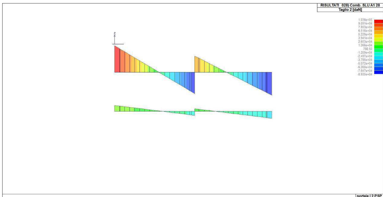
Figura 44. Taglio solettone di copertura (combinazione 28)
