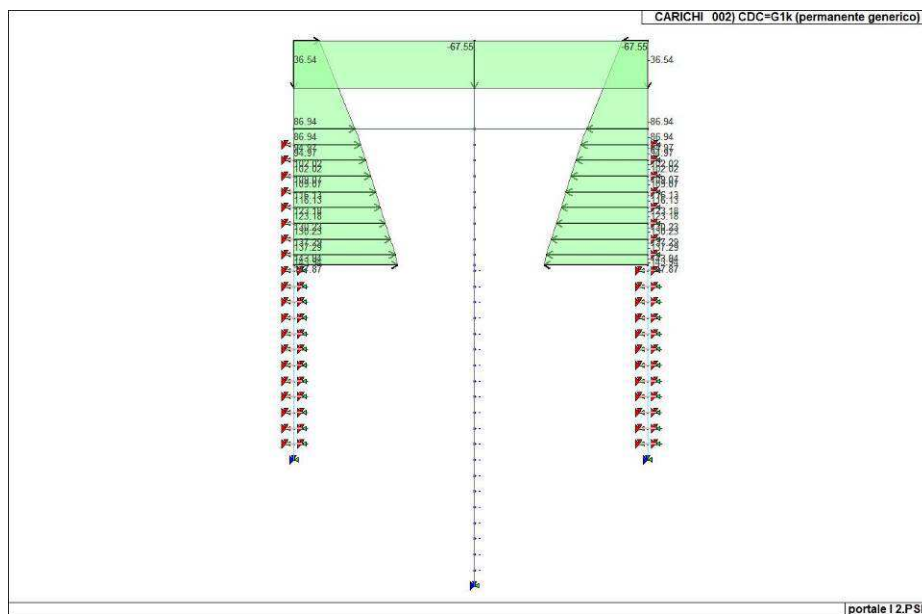
Figura 19. Caso di carico CDC 2 (permanente generico)
