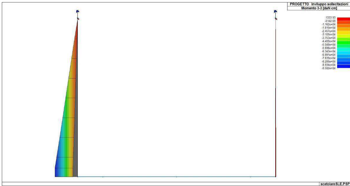
Figura 88. Involuppo del momento flettente delle fodere
