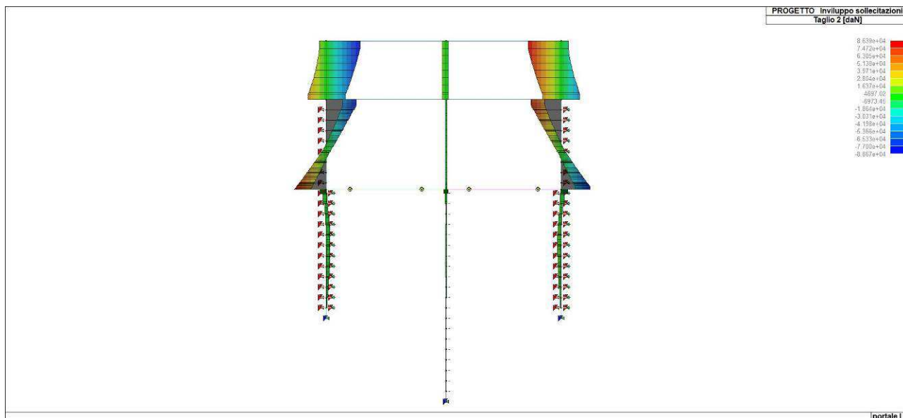
Figura 48. Involuppo del taglio di diaframmi e piedritti
