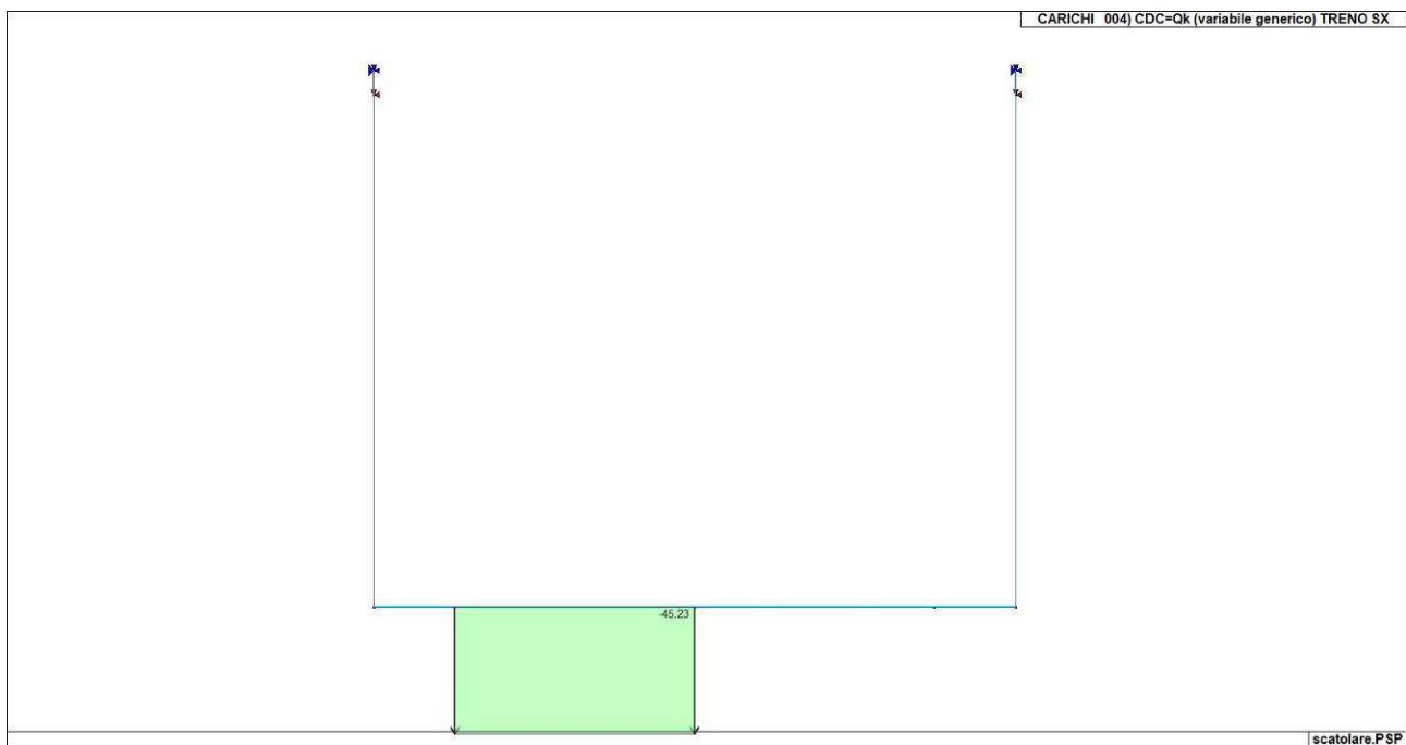
Figura 70. Caso di carico CDC 4 (Treno binario sinistra)
