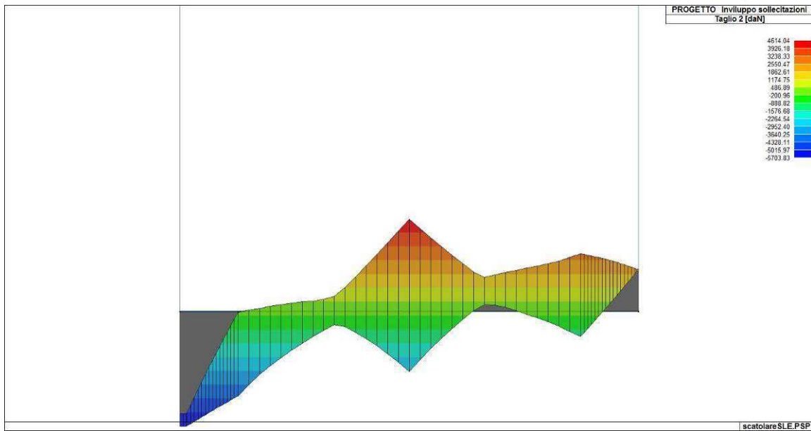
Figura 90. Involuppo del taglio del solettone di fondazione
