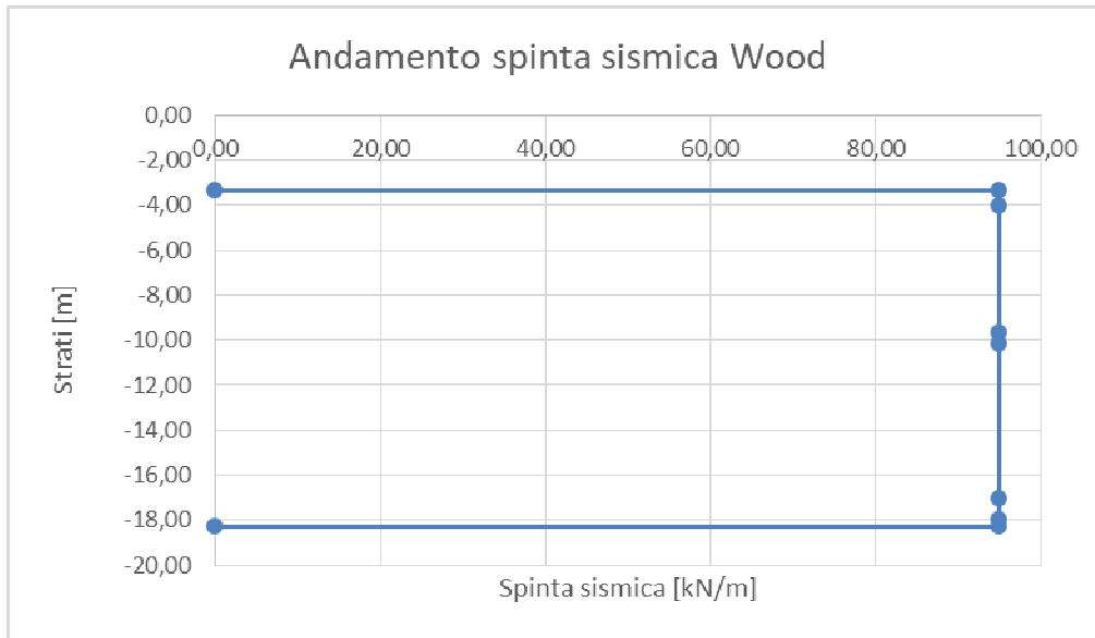
Figura 65. Diagramma andamento spinta Wood
