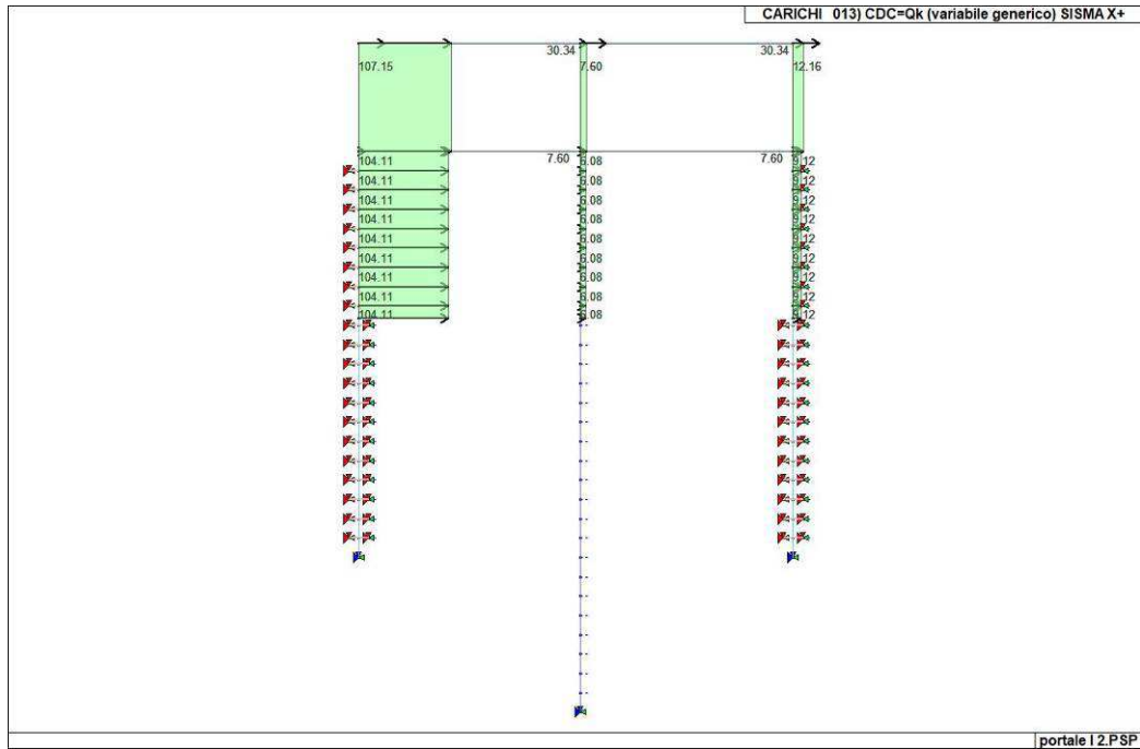
Figura 30. Caso di carico CDC 13 (Sisma X+)
