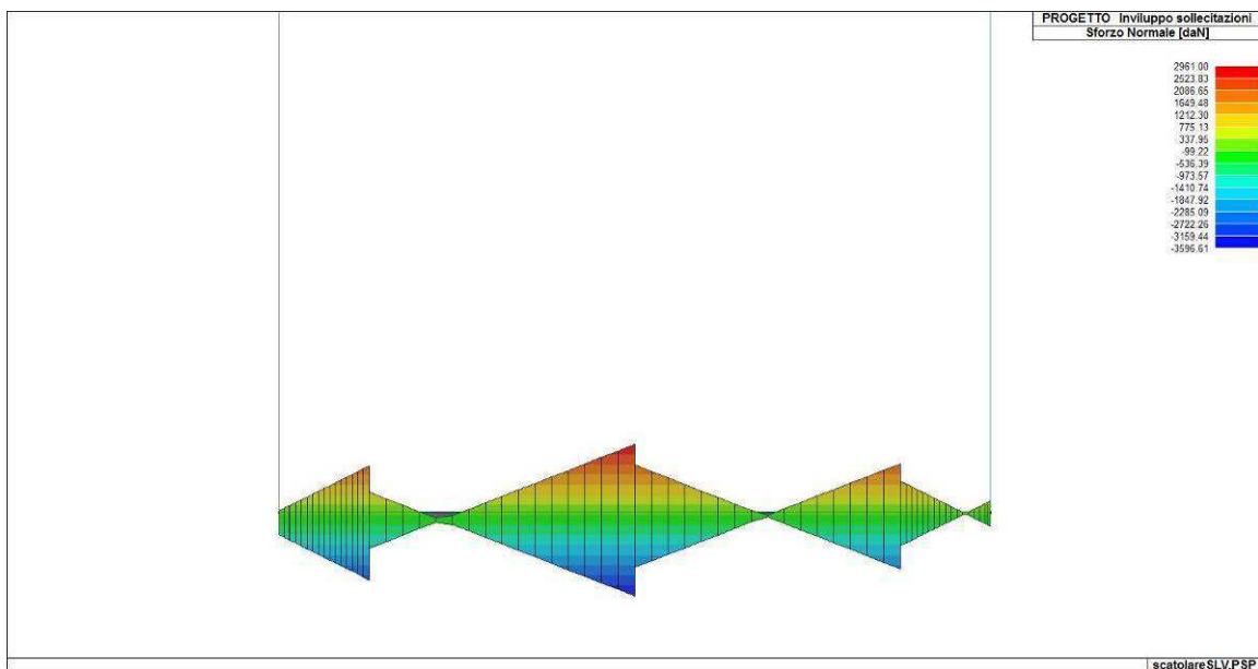
Figura 83. Involuppo dello sforzo normale del solettone di fondazione
