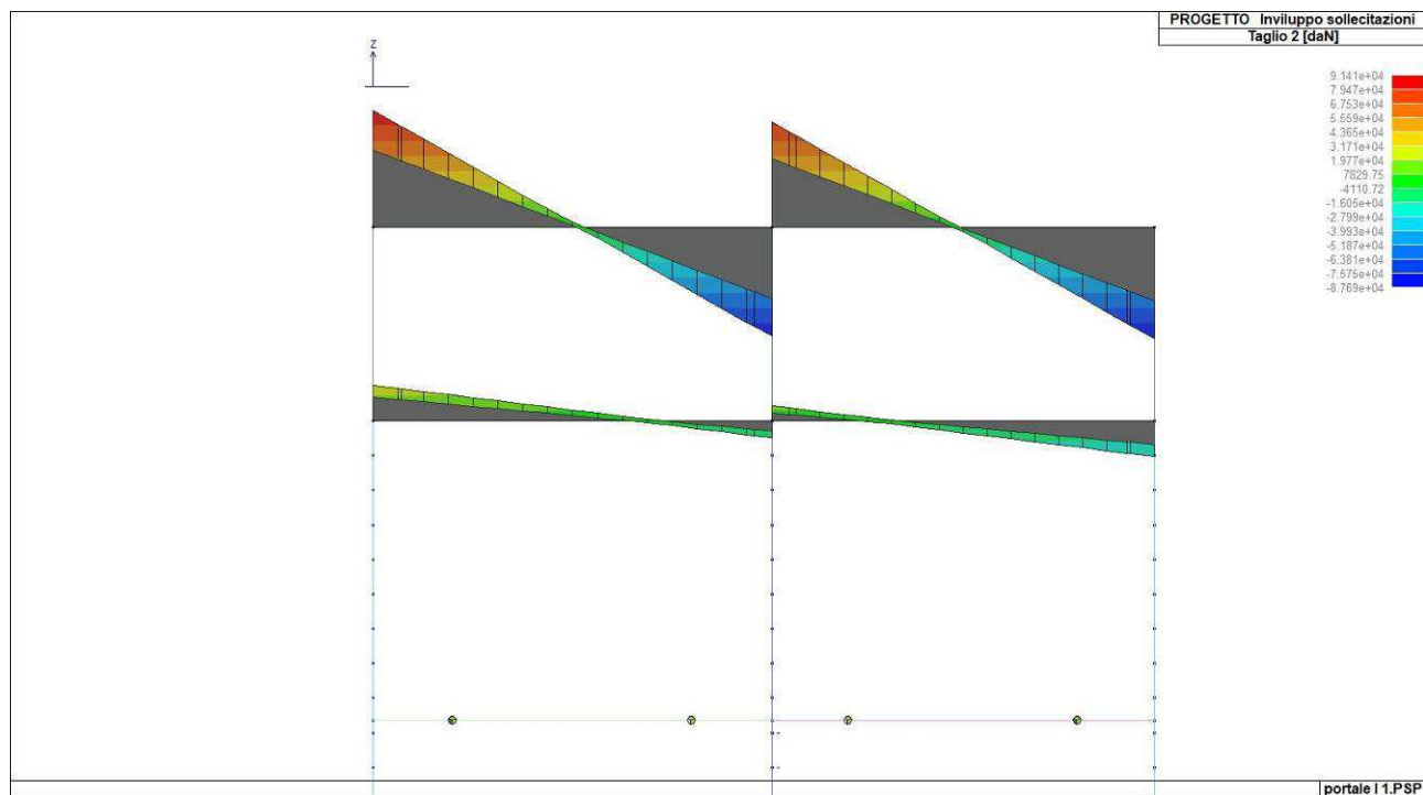
Figura 37. Involuppo del taglio del solettone di copertura
