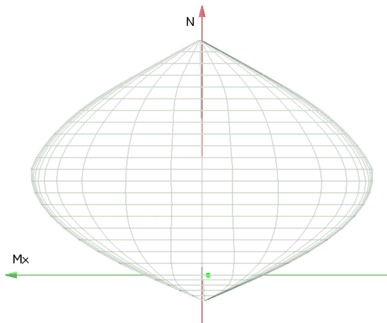
Figura 118. Dominio M-N
