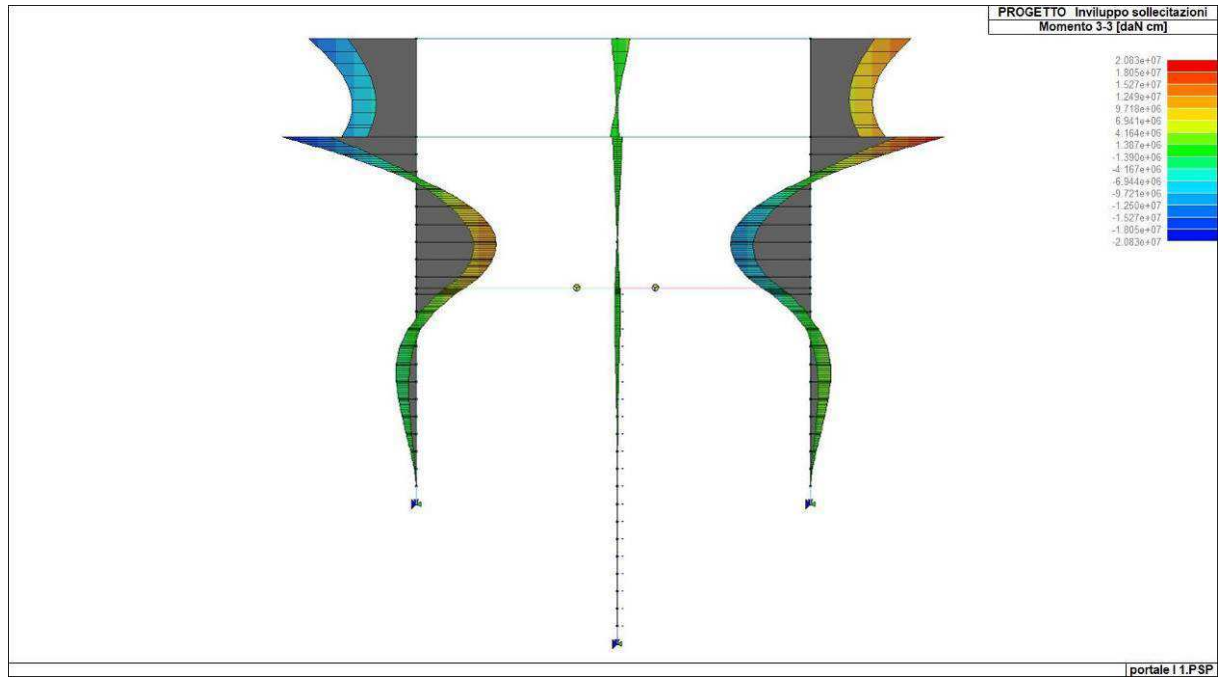
Figura 35. Involuppo del momento flettente di diaframmi e piedritti
