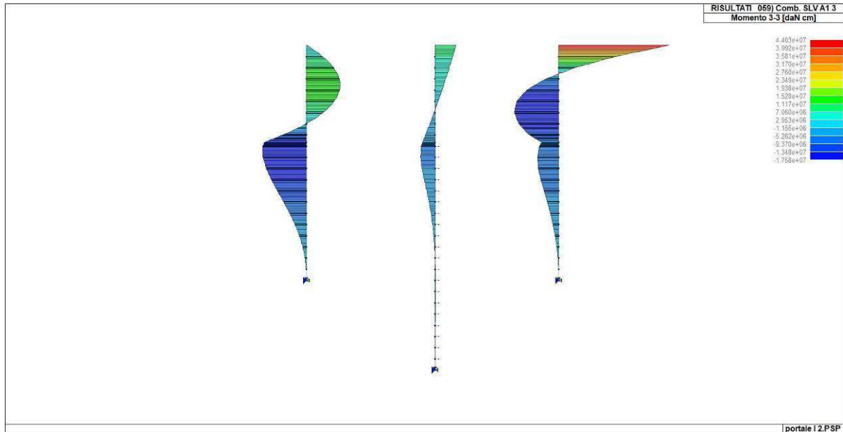
Figura 41. Momento flettente massimo diaframmi (combinazione 59)
