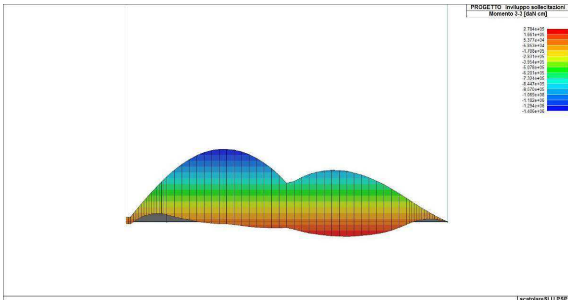
Figura 79. Involuppo del momento flettente del solettone di fondazione
