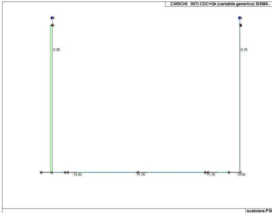
Figura 71. Caso di carico CDC 7 (Sisma X-)
