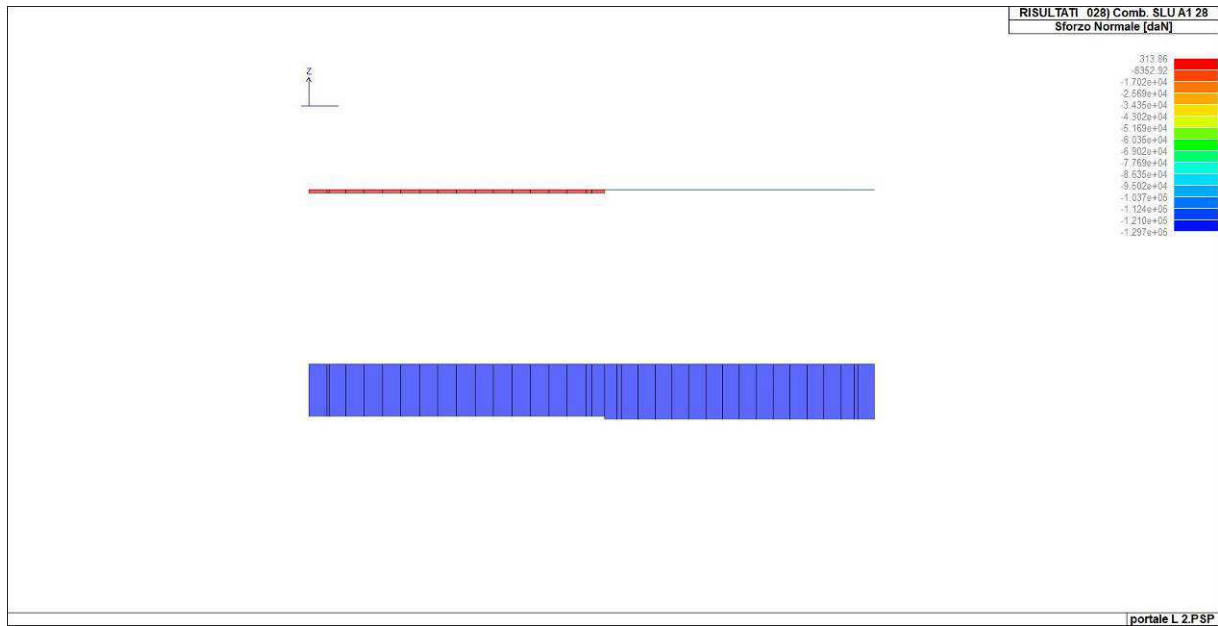
Figura 41. Sforzo normale solettone di copertura (combinazione 28)
