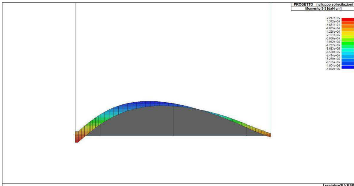
Figura 83. Involuppo del momento flettente del solettone di fondazione
