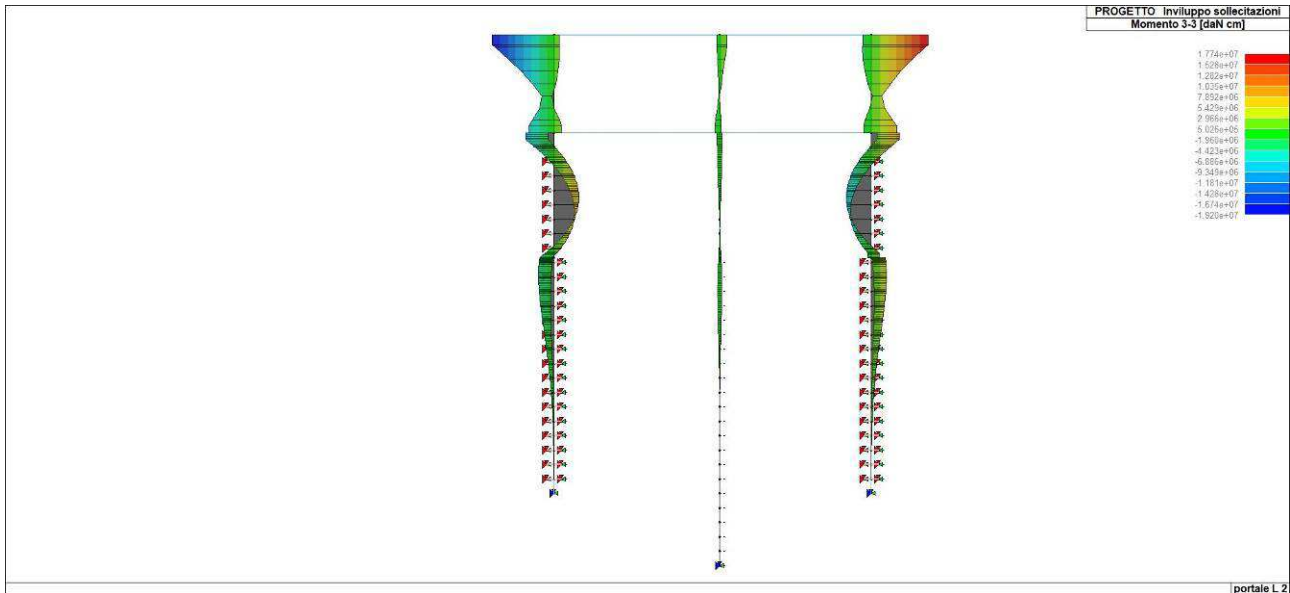
Figura 59. Involuppo del momento flettente di diaframmi e piedritti
