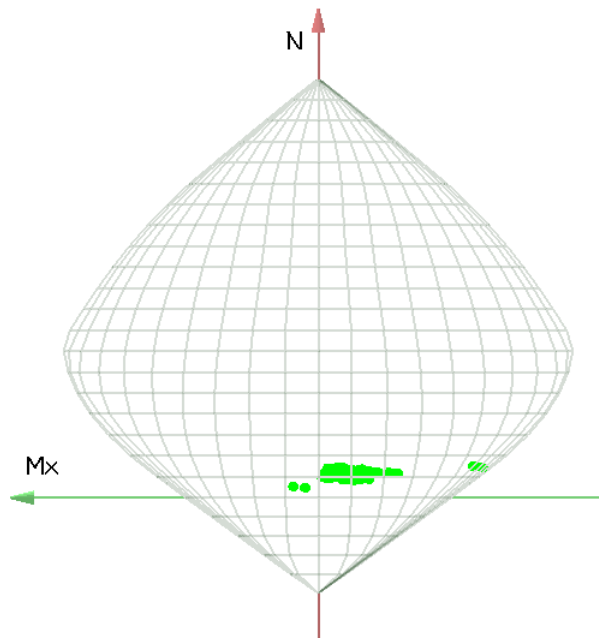
Figura 93. Dominio M-N
