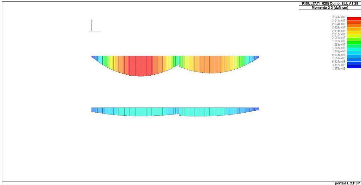
Figura 43. Momento flettente massimo solettone di copertura (combinazione 28)
