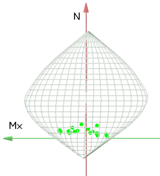
Figura 99. Dominio M-N
