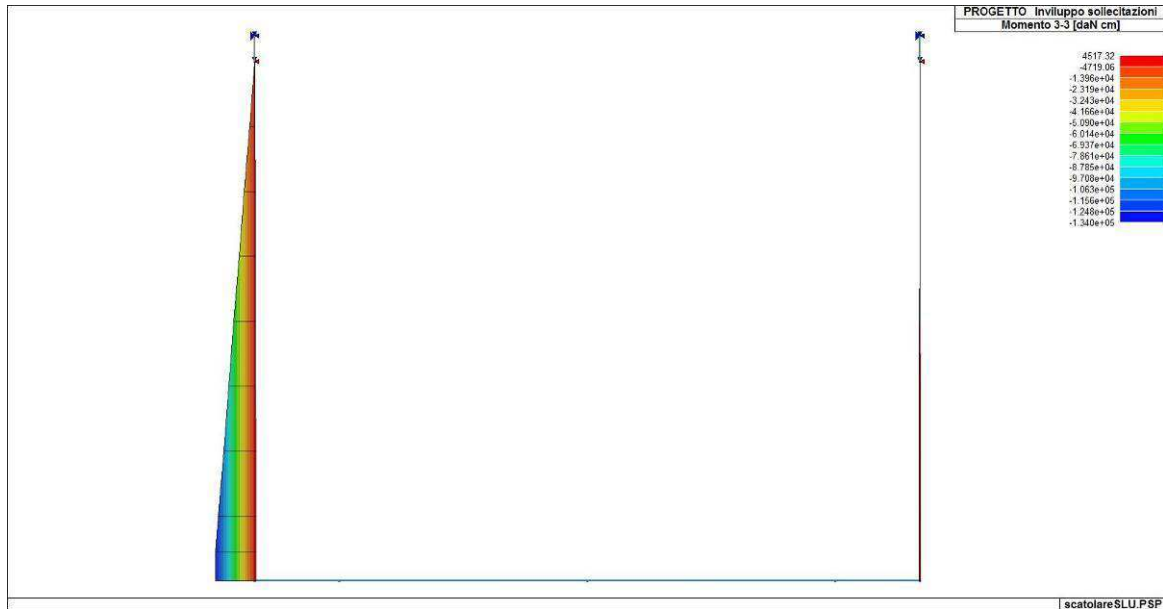
Figura 74. Involuppo del momento flettente delle fodere
