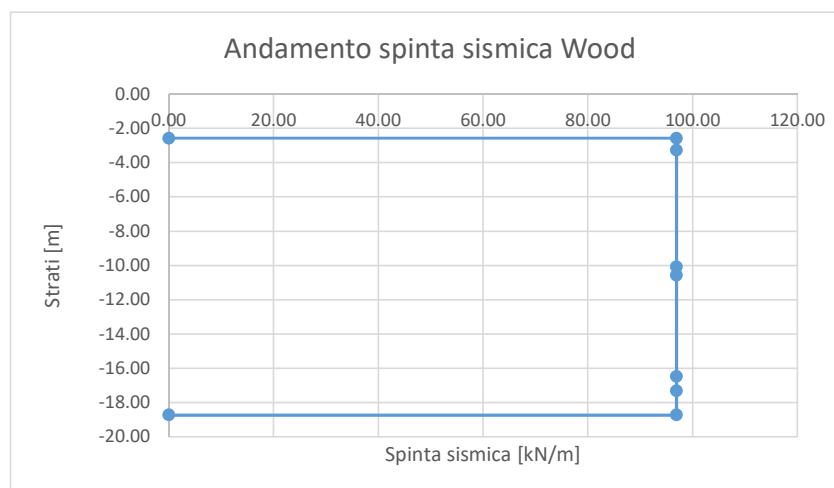
Figura 63. Diagramma andamento spinta Wood
