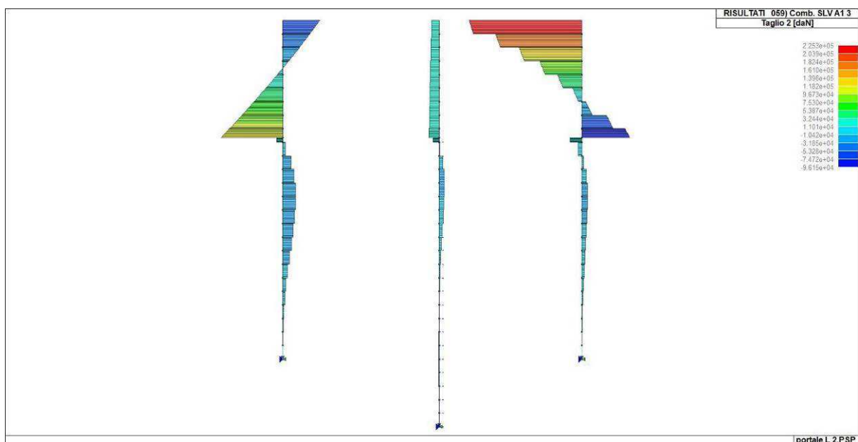
Figura 38. Taglio diaframmi (combinazione 59)
