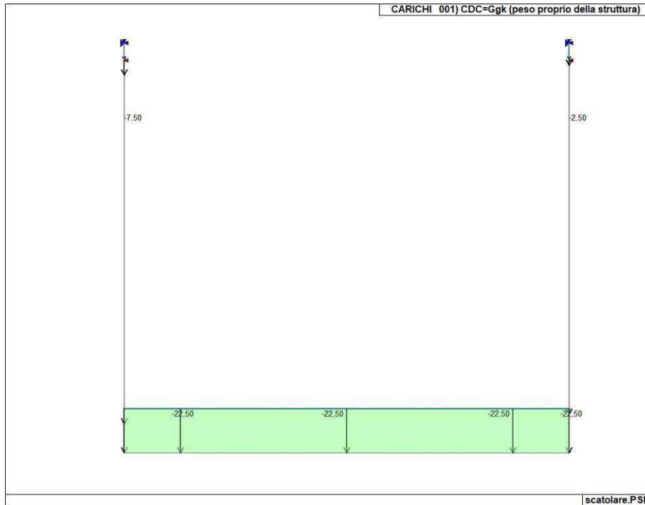
Figura 65. Caso di carico CDC 1 (Peso proprio della struttura)
