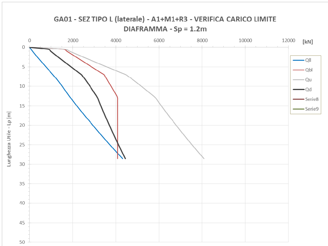
Figura 115. Curva di capacità portante diaframma laterale sezione L
