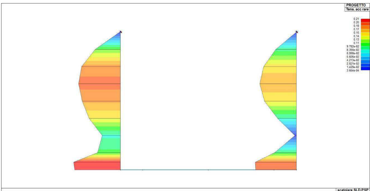
Figura 111. Indice di verifica della tensione dell'acciaio per combinazioni rare
