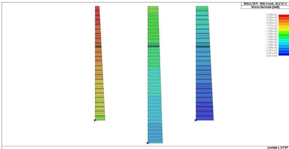
Figura 37. Storzio normale diaframmi (combinazione 59)
