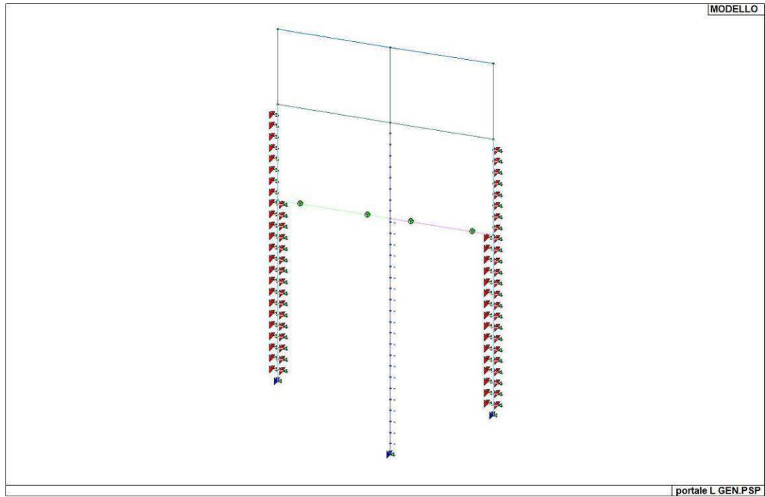
Figura 5. Vista unifilare del modello
