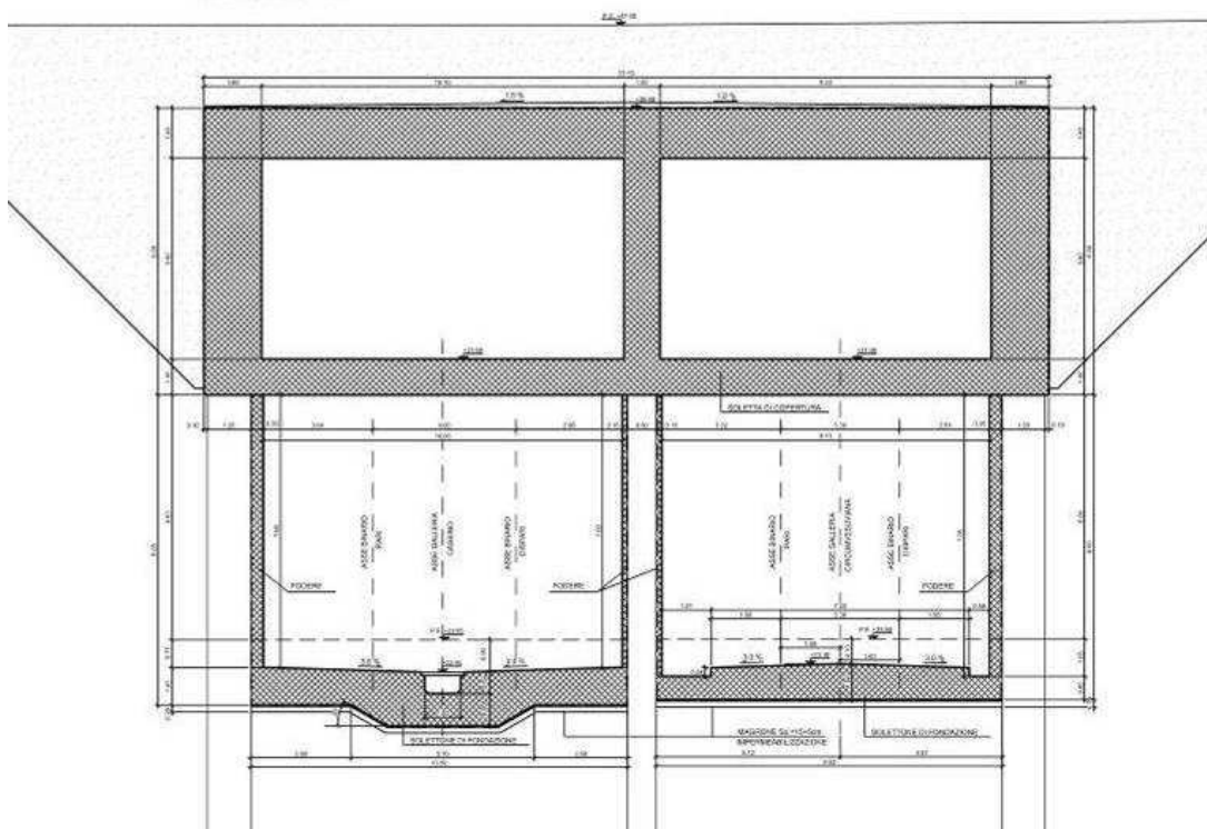
Figura 4. Sezione trasversale
