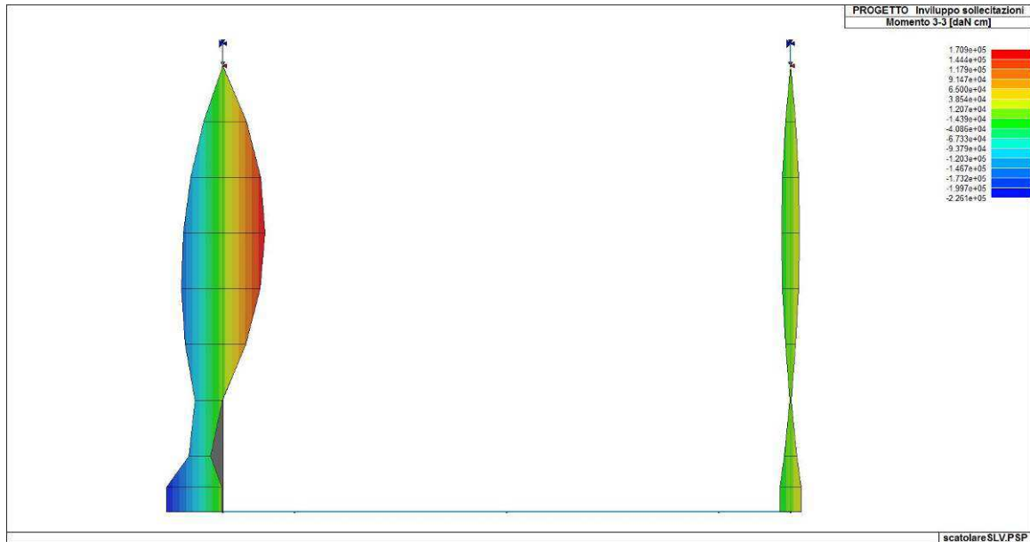
Figura 80. Involuppo del momento flettente delle fodere
