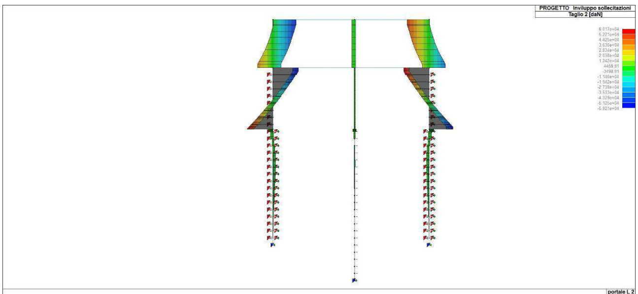
Figura 58. Inviluppo del taglio di diaframmi e piedritti
