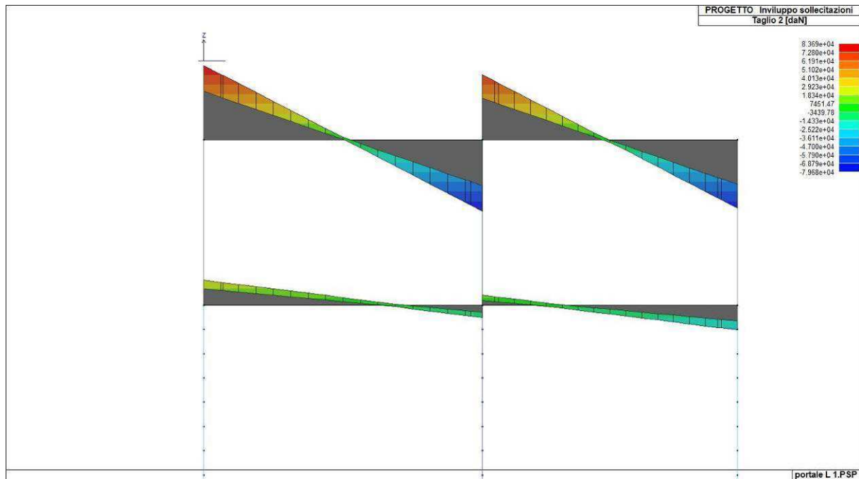
Figura 35. Involuppo del taglio del solettone di copertura
