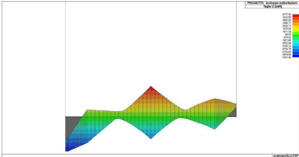
Figura 76. Involuppo del taglio del solettone di fondazione
