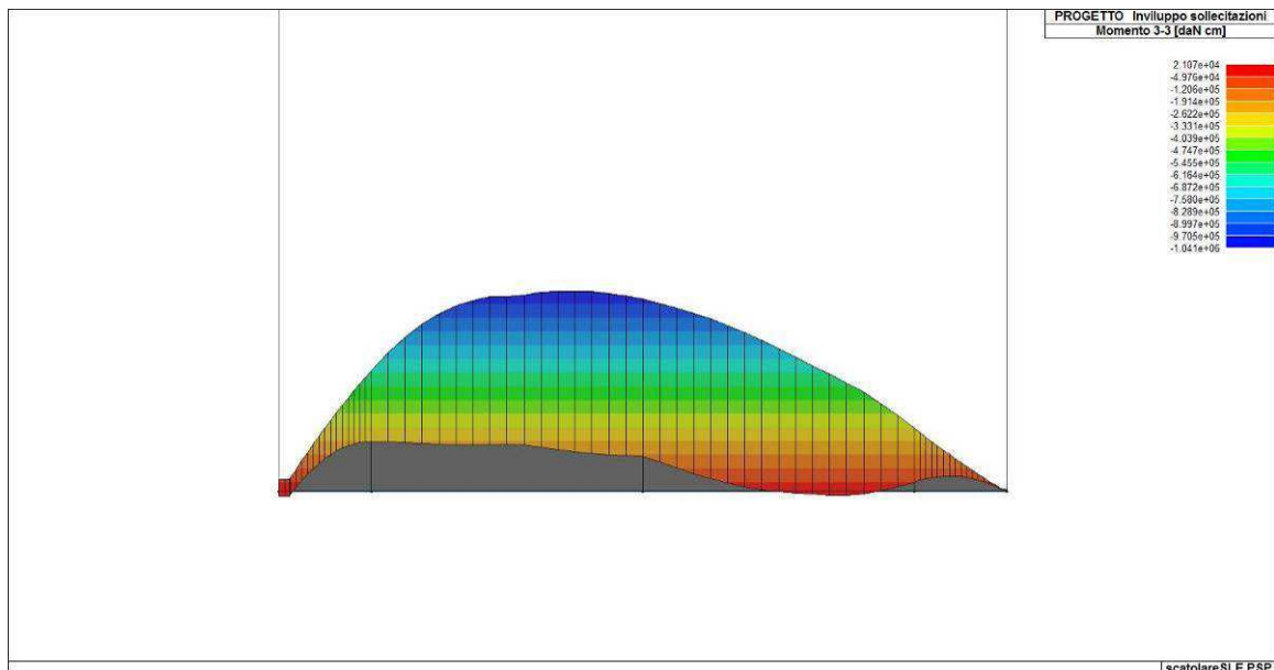
Figura 89. Inviluppo del momento flettente del solettone di fondazione
