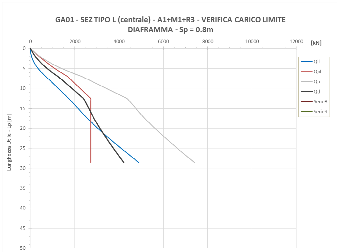
Figura 117. Curva di capacità portante diaframma centrale sezione L
