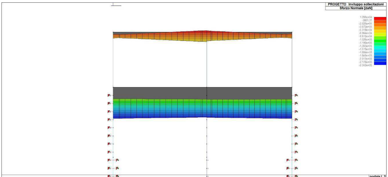
Figura 54. Involuppo dello sforzo normale del solettone di copertura
