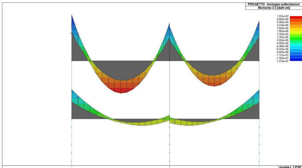
Figura 36. Involuppo del momento flettente del solettone di copertura
