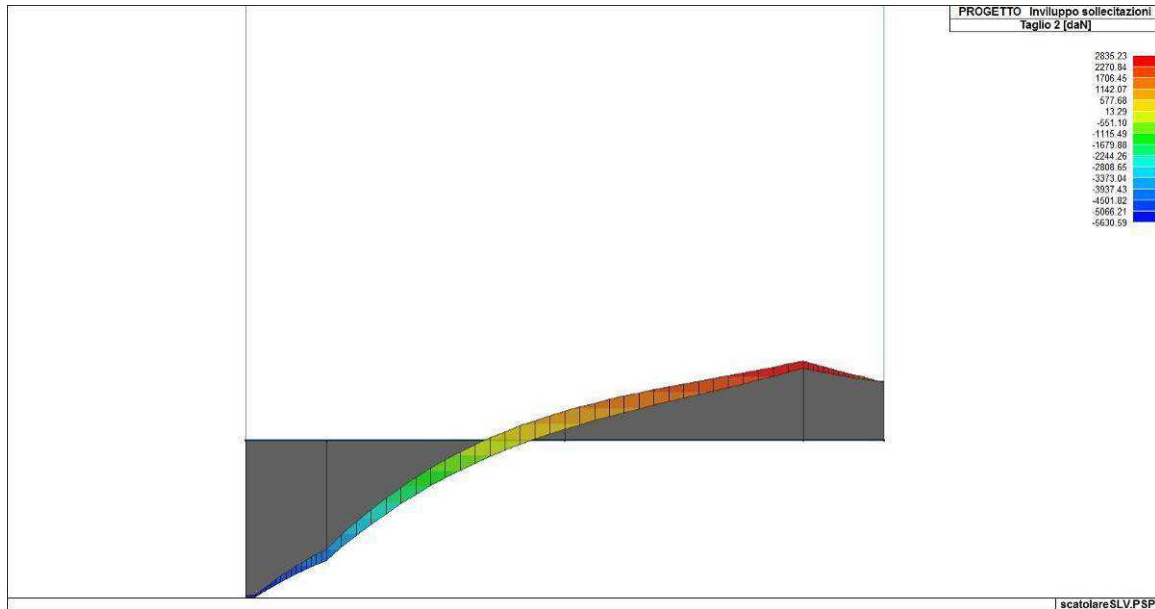
Figura 82. Involuppo del taglio del solettone di fondazione
