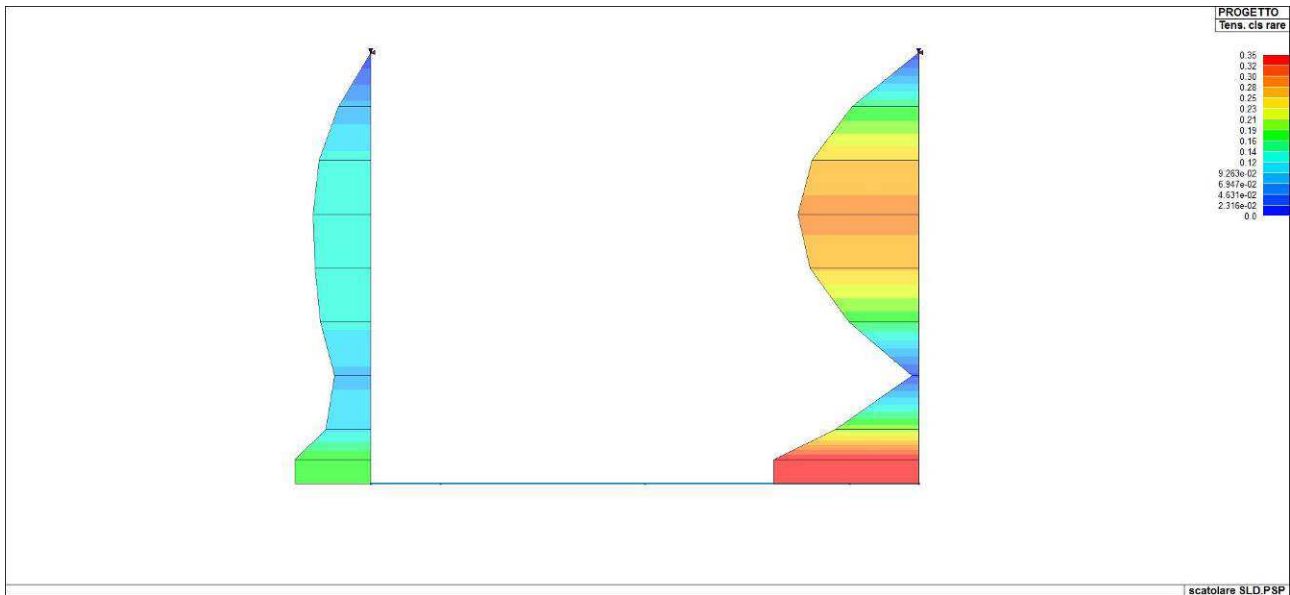
Figura 110. Indice di verifica della tensione del calcestruzzo per combinazioni rare
