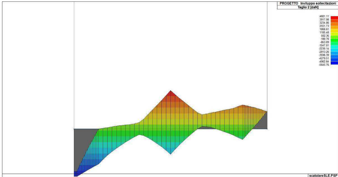
Figura 88. Inviluppo del taglio del solettone di fondazione
