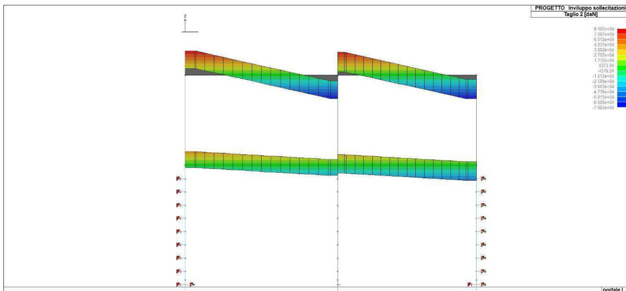
Figura 55. Inviluppo del taglio del solettone di copertura
