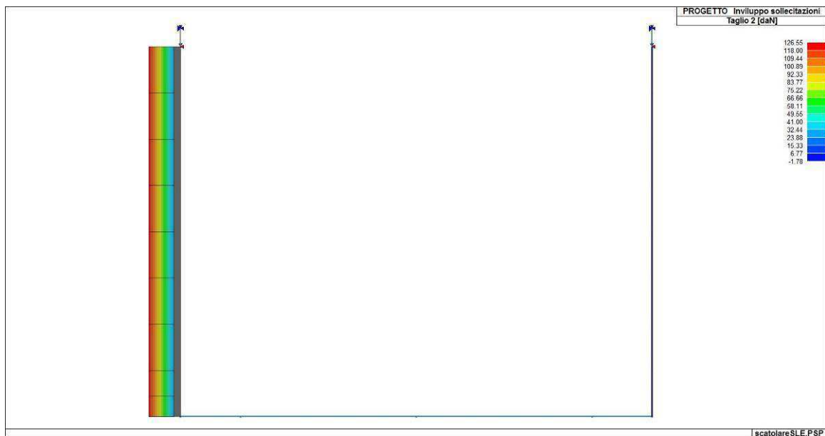
Figura 85. Involuppo del taglio delle fodere
