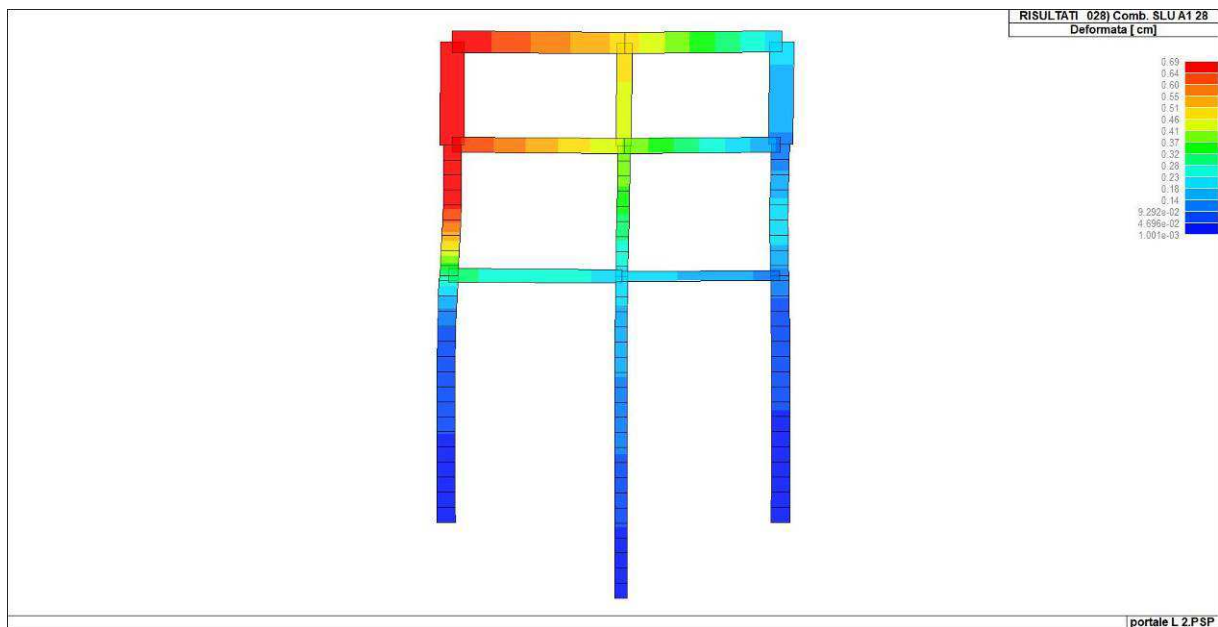
Figura 44. Deformata (combinazione 28)
