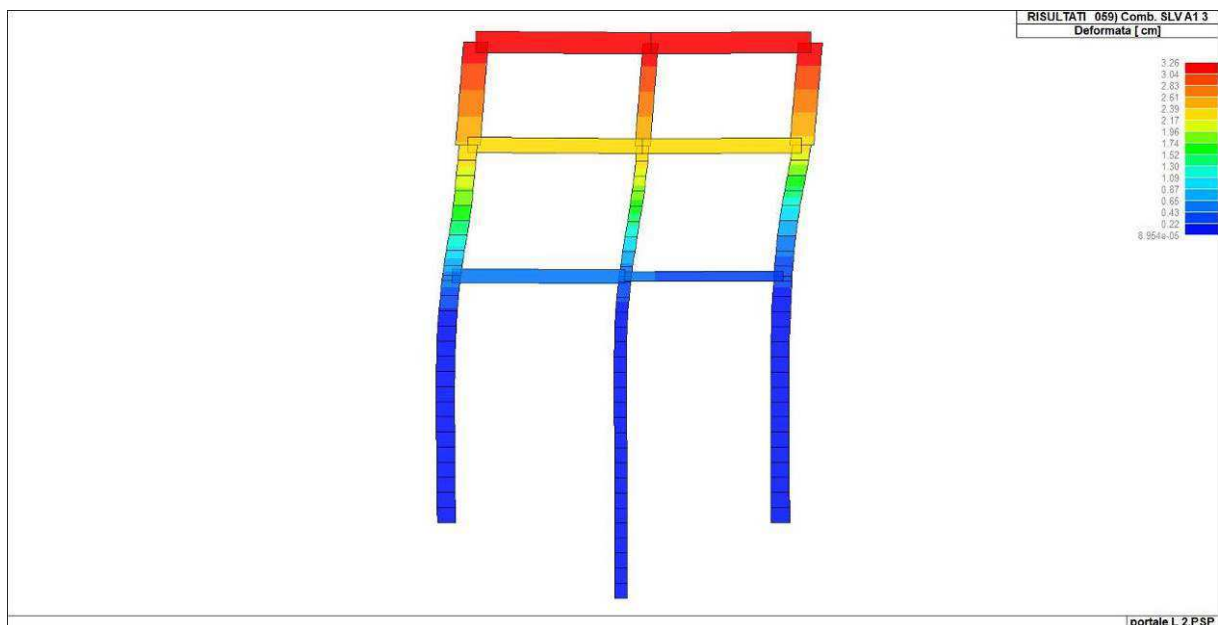
Figura 40. Deformata (combinazione 59)
