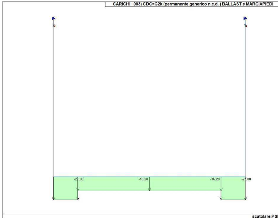
Figura 67. Caso di carico CDC 3 (Permanente ballast e marciapiedi)
