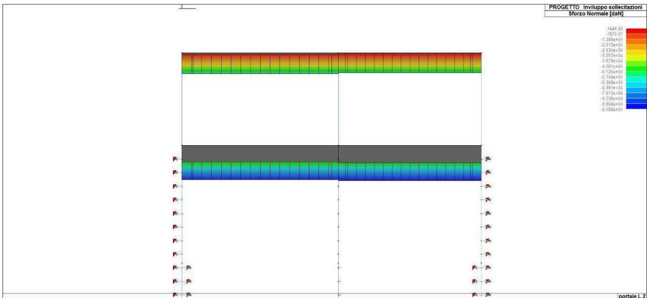
Figura 60. Involuppo dello sforzo normale del solettone di copertura
