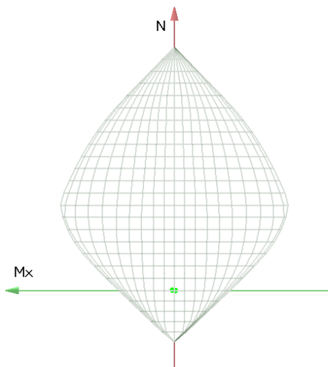
Figura 103. Dominio M-N
