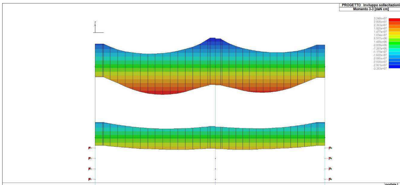
Figura 50. Involuppo del momento flettente del solettone di copertura
