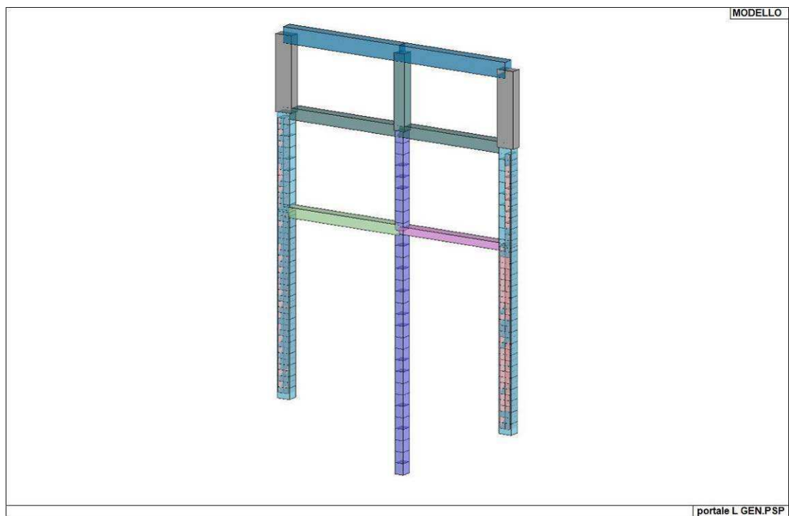
Figura 6. Vista solida del modello
