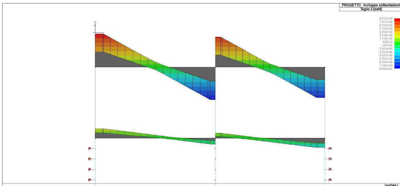
Figura 49. Involuppo del taglio del solettone di copertura
