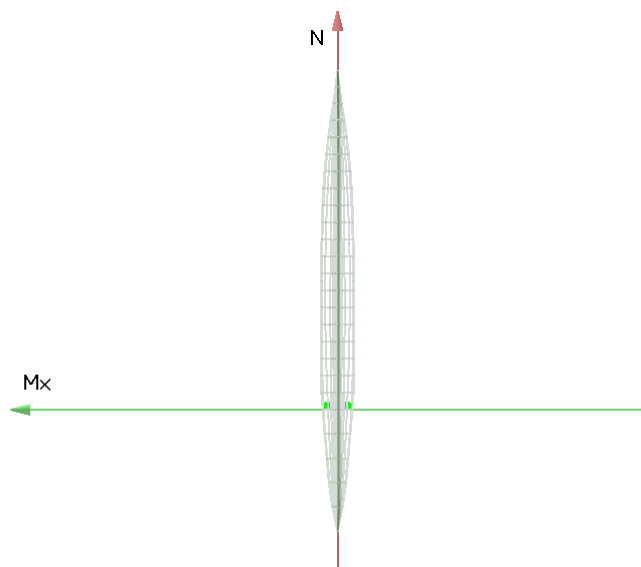
Figura 105. Dominio M-N
