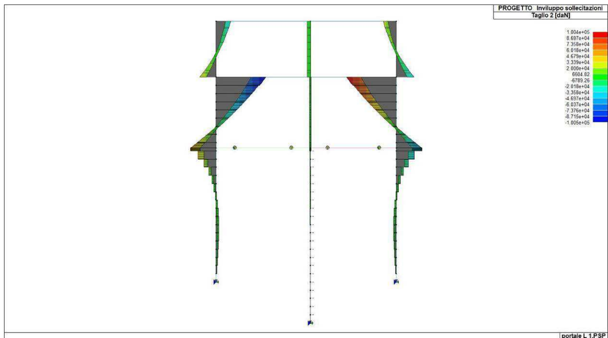
Figura 32. Inviluppo del taglio di diaframmi e piedritti
