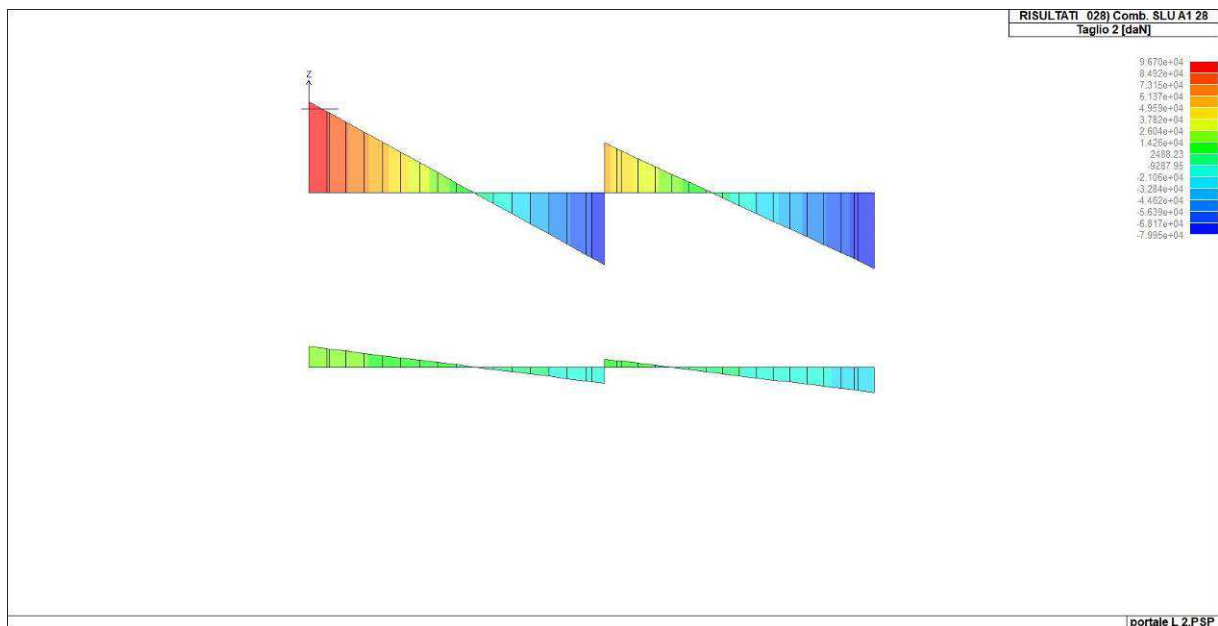
Figura 42. Taglio solettone di copertura (combinazione 28)
