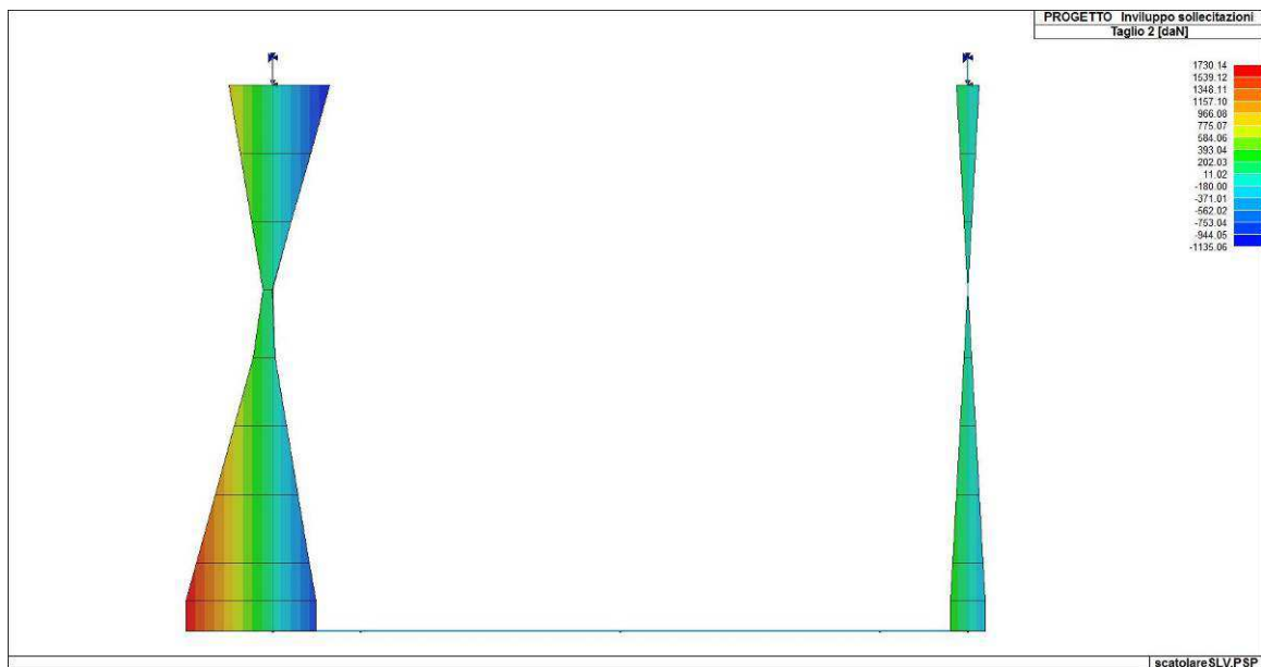
Figura 79. Inviluppo del taglio delle fodere
