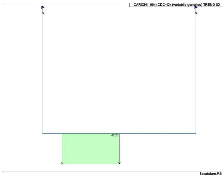
Figura 68. Caso di carico CDC 4 (Treno binario sinistra)
