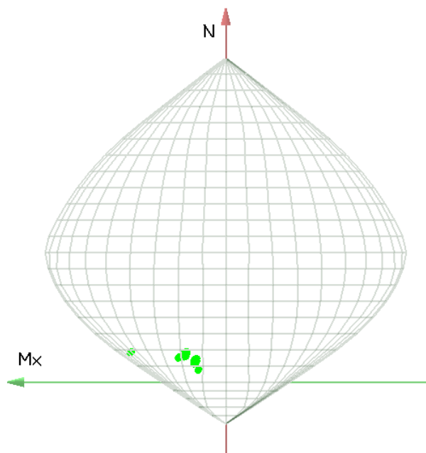
Figura 92. Dominio M-N
