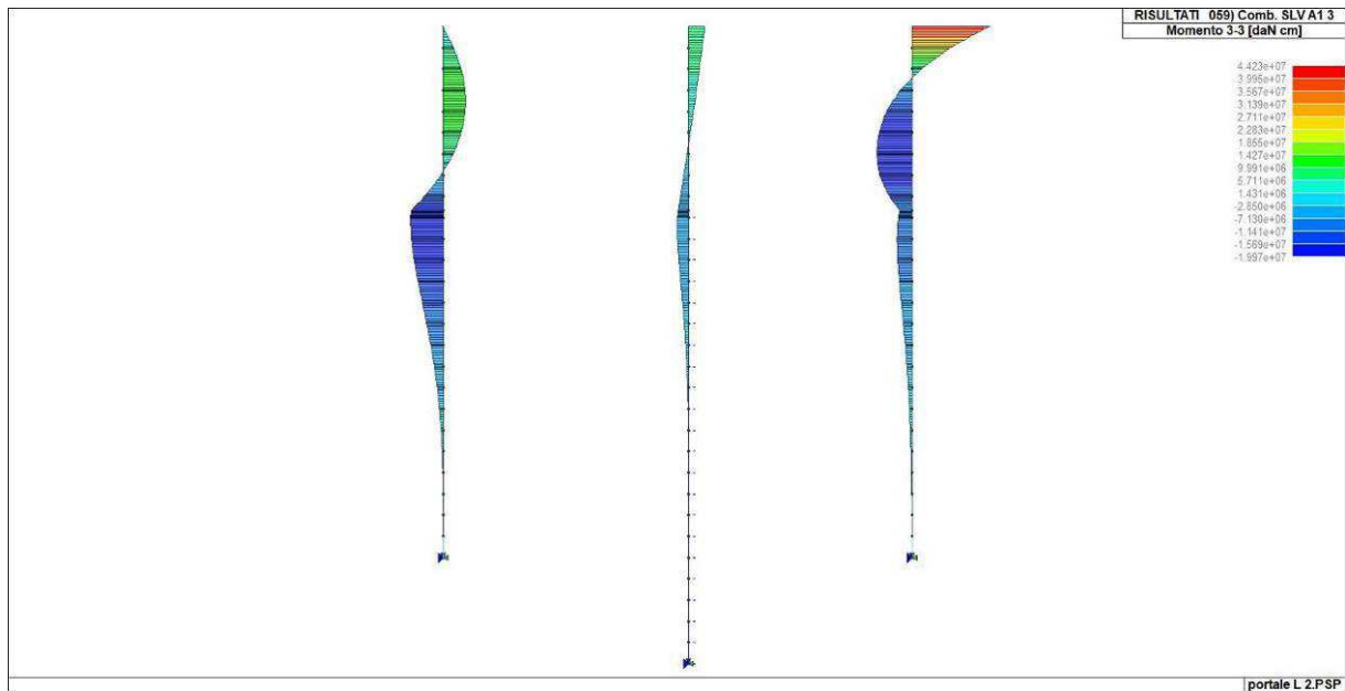
Figura 39. Momento flettente massimo diaframmi (combinazione 59)
