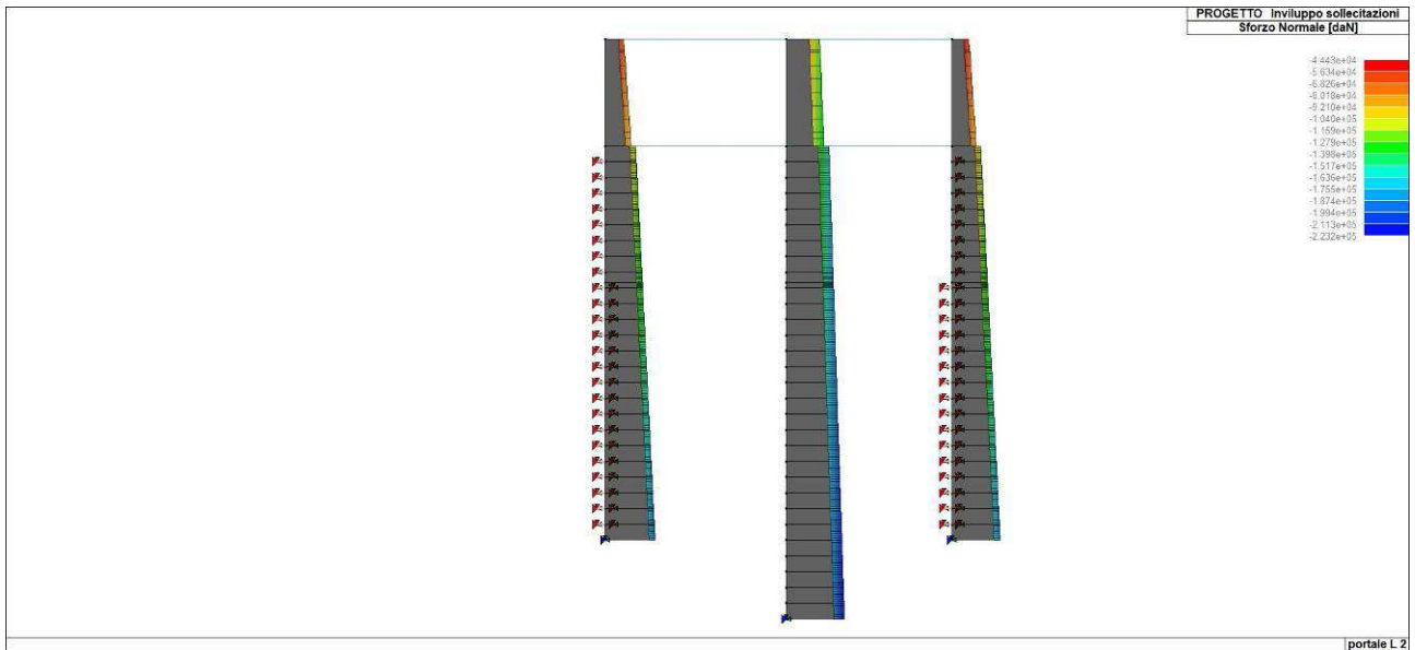
Figura 57. Inviluppo dello sforzo normale di diaframmi e piedritti
