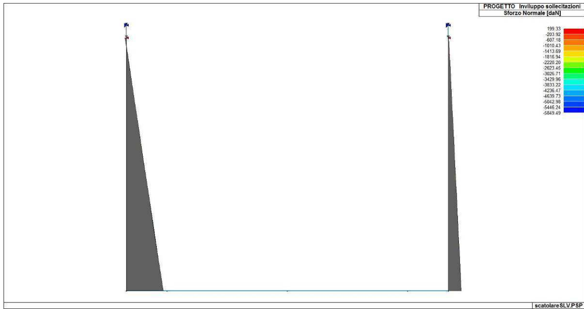
Figura 78. Inviluppo dello sforzo normale delle fodere
