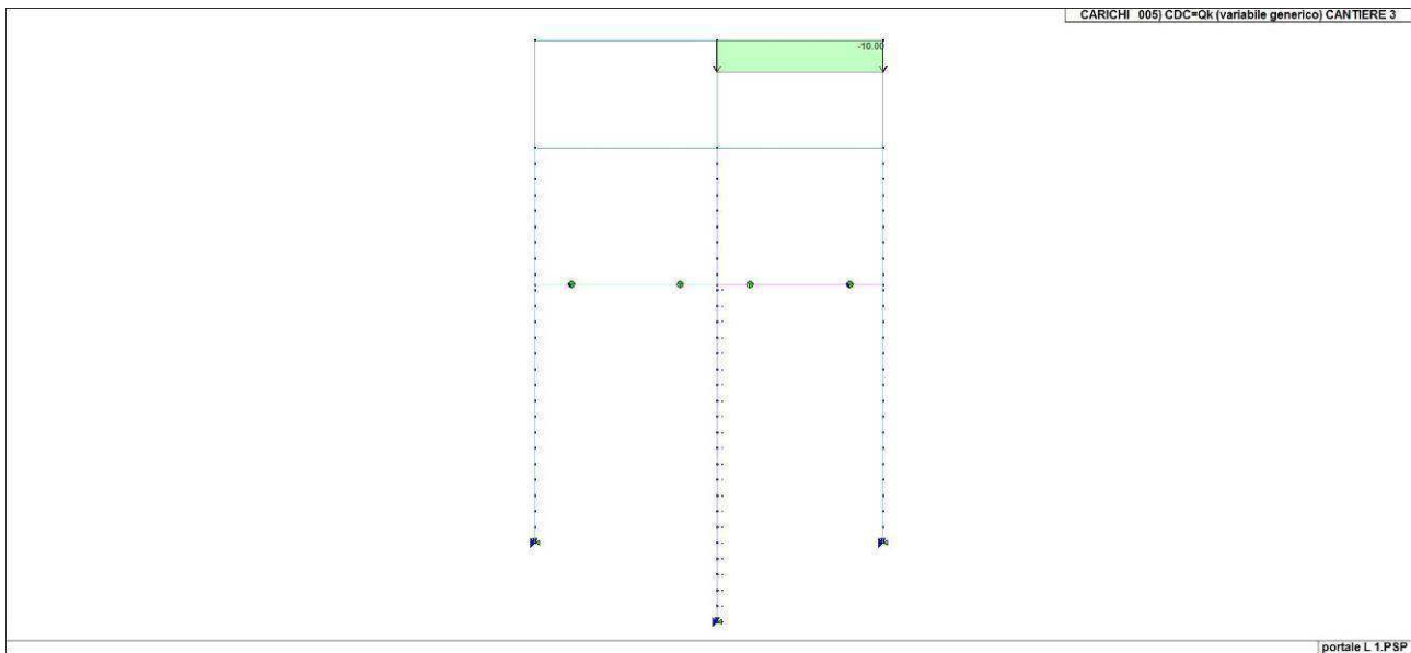
Figura 20. Caso di carico CDC 5 (Cantiere 3)
