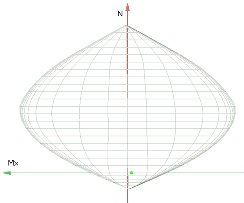
Figura 122. Dominio M-N
