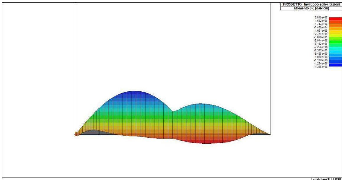
Figura 77. Involuppo del momento flettente del solettone di fondazione
