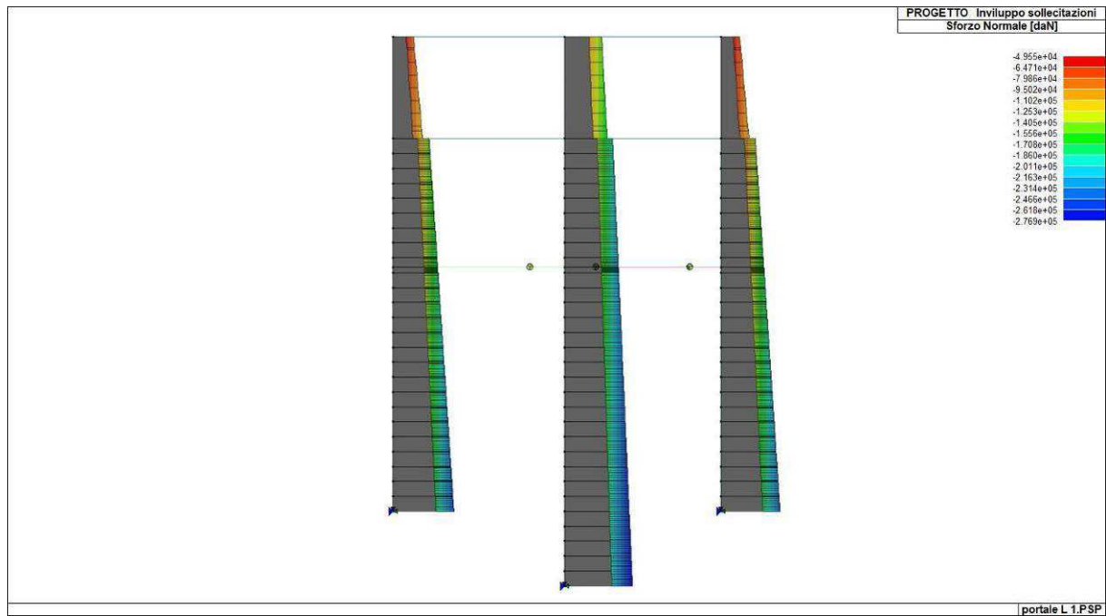
Figura 31. Inviluppo dello sforzo normale di diaframmi e piedritti
