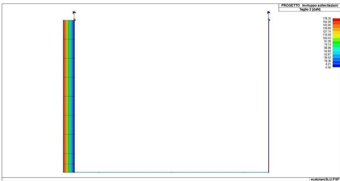
Figura 73. Involuppo del taglio delle fodere
