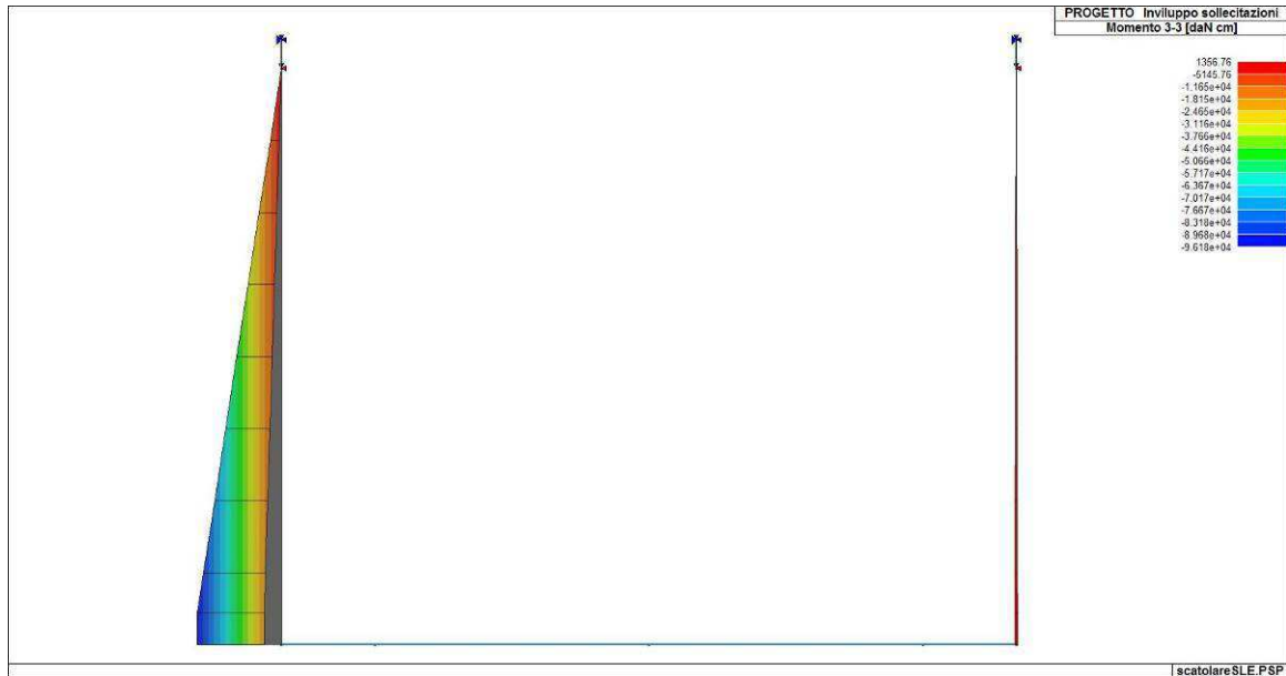
Figura 86. Involuppo del momento flettente delle fodere
