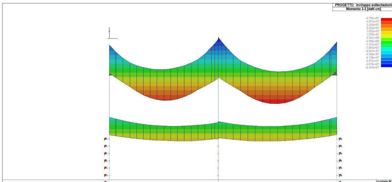
Figura 51. Involuppo del momento flettente del solettone di copertura
