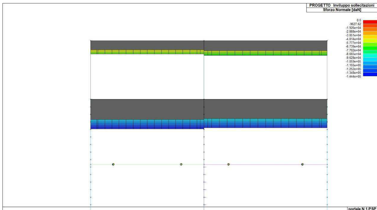
Figura 35. Involuppo dello sforzo normale del solettone di copertura
