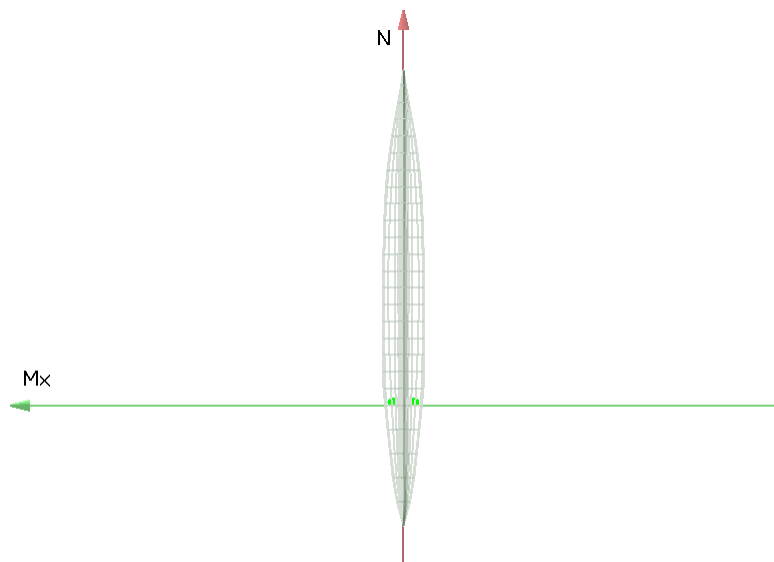
Figura 108. Dominio M-N
