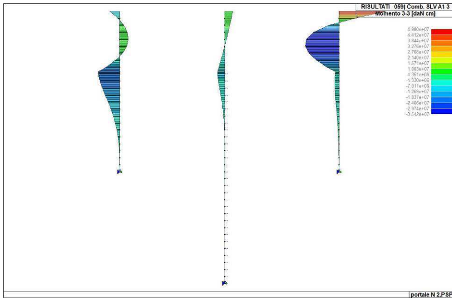
Figura 40. Momento flettente massimo diaframmi (combinazione 59)
