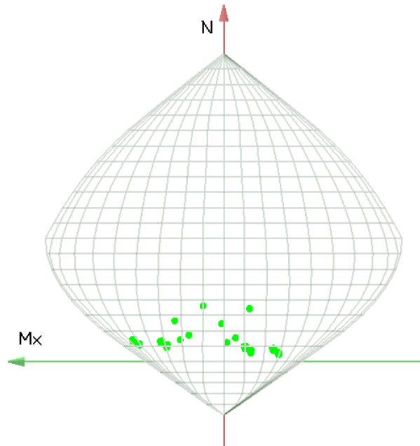
Figura 102. Dominio M-N
