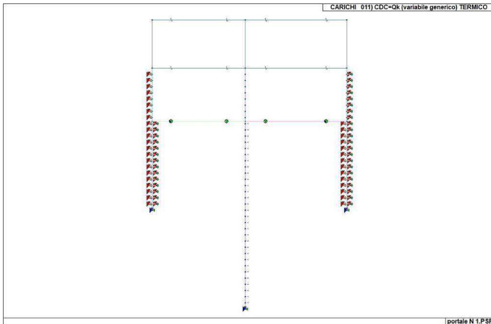
Figura 27. Caso di carico CDC 11 (Termico)
