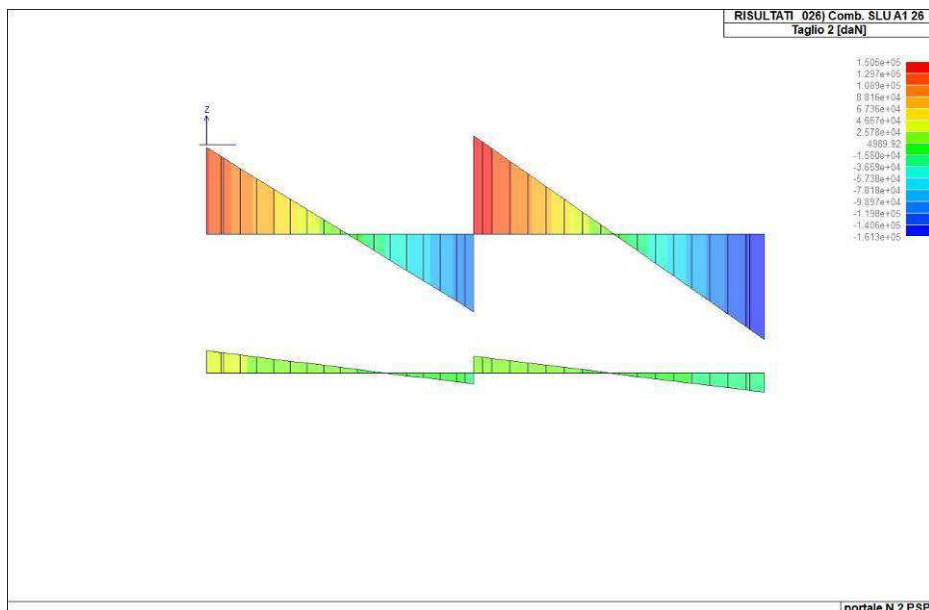
Figura 43. Taglio solettone di copertura (combinazione 26)
