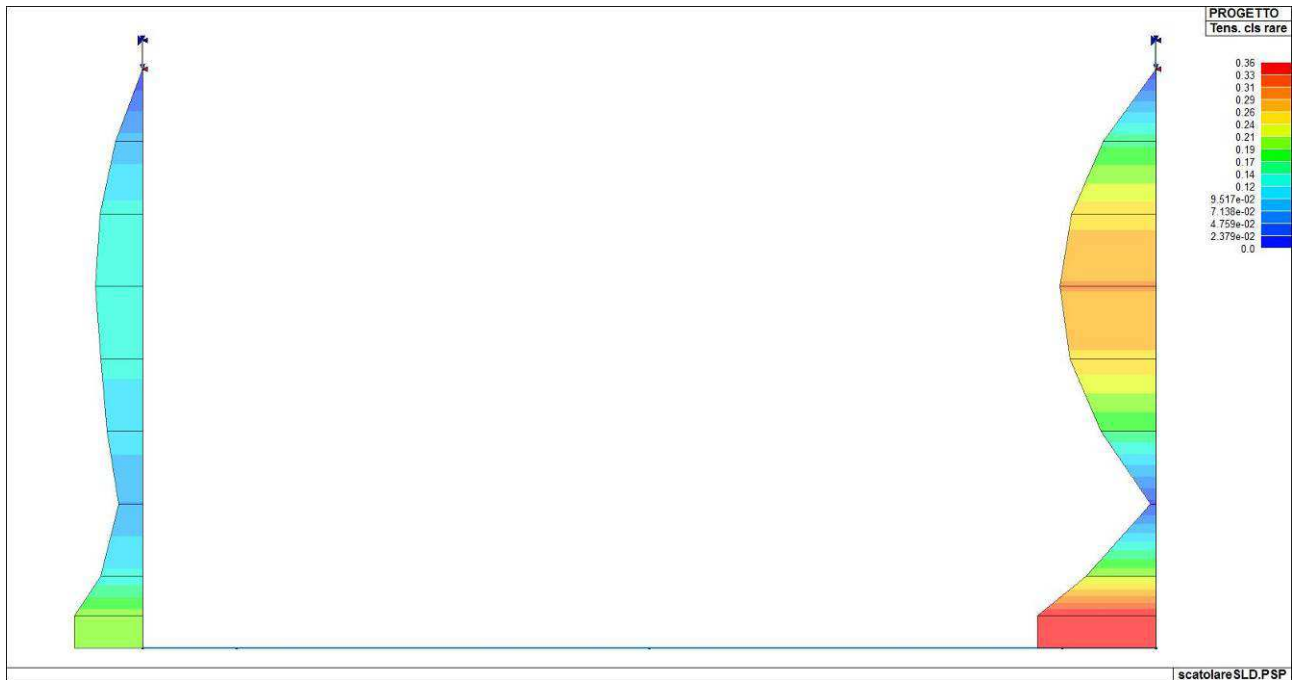
Figura 113. Indice di verifica della tensione del calcestruzzo per combinazioni rare
