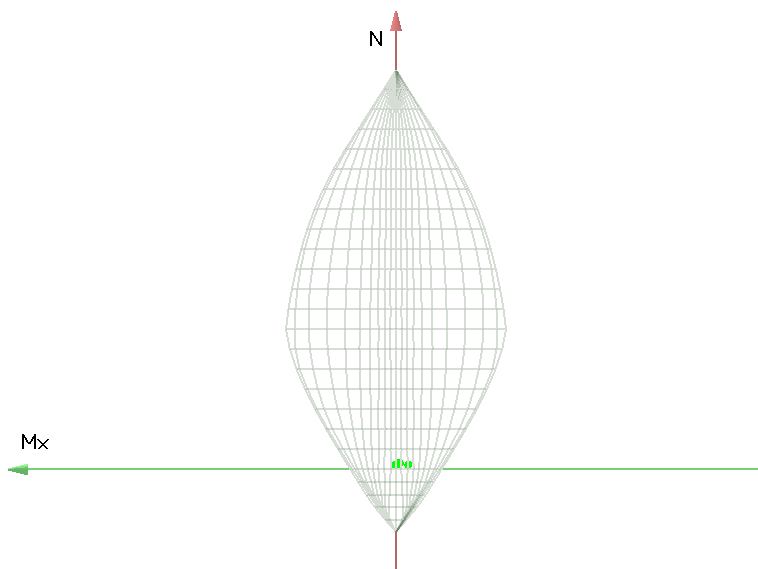
Figura 107. Dominio M-N
