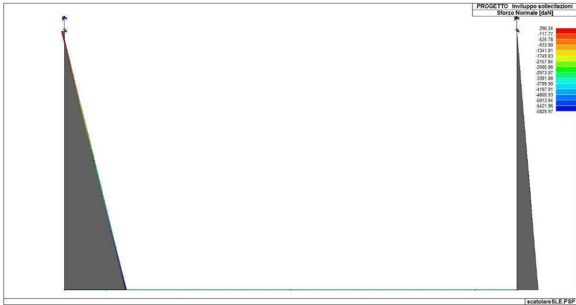
Figura 85. Involuppo dello sforzo normale delle fodere
