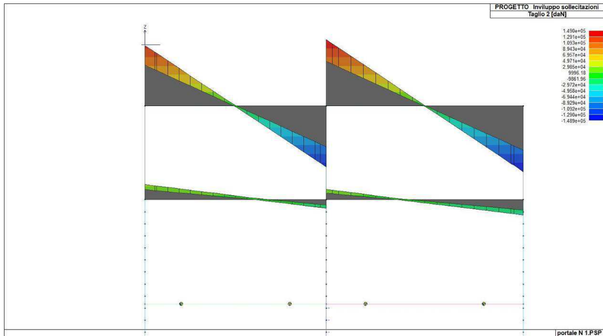
Figura 36. Involuppo del taglio del solettone di copertura
