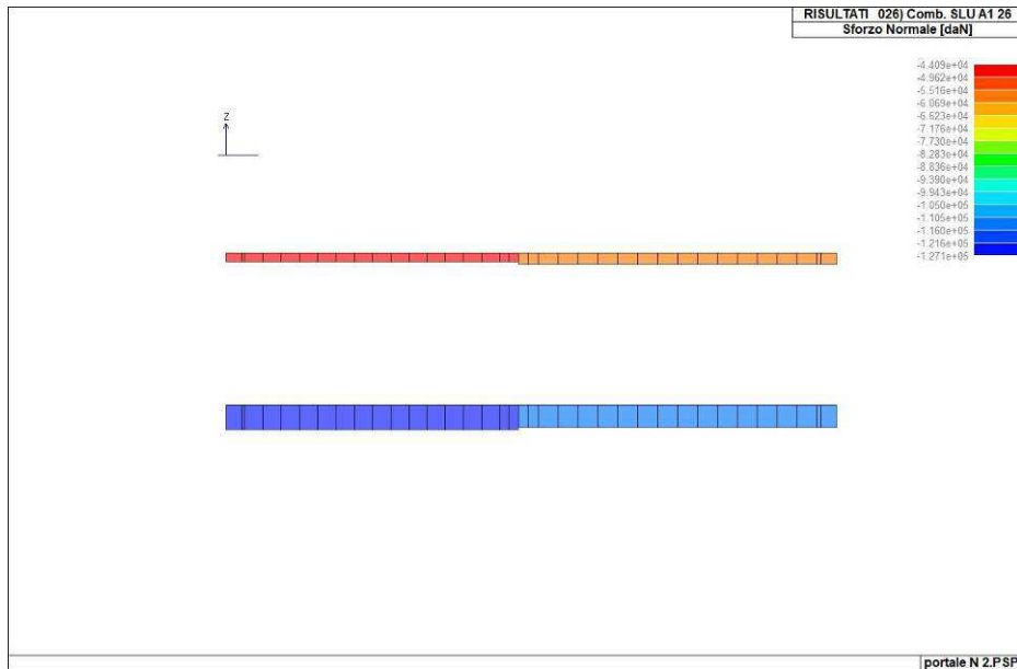
Figura 42. Sforzo normale solettone di copertura (combinazione 26)
