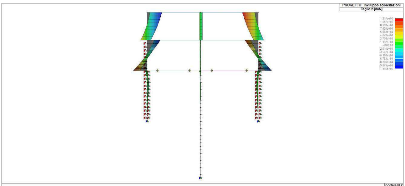
Figura 47. Inviluppo del taglio di diaframmi e piedritti
