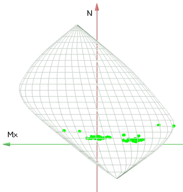
Figura 103. Dominio M-N
