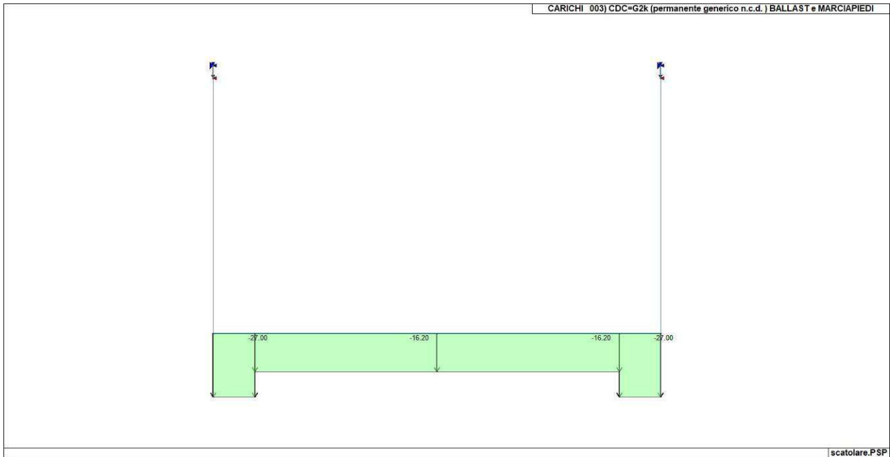
Figura 68. Caso di carico CDC 3 (Permanente ballast e marciapiedi)
