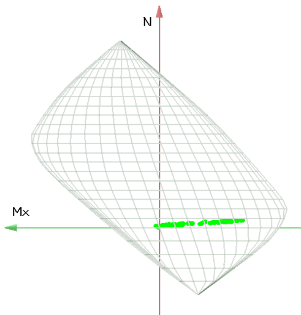
Figura 101. Dominio M-N
