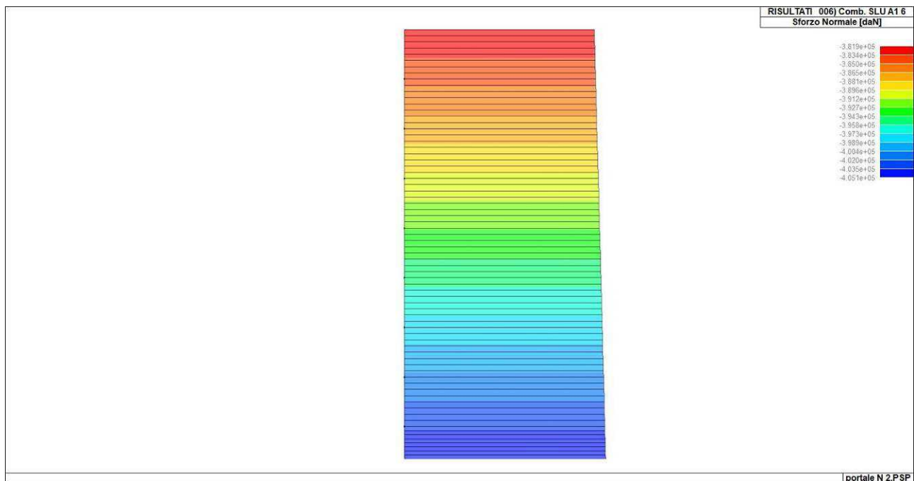
Figura 119. Sforzo normale massimo sul diaframma centrale
