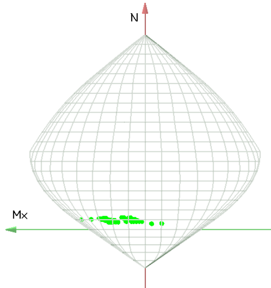
Figura 96. Dominio M-N
