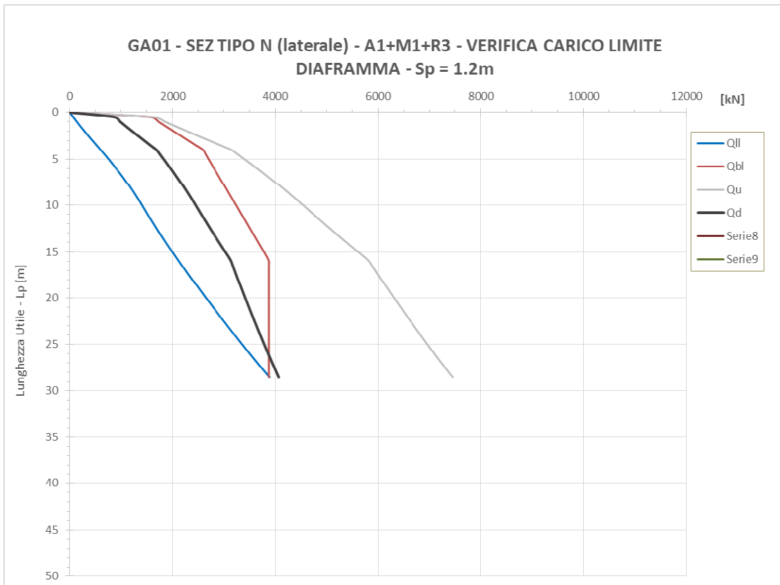
Figura 118. Curva di capacità portante diaframma laterale sezione N
