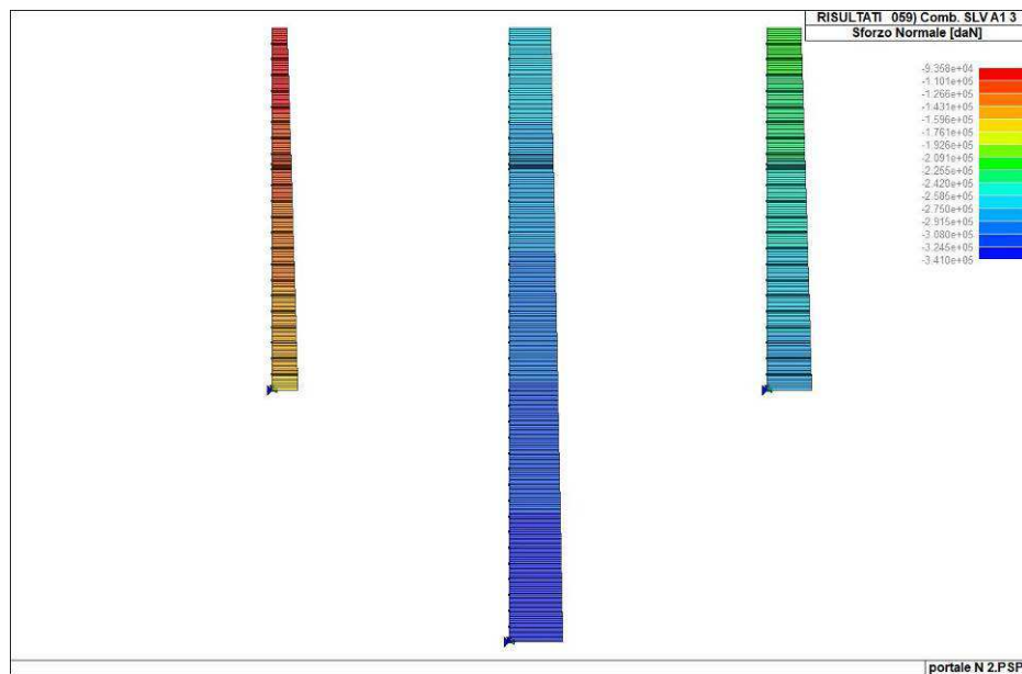
Figura 38. Sforzo normale diaframmi (combinazione 59)
