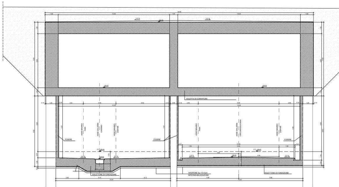
Figura 5. Sezione trasversale
