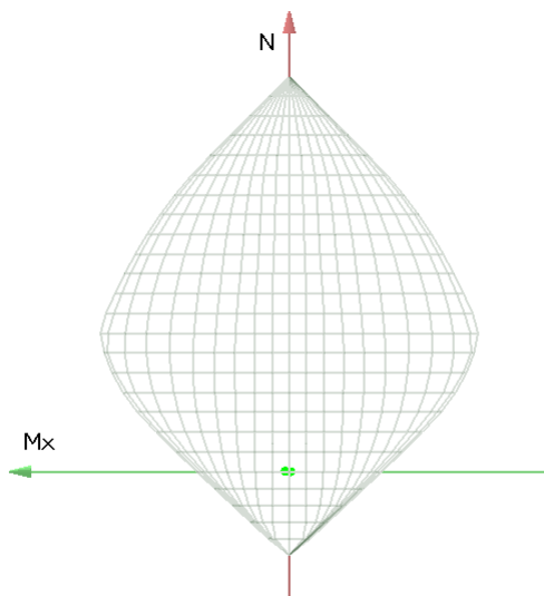
Figura 106. Dominio M-N
