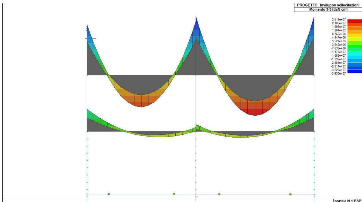
Figura 37. Involuppo del momento flettente del solettone di copertura
