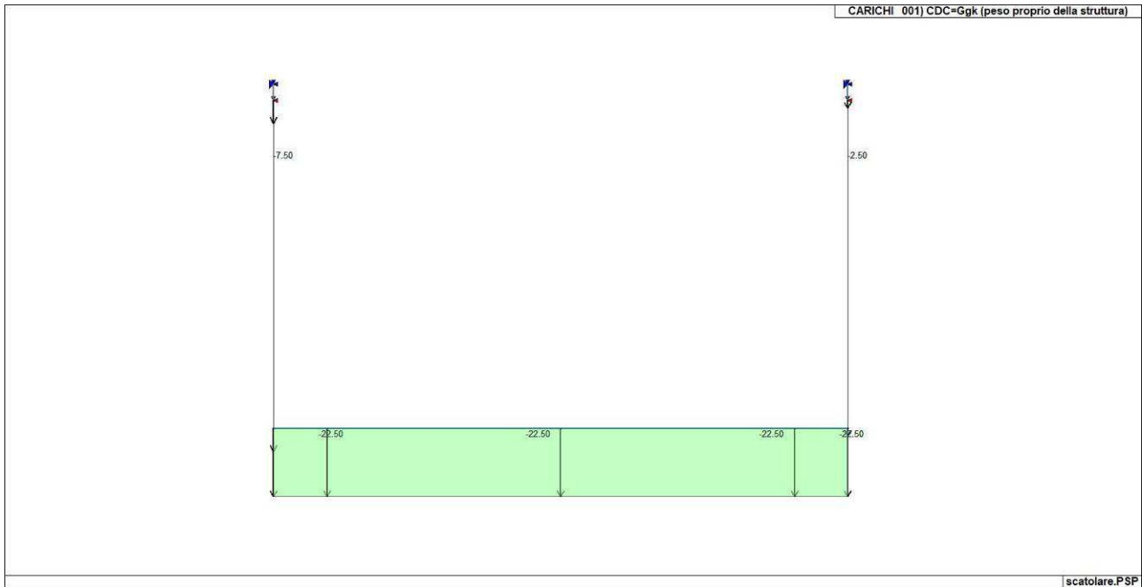
Figura 66. Caso di carico CDC 1 (Peso proprio della struttura)
