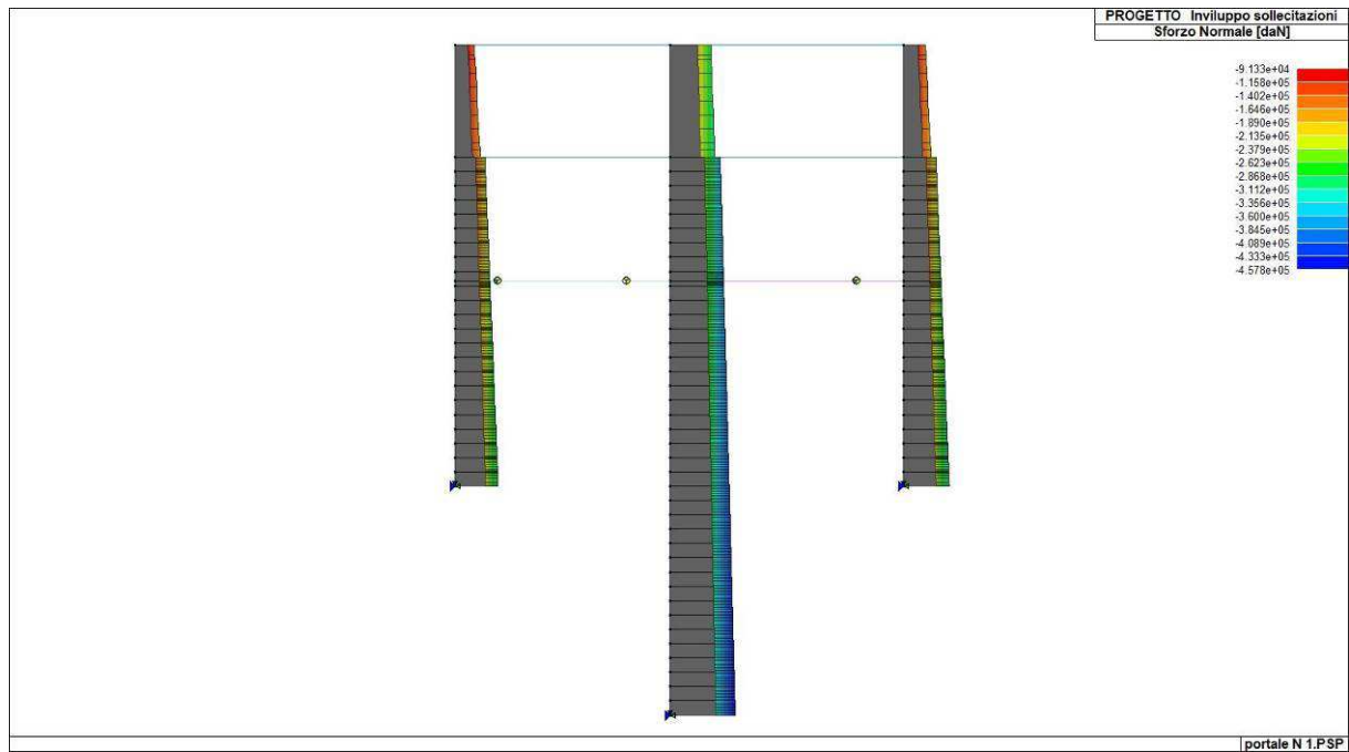
Figura 32. Inviluppo dello sforzo normale di diaframmi e piedritti
