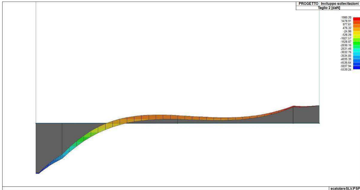
Figura 83. Inviluppo del taglio del solettone di fondazione
