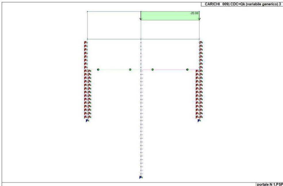
Figura 25. Caso di carico CDC 9 (Accidentale 3)
