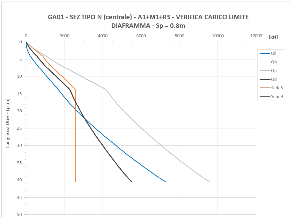
Figura 120. Curva di capacità portante diaframma centrale sezione N
