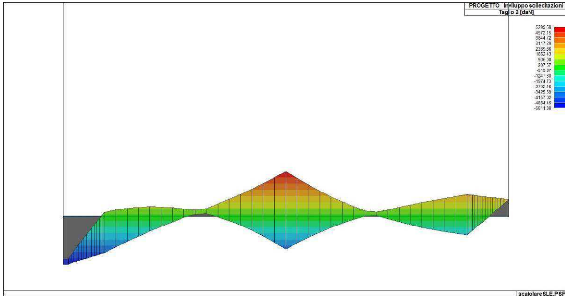
Figura 89. Involuppo del taglio del solettone di fondazione
