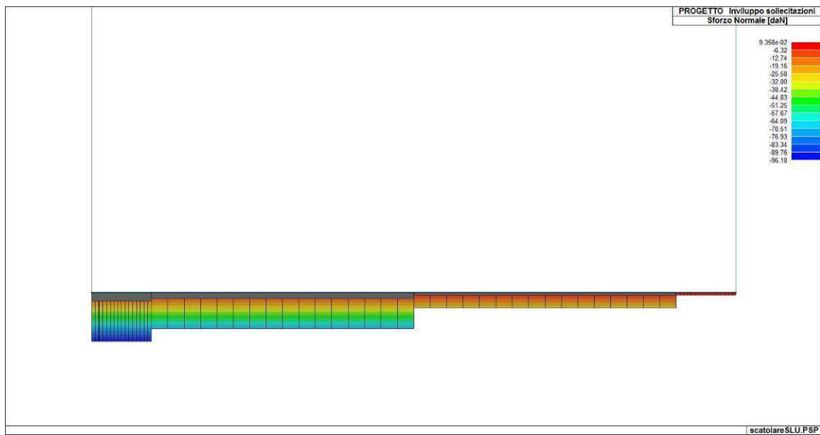
Figura 76. Involuppo dello sforzo normale del solettone di fondazione
