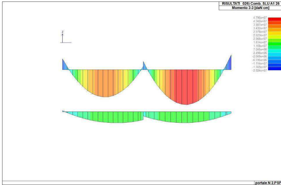
Figura 44. Momento flettente massimo solettone di copertura (combinazione 26)
