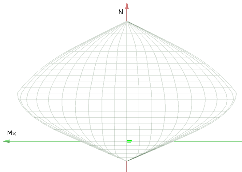
Figura 105. Dominio M-N
