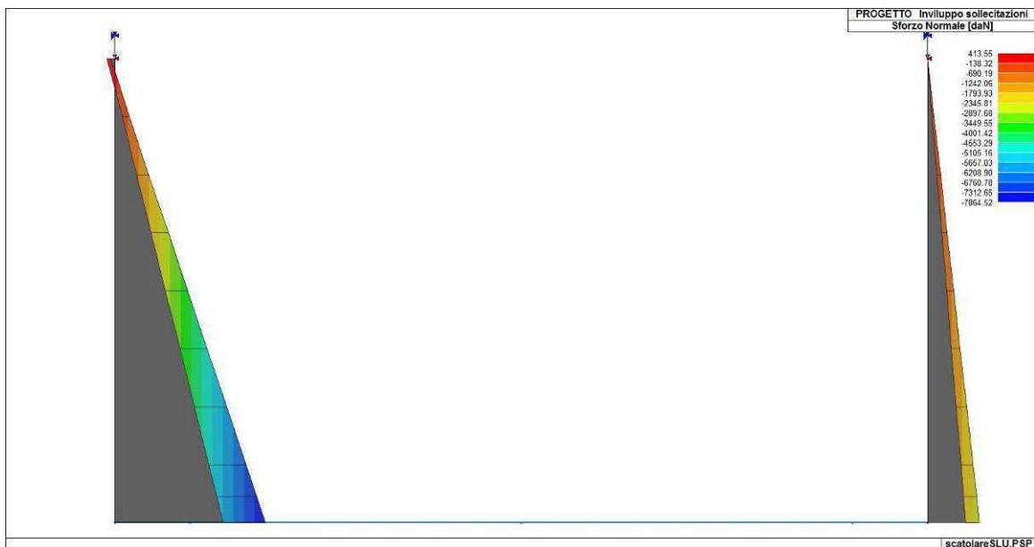
Figura 73. Involuppo dello sforzo normale delle fodere
