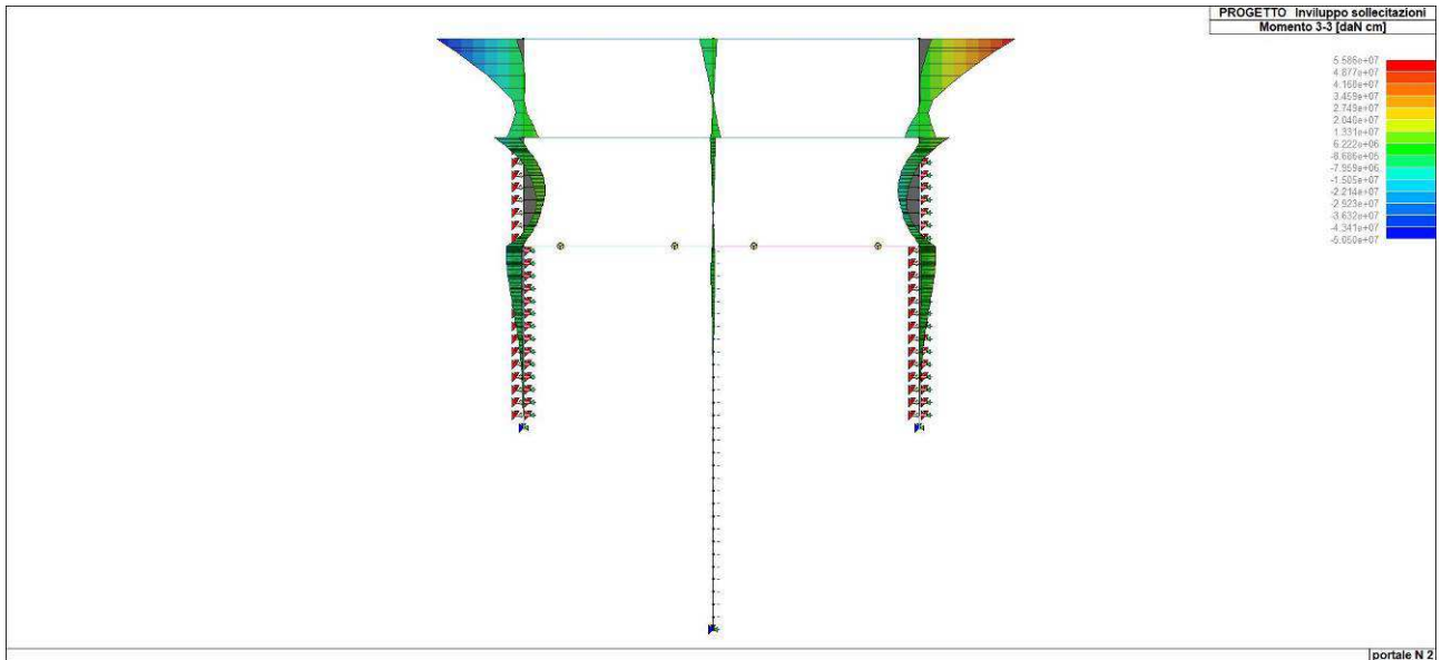
Figura 48. Inviluppo del momento flettente di diaframmi e piedritti
