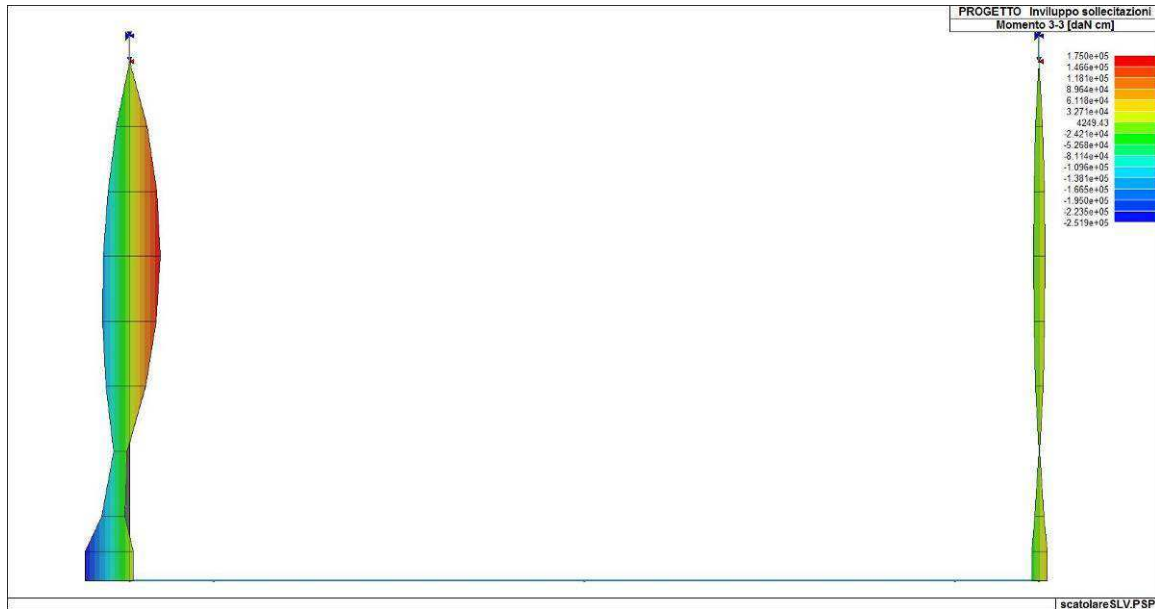
Figura 81. Involuppo del momento flettente delle fodere
