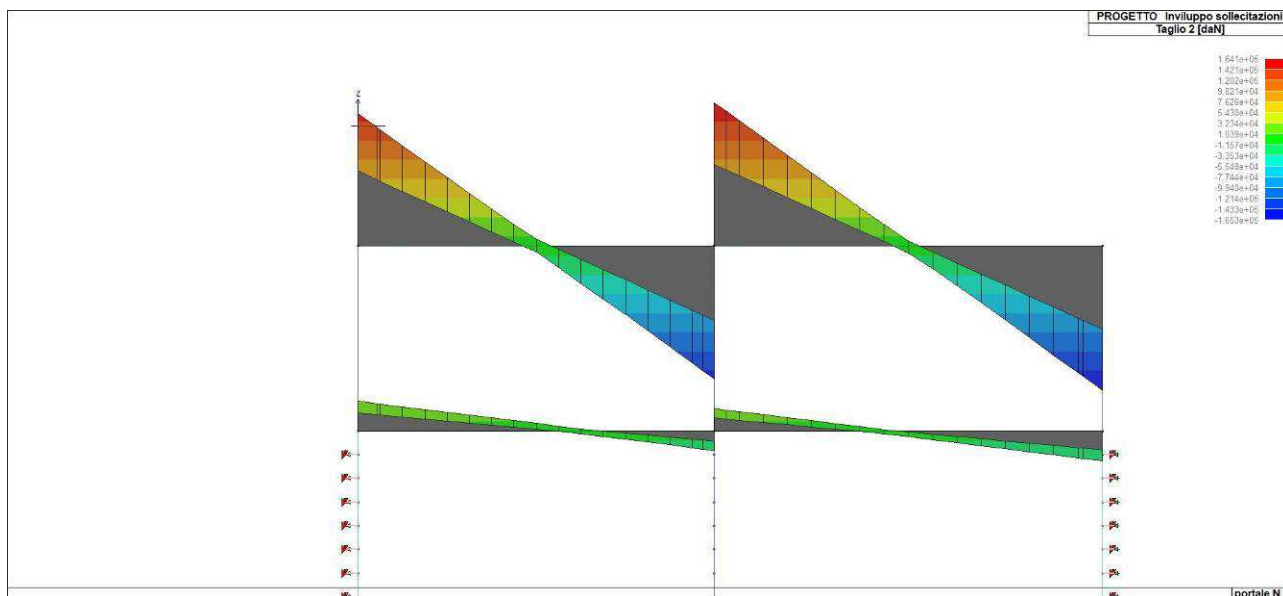
Figura 50. Involuppo del taglio del solettone di copertura
