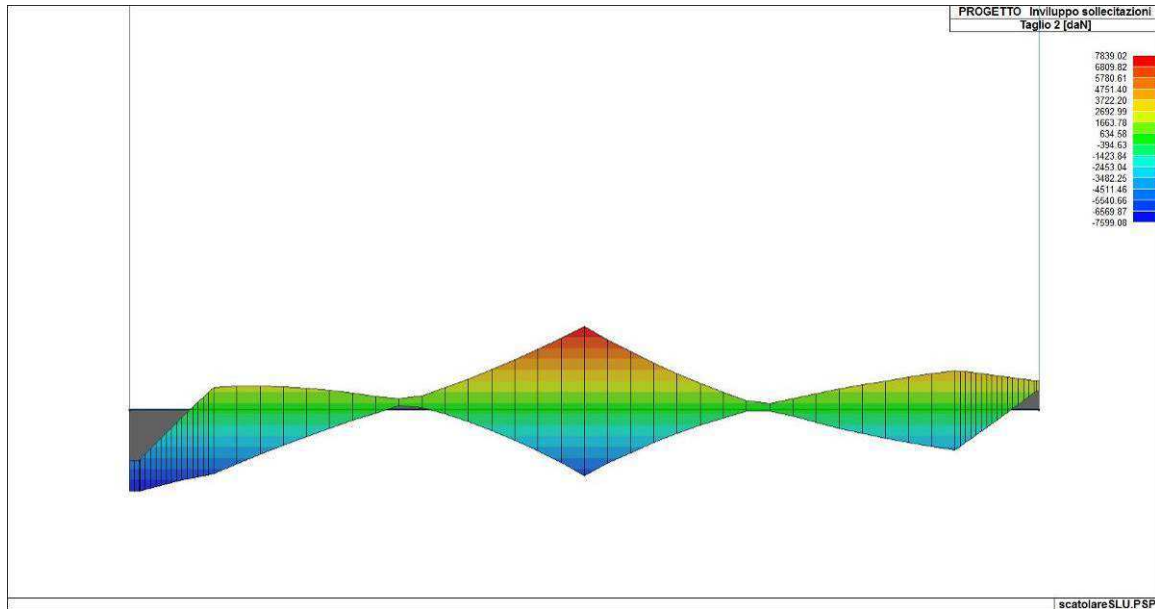
Figura 77. Involuppo del taglio del solettone di fondazione
