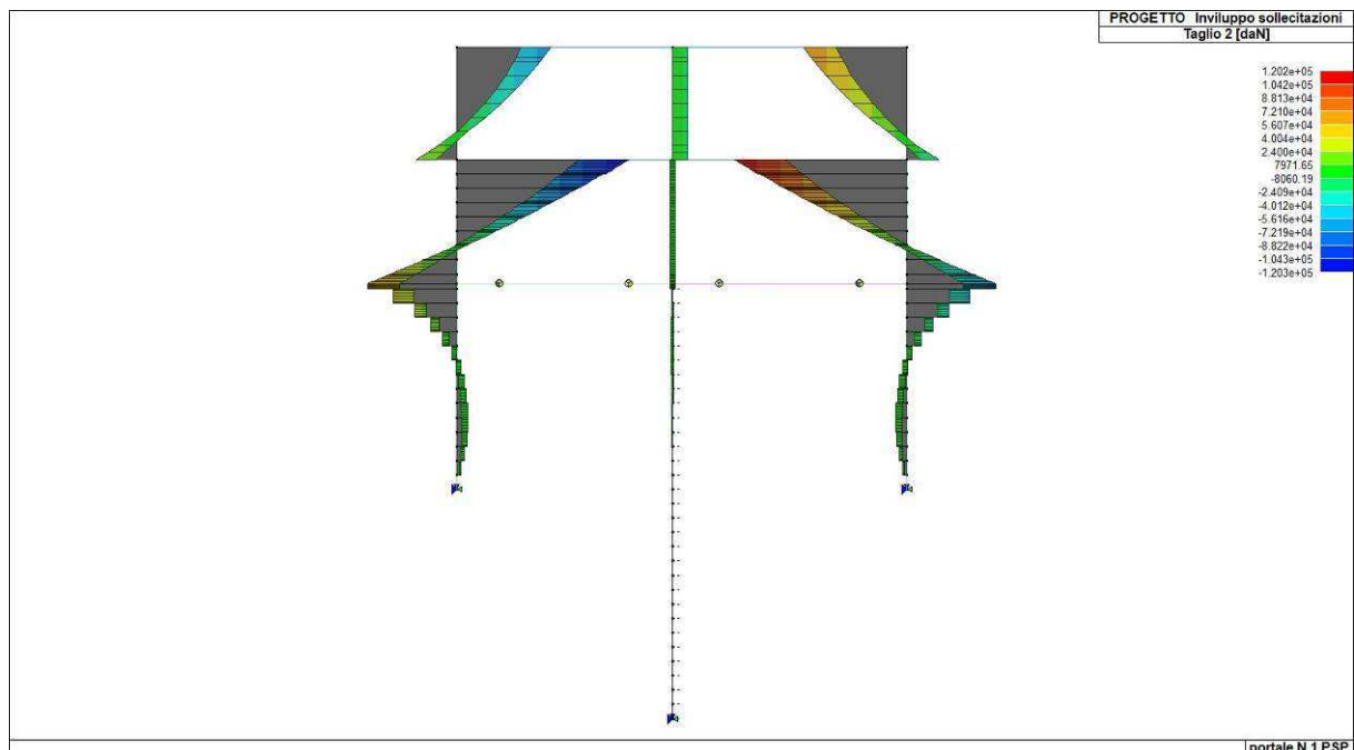
Figura 33. Inviluppo del taglio di diaframmi e piedritti
