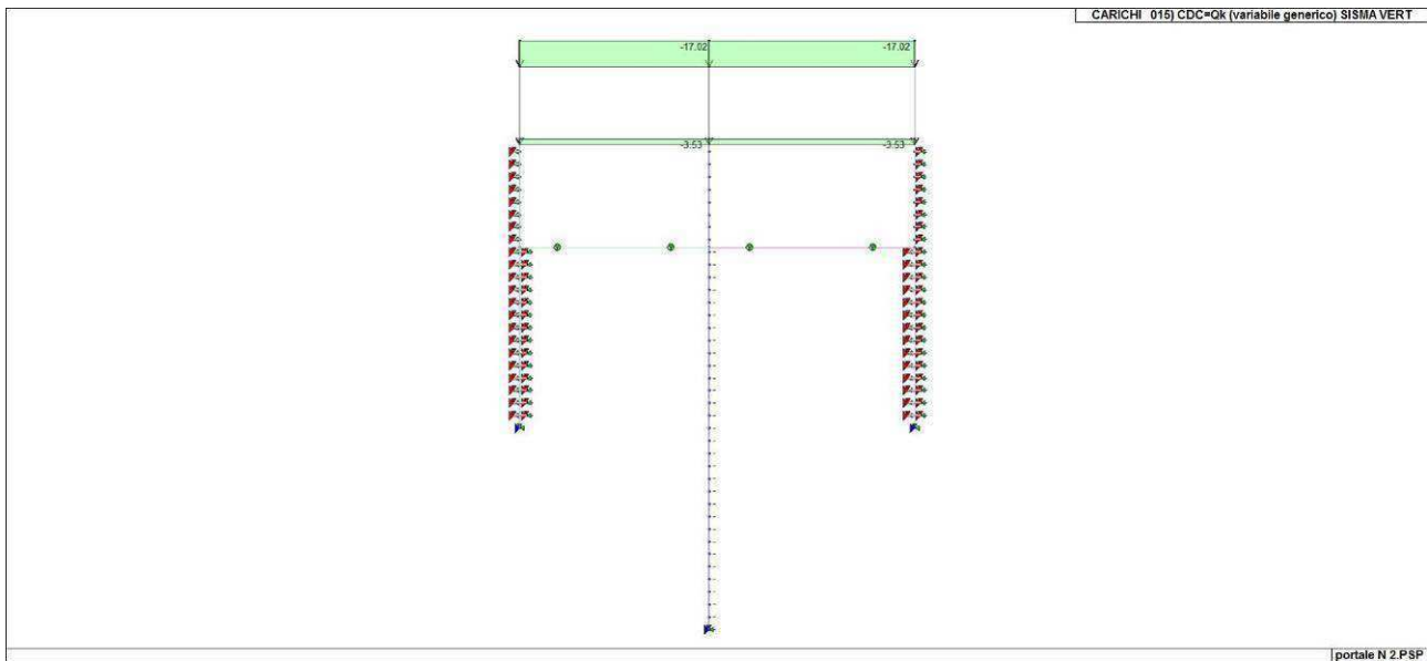
Figura 31. Caso di carico CDC 15 (Sisma verticale)
