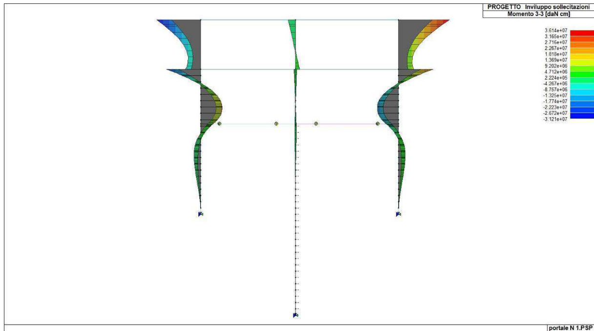
Figura 34. Involuppo del momento flettente di diaframmi e piedritti
