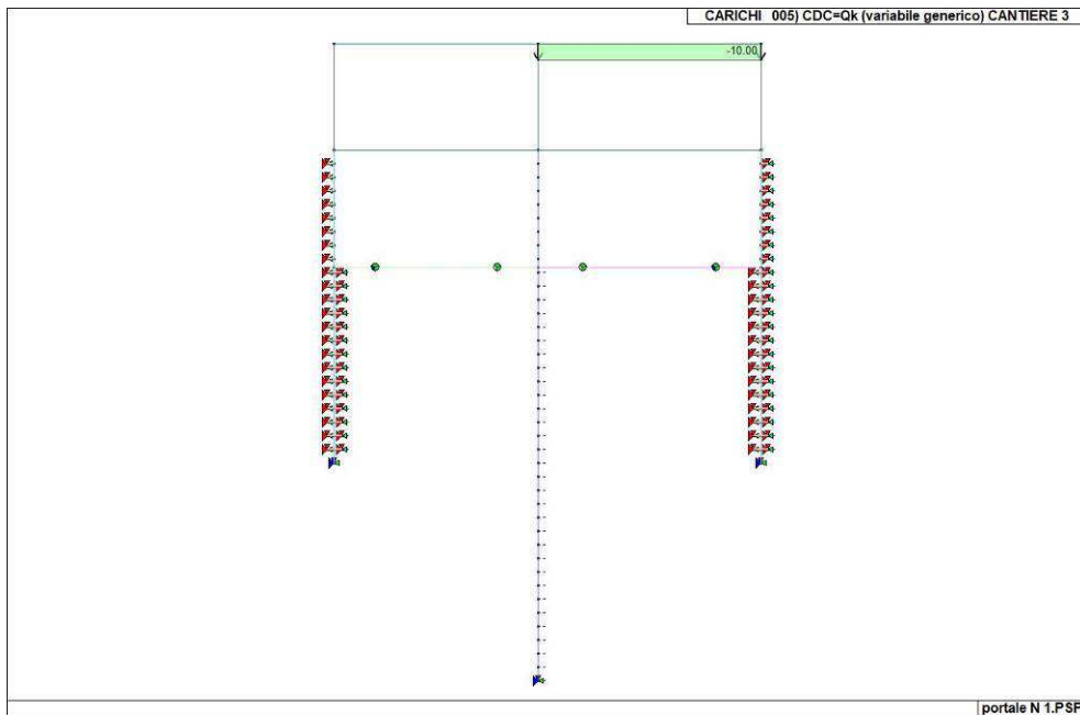
Figura 21. Caso di carico CDC 5 (Cantiere 3)
