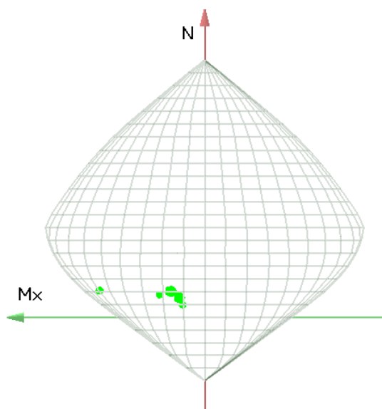
Figura 93. Dominio M-N
