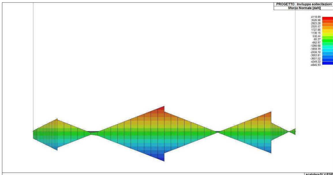
Figura 82. Involuppo dello sforzo normale del solettone di fondazione
