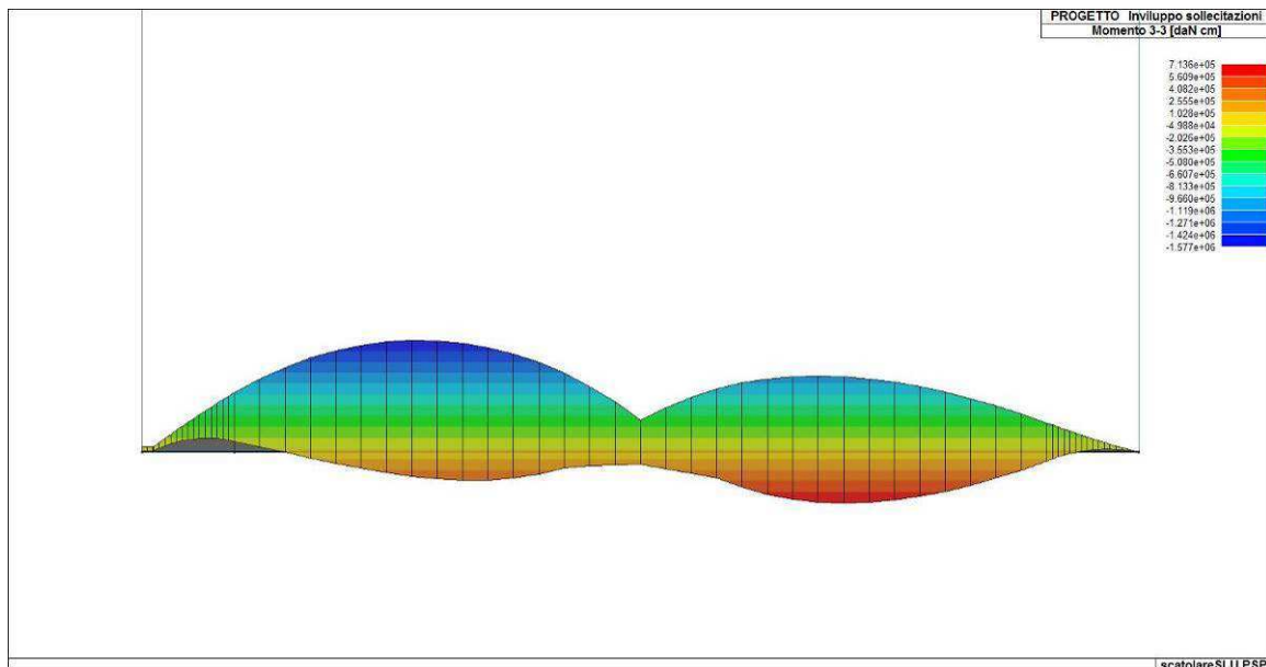
Figura 78. Involuppo del momento flettente del solettone di fondazione
