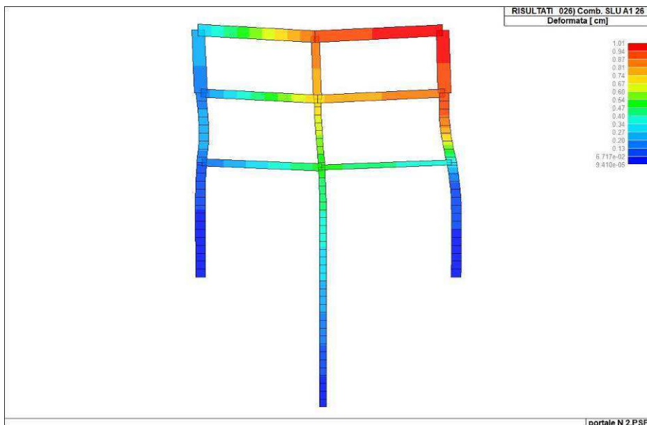
Figura 45. Deformata (combinazione 26)
