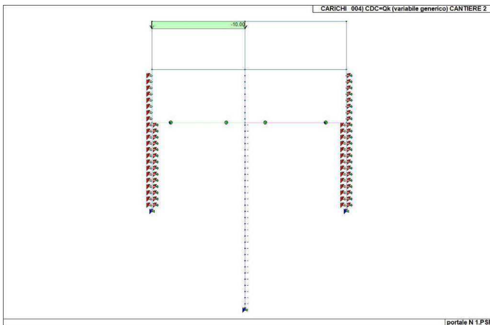
Figura 20. Caso di carico CDC 4 (Cantiere 2)
