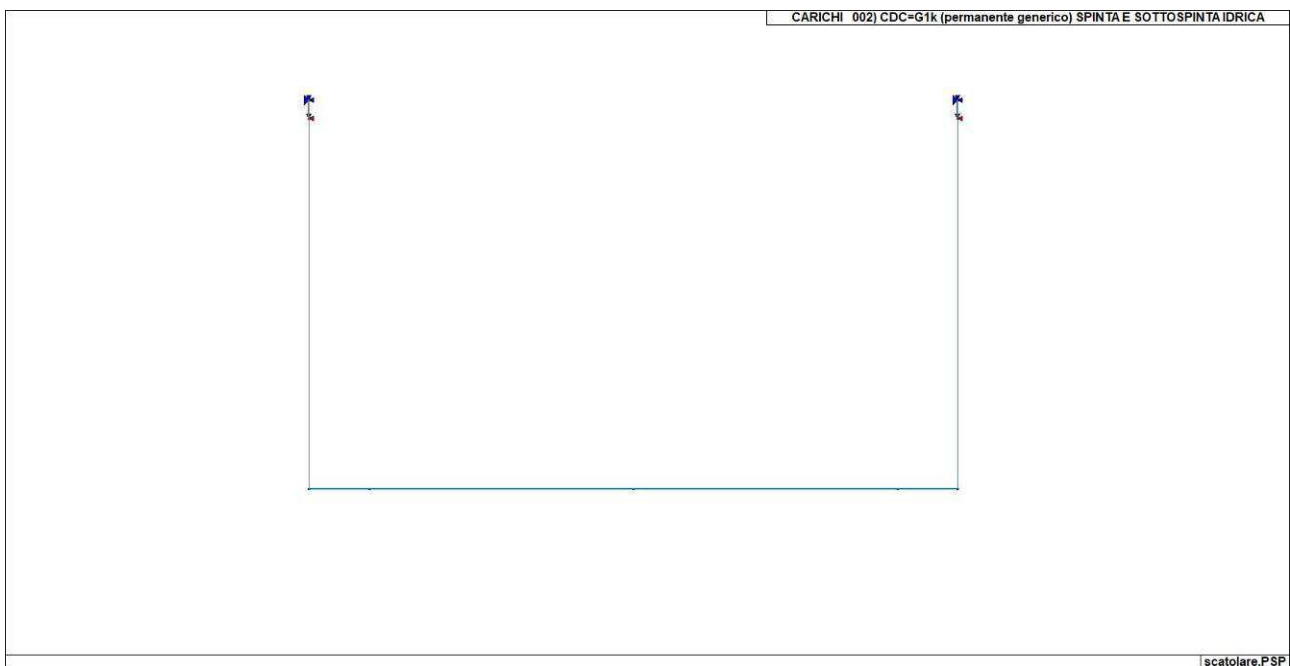
Figura 67. Caso di carico CDC 2 (Permanente spinta e sottospinta)
