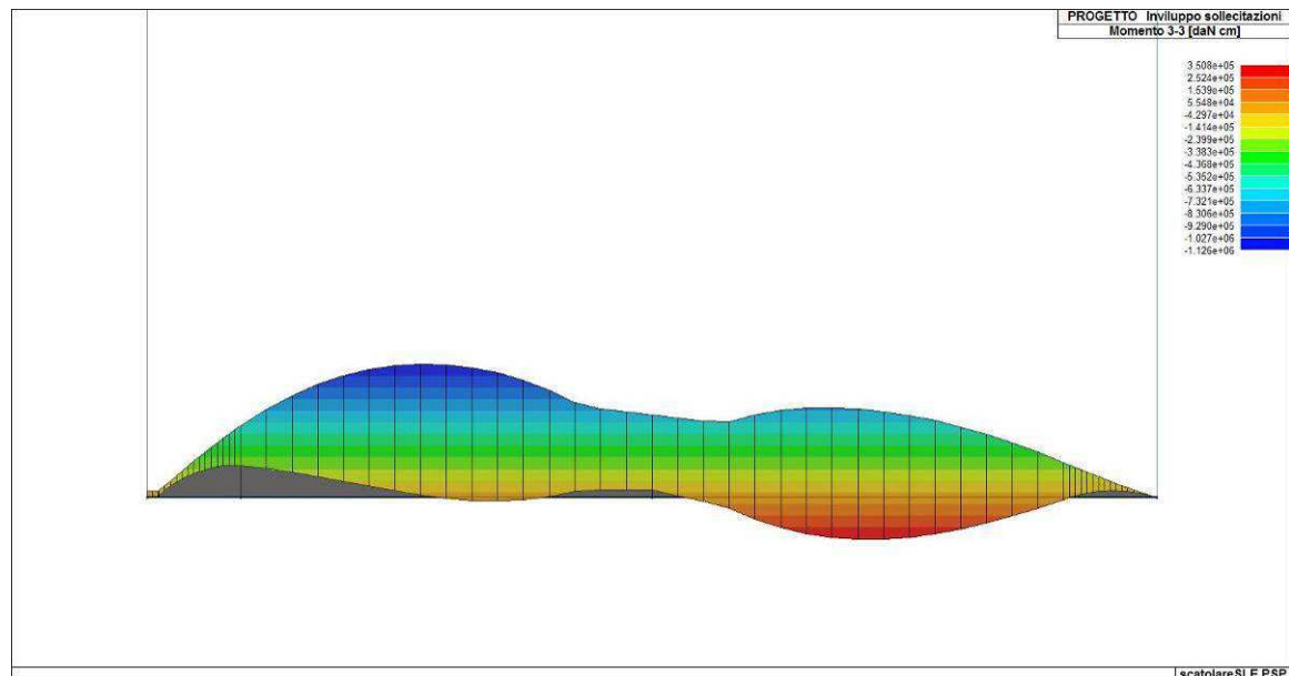
Figura 90. Involuppo del momento flettente del solettone di fondazione
