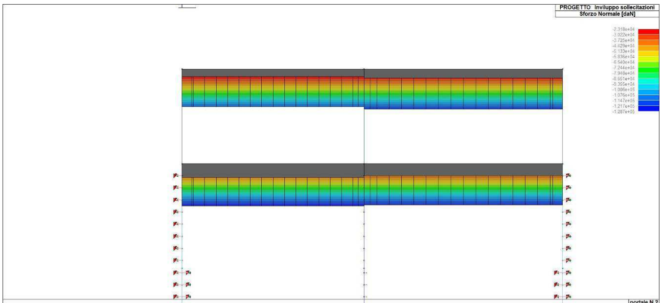
Figura 49. Inviluppo dello sforzo normale del solettone di copertura
