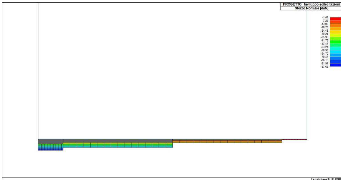
Figura 88. Involuppo dello sforzo normale del solettone di fondazione
