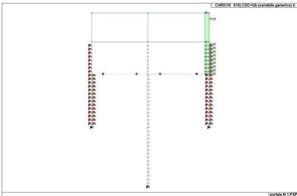
Figura 26. Caso di carico CDC 10 (Accidentale 4)
