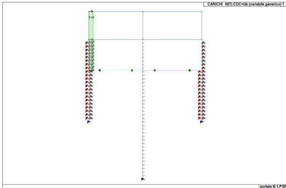
Figura 23. Caso di carico CDC 7 (Accidentale 1)
