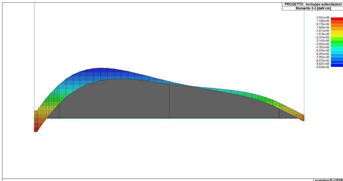
Figura 84. Inviluppo del momento flettente del solettone di fondazione
