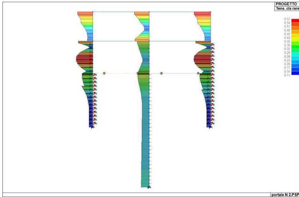
Figura 109. Indice di verifica della tensione del calcestruzzo per combinazioni rare
