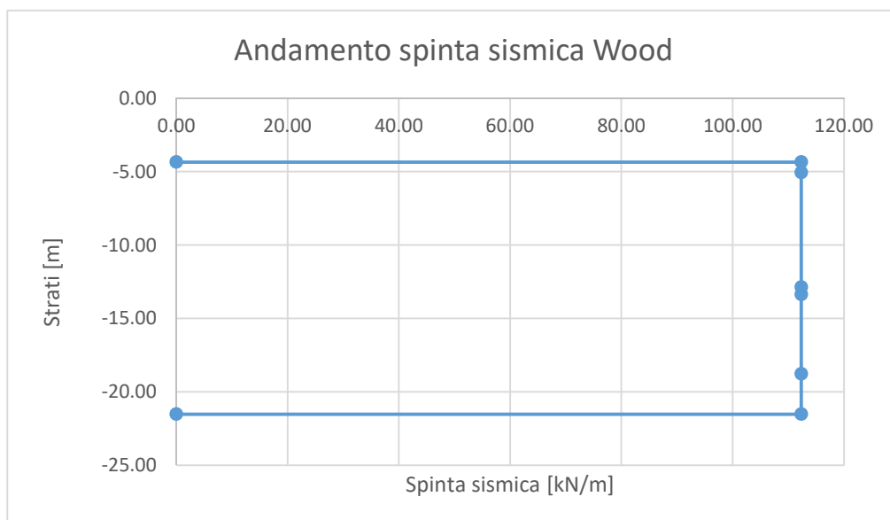
Figura 16. Diagramma andamento spinta Wood
