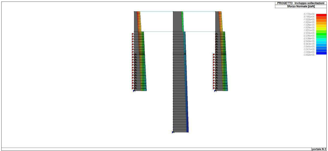
Figura 52. Involuppo dello sforzo normale di diaframmi e piedritti
