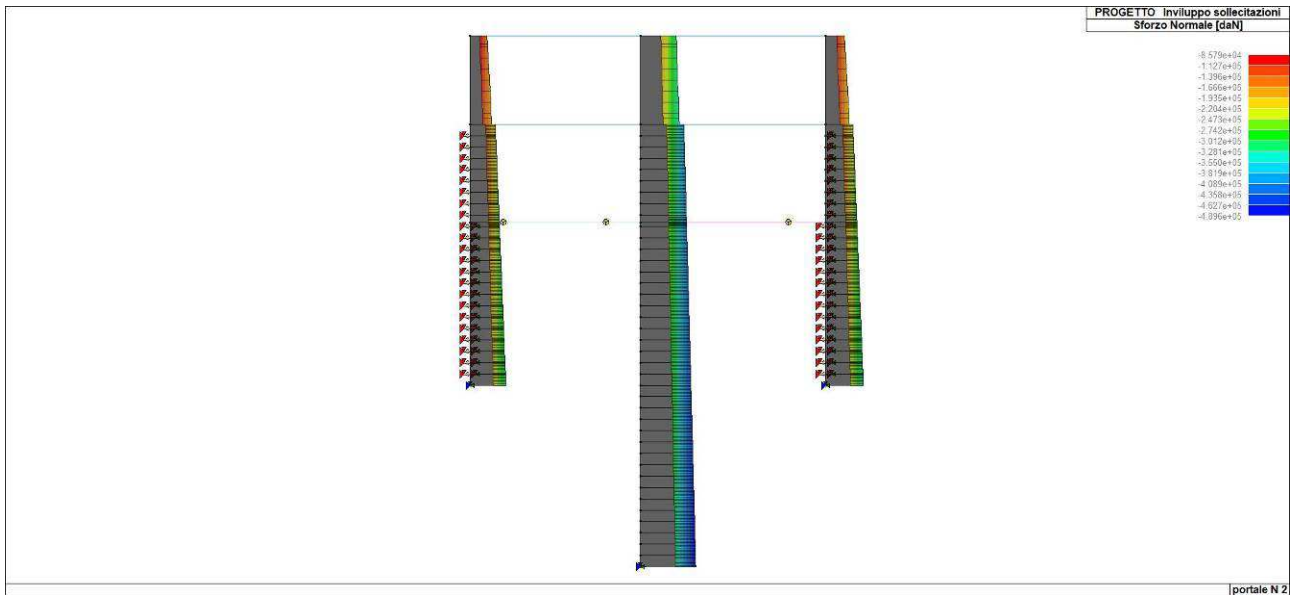
Figura 46. Inviluppo dello sforzo normale di diaframmi e piedritti
