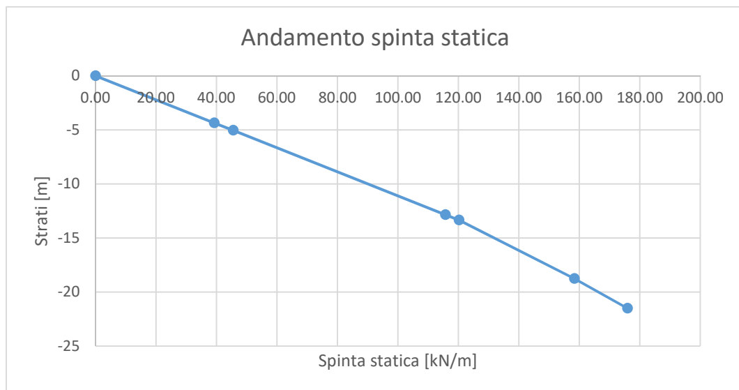
Figura 13. Diagramma andamento spinta statica terreno
