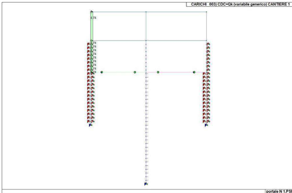
Figura 19. Caso di carico CDC 3 (Cantiere 1)
