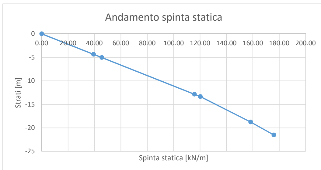
Figura 64. Diagramma andamento spinta Wood
