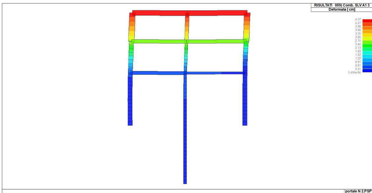
Figura 41. Deformata (combinazione 59)
