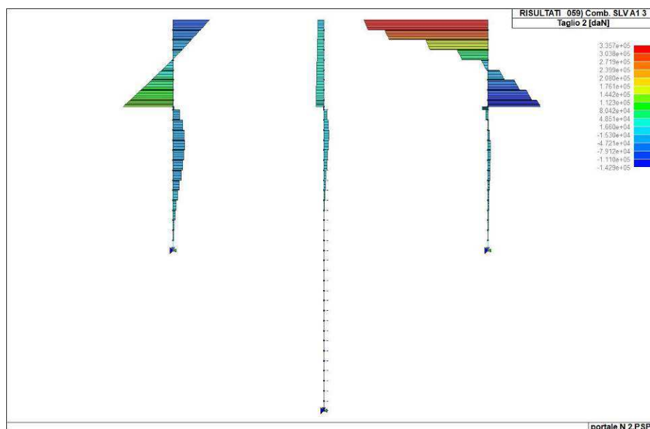
Figura 39. Taglio diaframmi (combinazione 59)
