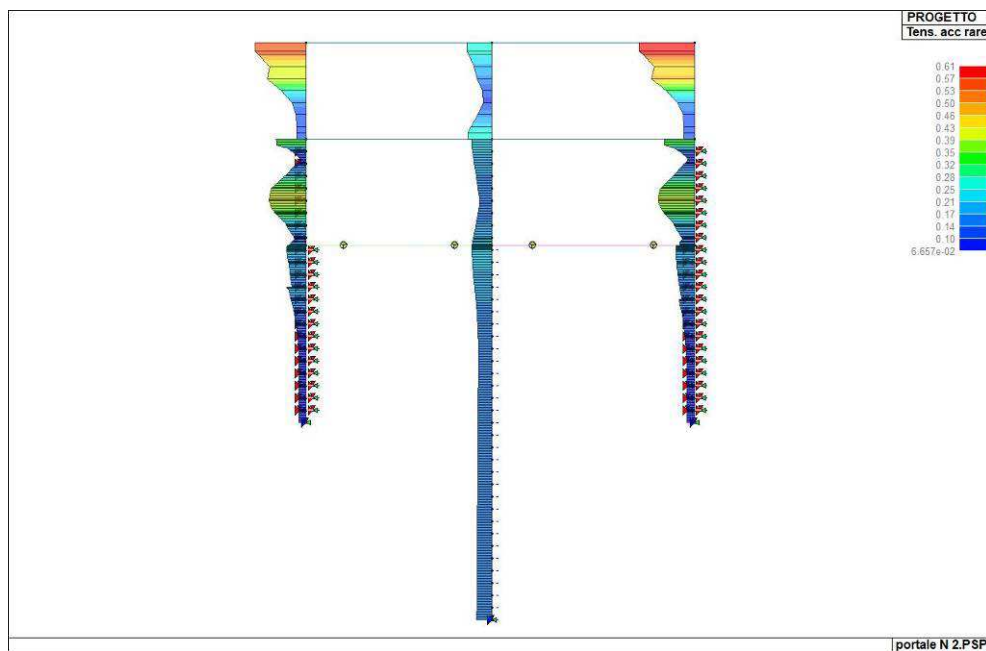
Figura 110. Indice di verifica della tensione dell'acciaio per combinazioni rare
