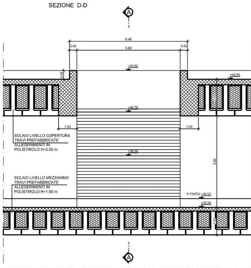
Figura 5. Sezione trasversale
