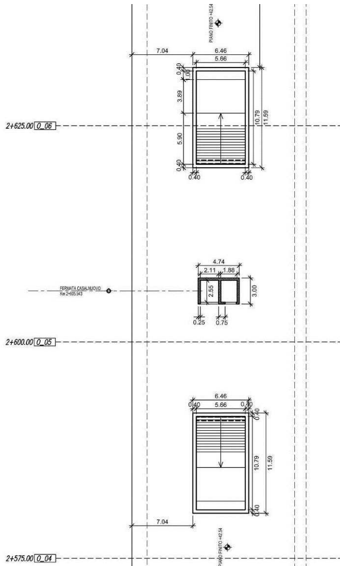
Figura 2. Pianta 1
