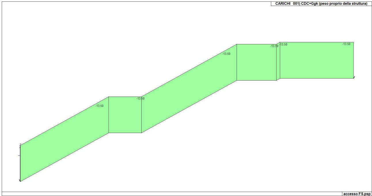
Il caso di carico CDC1 (peso proprio).
