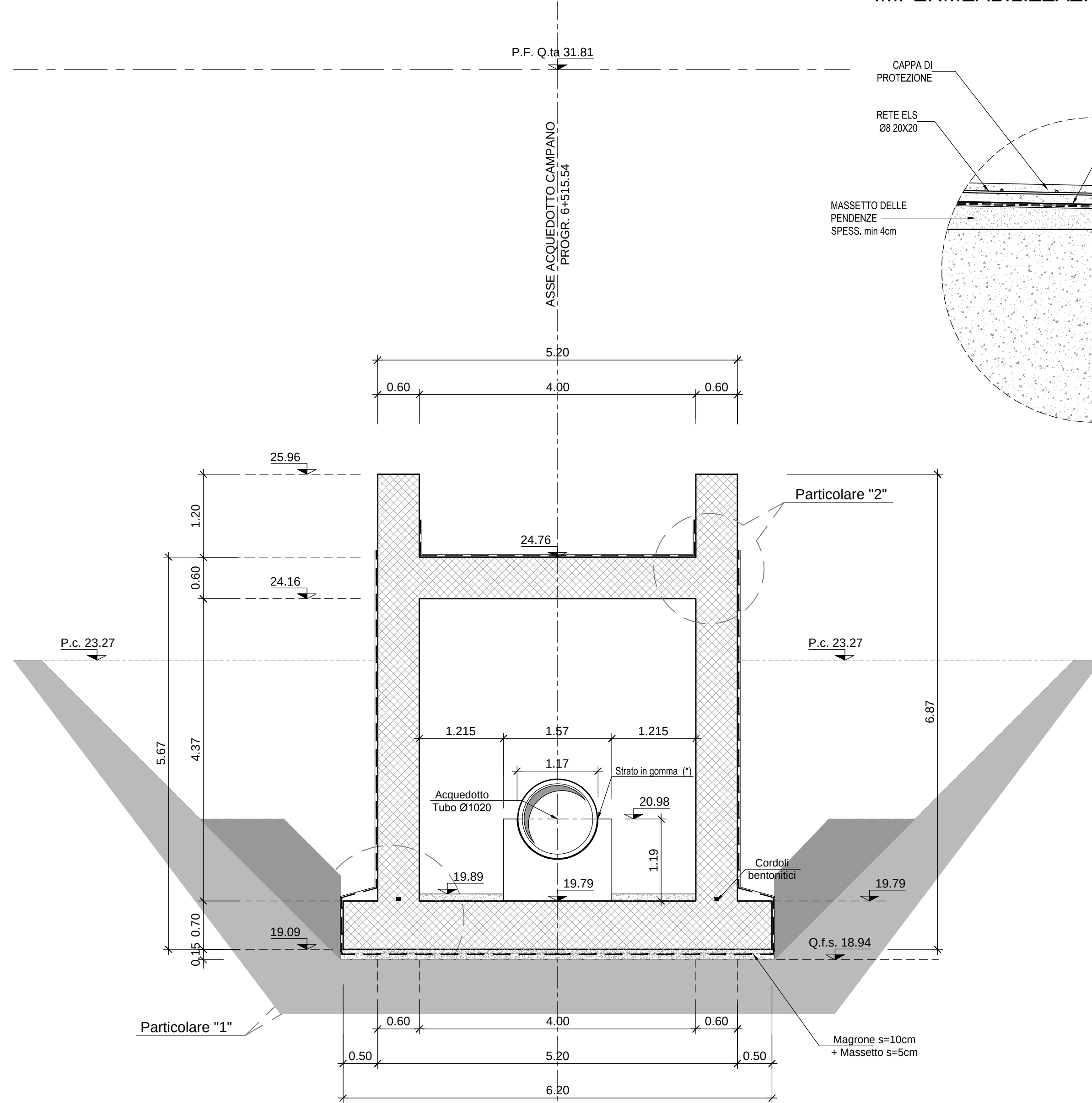
SEZIONE TIPO - B
