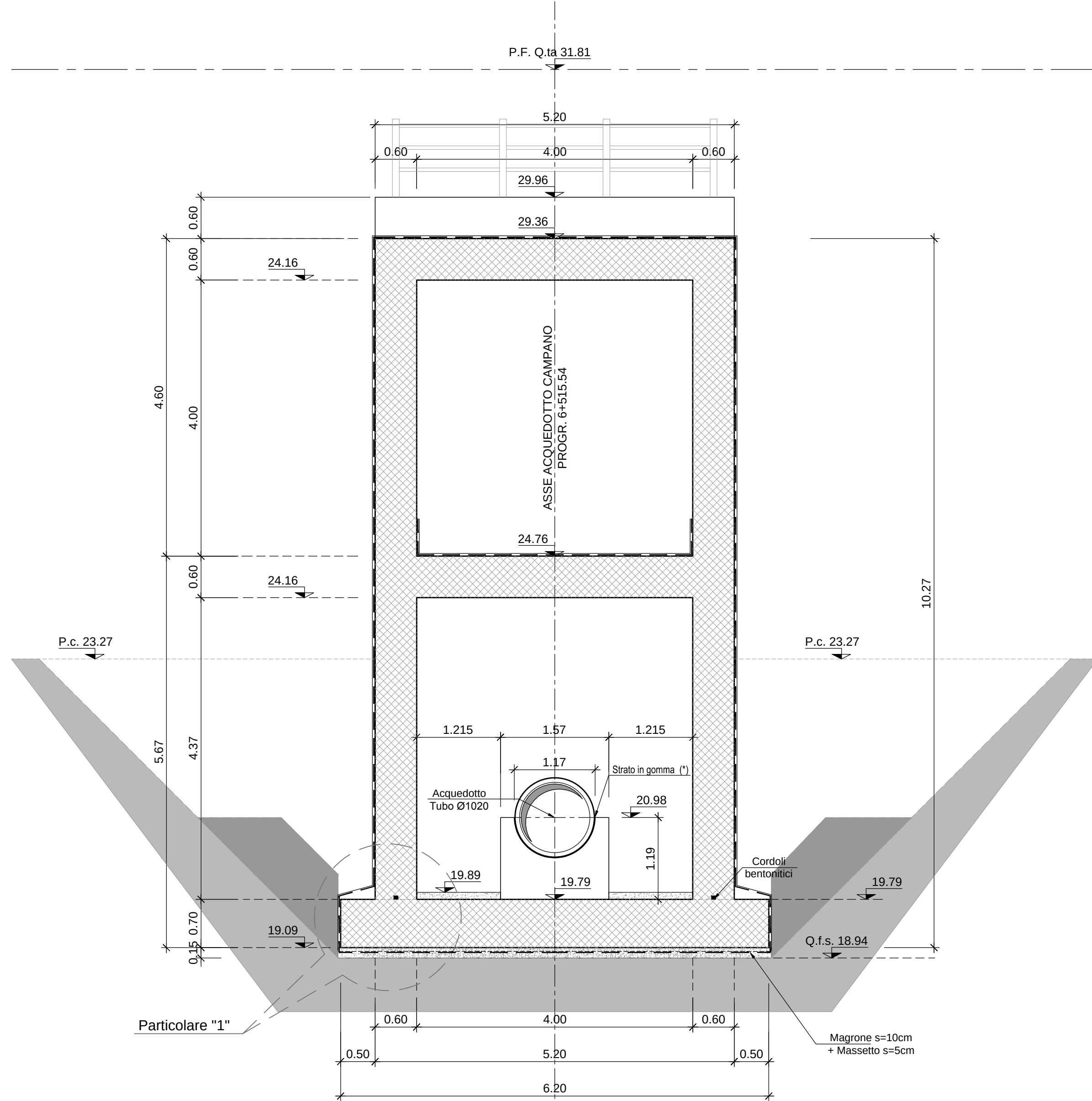
SEZIONE TIPO - A
