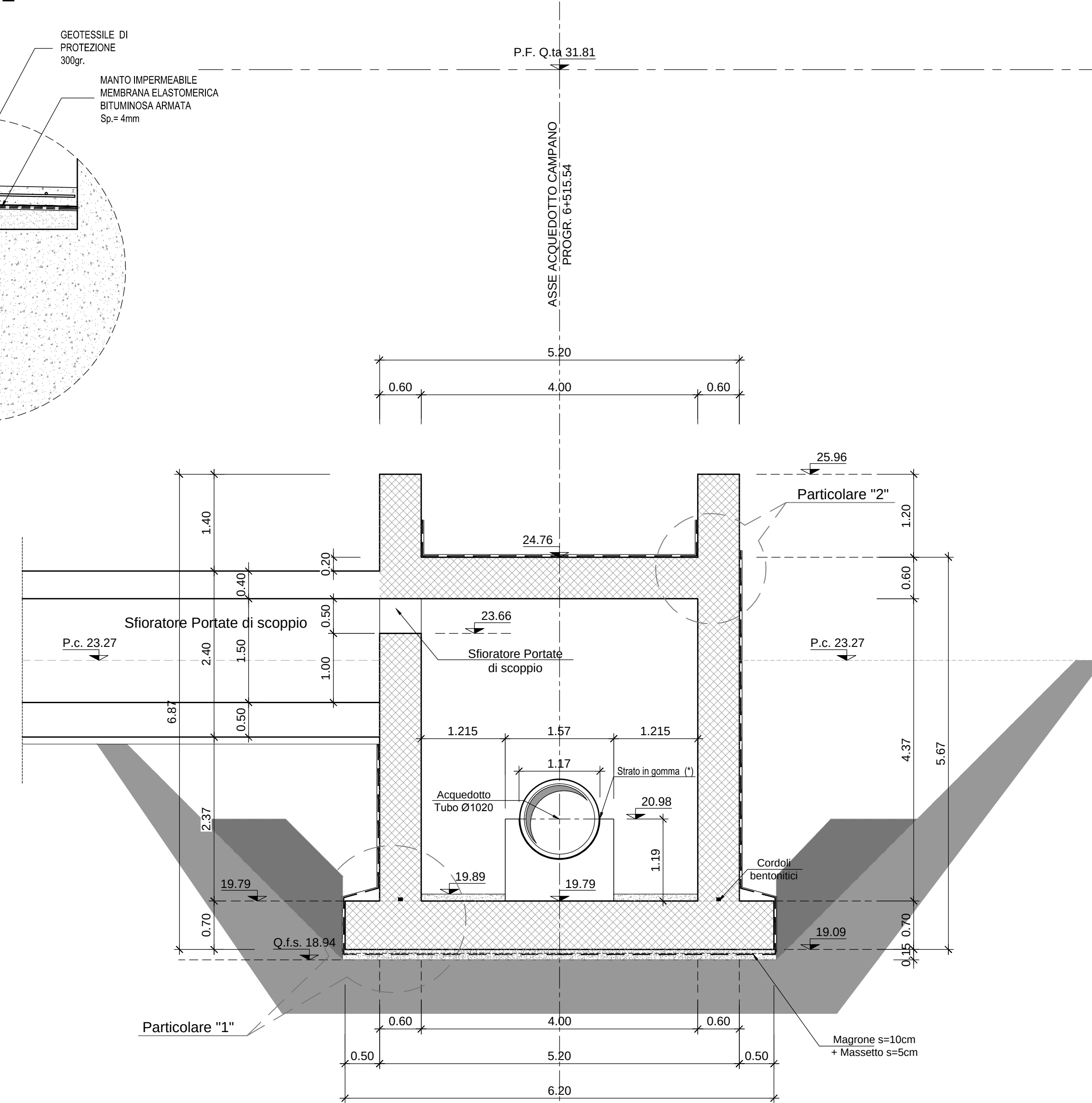
SEZIONE TIPO - C
