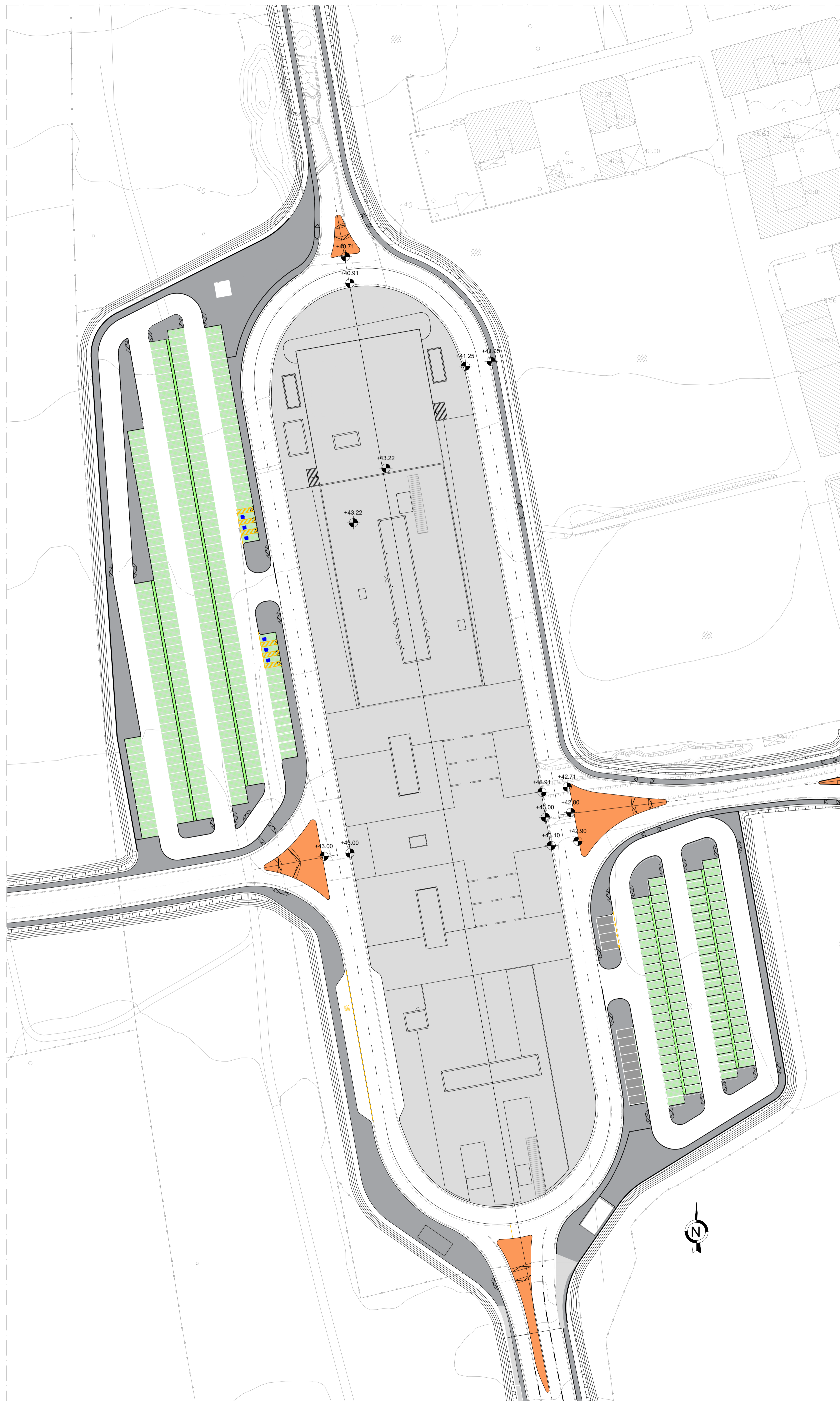
PLANIMETRIA GENERALE Scala 1:500
