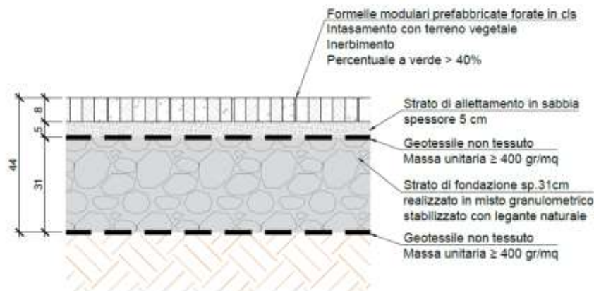
Figura 6: pavimentazione stalli di sosta
