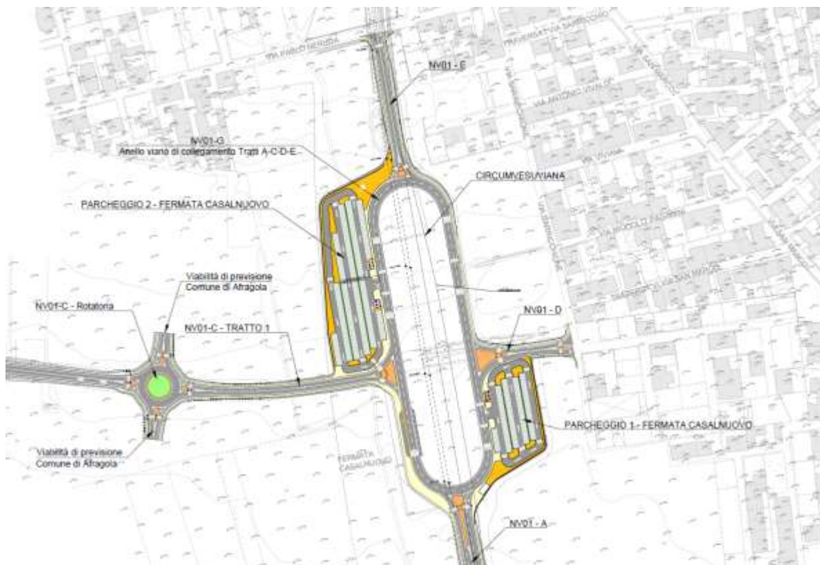
Figura 1: Sistema stradale Stazione Casalnuovo
