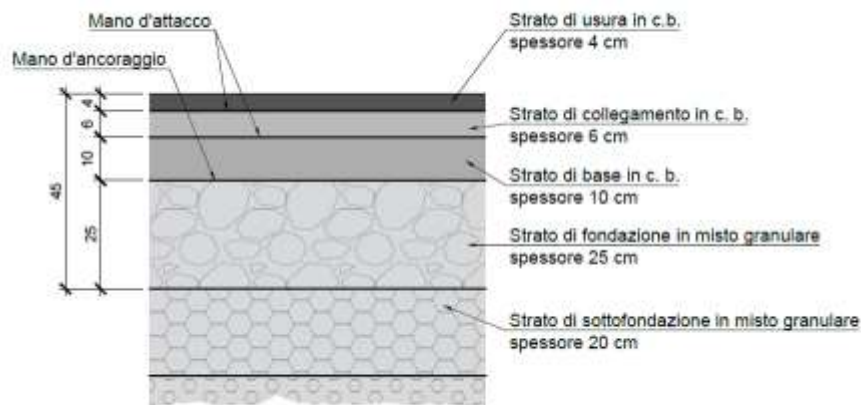
Figura 5: pavimentazione corsie di manovra
