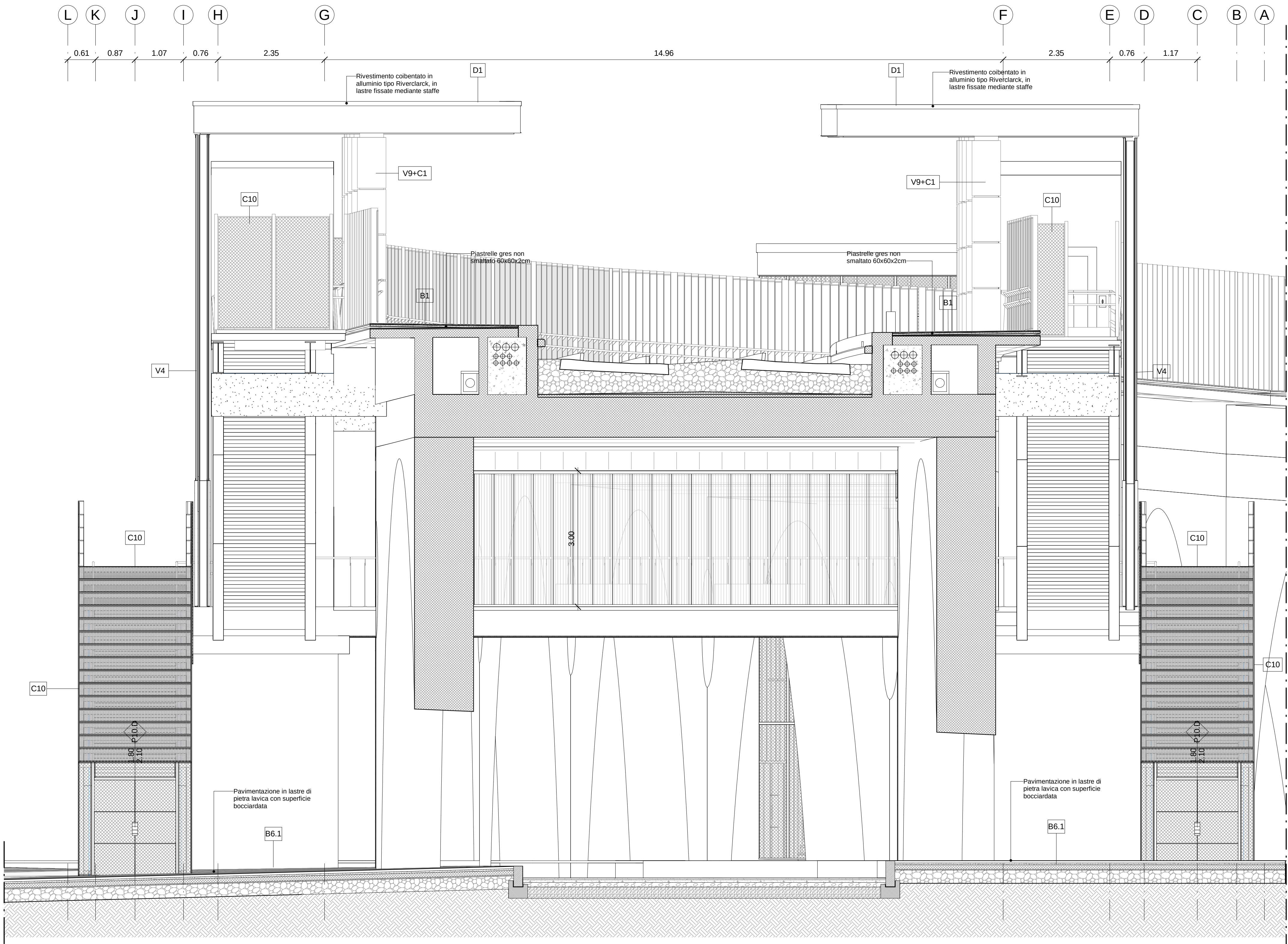
PROSPETTO 4 Scala 1:50
