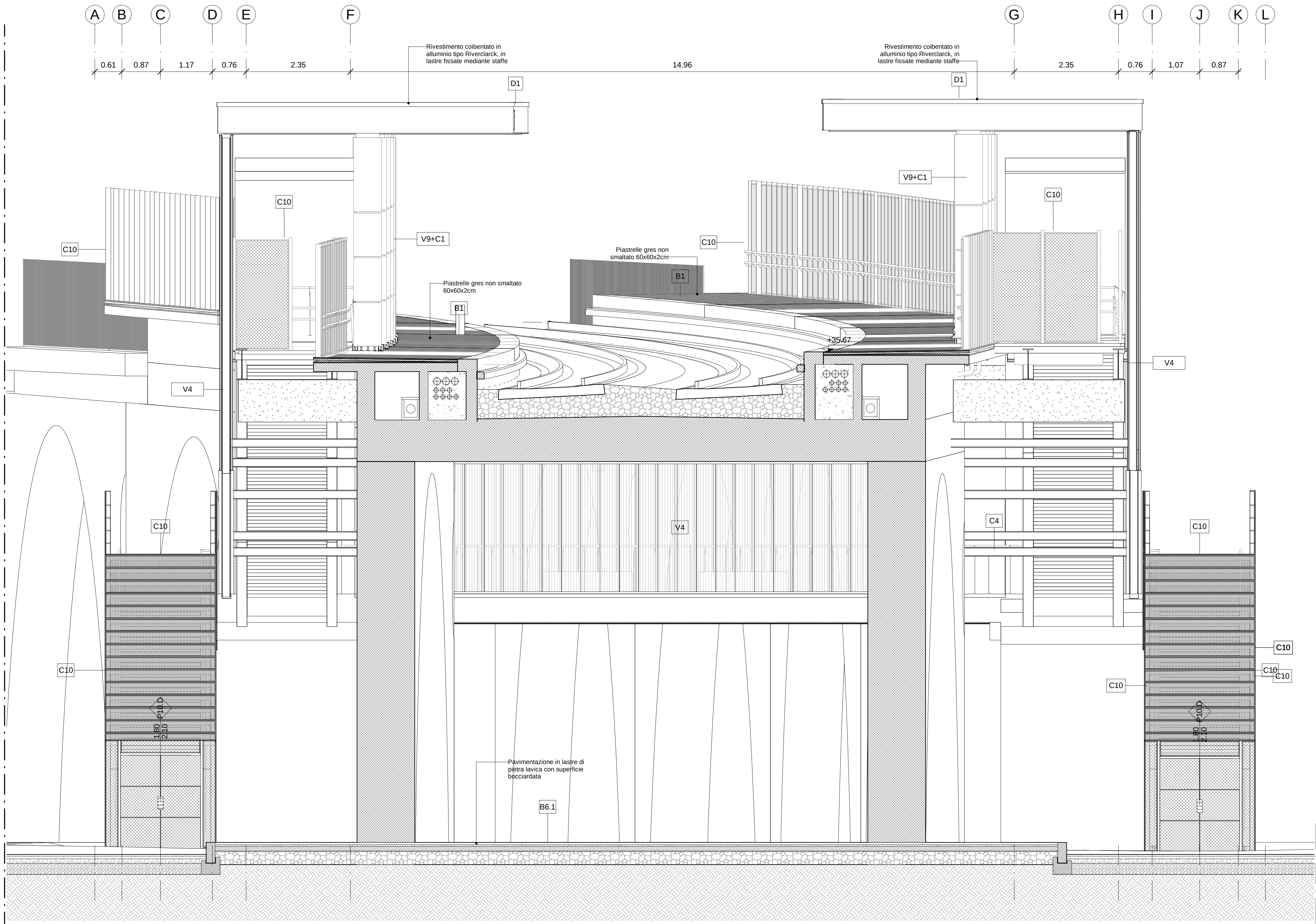
PROSPETTO 2 Scala 1:50
