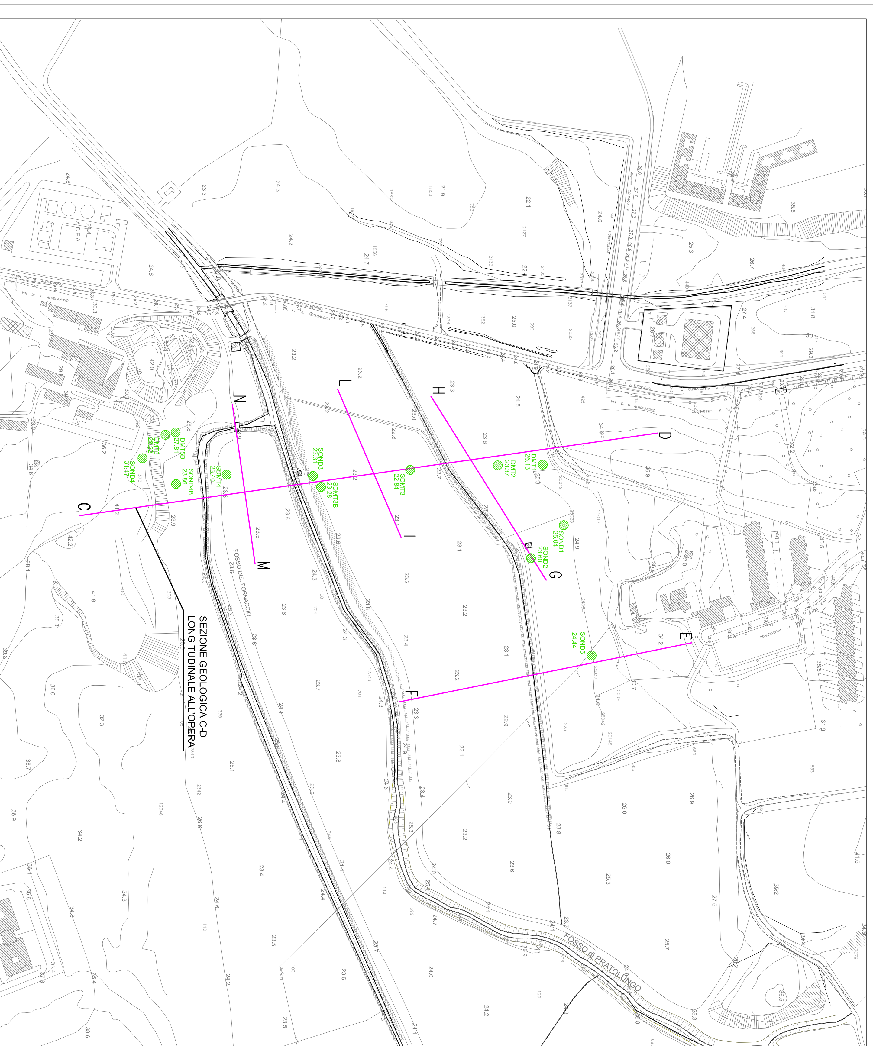
PLANIMETRIA CON UBICAZIONE DELLE SEZIONI GEOLOGICHE - SCALA 1:2000
