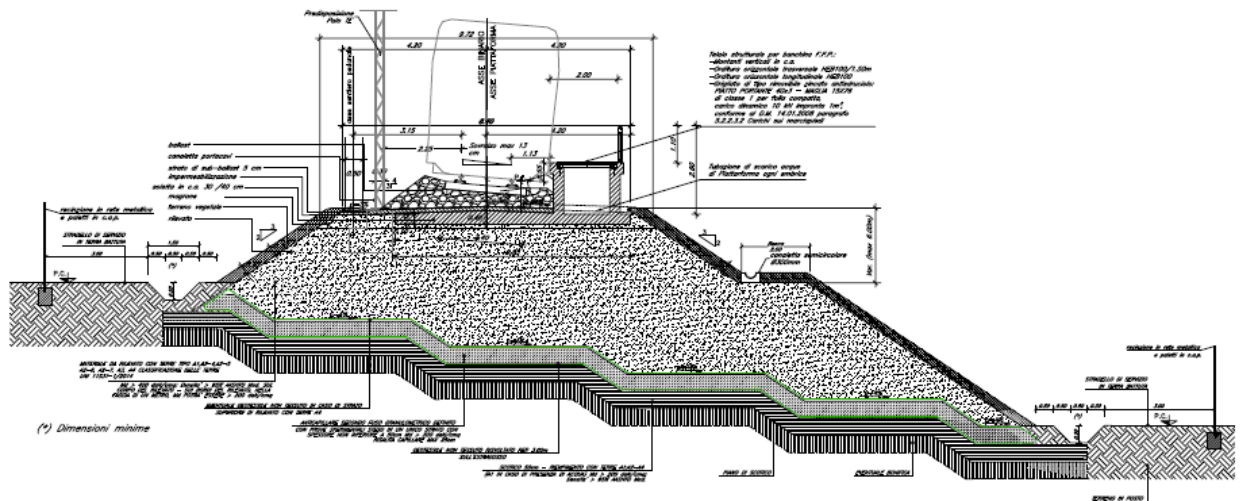
SEZIONI TIPO IN RILEVATO (sezione B-B) CON FFP Scala 1:50
