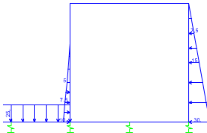
Schema dei carichi permanenti e delle spinte da essi prodotte sull'FFP: dettaglio
