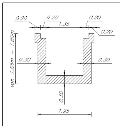
Manufatto in c.a. per FFP in trincea
