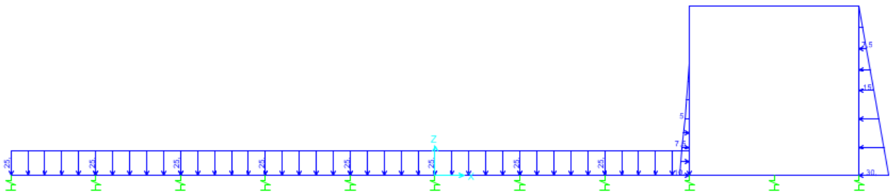
Schema dei carichi permanenti e delle spinte da essi prodotte sull'FFP
