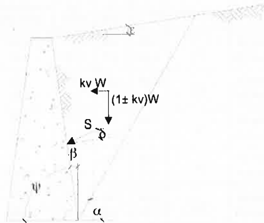
FIGURA 7.1: AZIONI SISMICHE
