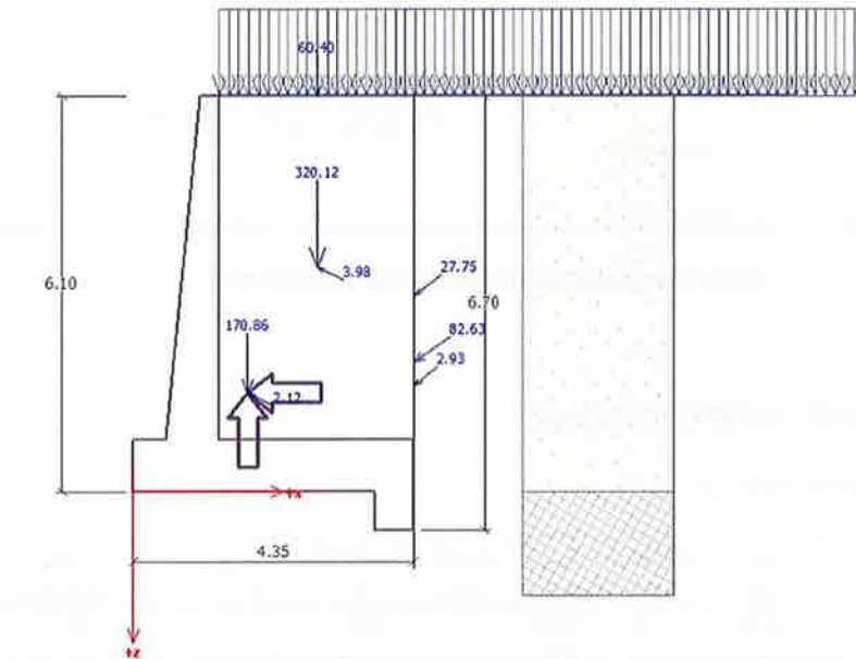
FIGURA 8.7: AZIONI AGENTI SUL MURO DI SOSTEGNO (M1)
