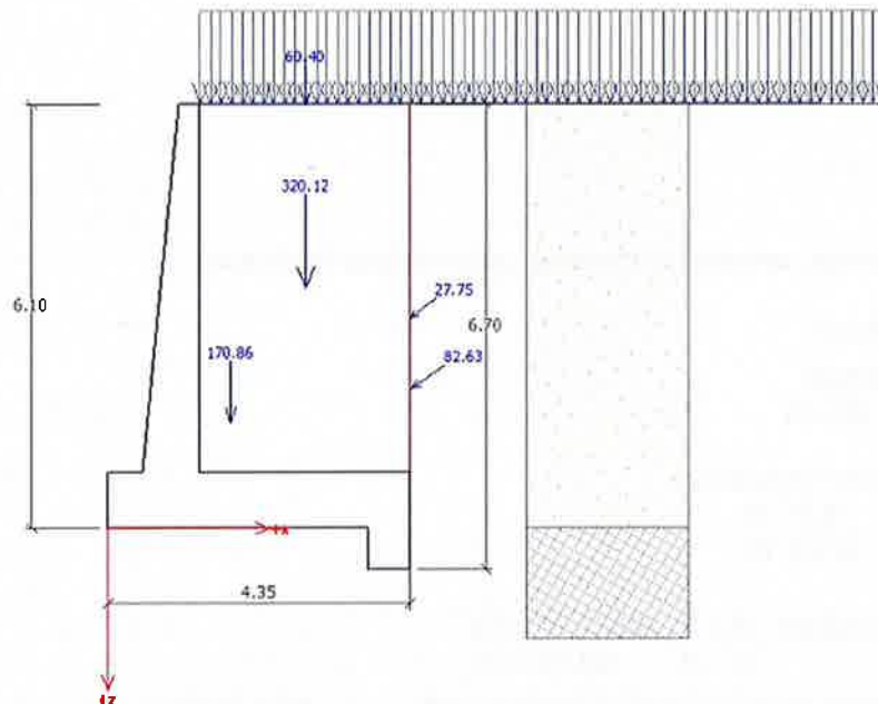
FIGURA 8.6: AZIONI AGENTI SUL MURO DI SOSTEGNO (M1)
