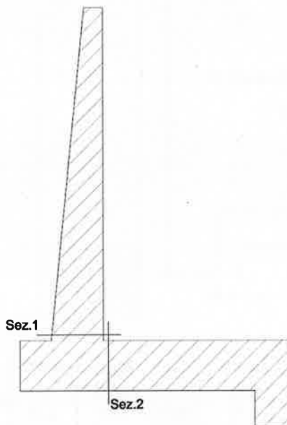
FIGURA 8.11: SEZIONI DI VERIFICA
