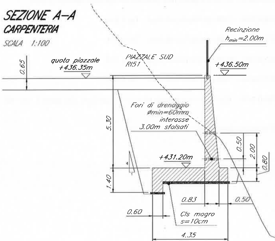
FIGURA 1.3: SEZIONE DI CALCOLO
