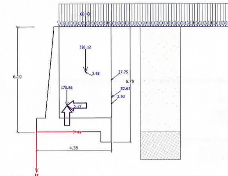
FIGURA 8.10: AZIONI AGENTI SUL MURO DI SOSTEGNO (M1)
