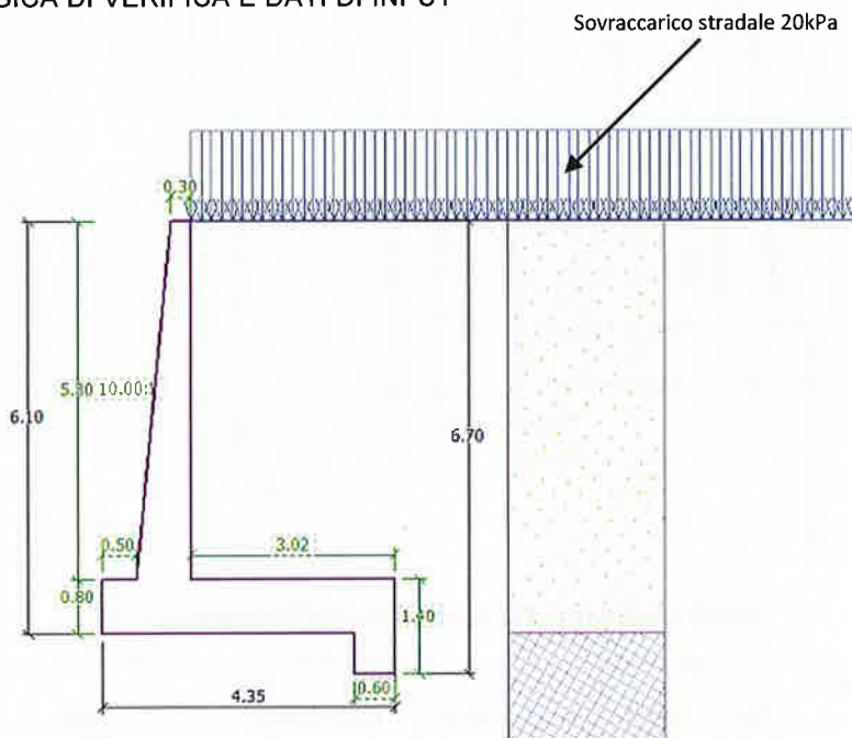
FIGURA 8.1: SEZIONE TIPOLOGICA DI VERIFICA
