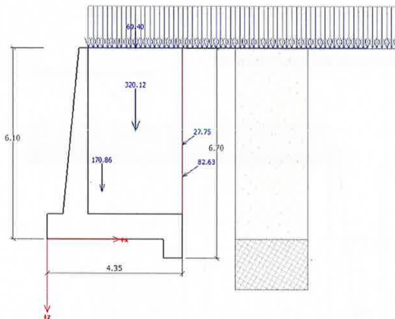
FIGURA 8.3: AZIONI AGENTI SUL MURO DI SOSTEGNO (M1)
