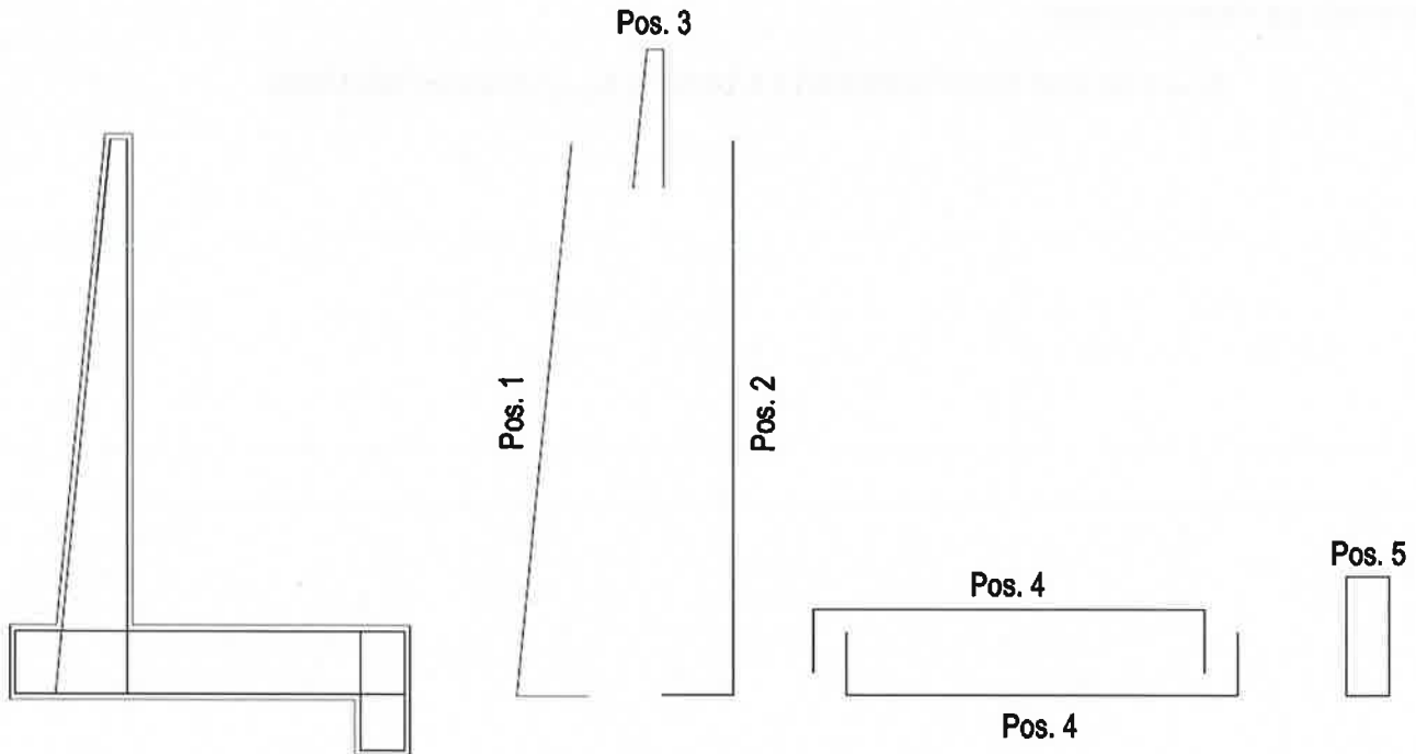
FIGURA 9.1: SCHEMA DELLE ARMATURE
