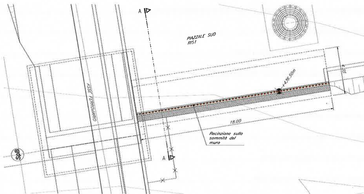
FIGURA 1.1: PLANIMETRIA
