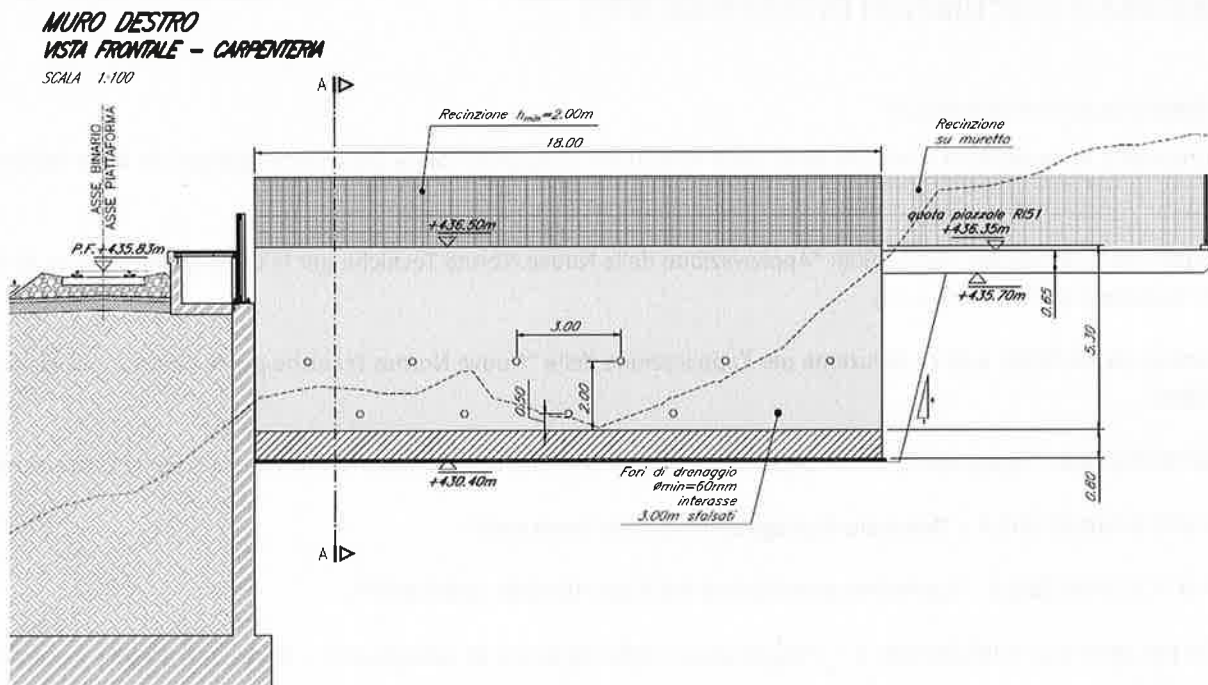
FIGURA 1.2: PROFILO LONGITUDINALE
