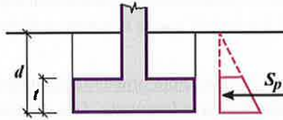
FIGURA 7.6: RESISTENZA DEL TERRENO
