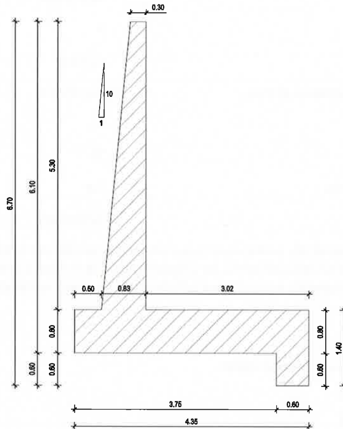
FIGURA 6.1: SEZIONE MURO DI SOSTEGNO
