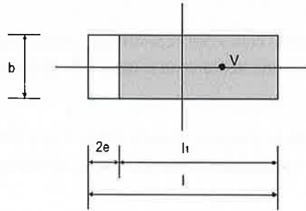
FIGURA 7.5: DETERMINAZIONE DELL'AREA EFFETTIVA NEL CASO DI ECCENTRICITÀ ASSIALE
