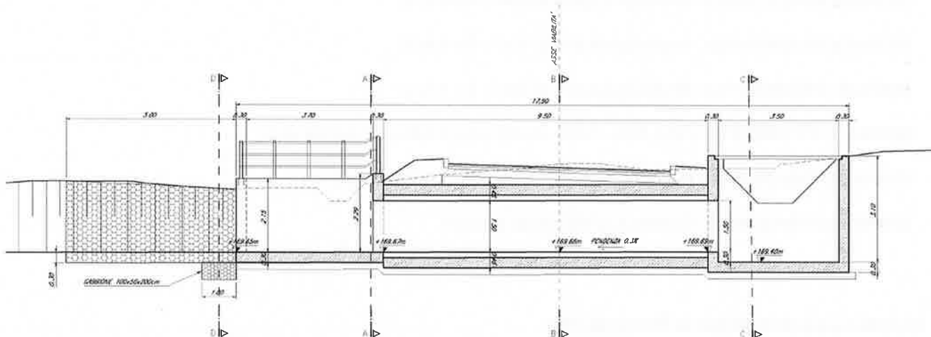
FIGURA 3-1: SEZIONE LONGITUDINALE TIPOLOGICA
