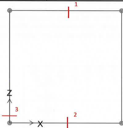
FIGURA 7-23: SEZIONI DI CALCOLO PER LE VERIFICHE A FESSURAZIONE
