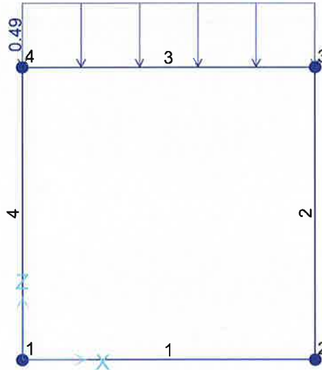
FIGURA 7-8: AZIONE STATICA EQUIVALENTE SISMA VERTICALE (SISMA_V)
