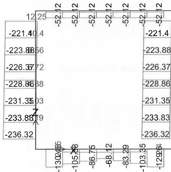
FIGURA 7-12: SFORZO NORMALE - INVILUPPO SLU/SLV
