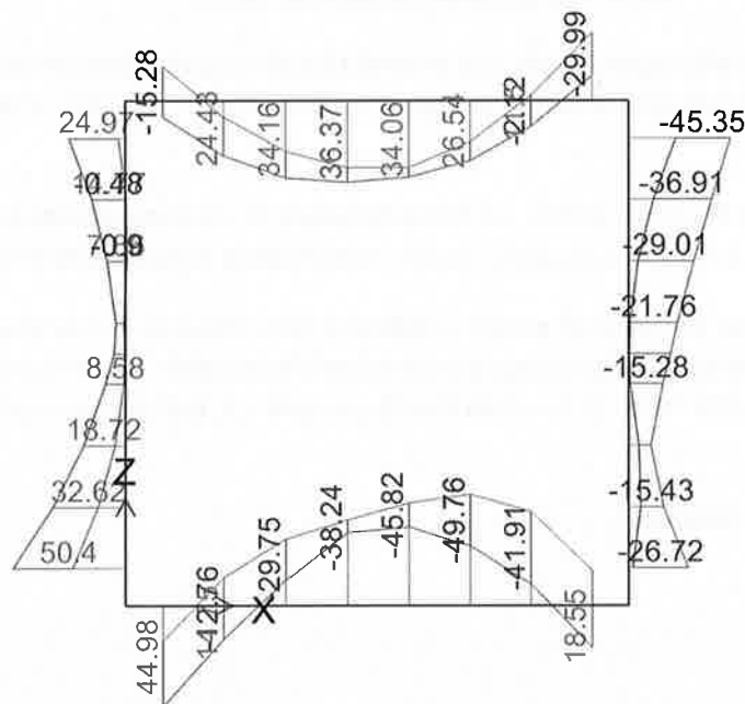
FIGURA 7-22: MOMENTO FLETTENTE - INVILUPPO SLE-RARA
