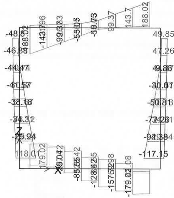
FIGURA 7-13: TAGLIO - INVILUPPO SLU/SLV
