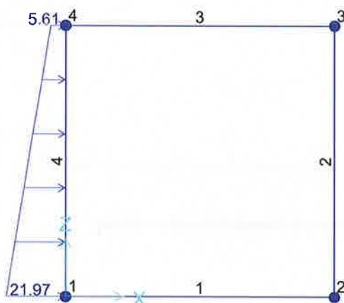
FIGURA 7-3: CARICO CONCENTRATO DOVUTO ALLA SPINTA DEL TERRENO (SPTSX)
