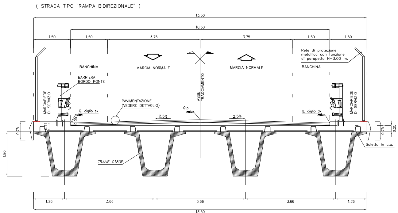
Sezione trasversale TIPO
