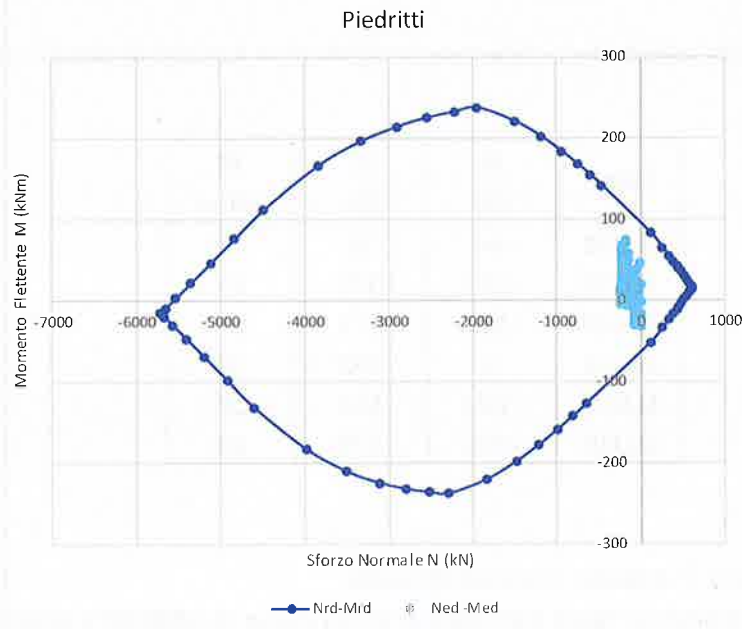
FIGURA 7-18: DOMINIO DI INTERAZIONE M-N PIEDRITTI
