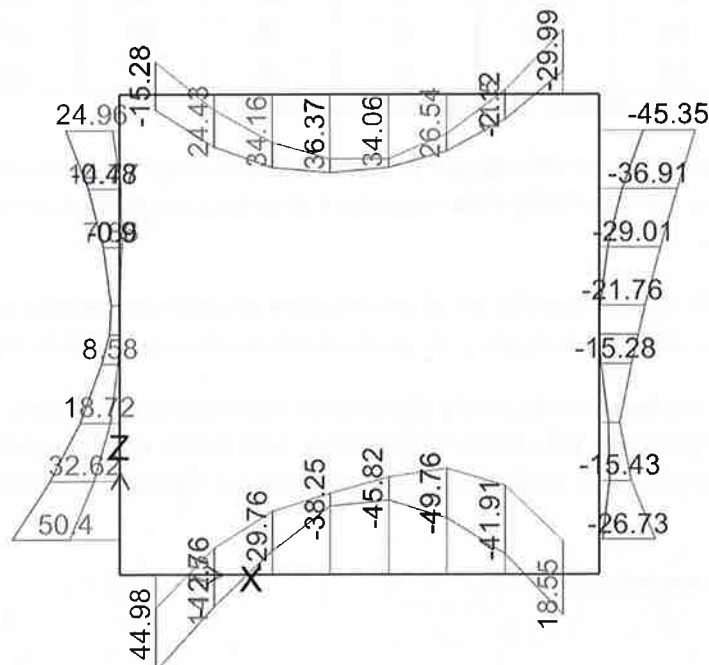
FIGURA 7-22: MOMENTO FLETTENTE - INVILUPPO SLE-RARA
