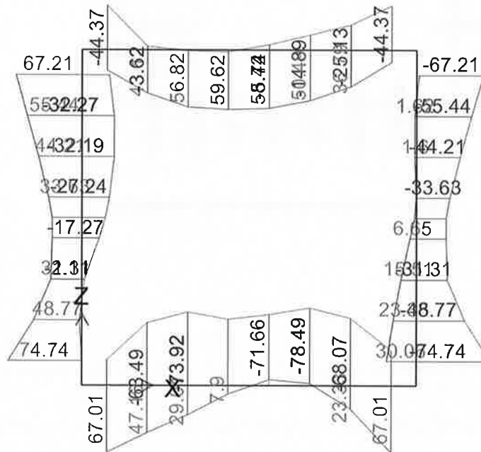
FIGURA 7-14: MOMENTO FLETTENTE - INVILUPPO SLU/SLV
