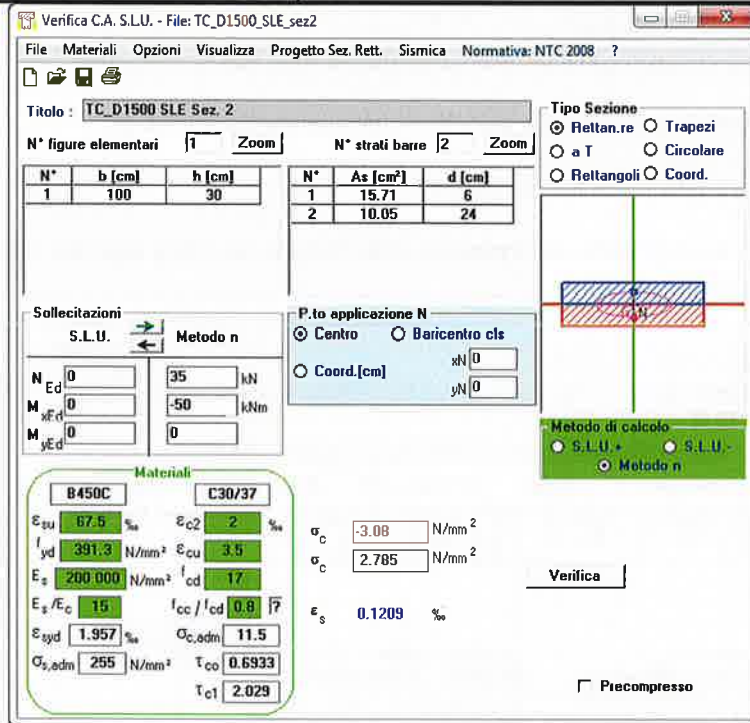
FIGURA 7-26: CALCOLO MASSIMA TENSIONE DI TRAZIONE NEL CALCESTRUZZO PER LA SEZIONE 2
