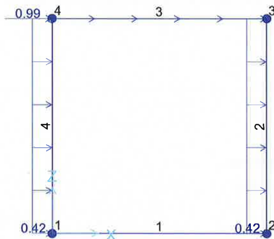
FIGURA 7-7: AZIONE STATICA EQUIVALENTE SISMA ORIZZONTALE (SISMA_H)
