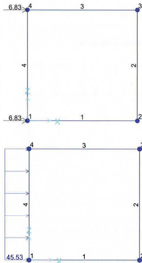
FIGURA 7-6: SOVRASPINTA DOVUTA AL CARICO FERROVIARIO (SPACCSX)
