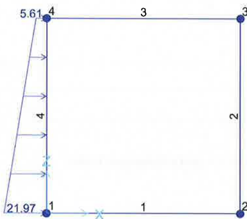
FIGURA 7-3: CARICO CONCENTRATO DOVUTO ALLA SPINTA DEL TERRENO (SPTSX)
