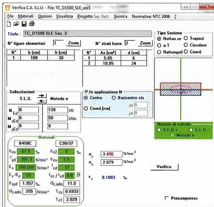
FIGURA 7-27: CALCOLO MASSIMA TENSIONE DI TRAZIONE NELLE BARRE PER LA SEZIONE 3
