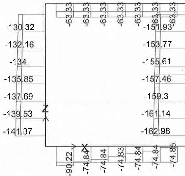
FIGURA 7-21: SFORZO NORMALE - INVILUPPO SLE-RARA
