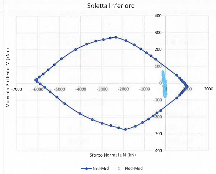
FIGURA 7-20: DOMINIO DI INTERAZIONE M-N SOLETTA INFERIORE
