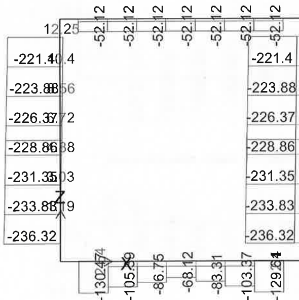
FIGURA 7-12: SFORZO NORMALE - INVILUPPO SLU/SLV
