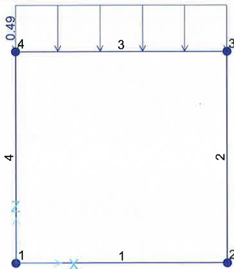
FIGURA 7-8: AZIONE STATICA EQUIVALENTE SISMA VERTICALE (SISMA_V)
