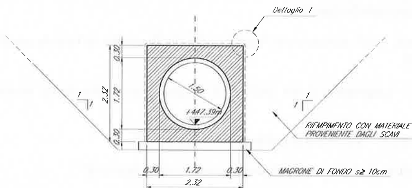
FIGURA 3-2: SEZIONE TRASVERSALE TIPOLOGICA
