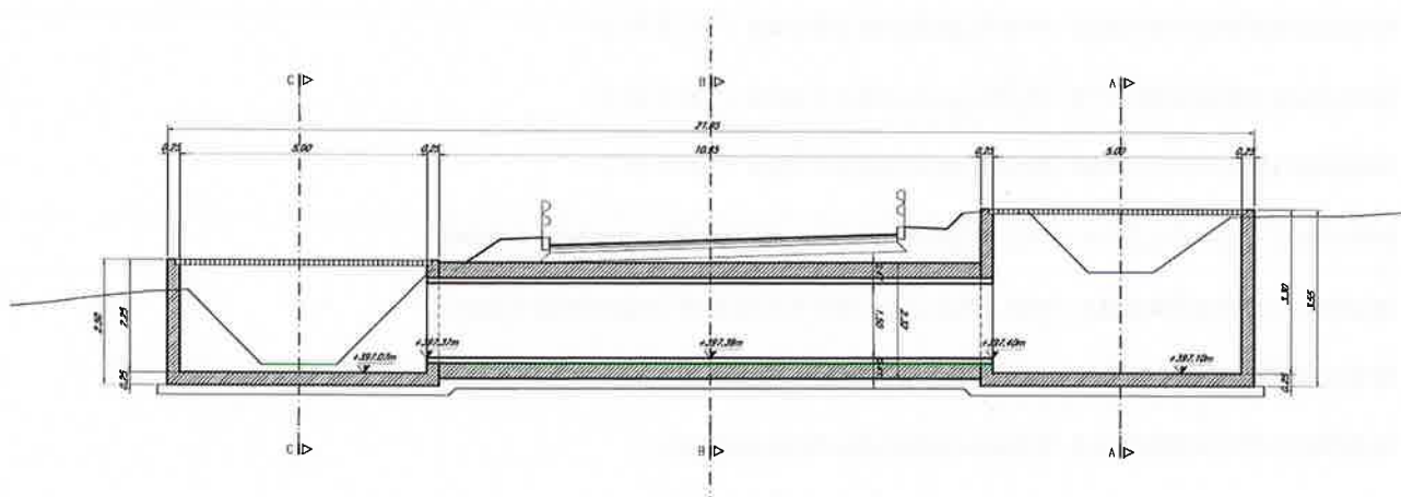
FIGURA 3-1: SEZIONE LONGITUDINALE TIPOLOGICA
