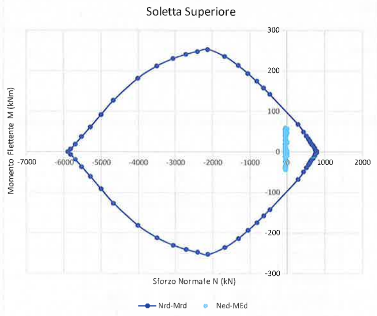
FIGURA 7-16: DOMINIO DI INTERAZIONE M-N SOLETTA SUPERIORE
