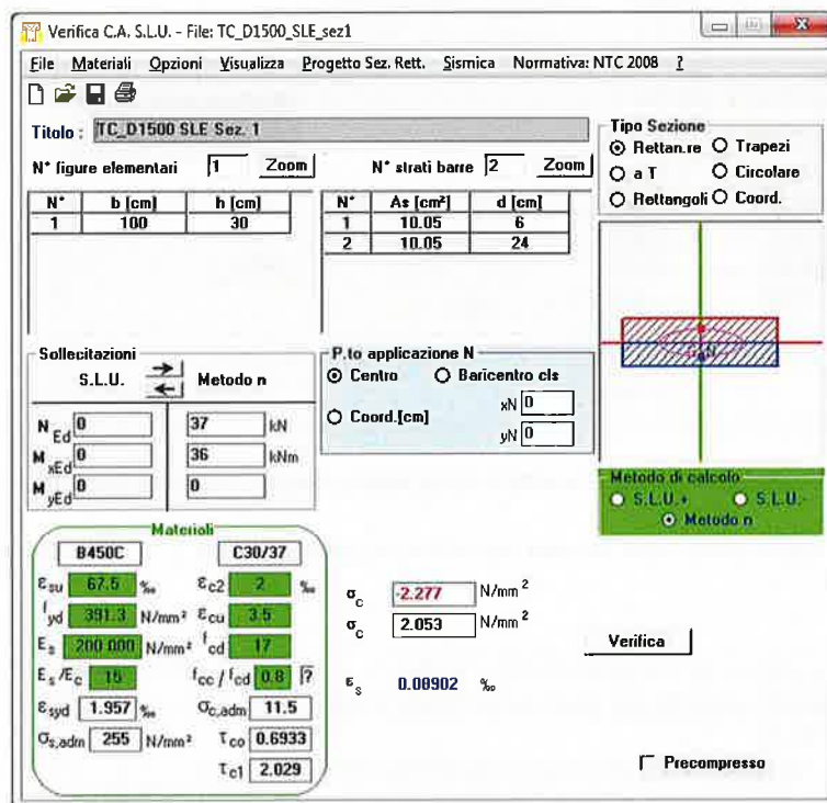
FIGURA 7-25: CALCOLO MASSIMA TENSIONE DI TRAZIONE NEL CALCESTRUZZO PER LA SEZIONE 1
