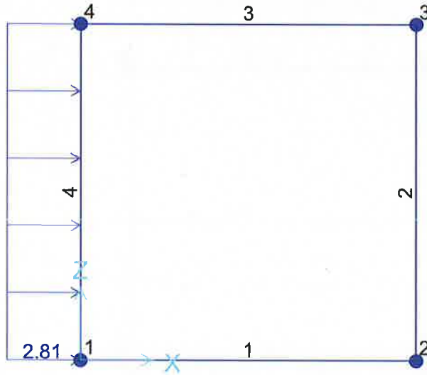
FIGURA 7-9: SPINTA DEL TERRENO IN FASE SISMICA
