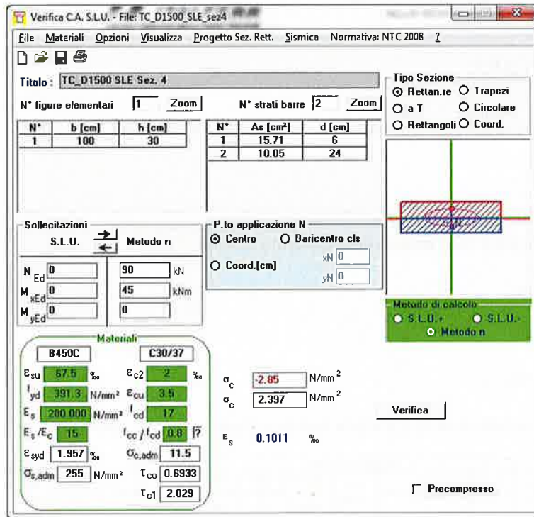
FIGURA 7-28: CALCOLO MASSIMA TENSIONE DI TRAZIONE NEL CALCESTRUZZO PER LA SEZIONE 4
