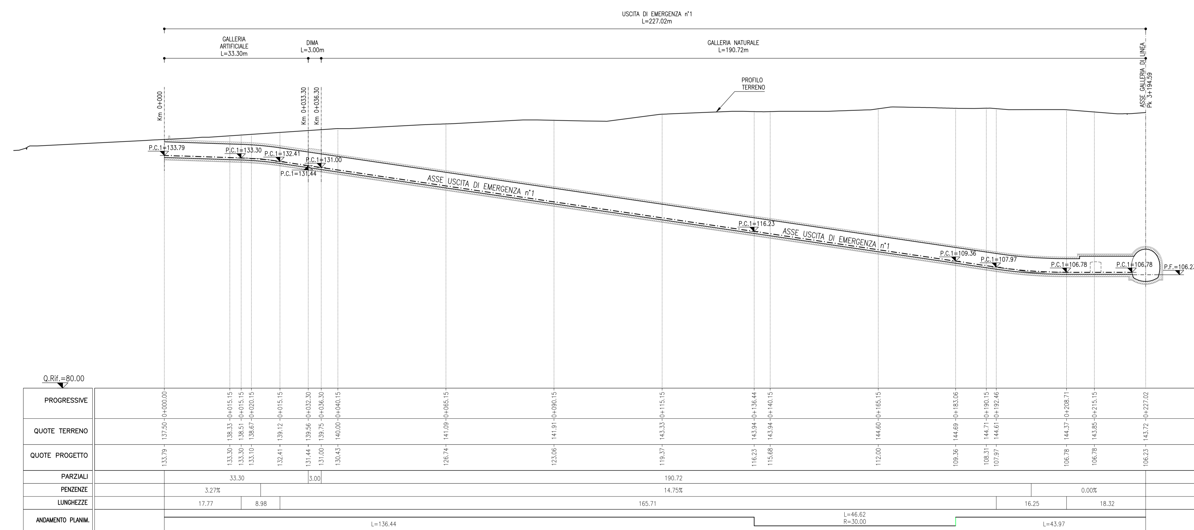
PROFILO LONGITUDINALE SCALA 1:500 USCITA DI EMERGENZA n°1 Pk 3+194.59
